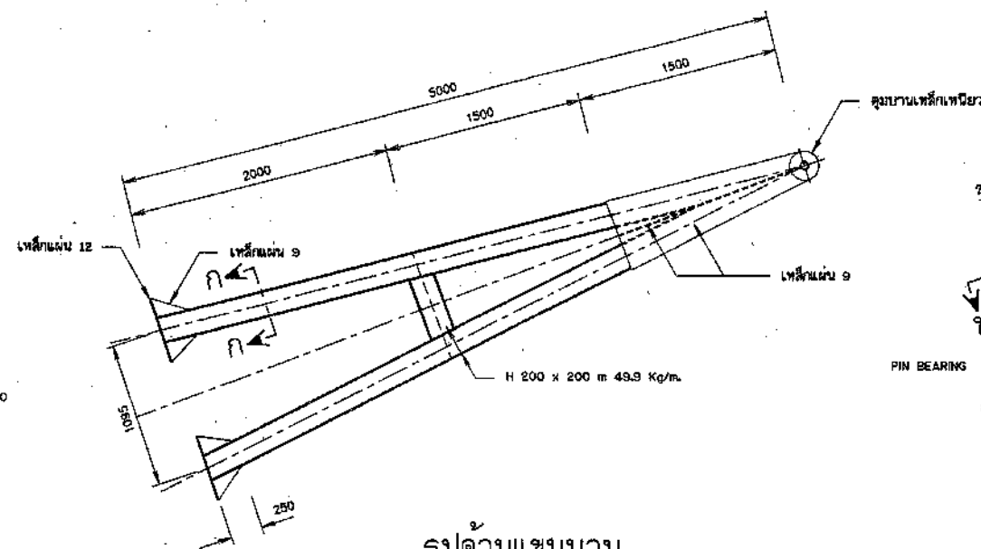
รูปด้านแขนบาน
