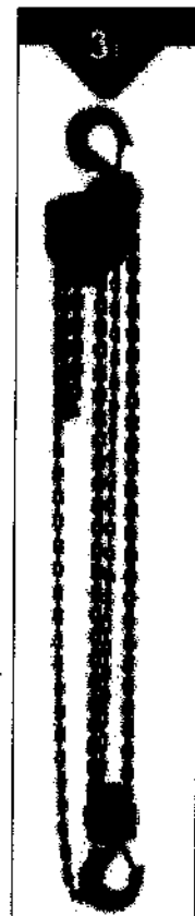
จอกโซ่มือสาว ขนาด 3 ตัน น้ำหนักยก 3(ตัน) Test Load 4.75(ตัน) ยกลูก 3(เมตร) จำนวนทาบโซ่ 2 โซ่ยก 7.1 x 21 โซ่ดึง 5.0 x 22.8 ระยะห่างระหว่างตะขอ 475 (mm) น้ำหนักจอก 23.0 (kg) การออกแรงยก 35 kgf
