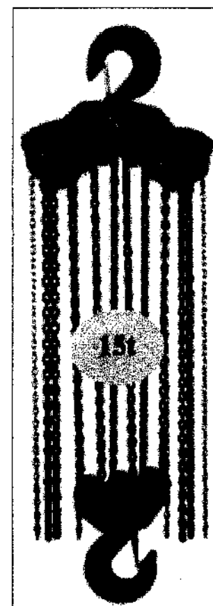
จอกโซ่มือสาว ขนาด 15 ตัน น้ำหนักยก 15(ตัน) Test Load 20(ตัน) ยกลูก 3.5(เมตร) จำนวนทาบโซ่ 6 โซ่ยก 9.0 x 27 โซ่ดึง 5.5 x 23.6 ระยะห่างระหว่างตะขอ 850 (mm) น้ำหนักจอก 150.0 (kg) การออกแรงยก 41 x 2 kgf
