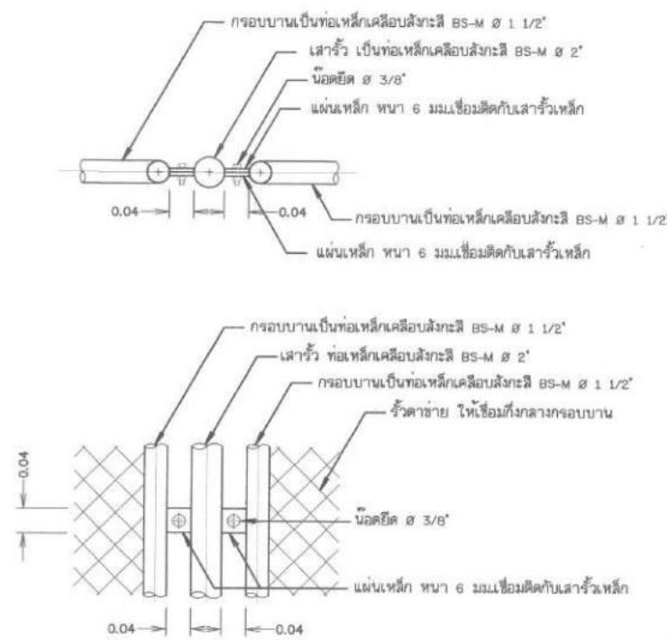
แบบขยายบานพับหัวเหล็ก ไม่แสดงมาตรฐาน
