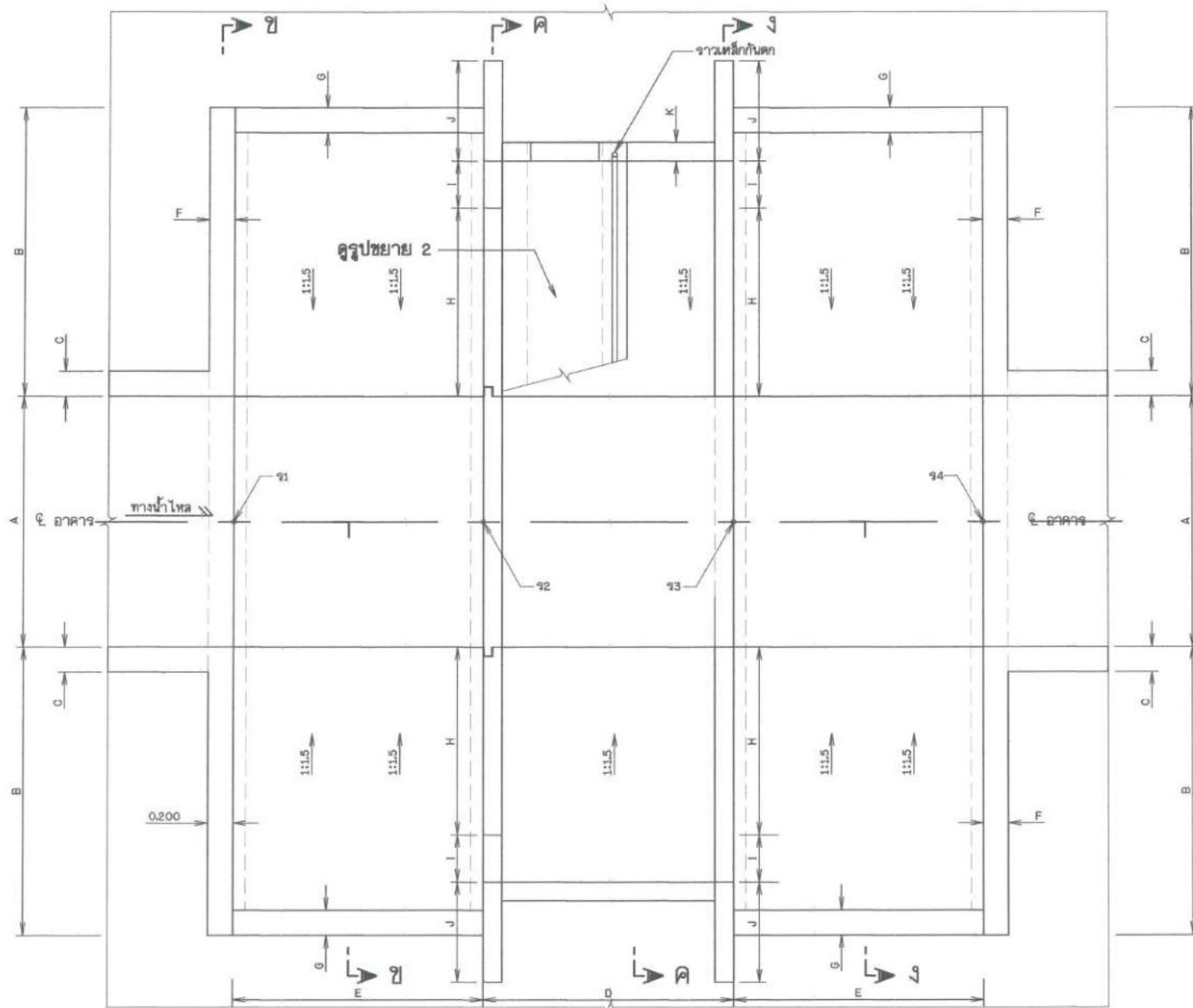
แปลนอาคารอัดน้ำ
