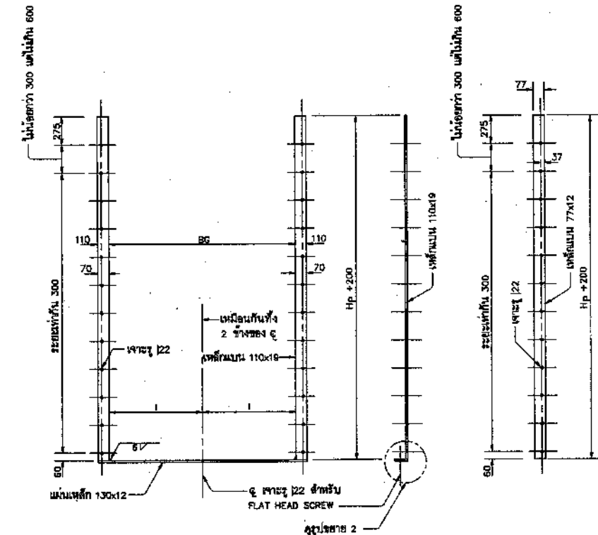
กรอบบาน เหล็กเหล็กรัด ไม่แสดงขนาดส่วน
