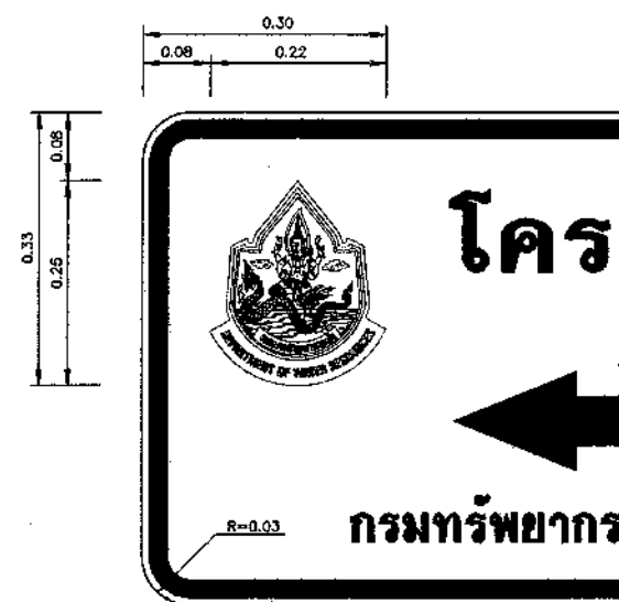
ป้ายแนะนำโครงการ มาตรฐาน 1:10
