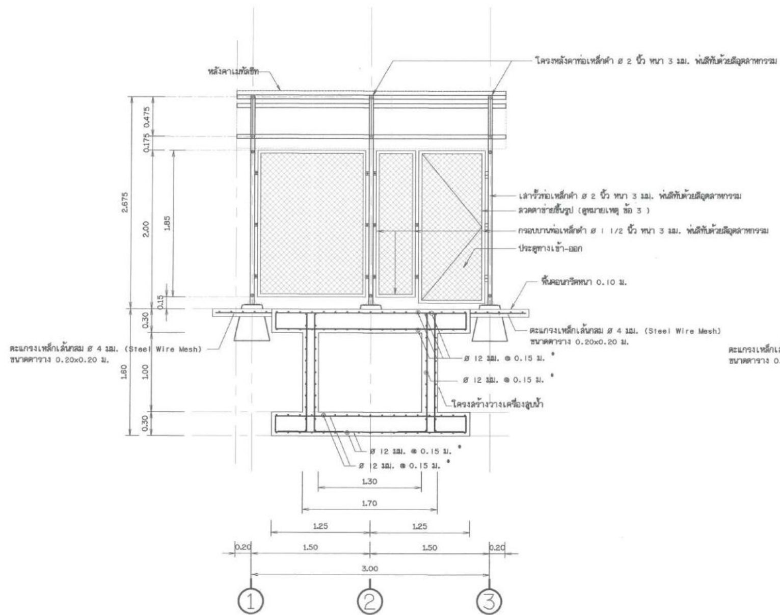
รูปตัด ก - ก ไม่แสดงขนาดจั่วส่วน
