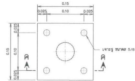
รูปขยายแผ่นเหล็กหน้าแปลน มาตรฐาน 1:10
