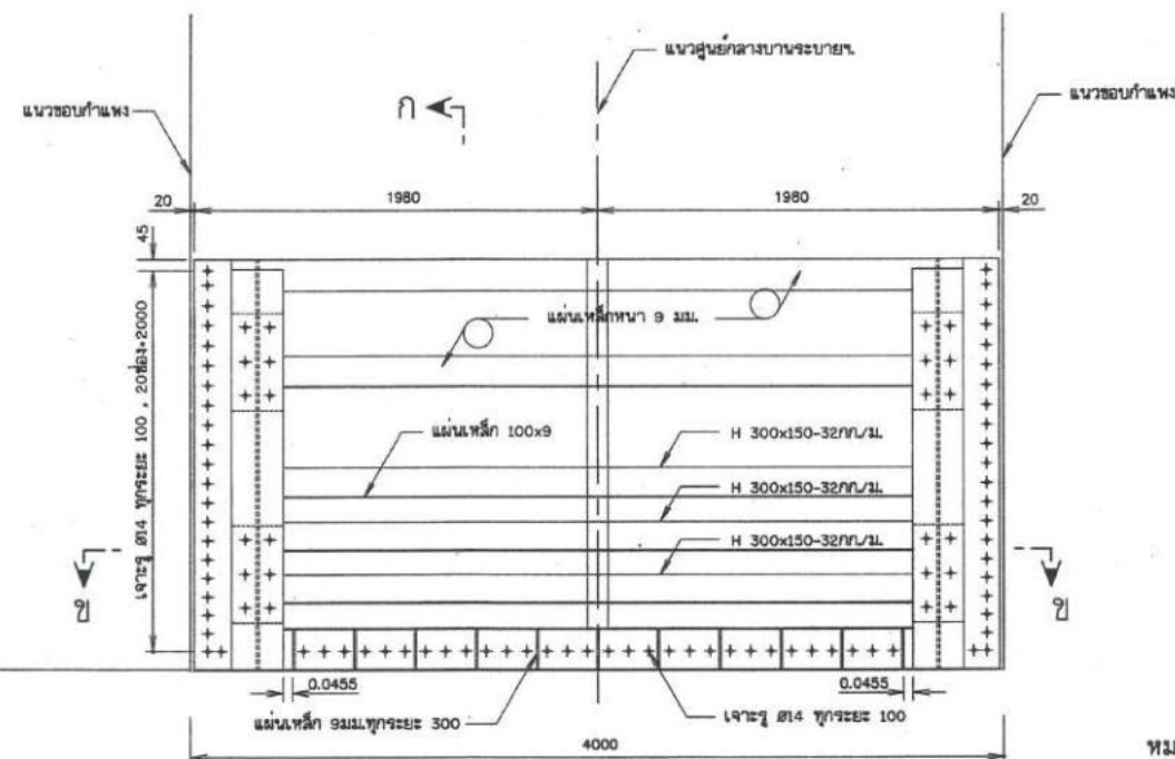
บ้านระบายด้านท้ายน้ำ
