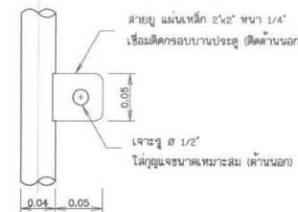
แบบขยายสายยู ไม่แสดงมาตรฐาน
