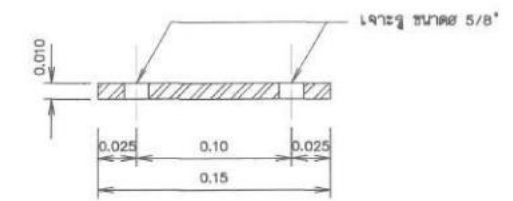
รูปตัด ค-ค มาตรฐาน 1:10
