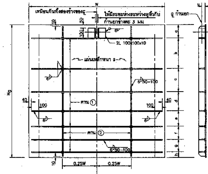
ตัวบานแบบ ข เหล็กเหล็กรัด ไม่แสดงขนาดส่วน
