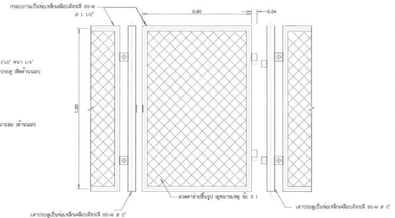
แบบขยายรายละเอียดประตู ไม่แสดงมาตรฐาน
