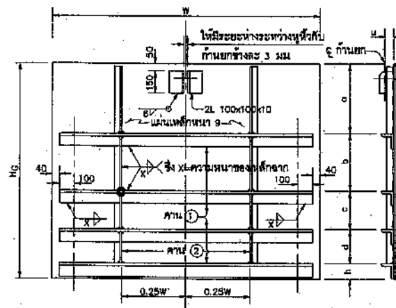
ตัวบานแบบ ก เหล็กเหล็กรัด ไม่แสดงขนาดส่วน
