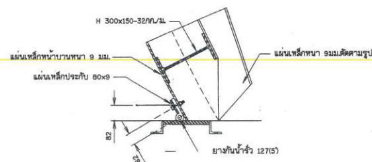
รูปขยายยางกันน้ำรั่วใต้บ้าน
