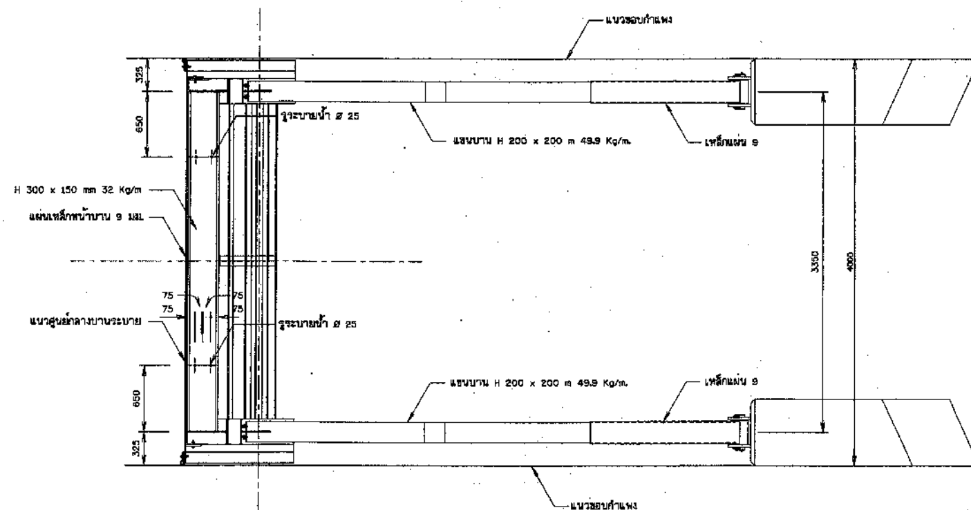
แปลนแขนบาน
