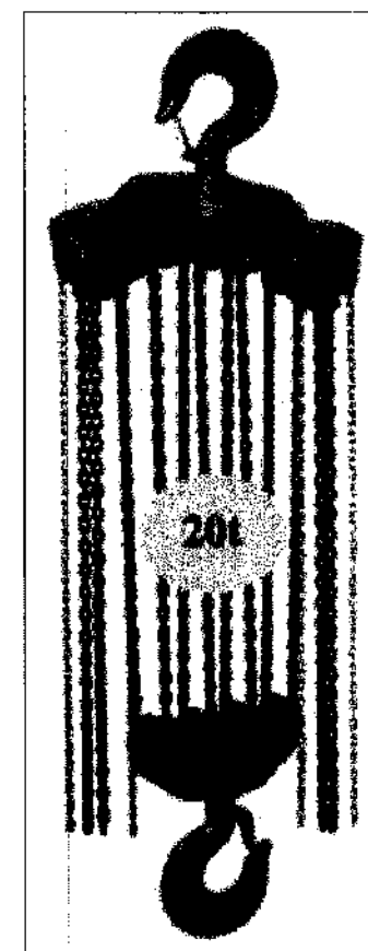
จอกโซ่มือสาว ขนาด 20 ตัน น้ำหนักยก 20(ตัน) Test Load 25(ตัน) ยกลูก 3.5(เมตร) จำนวนทาบโซ่ 8 โซ่ยก 9.0 x 27 โซ่ดึง 5.5 x 23.6 ระยะห่างระหว่างตะขอ 870 (mm) น้ำหนักจอก 190.0 (kg) การออกแรงยก 41 x 2 kgf
