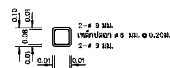
รูปตัด ข-ข มาตรฐาน 1:10
