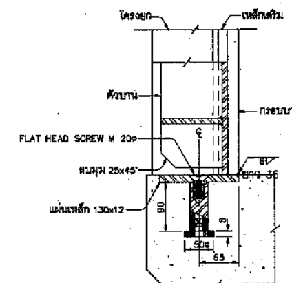
รูปขยาย 2 ไม่แสดงขนาดส่วน
