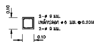
รูปตัด ก-ก มาตรฐาน 1:10
