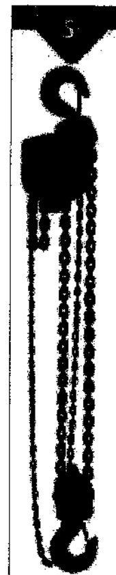
จอกโซ่มือสาว ขนาด 5 ตัน น้ำหนักยก 5(ตัน) Test Load 6.3(ตัน) ยกลูก 3(เมตร) จำนวนทาบโซ่ 2 โซ่ยก 9.0 x 27 โซ่ดึง 5.5 x 23.6 ระยะห่างระหว่างตะขอ 635 (mm) น้ำหนักจอก 41.0 (kg) การออกแรงยก 39 kgf
