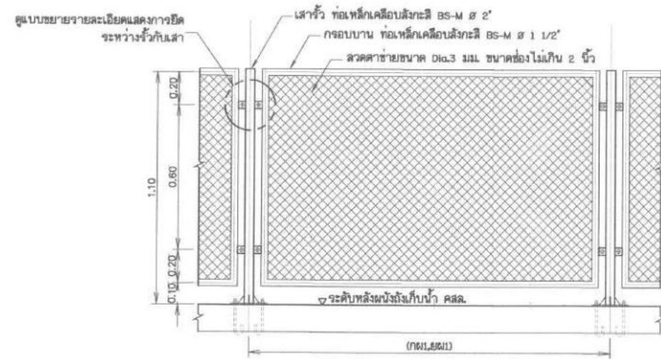
แบบขยายราวกันตก สำหรับบันไดบ้าน คสล. แบบไม่มีฝ้า
