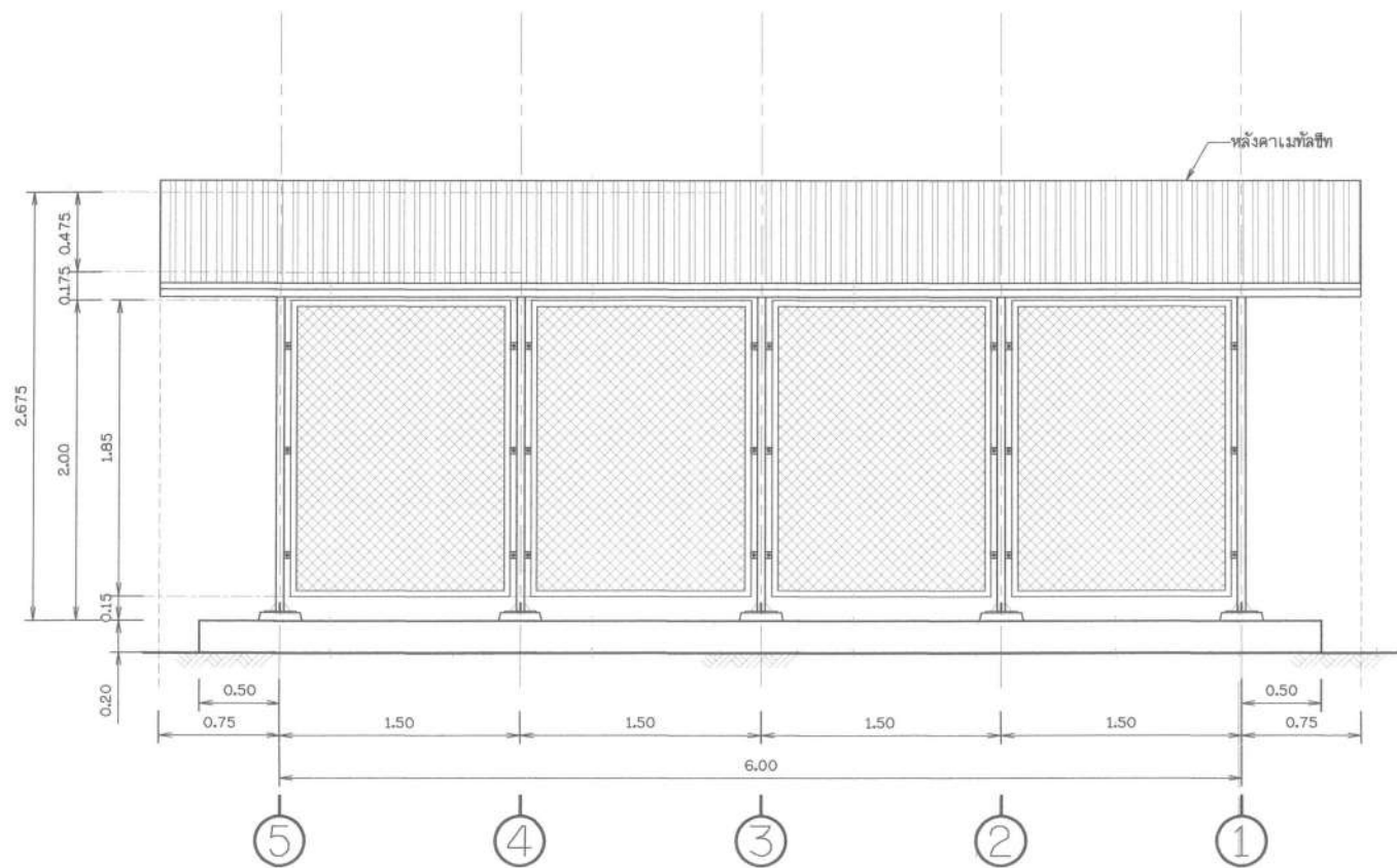
รูปด้าน 3 โมเดลตามมาตรฐาน
