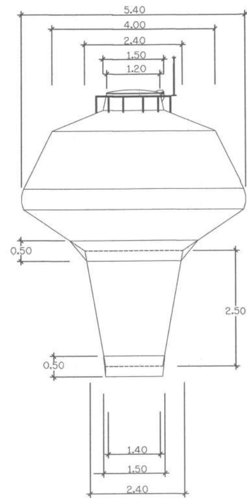
แบบขยายแมนโฮลบนถังแฉมแปญ
