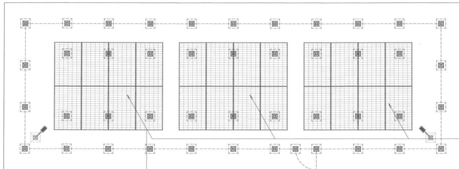
แผนการติดตั้งแผงเซลล์แสงอาทิตย์ ขนาด 7.5 กิโลวัตต์ พร้อมรั้ว
