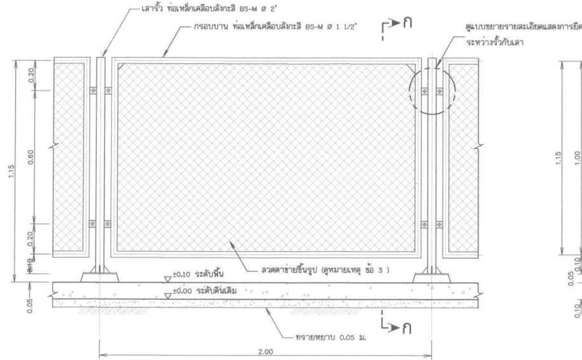
แบบขยายรื้อลวดตาข่าย
