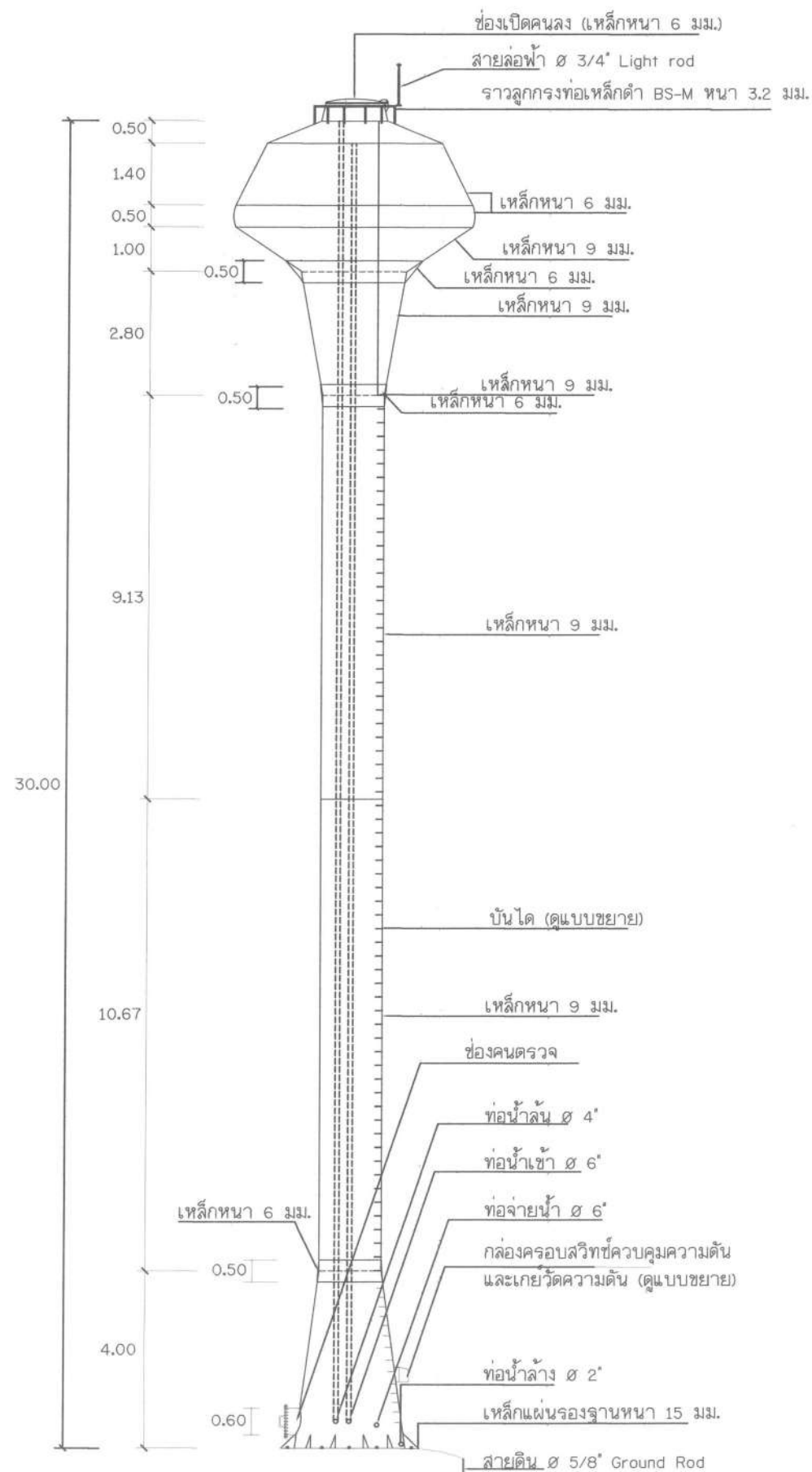
รูปด้านข้างหอถังสูง แบบถังเหล็กรูปทรงถ้วยแฉมแปญ
