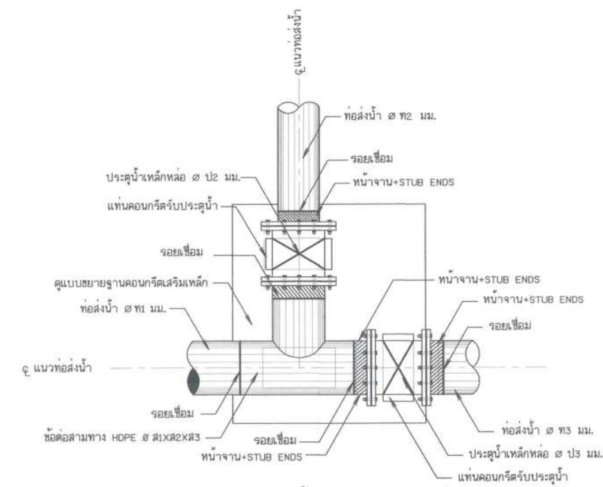
รูปขยายการติดตั้งอาคารจตุรแฉก
