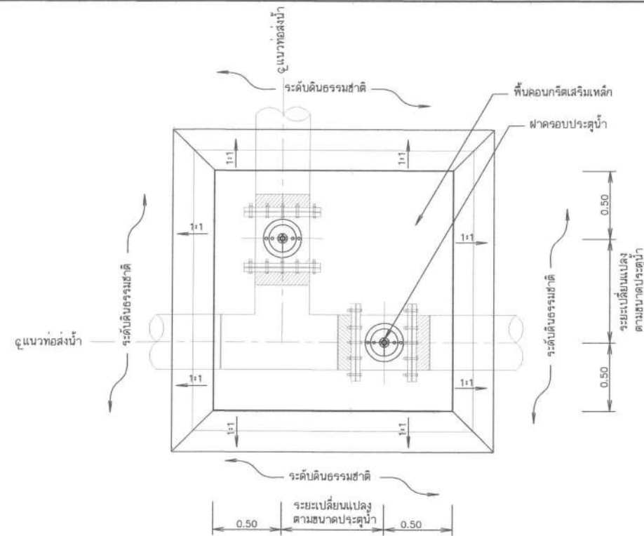
แปลนอาคารจตุรแฉก
