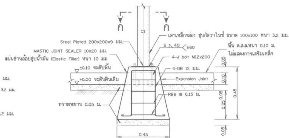
รูปขยายฐานรากโครงสร้างรับแผง F1 (ค่อม คสล. หล่อสำเร็จรูปพร้อมติดตั้ง) ไม่แสดงมาตราส่วน
