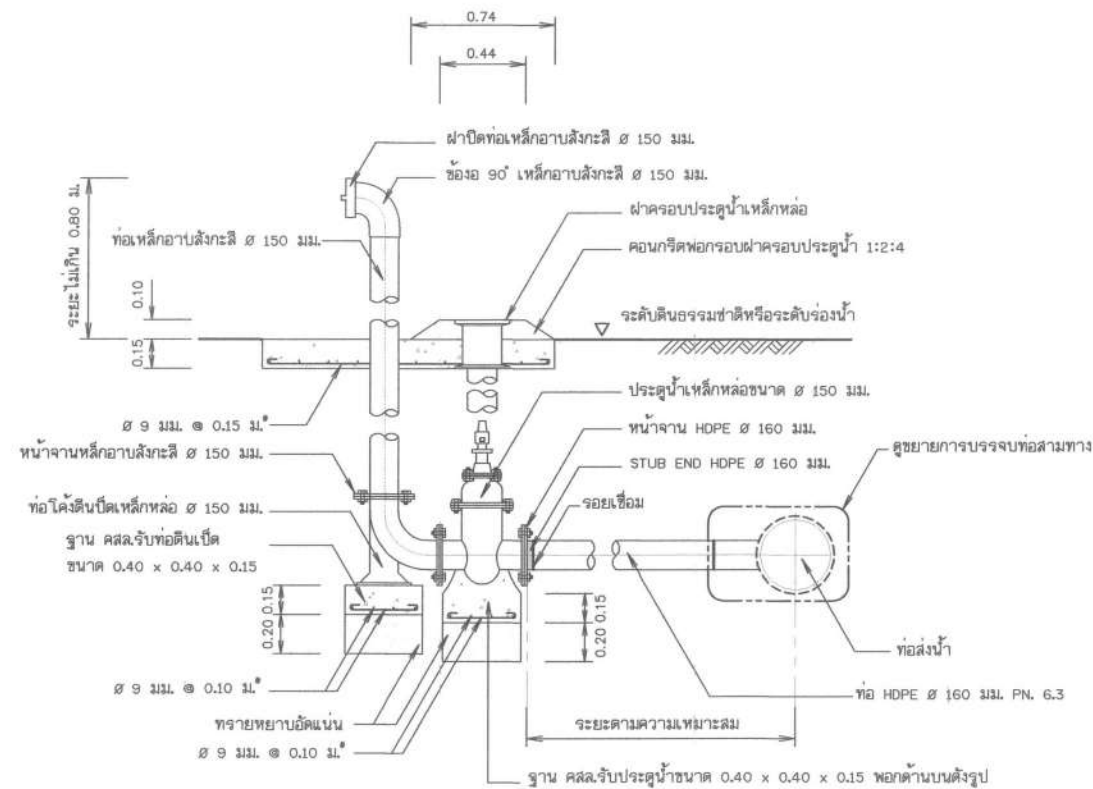
รูปตัด ก - ก แสดงการติดตั้งประตูลอยตะกอน
