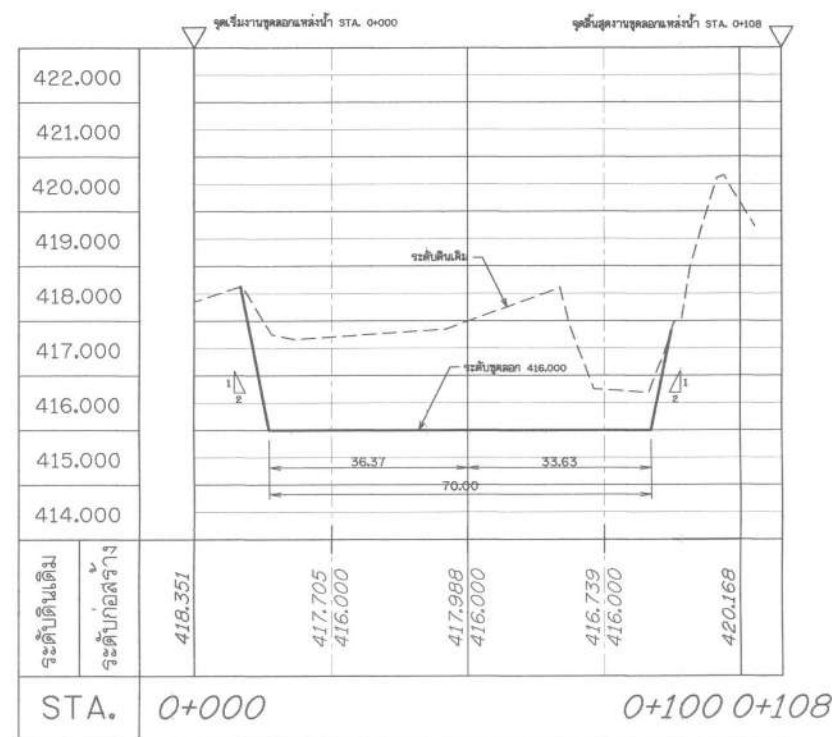
รูปตัดตามแนวยาว ไม่แสดงค่าพิกัด
