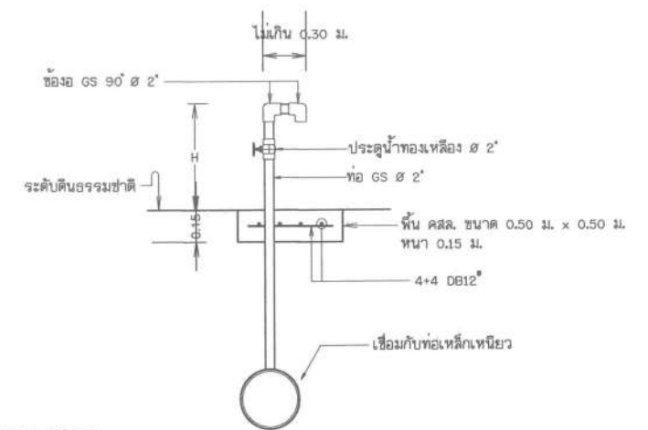
ก๊อกน้ำสำหรับล้างแผง มาตราส่วน 1 : 20
