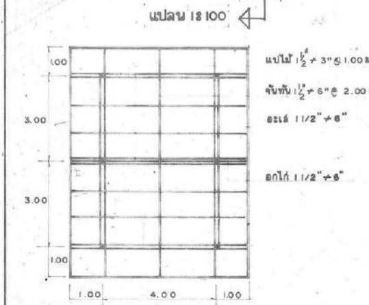
แปลนโครงหลังคา 18100
