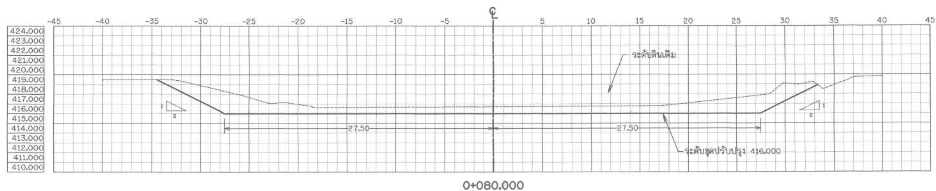
รูปตัดแสดงงานดิน
