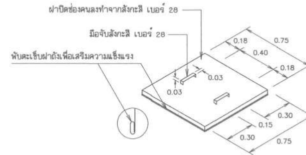
ขยายแปลนช่องคนลง มาตราส่วน not to scale
