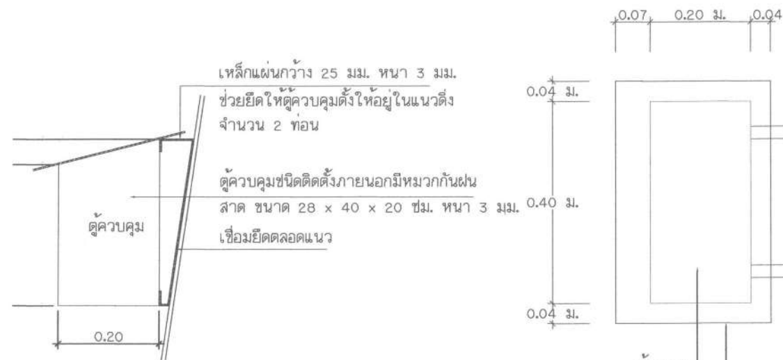
แบบขยายตุ้บคุม
