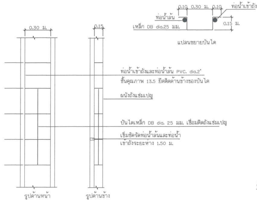
แบบขยายบันได และการยึดท่อน้ำขึ้นและท่อน้ำเข้าถึง
