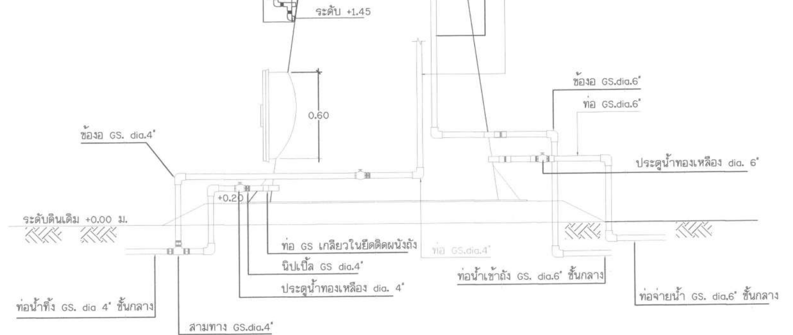
แบบแสดงการเดินท่อในถังแชมเปญ
