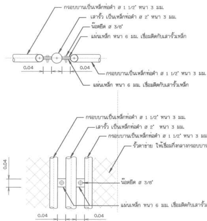
แบบขยายรายละเอียดแสดงการยึดระหว่างรั้วกับเล้า ไม่แสดงขนาดราส่วน
