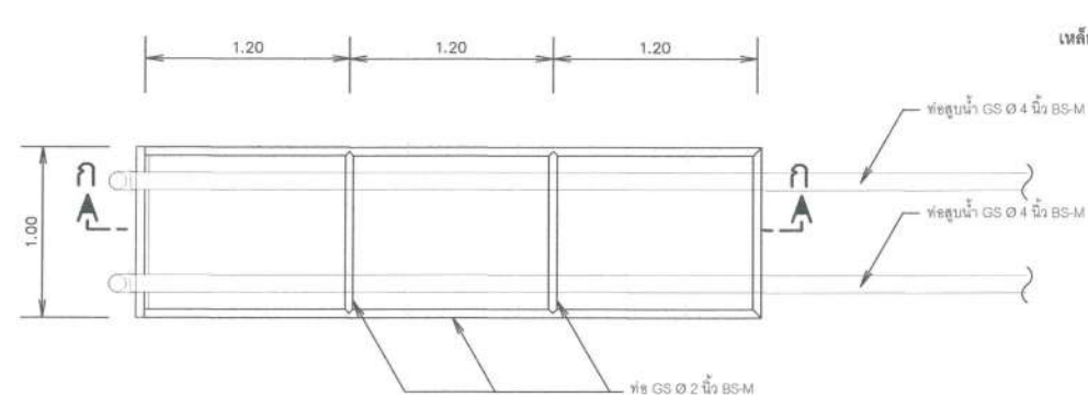
แปลนโครงสร้างรับท่อสูบน้ำ
