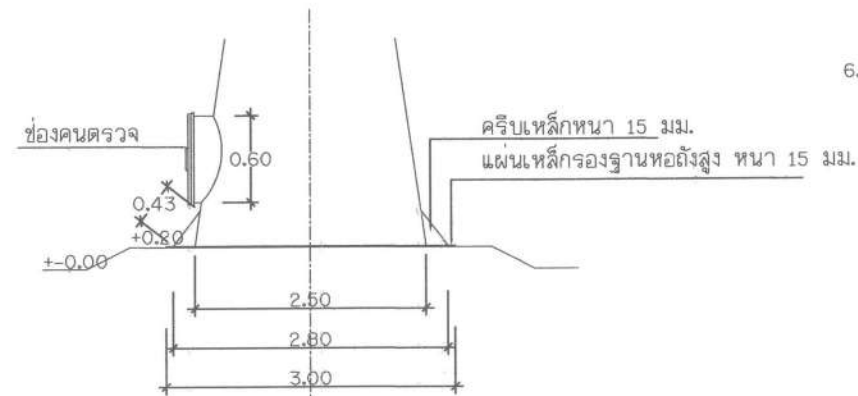
แบบขยายแมนโฮลล่างถังแฉมแปญ
