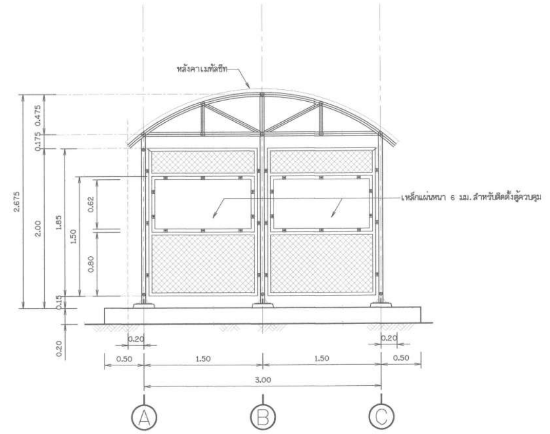
รูปด้าน 2 โมเดลตามมาตรฐาน
