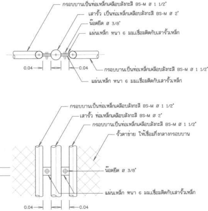
แบบขยายรายละเอียดแสดงการยึดระหว่างรื้อกับเสา
