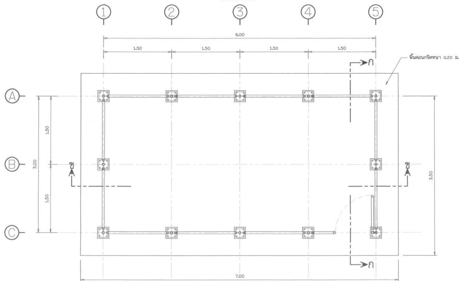
แปลนเสาและรื้อ
