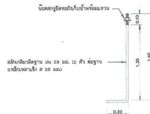
แบบขยายหลักเกิลียอดฐาน
