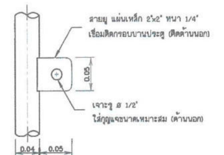
แบบขยายสายขู ไม่แสดงมาตราส่วน
