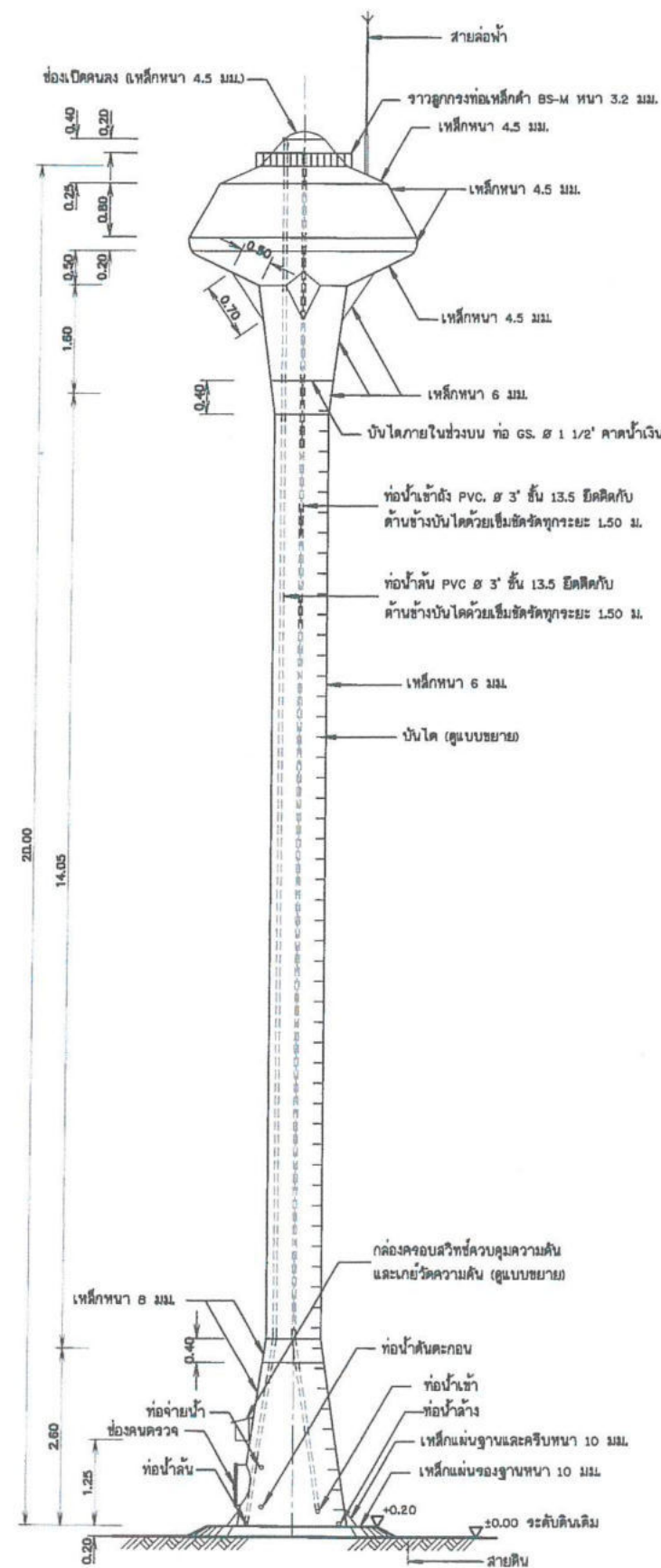
รูปด้านข้างหอถังสูง แบบถังเหล็กทรงกลมแป้น ไม่แสดงมาตราส่วน
