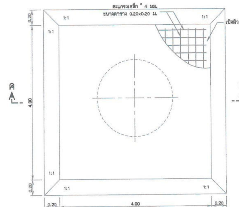
แปลงพื้นคอนกรีตเสริมเหล็ก
