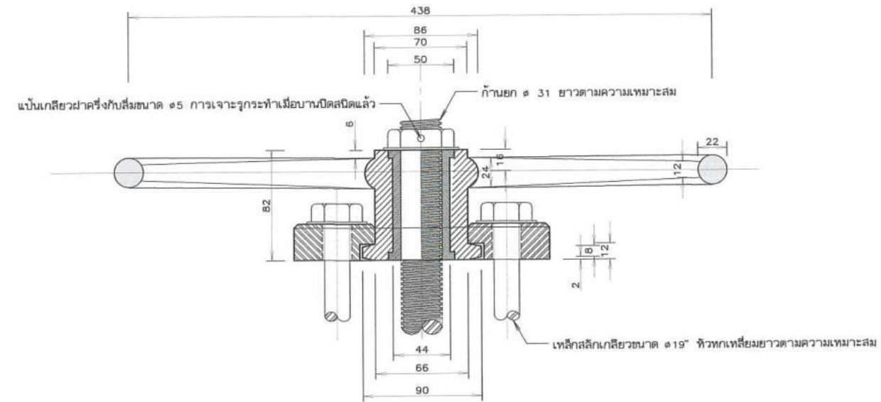
แสดงการติดตั้ง มาตราส่วน 1:2
