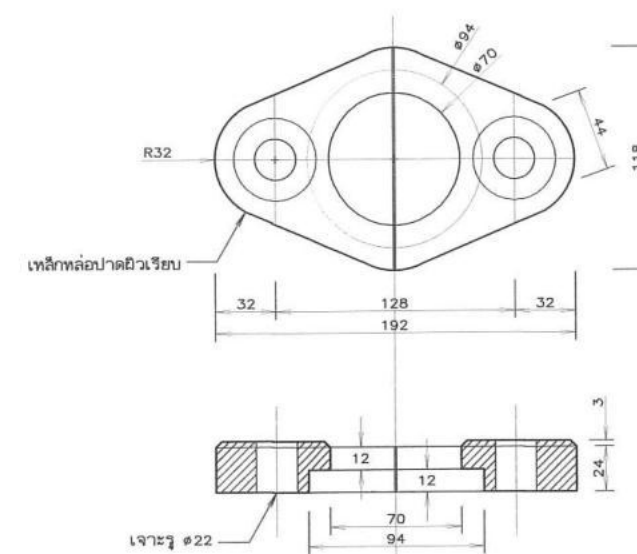
เหล็กหล่อ 1.5 กก. แผ่นปิด มาตราส่วน 1:2
