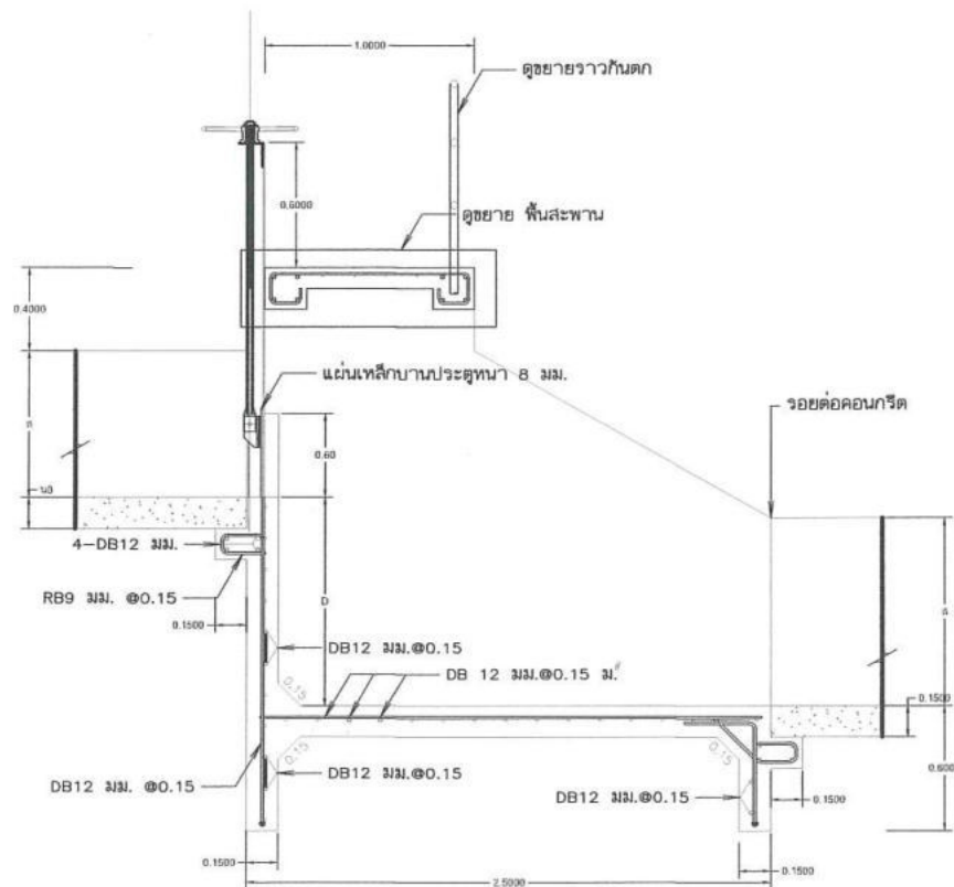
รูปตัดแนว ก - ก มาตราส่วน 1:20
