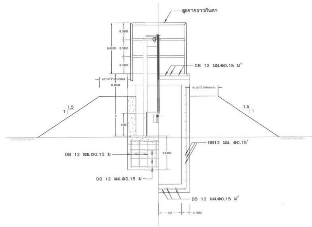
รูปตัดแนว ข - ข มาตราส่วน 1:20
