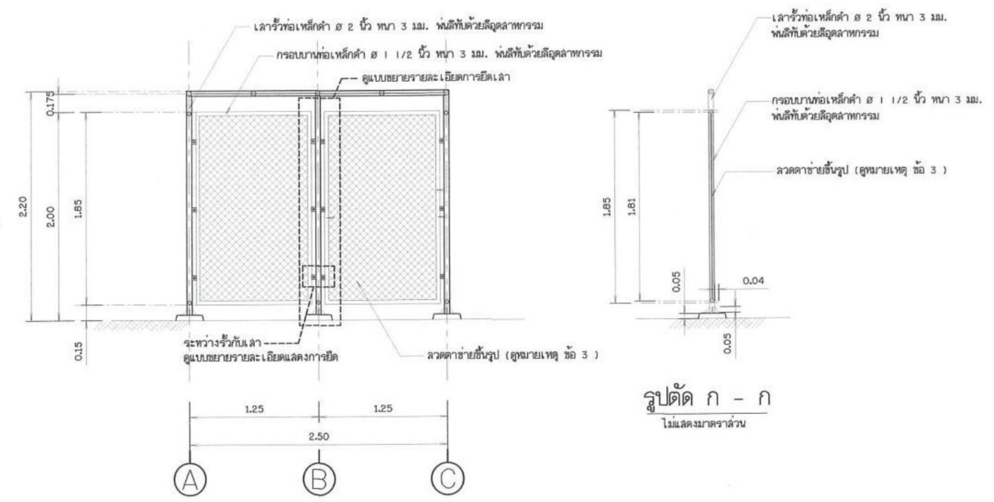
แบบขยายรั้ว 2 ไม่แสดงมาตราส่วน
