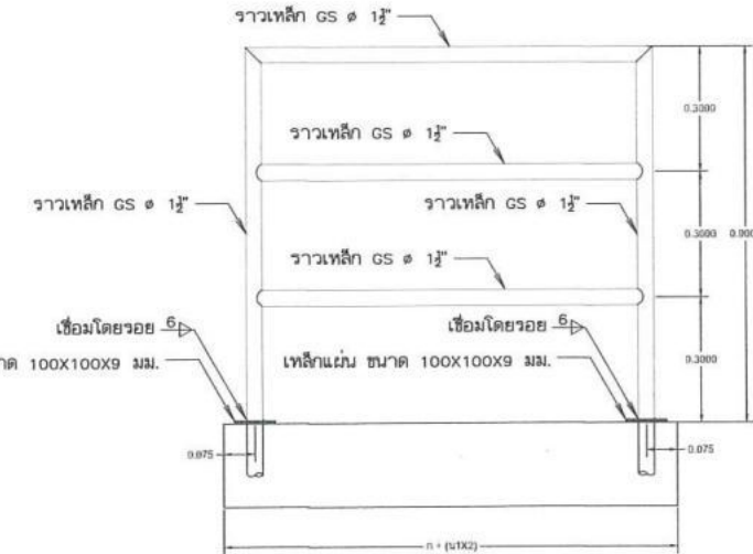
ขยายราวกันตก มาตราส่วน 1:10
