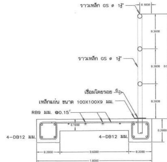
รูปตัดแนว A - A มาตราส่วน 1:10
