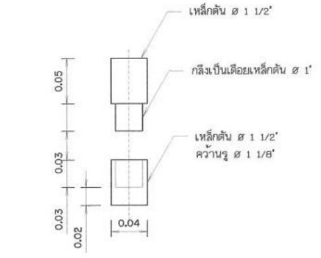
แบบขยายบานพับประตูเหล็ก ไม่แสดงมาตราส่วน
