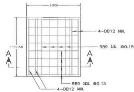
แปลนขยาย พื้นสะพาน มาตราส่วน 1:20
