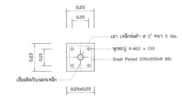
ฐานรากโครงสร้างอาคารคลุม ไม่แสดงมาตราส่วน
