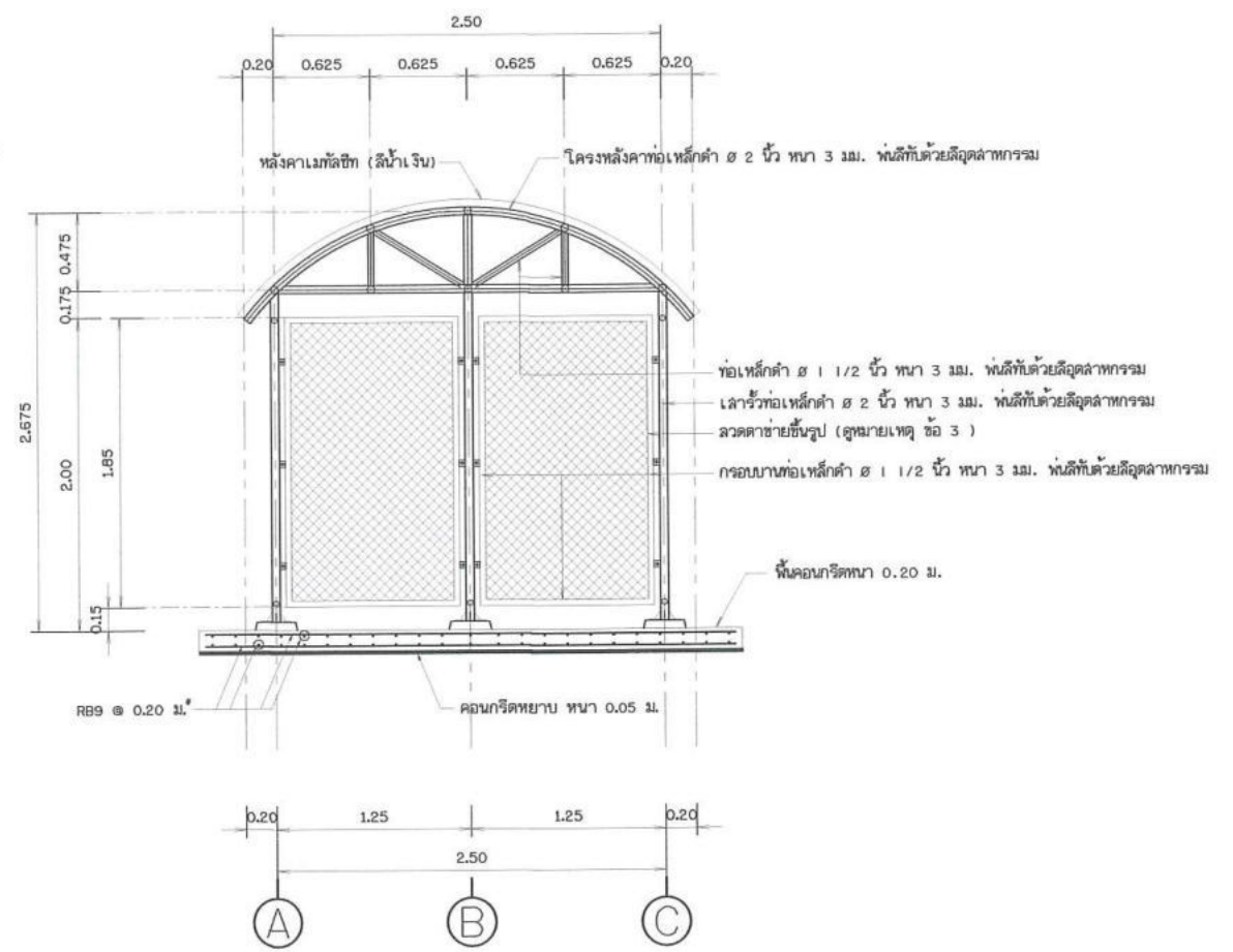
รูปตัด ข - ข โมเมนต์มาตรฐาน
