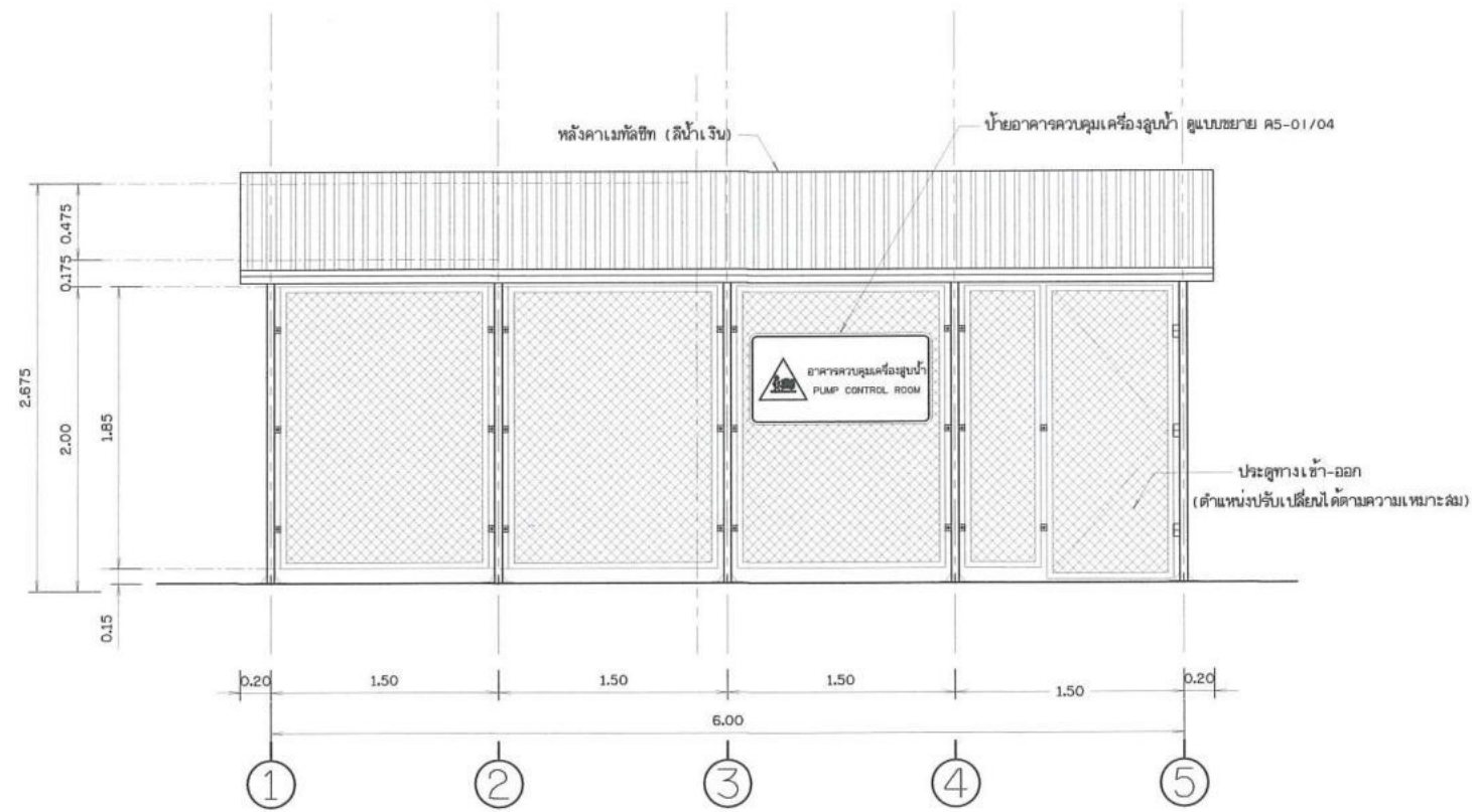
รูปด้าน 1 โมเดลขนาดจริง
