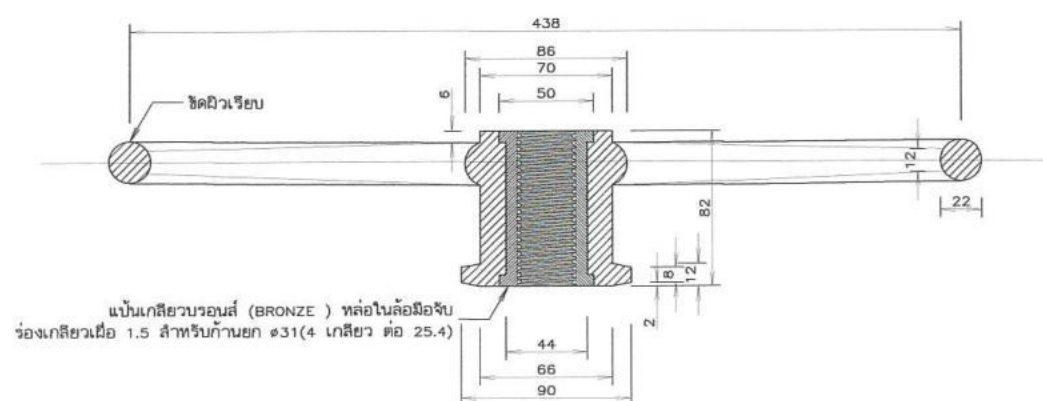
เหล็กหล่อและบรอนซ์ (PHOSPHOR BRONZE) 9.5 กก. ล้อยมือจับและแป้นเกลียวยก มาตราส่วน 1:2
