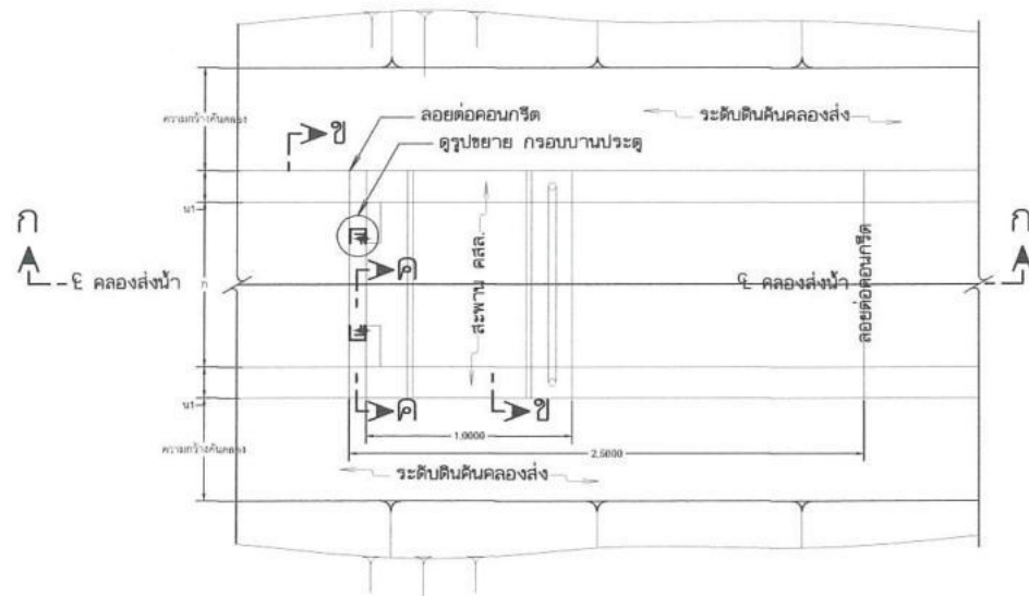
แปลนอาคารอัดน้ำลดระดับ มาตราส่วน 1:20
