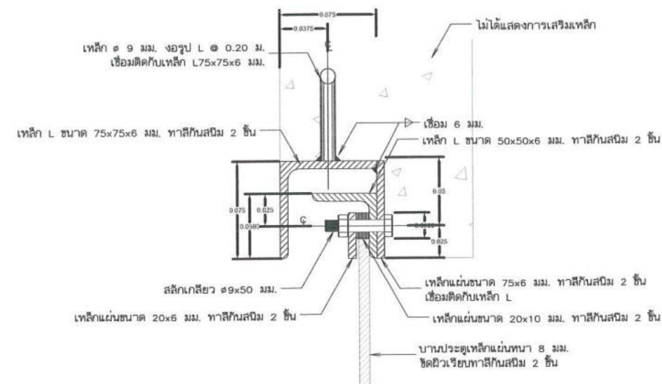
แบบขยาย แสดงการติดตั้งบานประตู
