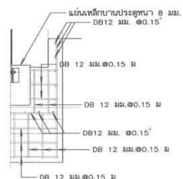
รูปตัดแนว ค - ค มาตราส่วน 1:20
