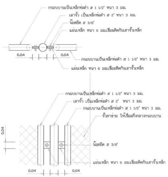
แบบขยายรายละเอียดแสดงการยึดระหว่างรั้วกับเล้า ไม่แสดงมาตราส่วน
