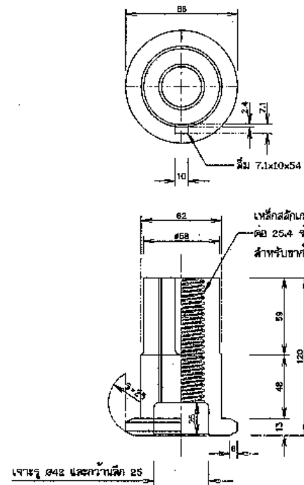
③ แป้นเกลียวยก มาตราส่วน 1:2 บรอนซ์ (BRONZE) ขัดผิวเรียบทั้งหมด
