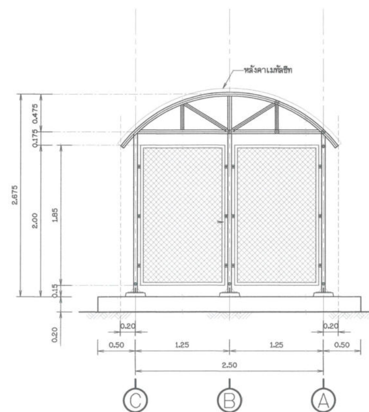
รูปด้าน 4 โมเดลขนาดจริง
