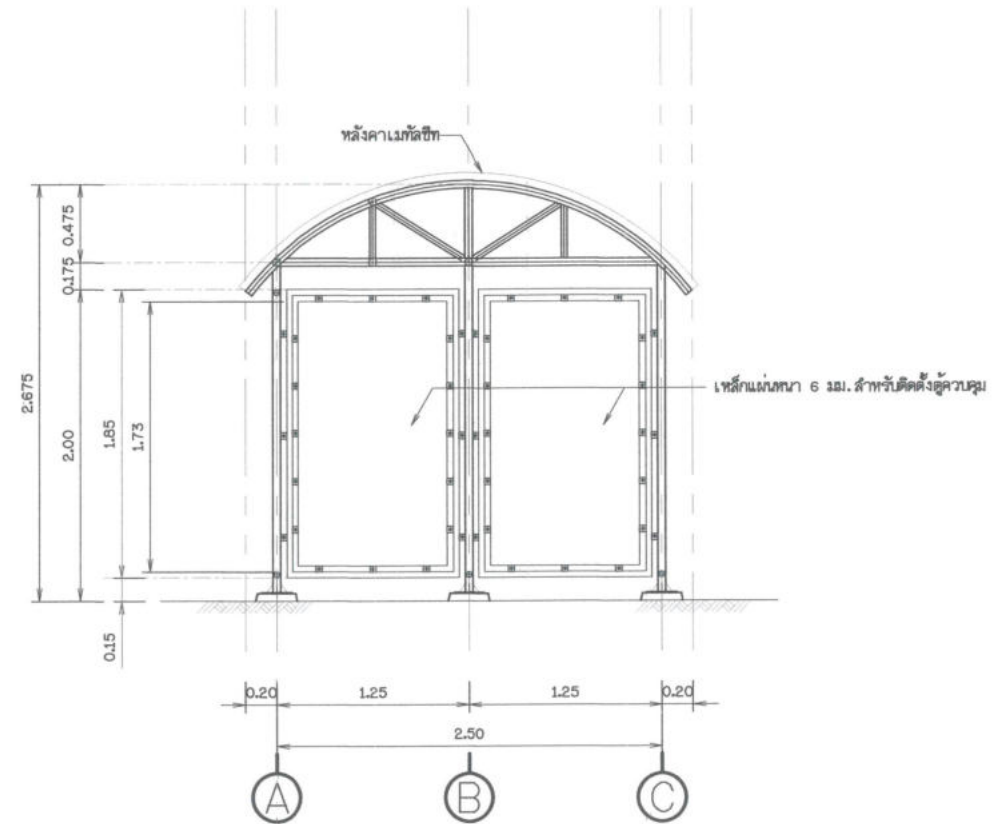
รูปด้าน 2 โมเมนต์มาตรฐาน
