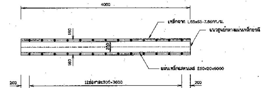
การติดตั้งเหล็กกรง มาตราส่วน 1:25
