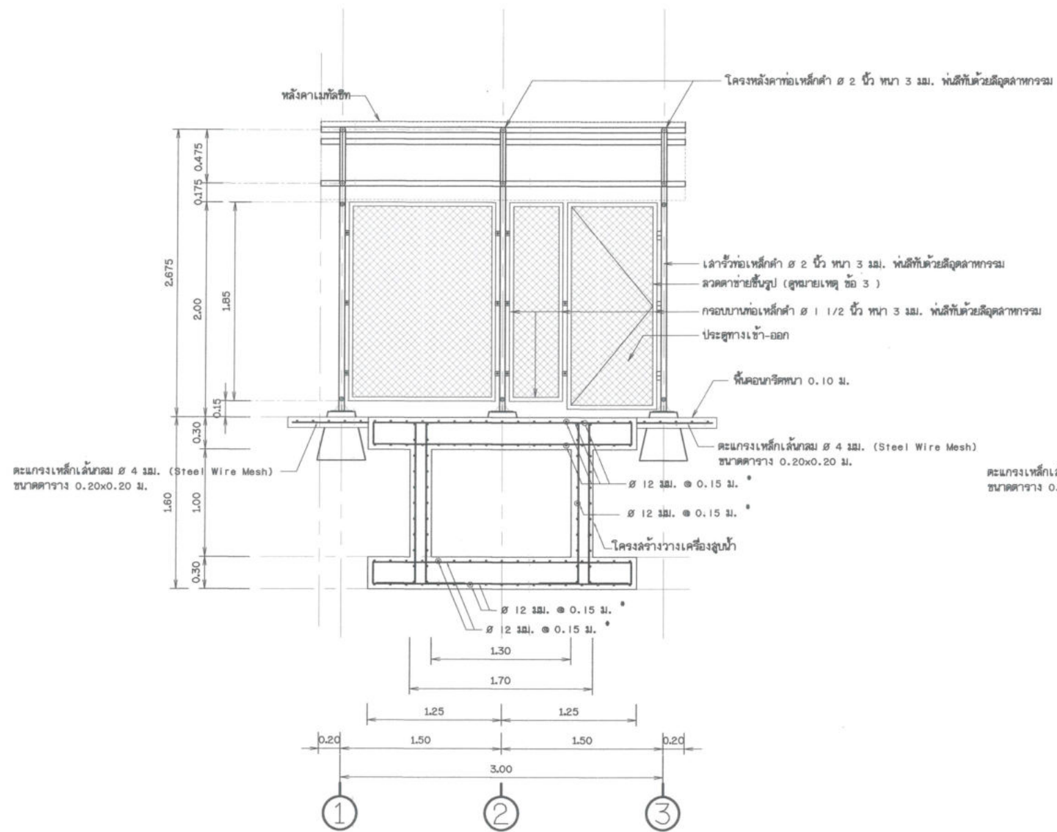
รูปตัด ก - ก ไม่แสดงขนาดราวล้วน
