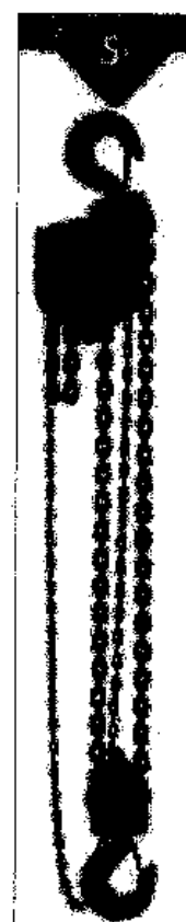
จอกใช้มือส่ว ขนาด 5 ตัน น้ำหนักยก 5(ตัน) Test Load 5.30(ตัน) ยกลูก 3(เมตร) จำนวนทาบโซ่ 2 โซ่ยก 9.0 x 27 โซ่ดึง 5.5 x 23.6 ระยะห่างระหว่างตะขอ 635 (mm) น้ำหนักจอก 43.0 (kg) การออกแรงยก 39 kgf
