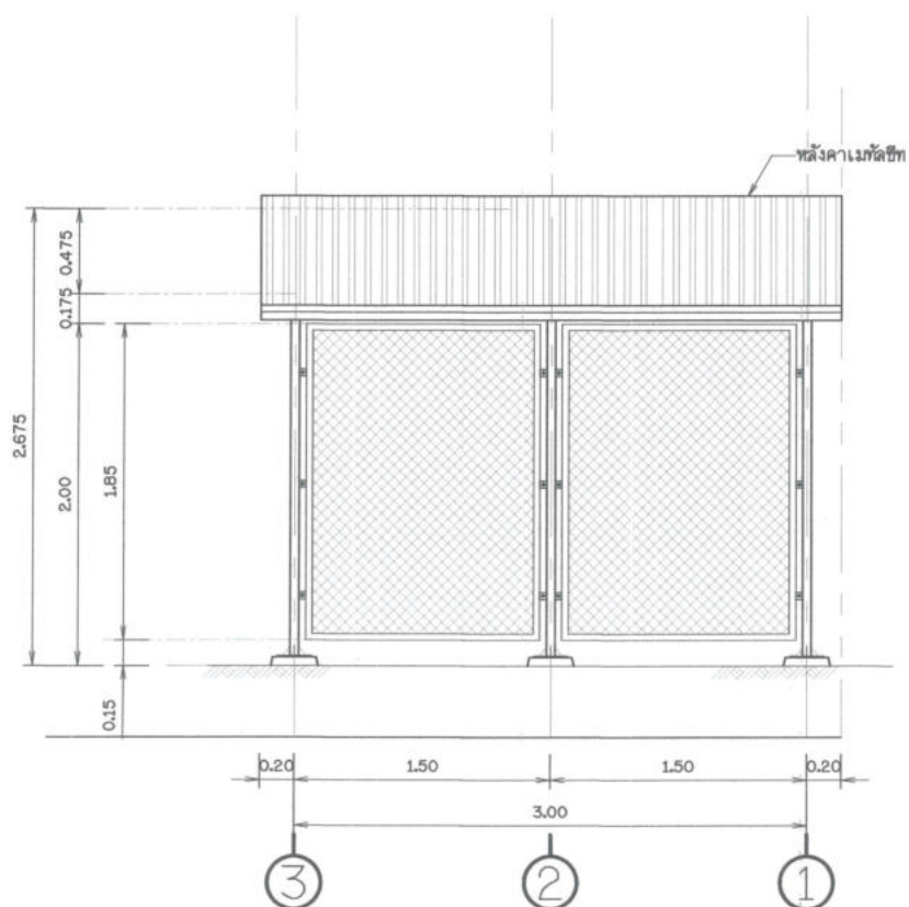
รูปด้าน 1 โมเมนต์มาตรฐาน
