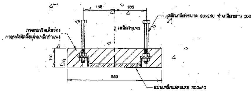
การติดตั้งเหล็กค้ำพอง มาตราส่วน 1:5
