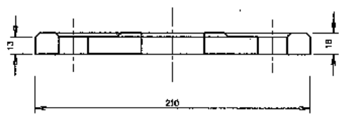
① ฐาน เหล็กหล่อ มาตราส่วน 1:2
