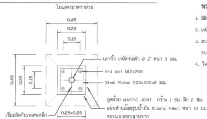
รูปขยายฐานจากโครงสร้างรับแผง F2 (ต่อม่อ คลล. หล่อสำเร็จรูปพร้อมติดตั้ง)
