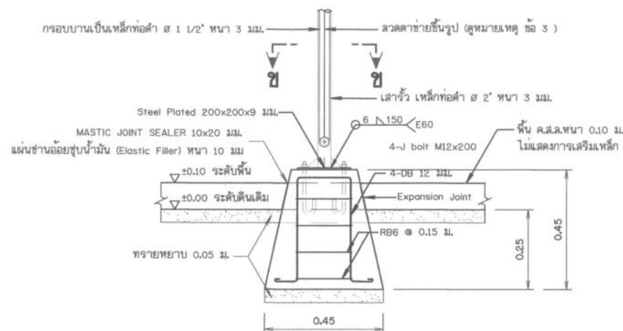
รูปขยายฐานจากโครงสร้างรับแผง F2 (ต่อม่อ คลล. หล่อสำเร็จรูปพร้อมติดตั้ง)
