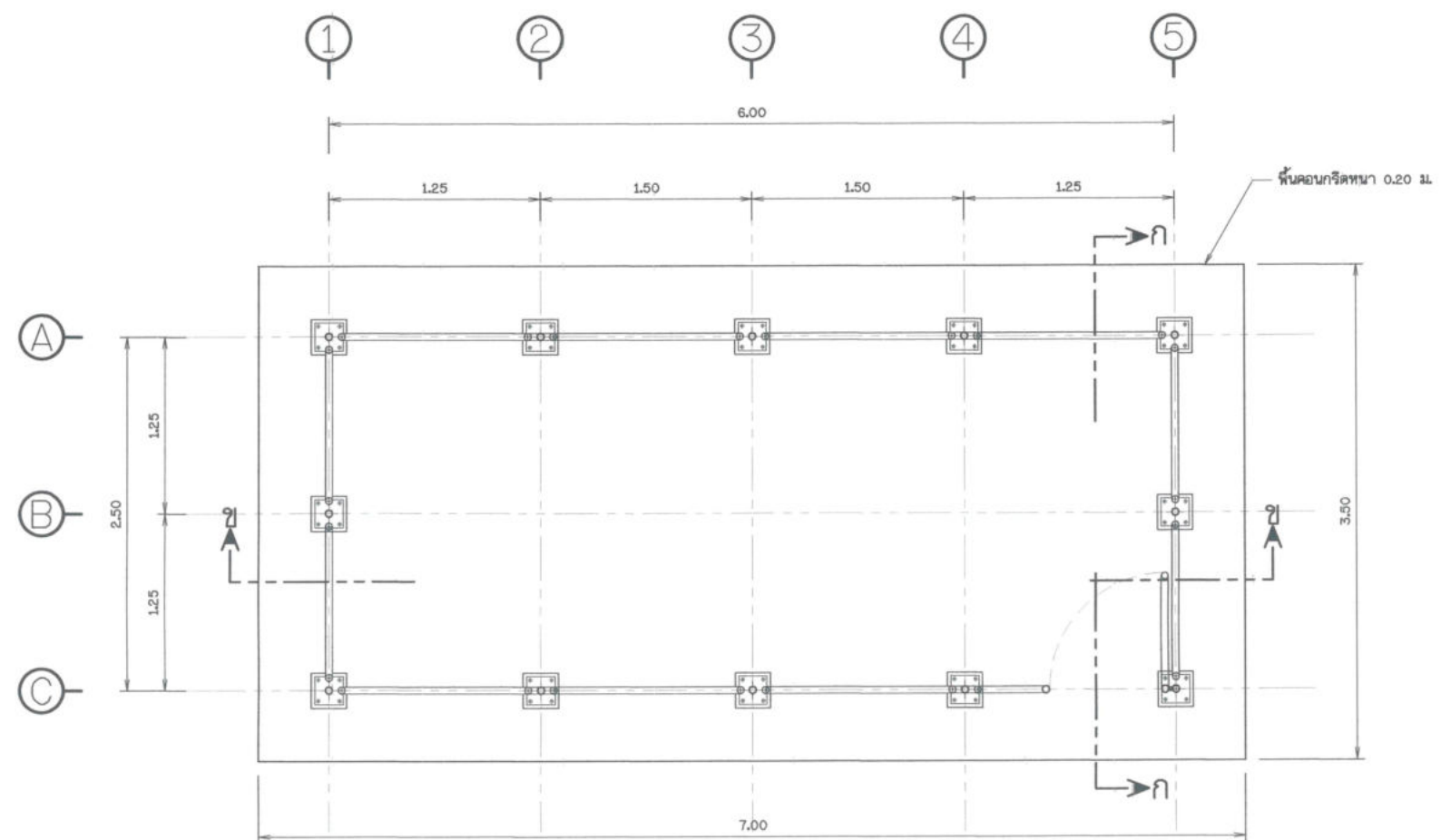
แปลนเสาและรั้ว โรงผลิตน้ำตาลส่วน
