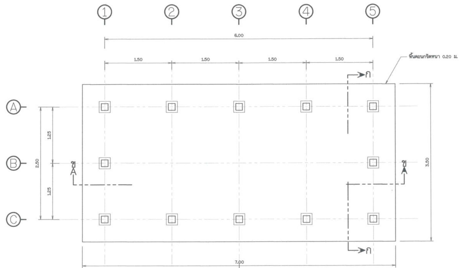
แบบแปลน โรงผลิตน้ำตาลส่วน
