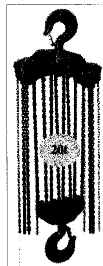
จอกใช้มือส่ว ขนาด 20 ตัน น้ำหนักยก 20(ตัน) Test Load 25(ตัน) ยกลูก 3.5(เมตร) จำนวนทาบโซ่ 8 โซ่ยก 9.0 x 27 โซ่ดึง 5.5 x 23.6 ระยะห่างระหว่างตะขอ 870 (mm) น้ำหนักจอก 190.0 (kg) การออกแรงยก 41 x 2 kgf
