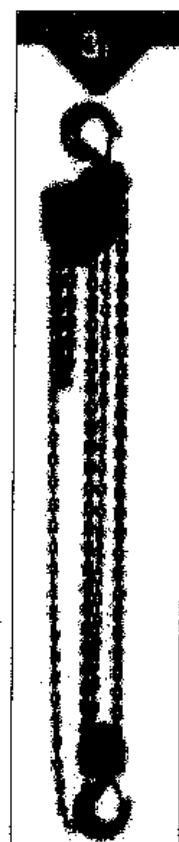
จอกใช้มือส่ว ขนาด 3 ตัน น้ำหนักยก 3(ตัน) Test Load 4.75(ตัน) ยกลูก 3(เมตร) จำนวนทาบโซ่ 2 โซ่ยก 7.1 x 21 โซ่ดึง 5.0 x 22.8 ระยะห่างระหว่างตะขอ 475 (mm) น้ำหนักจอก 23.0 (kg) การออกแรงยก 35 kgf
