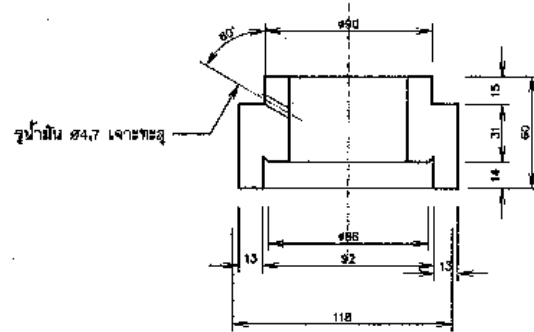
④ แผ่นปิด มาตราส่วน 1:2
