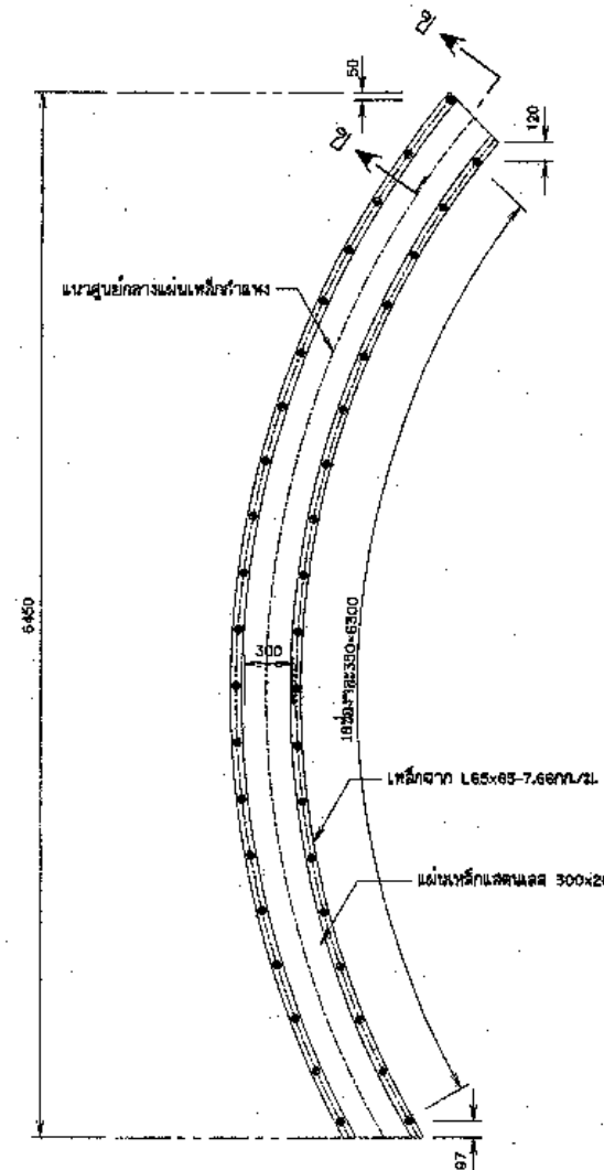
การติดตั้งเหล็กค้ำพอง มาตราส่วน 1:25
