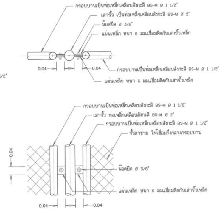
แบบขยายรายละเอียดแสดงการยึดระหว่างรั้วกับเสา
