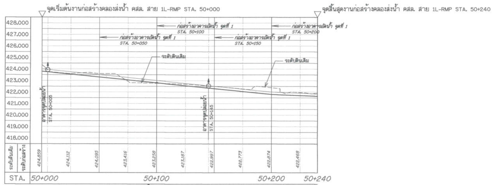
รูปตัดตามแนวยาว มาตราส่วน แนวนอน 1:1,000 แนวตั้ง 1:100
