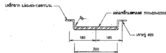
รูปขยายเหล็กค้ำพอง มาตราส่วน 1:5
