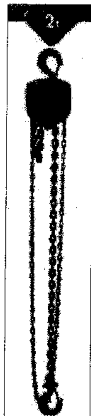
จอกใช้มือส่ว ขนาด 2 ตัน น้ำหนักยก 2(ตัน) Test Load 30(ตัน) ยกลูก 30(เมตร) จำนวนทาบโซ่ 1 โซ่ยก 7.9 x 23 โซ่ดึง 5.5 x 23.6 ระยะห่างระหว่างตะขอ 390 (mm) น้ำหนักจอก 21.6 (kg) การออกแรงยก 34 kgf
