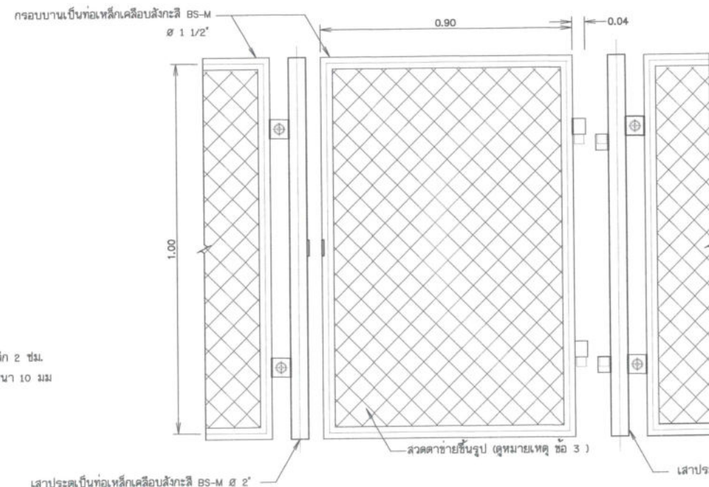
แบบขยายรายละเอียดประตู
