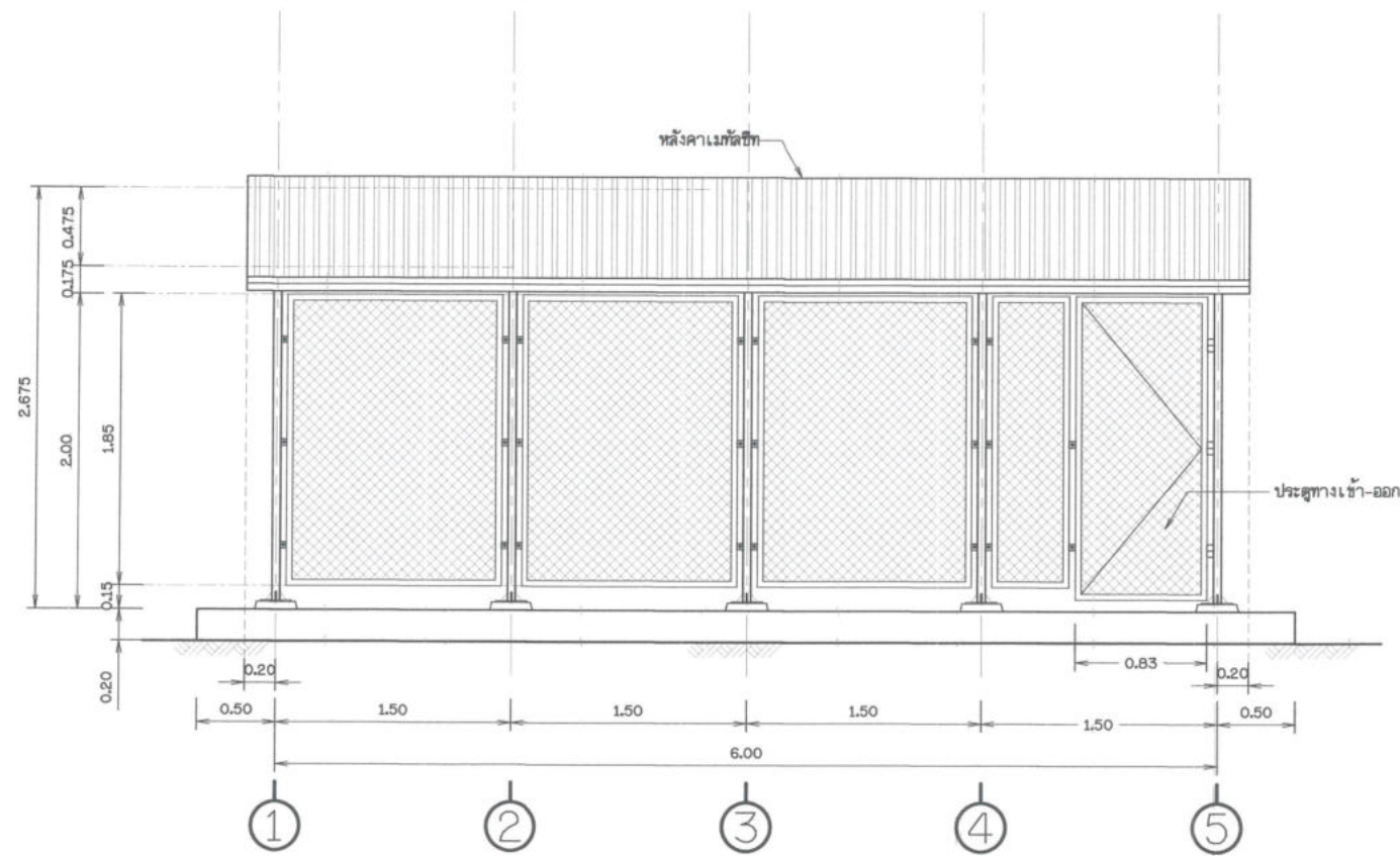
รูปด้าน 1 โมเดลขนาดจริง
