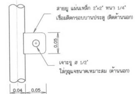
แบบขยายสายยู
