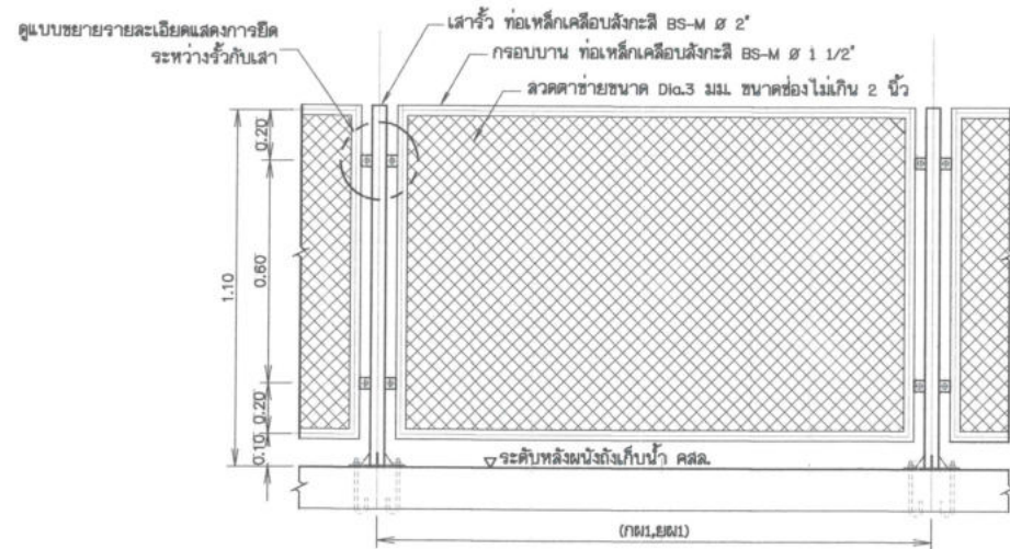
แบบขยายราวกันตก (สำหรับรั้วกับเสา คสล. แบบไม่มีฝ้า)
