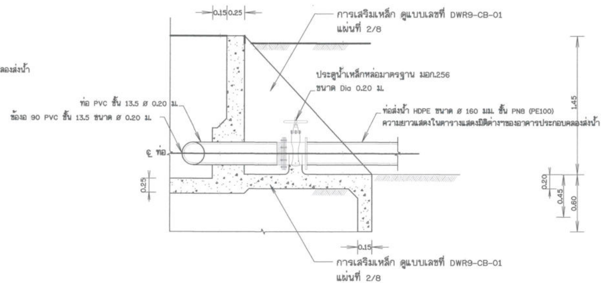
รูปตัดตามแนว ค - ค ไม่แสดงมาตราส่วน
