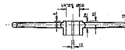
② ล้อมือหมุน มาตราส่วน 1:5 เหล็กหล่อ
