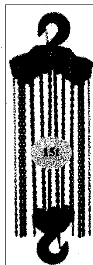
จอกใช้มือส่ว ขนาด 15 ตัน น้ำหนักยก 15(ตัน) Test Load 20(ตัน) ยกลูก 3.5(เมตร) จำนวนทาบโซ่ 6 โซ่ยก 9.0 x 27 โซ่ดึง 5.5 x 23.6 ระยะห่างระหว่างตะขอ 850 (mm) น้ำหนักจอก 150.0 (kg) การออกแรงยก 41 x 2 kgf
