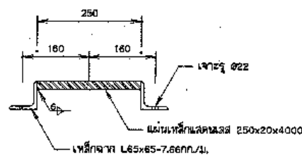
รูปขยายเหล็กกรง มาตราส่วน 1:5
