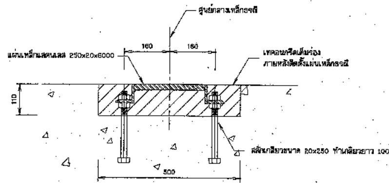
การติดตั้งเหล็กกรง มาตราส่วน 1:5
