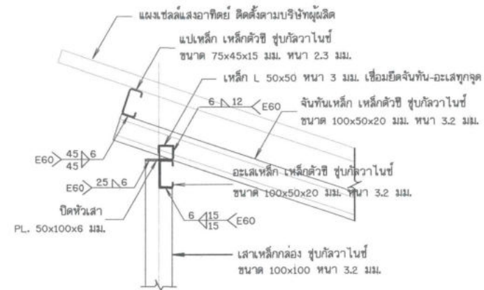
รูปขยาย การติดตั้งโครงหลังคา โมเดลตามตราส่วน
