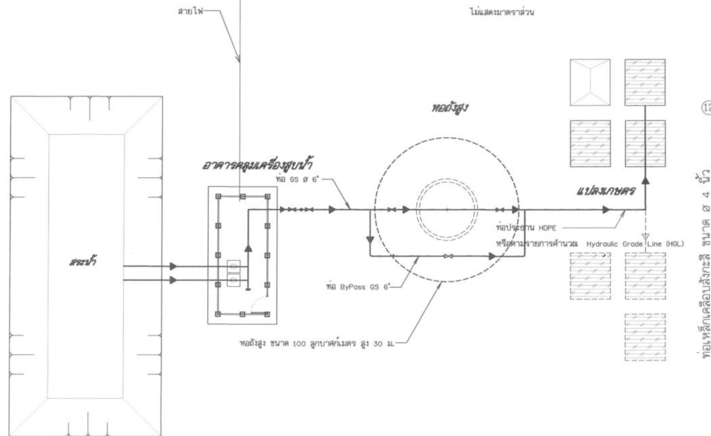
แผนผังระบบกระจายน้ำด้วยพลังงานแสงอาทิตย์ ขนาด 7.5 กิโลวัตต์
