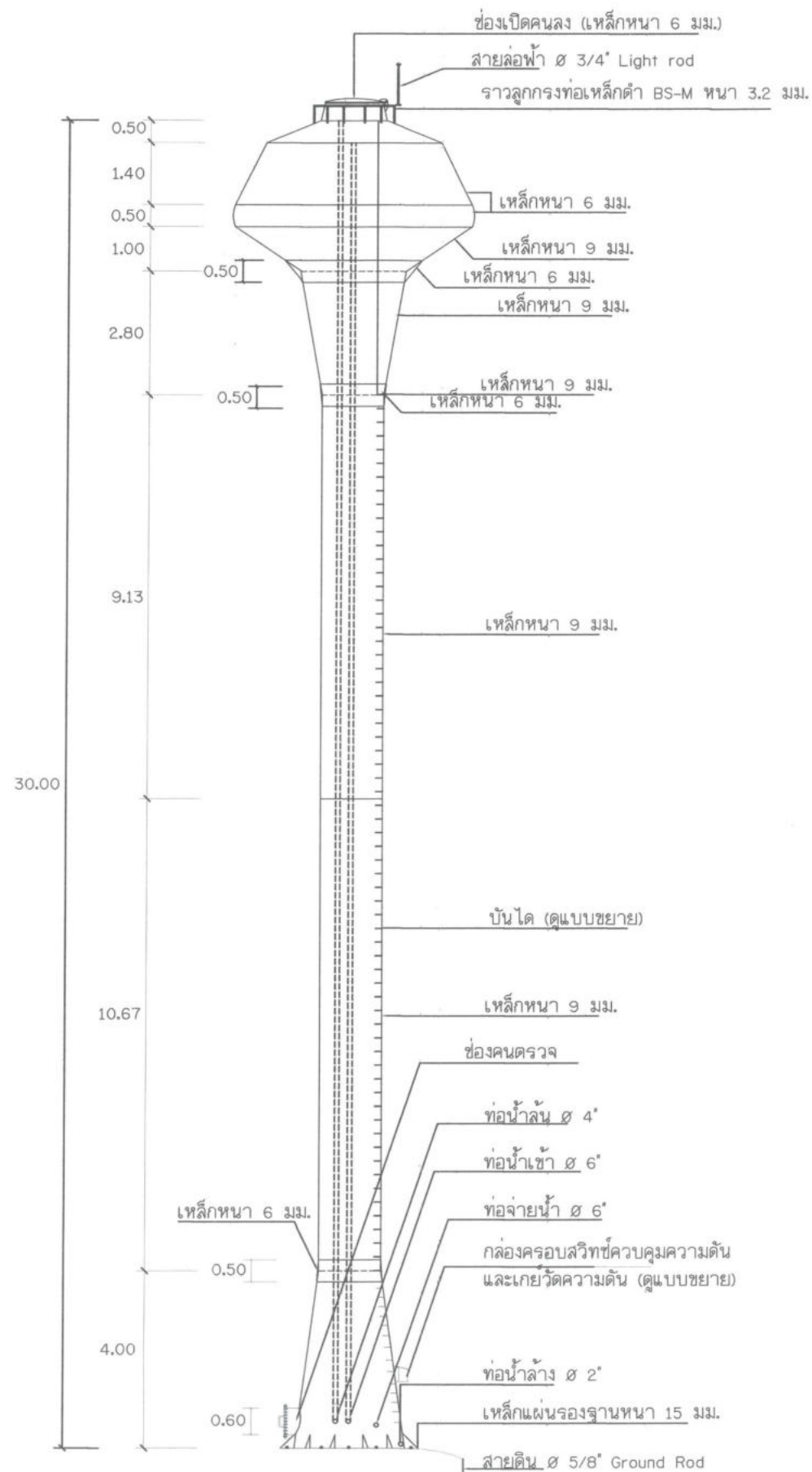
รูปด้านข้างของถังสูง แบบถังเหล็กรูปทรงถ้วยแฉมแปญ ไม่แสดงมาตราส่วน
