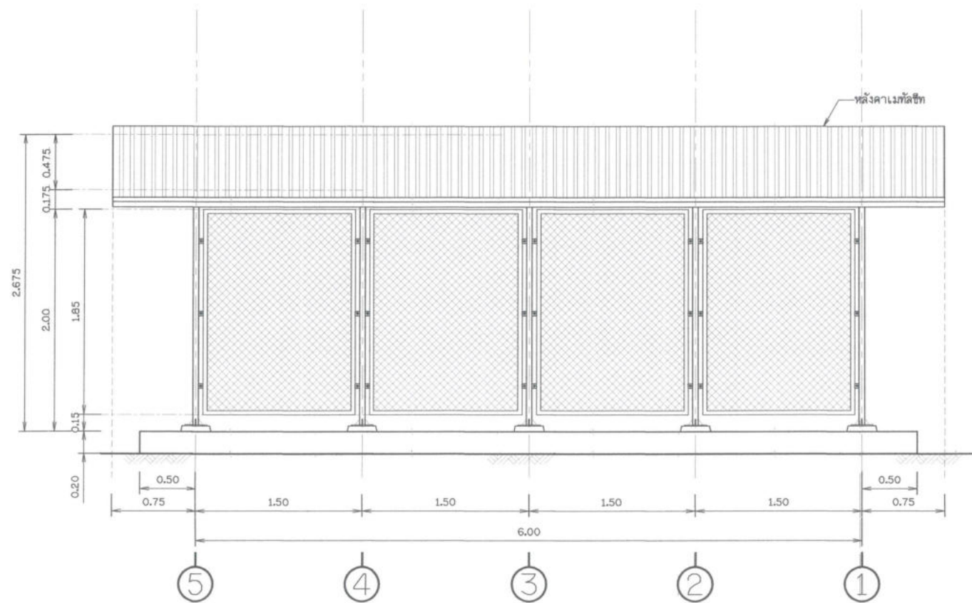
รูปด้าน 3 โมเดลตามมาตรฐาน
