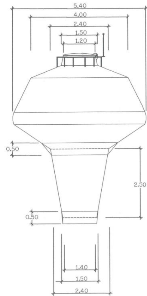
แบบขยายแมนโฮลบนถังแฉมแปญ ไม่แสดงมาตราส่วน
