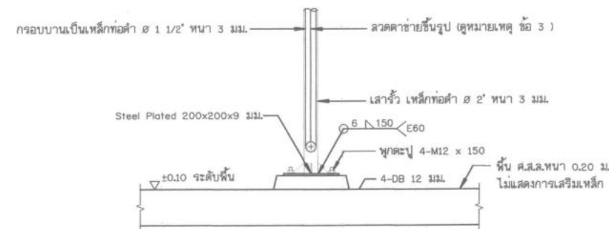
แบบขยายรายละเอียดแสดงการยึด ไม่แสดงขนาดราส่วน
