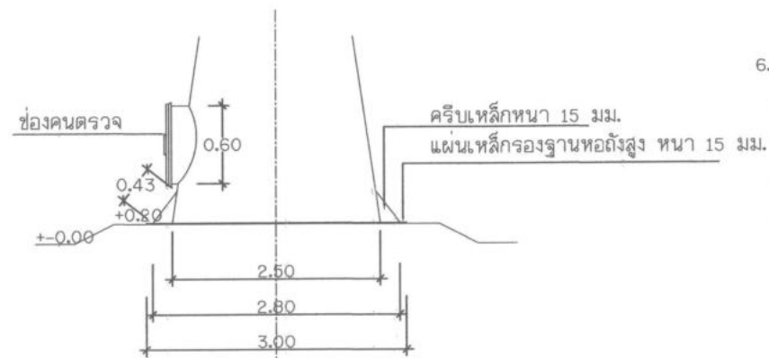
แบบขยายแมนโฮลบนถังแฉมแปญ ไม่แสดงมาตราส่วน
