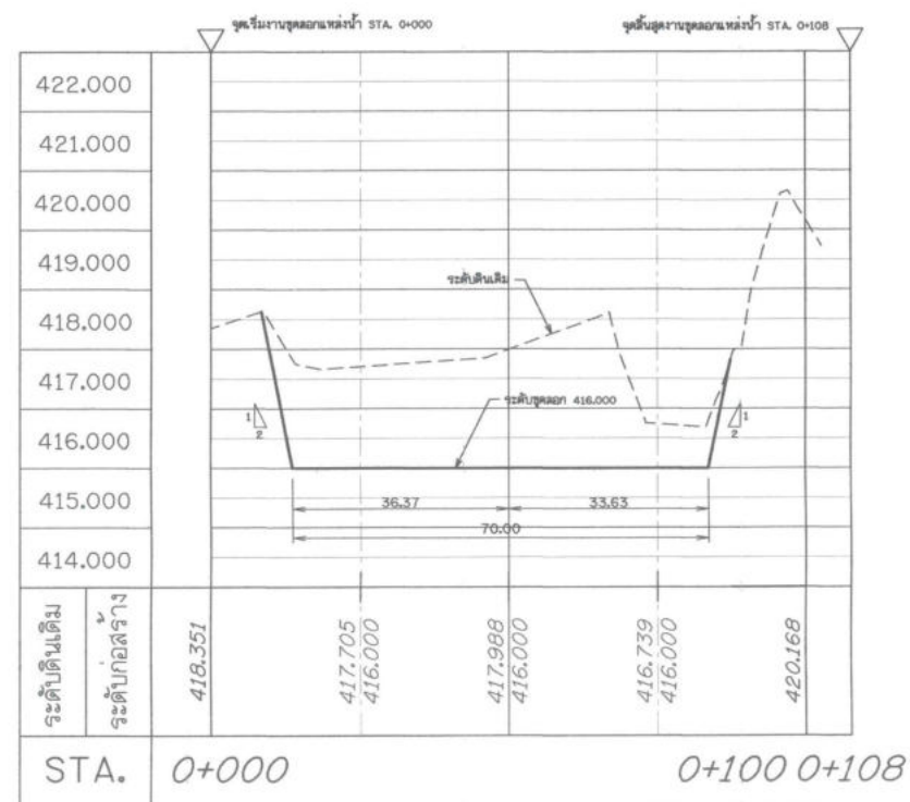
รูปตัดตามแนวยาว ไม่แสดงมาตราส่วน
