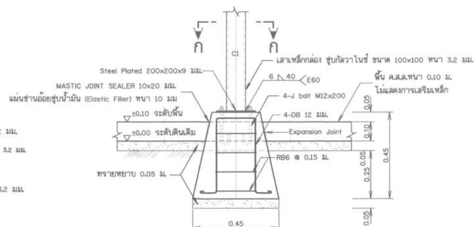
รูปขยายฐานรากโครงสร้างรับแผง F1 (ต่อม่อ คสล. ท่อส่งน้ำเรียงพร้อมติดตั้ง) ไม่แสดงขนาดราส่วน
