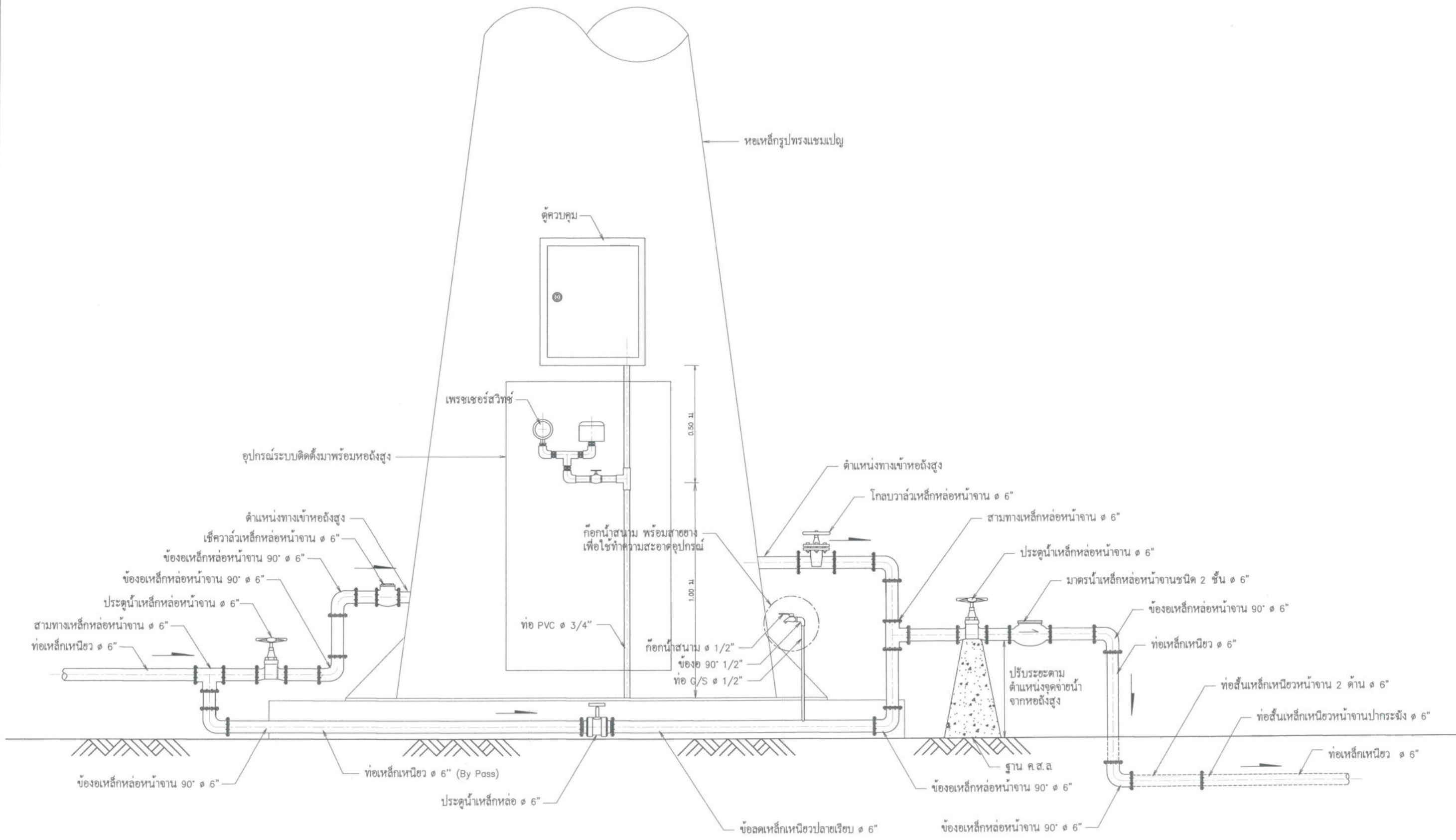
รูปแสดงรายละเอียดการต่อท่อและอุปกรณ์ออกจากถังกระจายน้ำ โมแสดงมาตราส่วน
