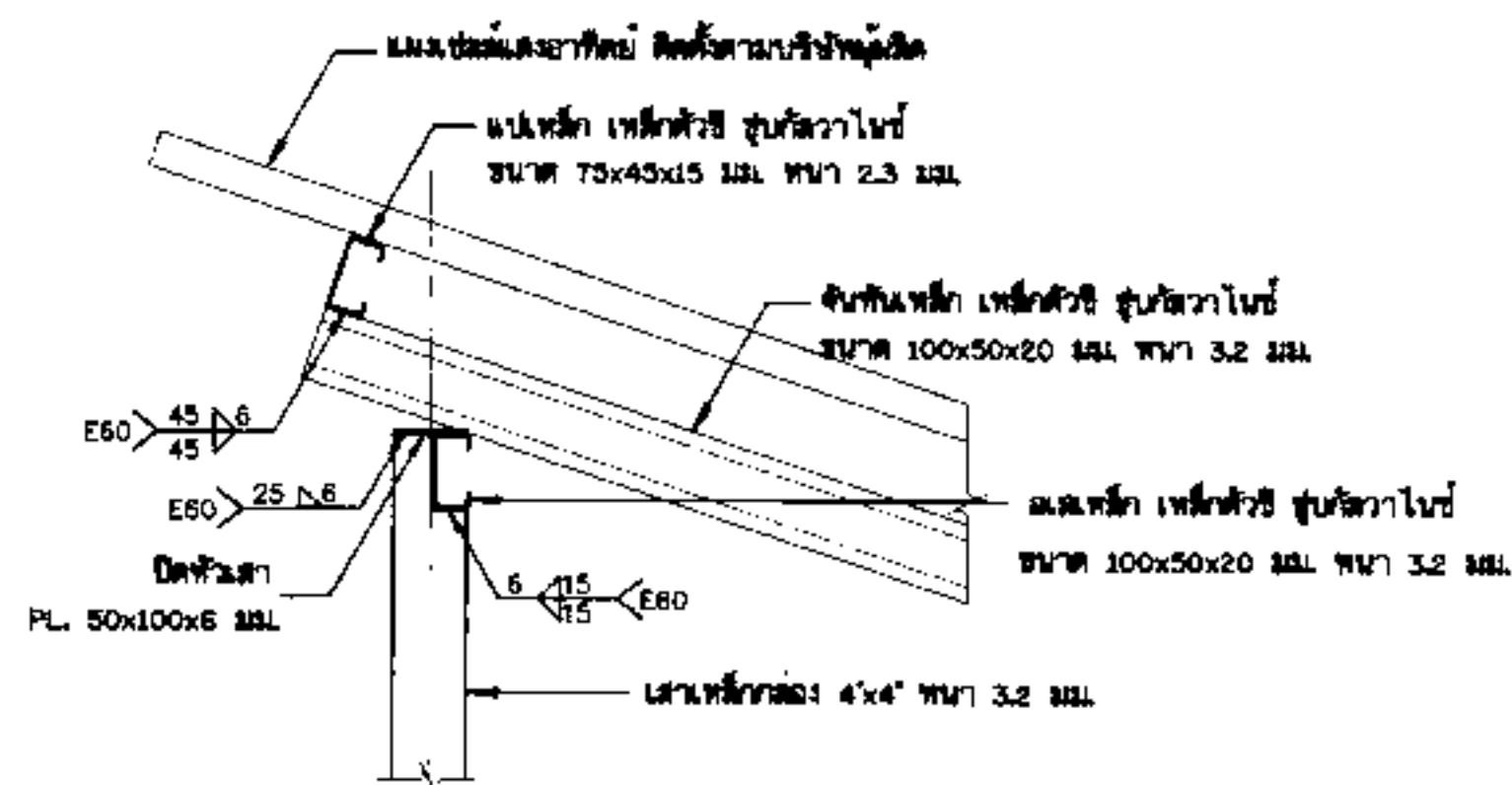
รูปขยาย การติดตั้งโครงหลังคา ไม่แสดงมาตราส่วน
