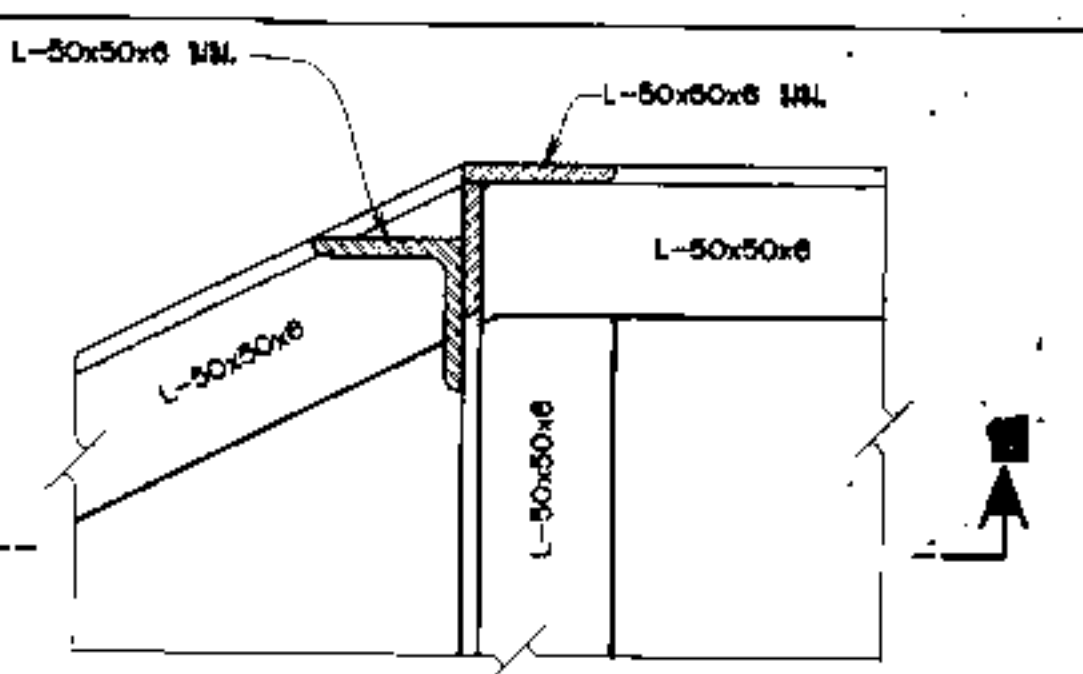
รูปขยาย 5 มาตราส่วน 1 : 2.5
