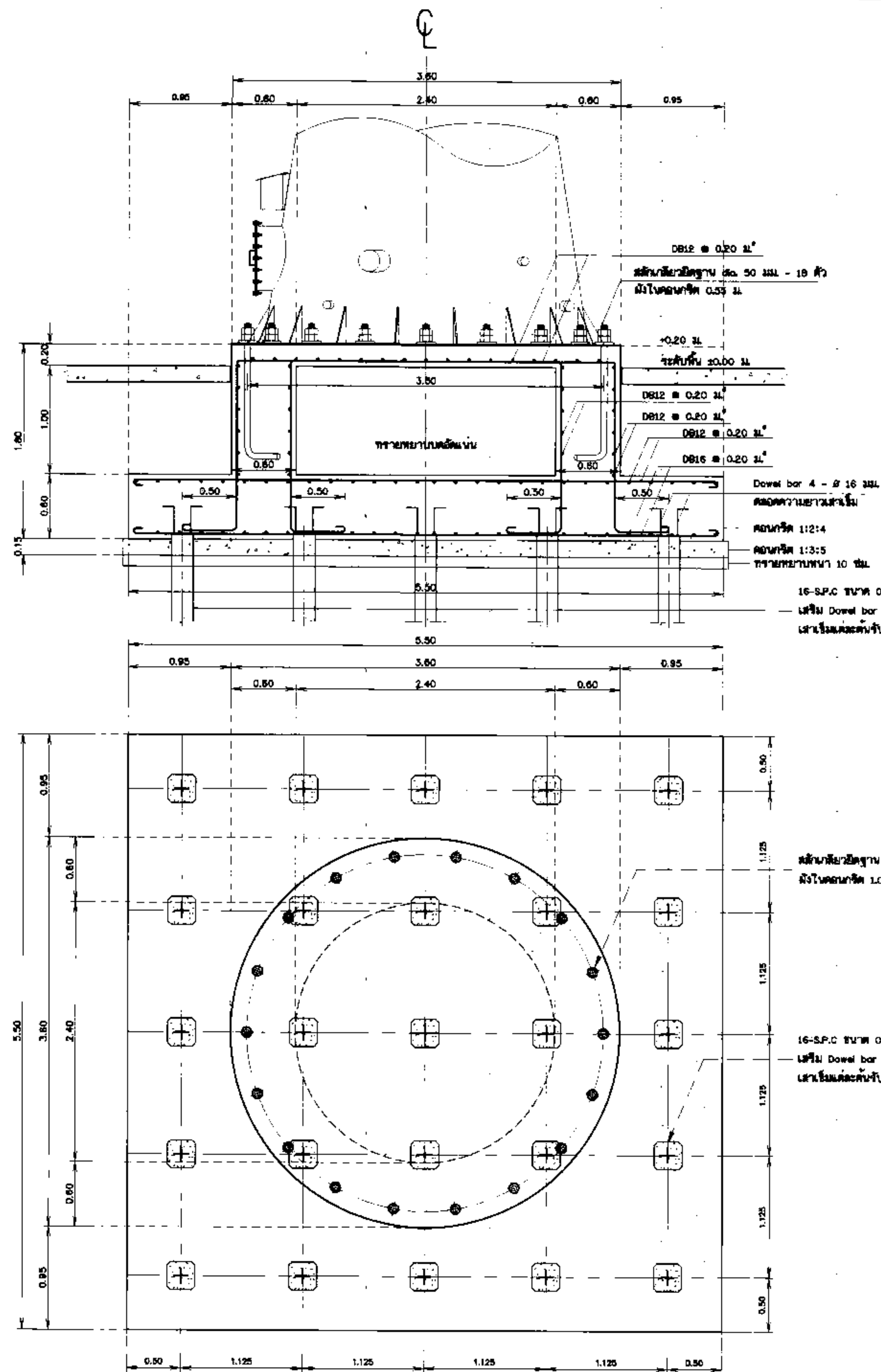
แบบขยายฐานรากท่อสูง (แบบเสาเข็ม)
