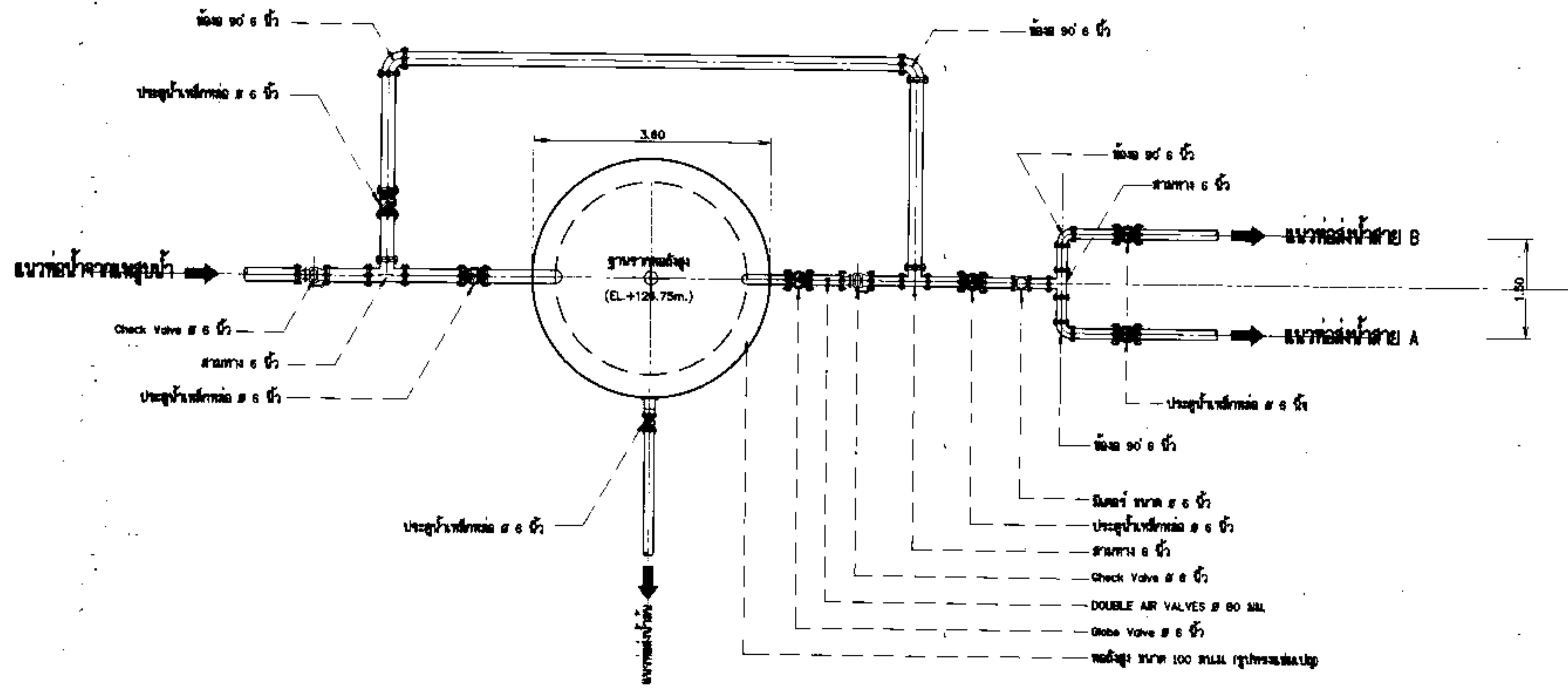
แปลนระบบท่อถังเก็บน้ำ มาตราส่วน 1:50
