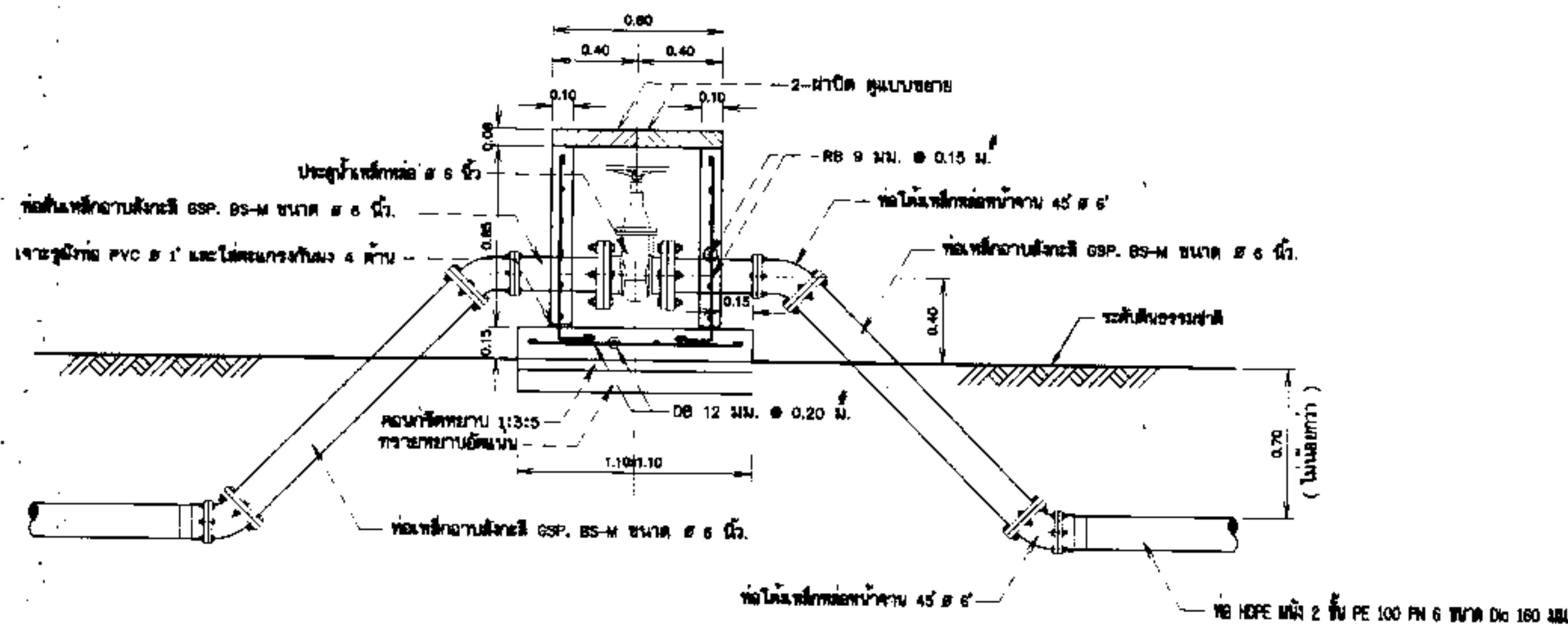
รูปตัด ก - ก มาตราส่วน 1:20
