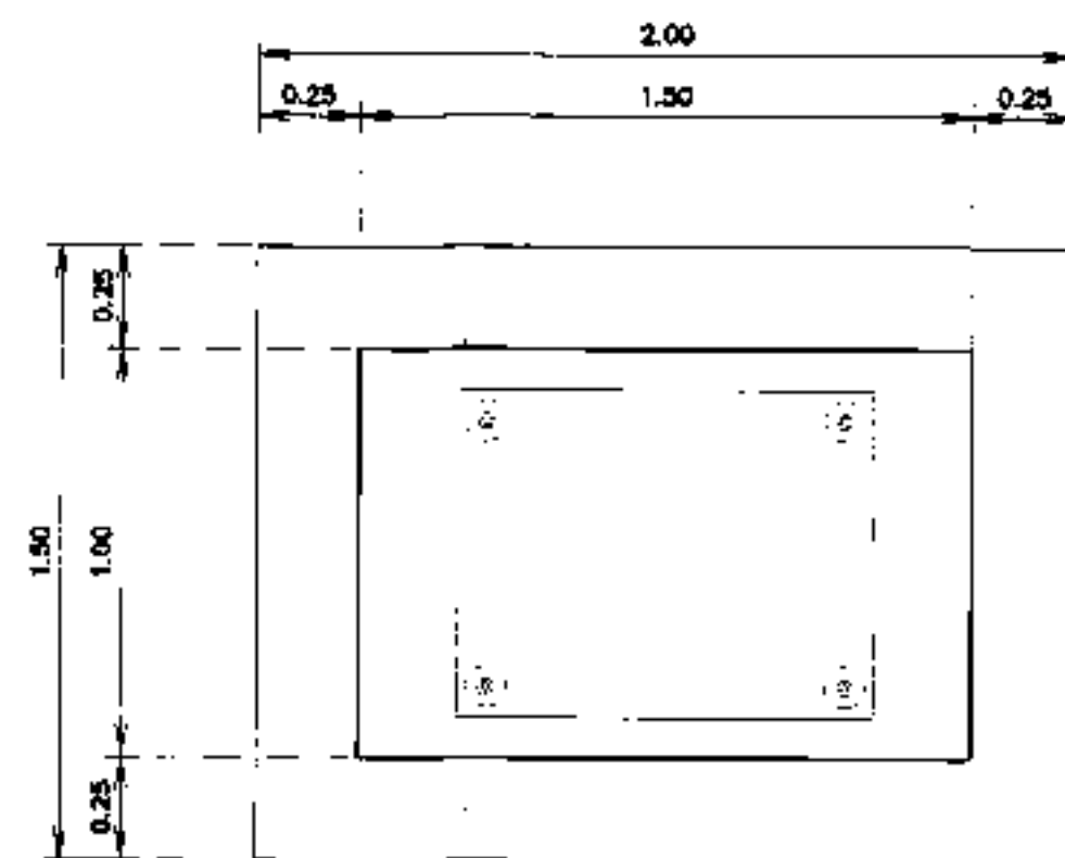
แปลนแท่นเครื่องกวด ไม่แสดงมาตราส่วน
