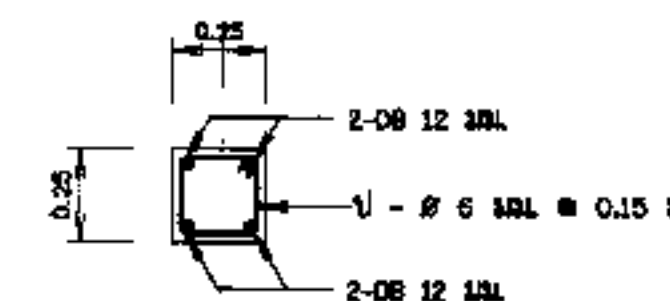
เสาตอม่อ มาตราส่วน 1:20
