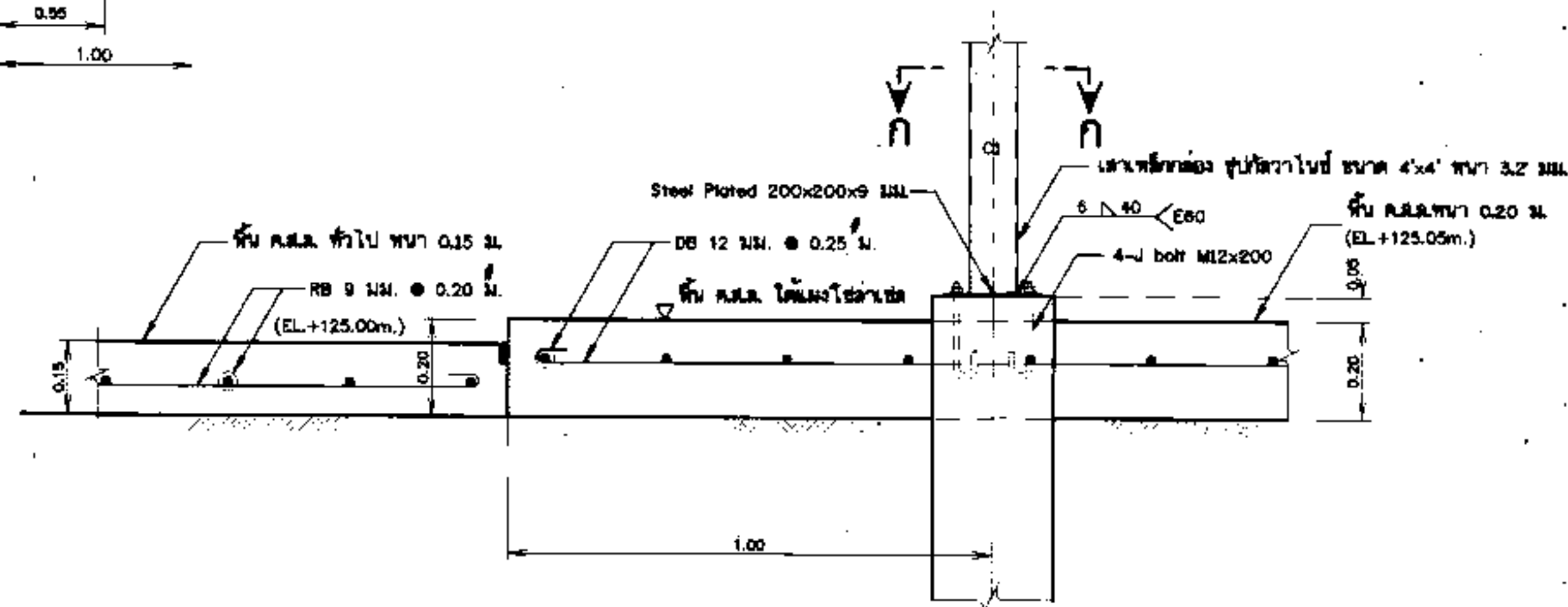
ขยายพื้น มาตราส่วน 1:10
