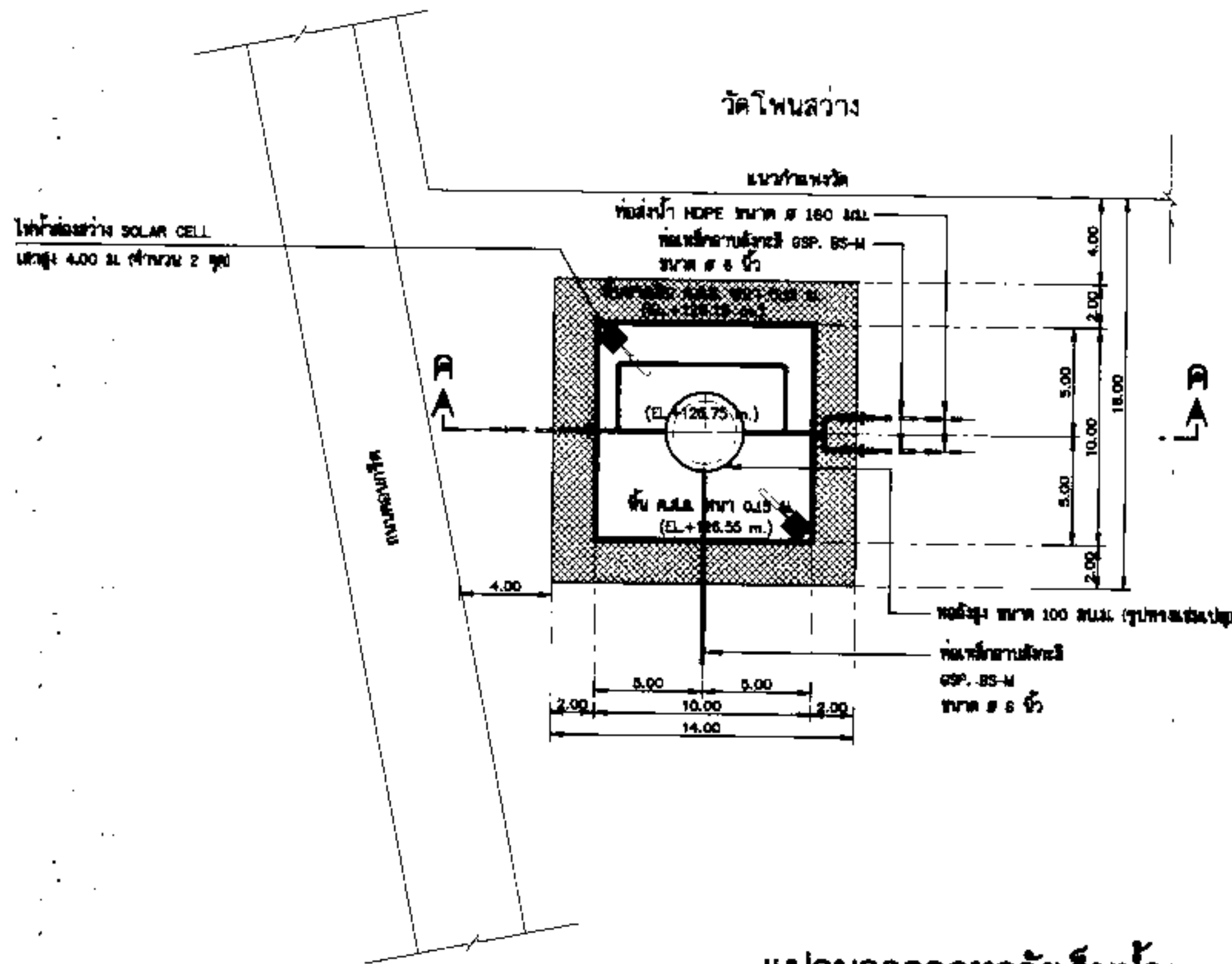
แปลนอาคารท่อถังเก็บน้ำ มาตราส่วน 1:200
