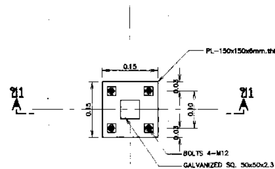
แบบขยายเสา 2
