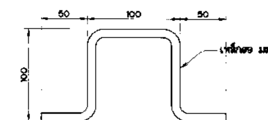
รูปขยายเหล็กหัวเสา MANHOLE
