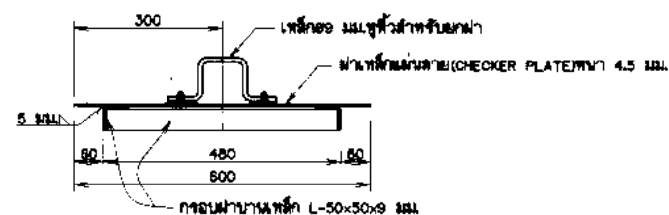
รูปตัด จ-จ
