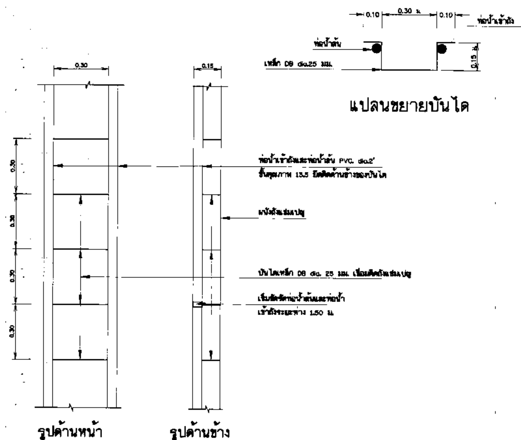
แบบขยายบันได และการยึดท่อน้ำล้นและท่อน้ำเข้าถัง
