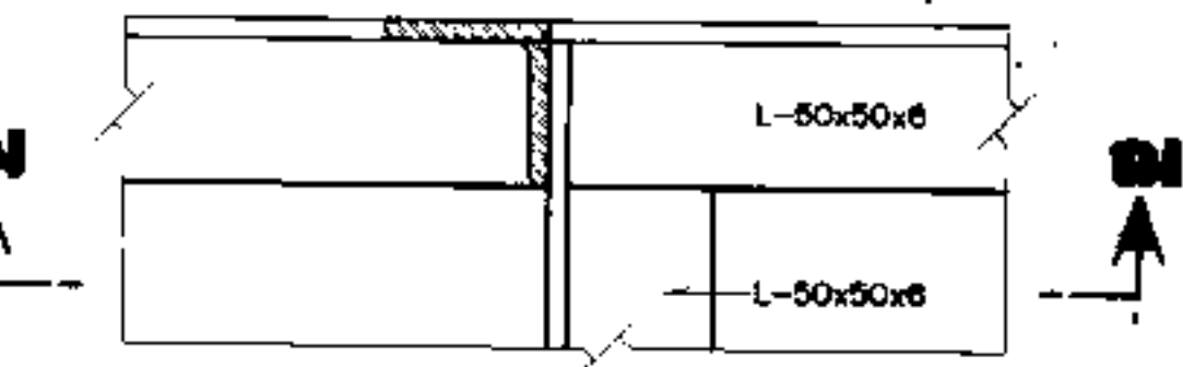
รูปขยาย 6 มาตราส่วน 1 : 2.5
