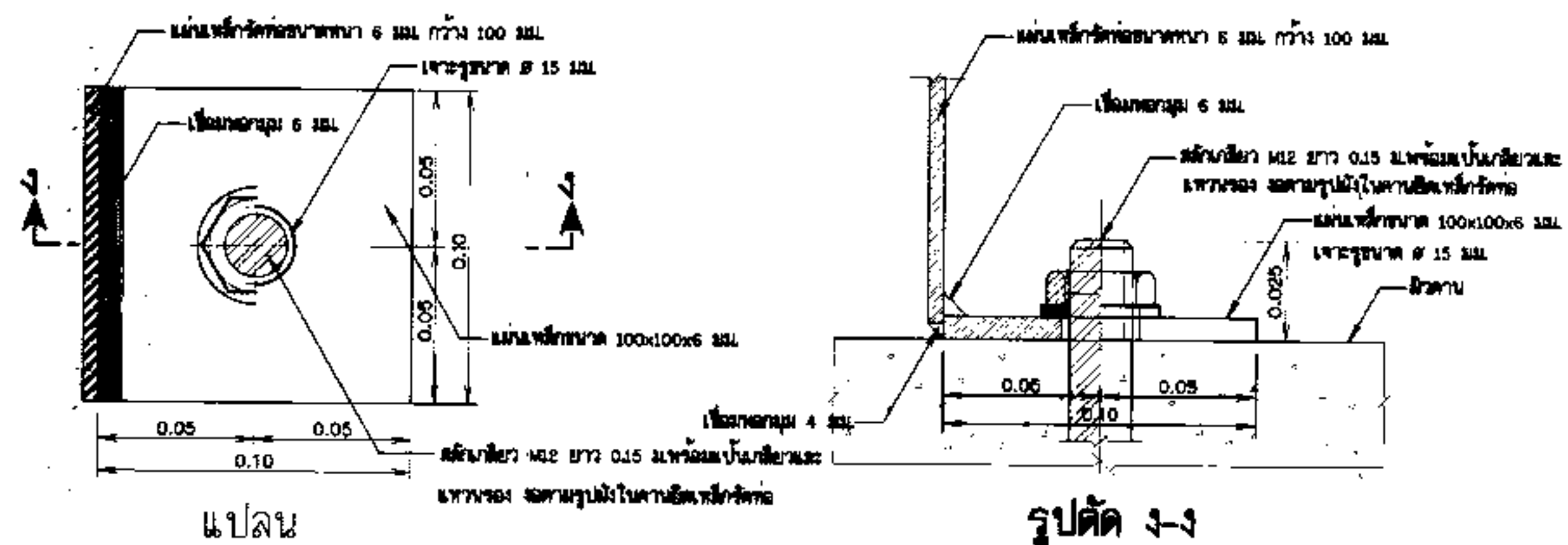
รายละเอียดแผ่นเหล็กยึดท่อ ไม่แสดงมาตรฐาน
