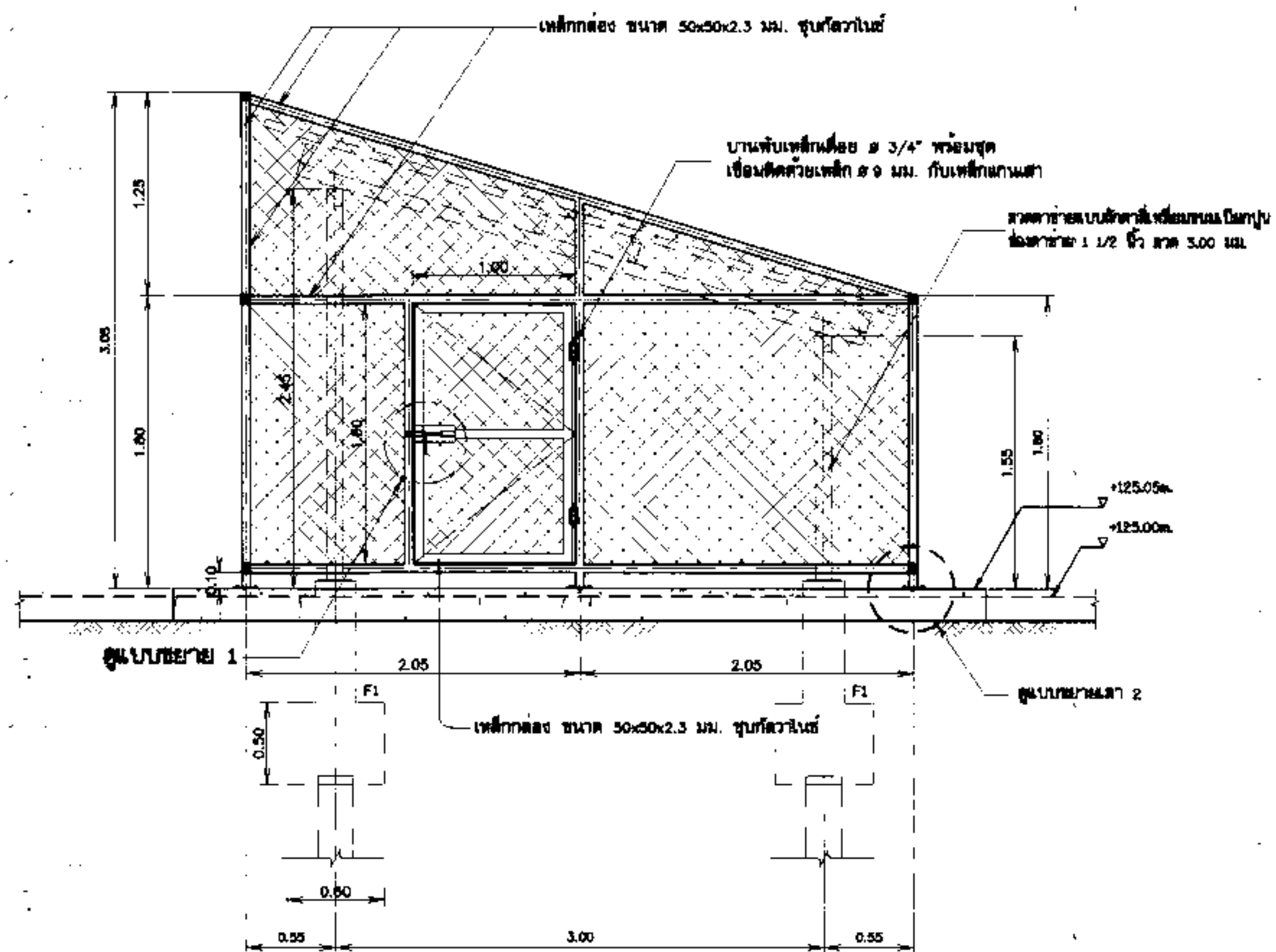
รูปตัด ก1 - ก1
