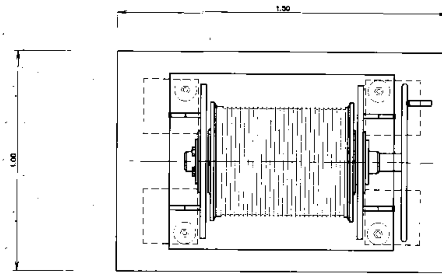
แปลนเครื่องกวด ไม่แสดงมาตราส่วน
