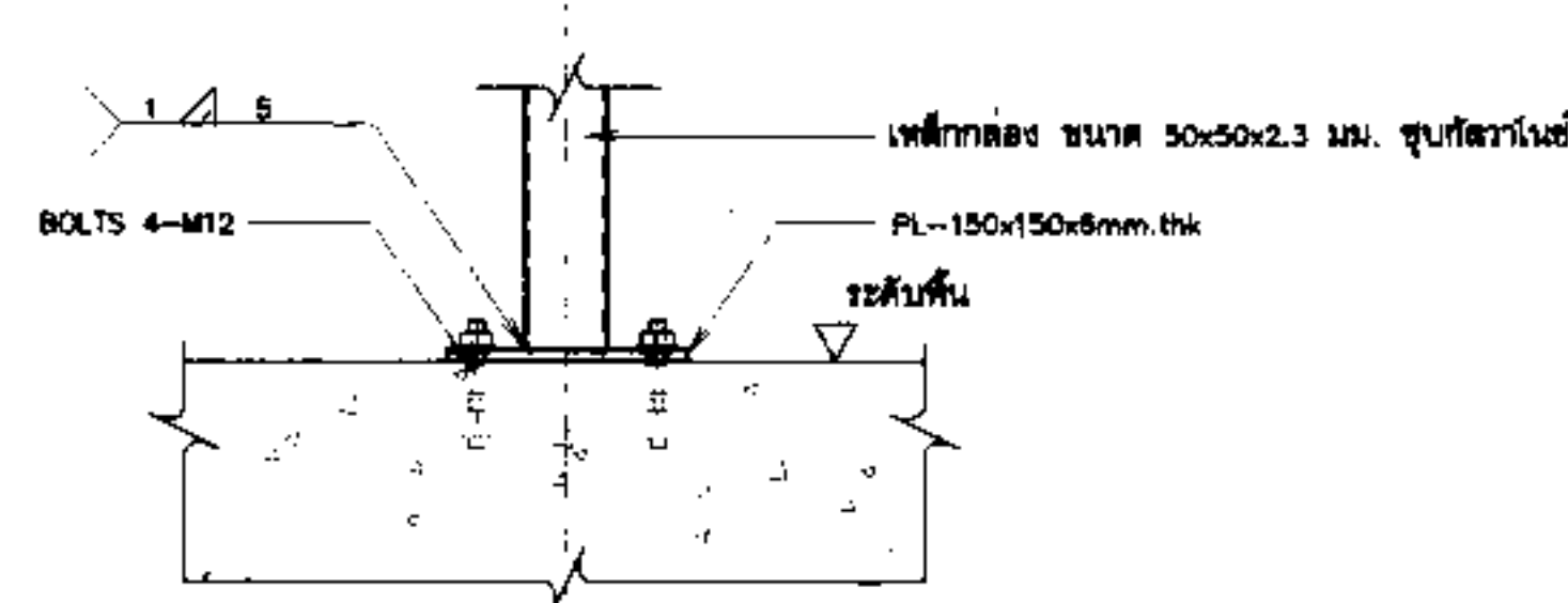
รูปตัด ข1 - ข1
