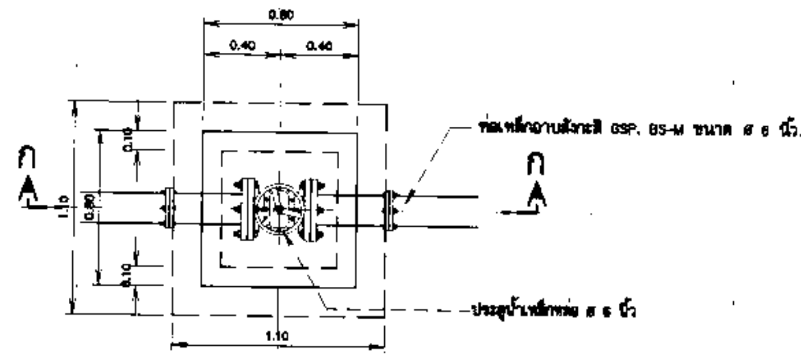
อาคารบ่อประตูปรับระดับน้ำ มาตราส่วน 1:20
