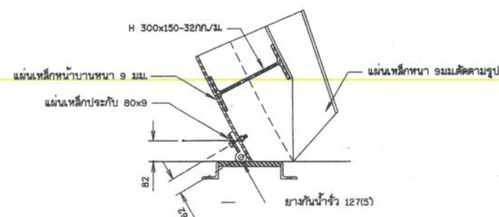
รูปขยายยงกันน้ำรั่วใต้บ้าน
