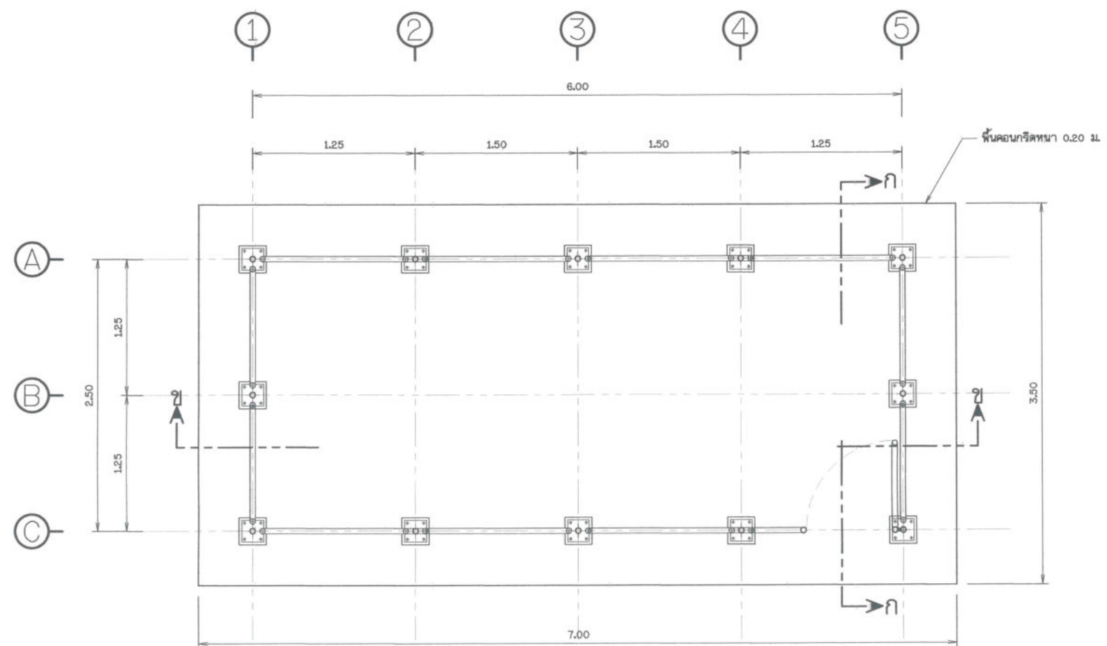
แปลนเสาและรื้อ โรงผลิตนมสดราส่วน
