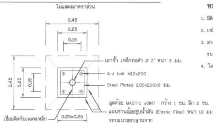
รูปขยายฐานจากโครงสร้างรับแผง F2 (ต่อม่อ คลส. หล่อสำเร็จรูปพร้อมติดตั้ง)
