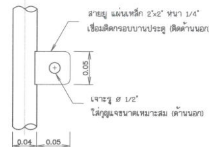
แบบขยายสลัวยู
