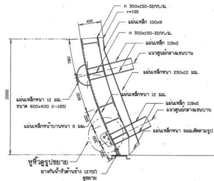
รูปตัด ก - ก
