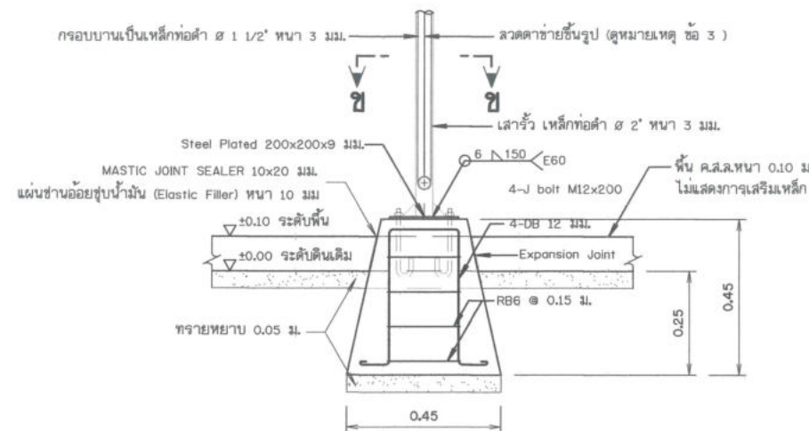
รูปขยายฐานจากโครงสร้างรับแผง F2 (ต่อม่อ คลส. หล่อสำเร็จรูปพร้อมติดตั้ง)
