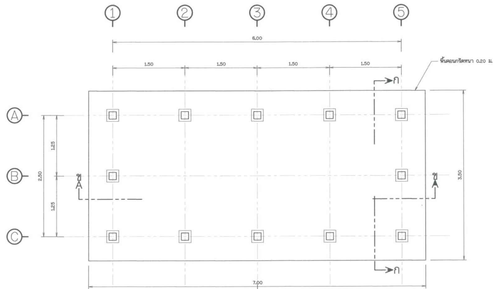
แบบแปลน โรงผลิตนมสดราส่วน
