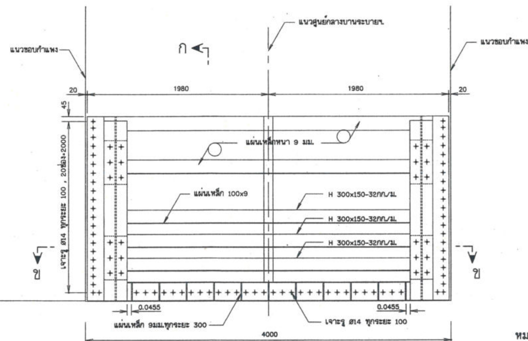
รูปตัด ก - ก บ้านระบายนด้านท้ายน้ำ
