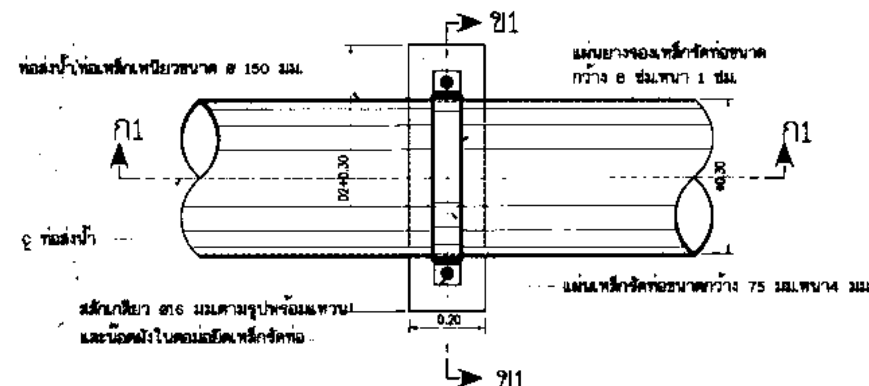
แบบการยึดท่อ ไม่แสดงมาตราส่วน
