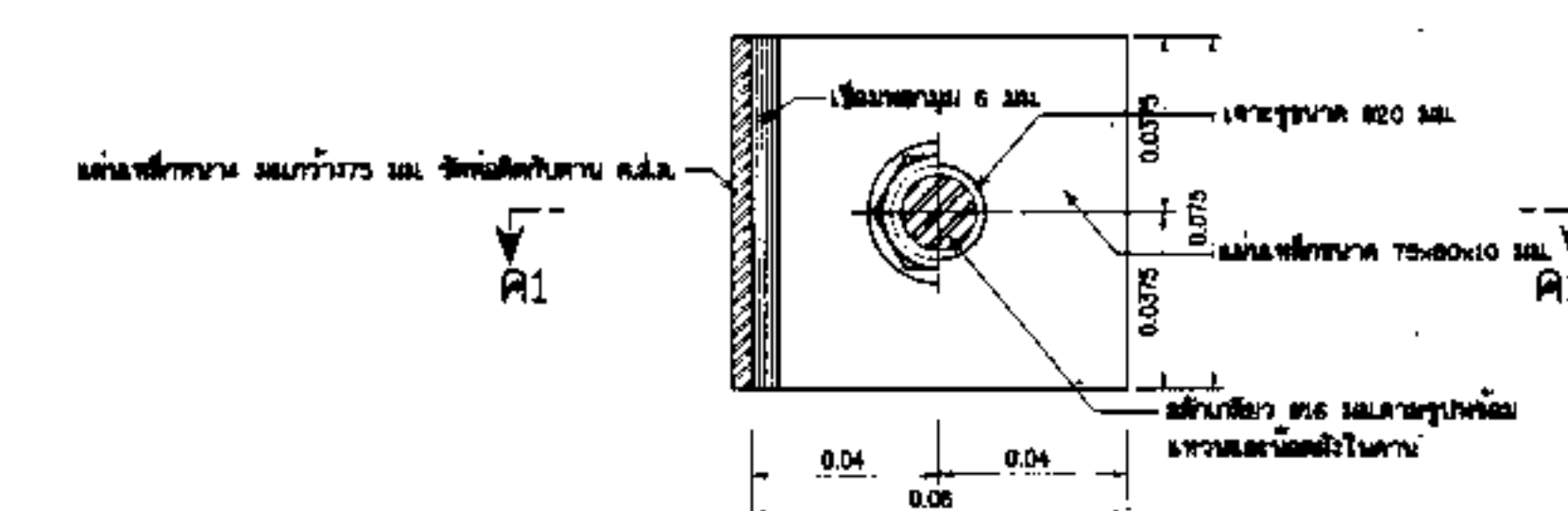
แบบแผ่นเหล็กยึดท่อ ไม่แสดงมาตราส่วน
