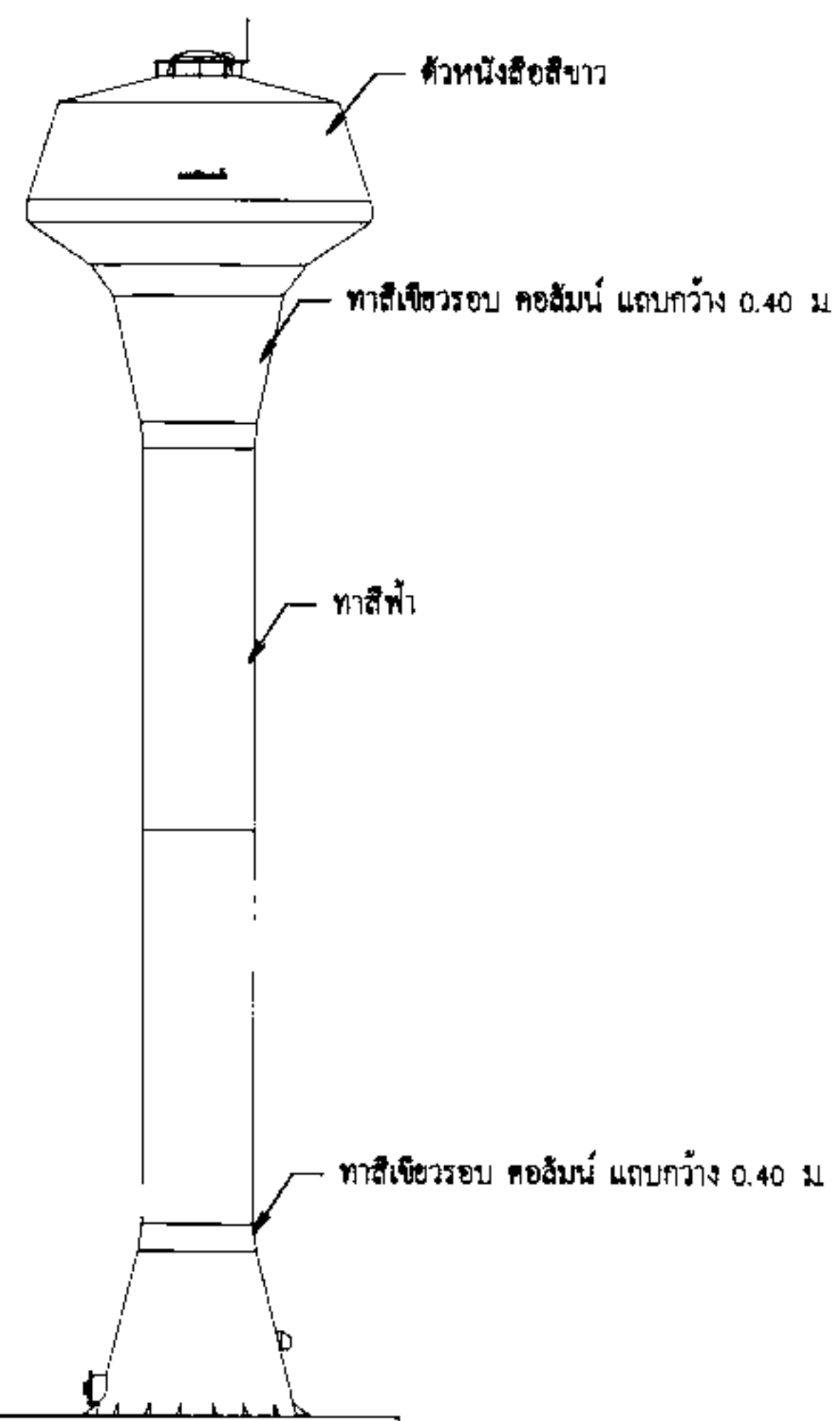
รูปด้าน ไม่แสดงขนาดจริง
