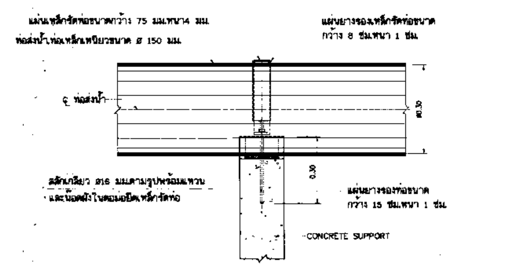
รูปตัด ก1 - ก2 ไม่แสดงมาตราส่วน
