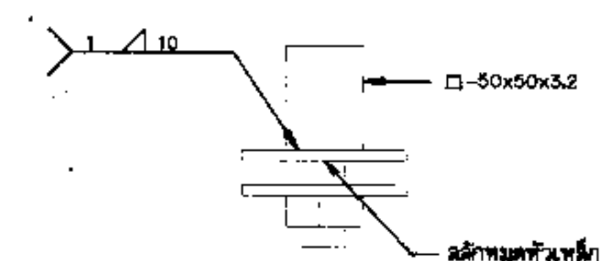
แบบขยาย สลักหมุดยึด
