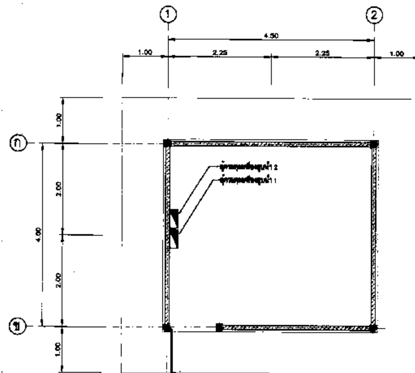
แบบควบคุมเครื่องสูบน้ำ
