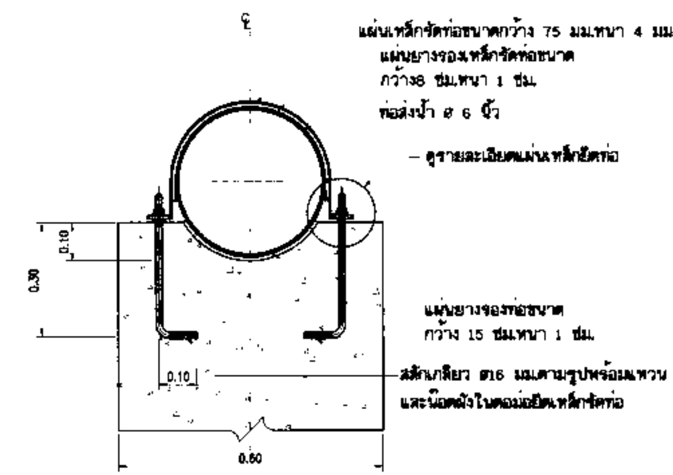
รูปตัด ข1 - ข2 ไม่แสดงมาตราส่วน
