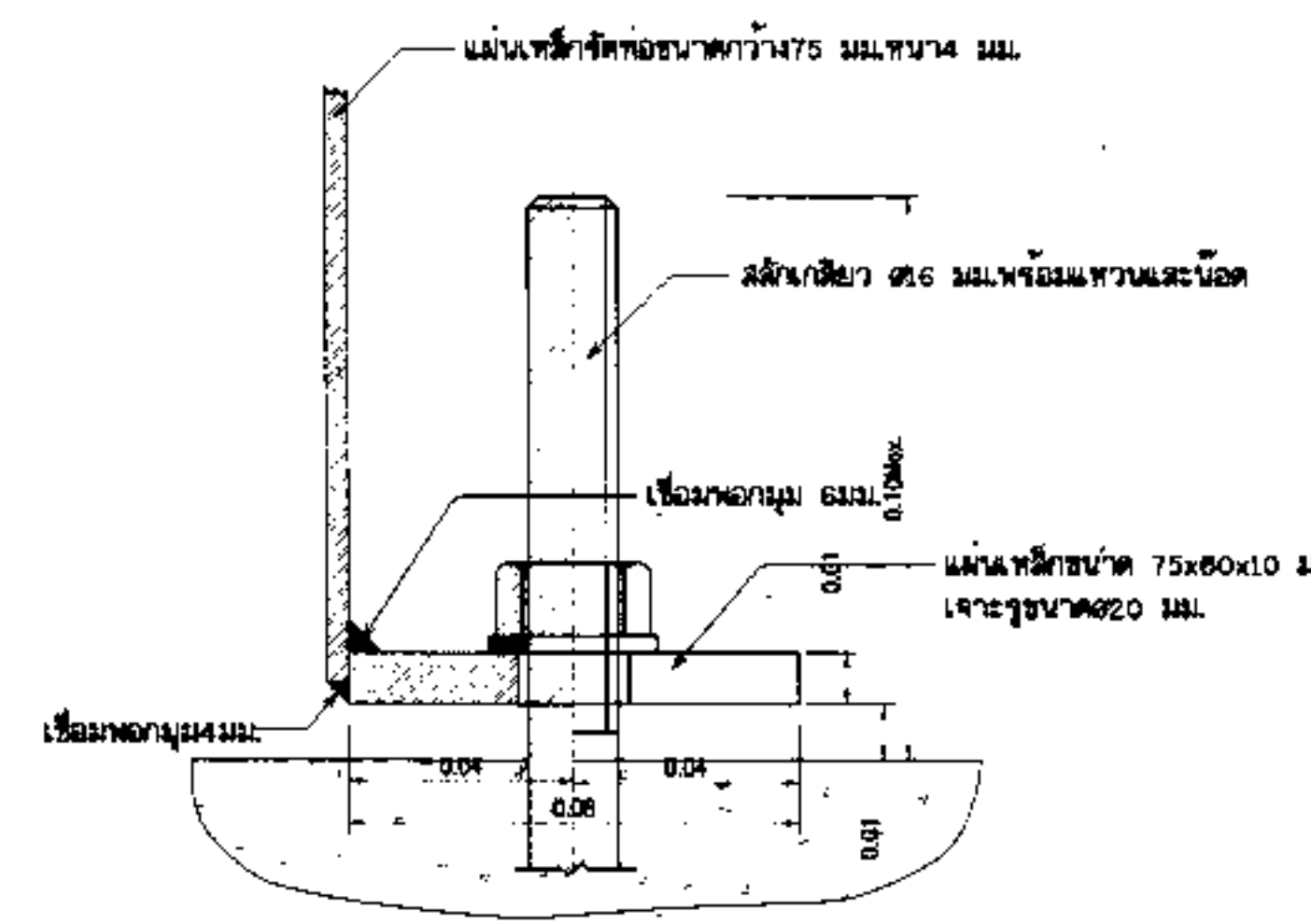
รูปตัด ค1 - ค2 ไม่แสดงมาตราส่วน
