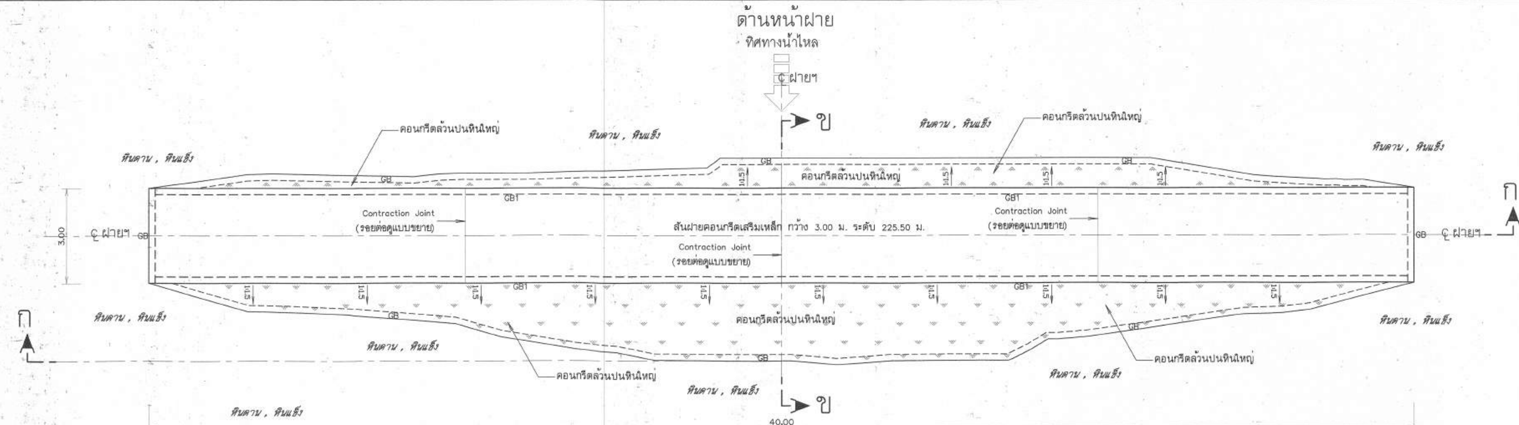
ด้านท้ายฝาย แปลนทั่วไป มาตราส่วน 1:75
