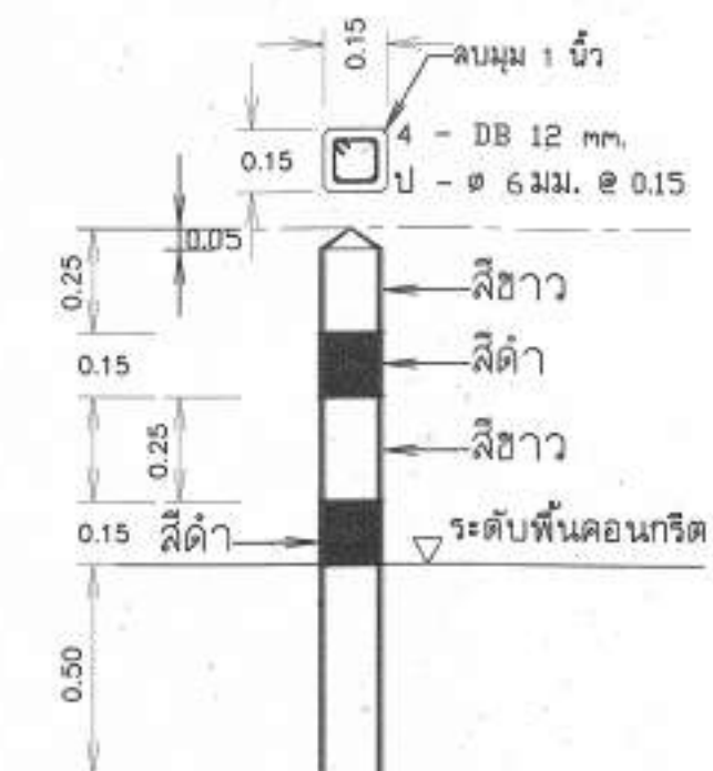
แบบขยายหลักบ่อแก้ว มาตราส่วน 1:20
