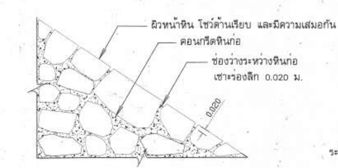
ขยายผิวหน้าคอนกรีตล้นบนหินใหญ่ ไม่มีมาตราส่วน
