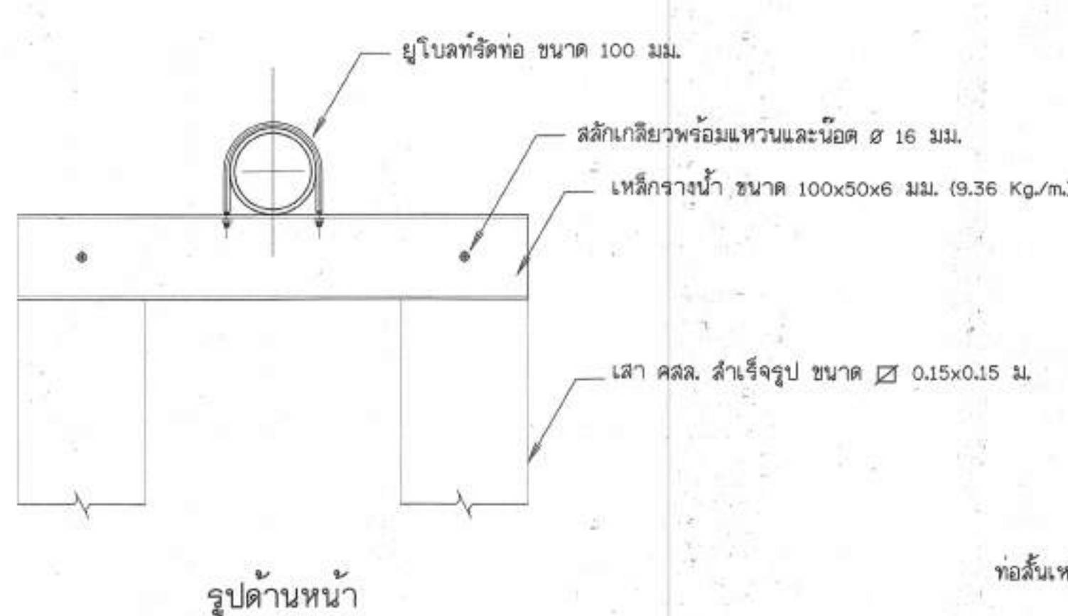
13. เสาคอม่อรับท่อชุด และแบบขยายอุปกรณ์รัดท่อ ไม่แสดงมาตราส่วน
