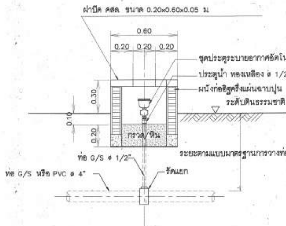
การติดตั้งประตุน้ำอากาศอัดในมิติ มาตราส่วน 1:20
