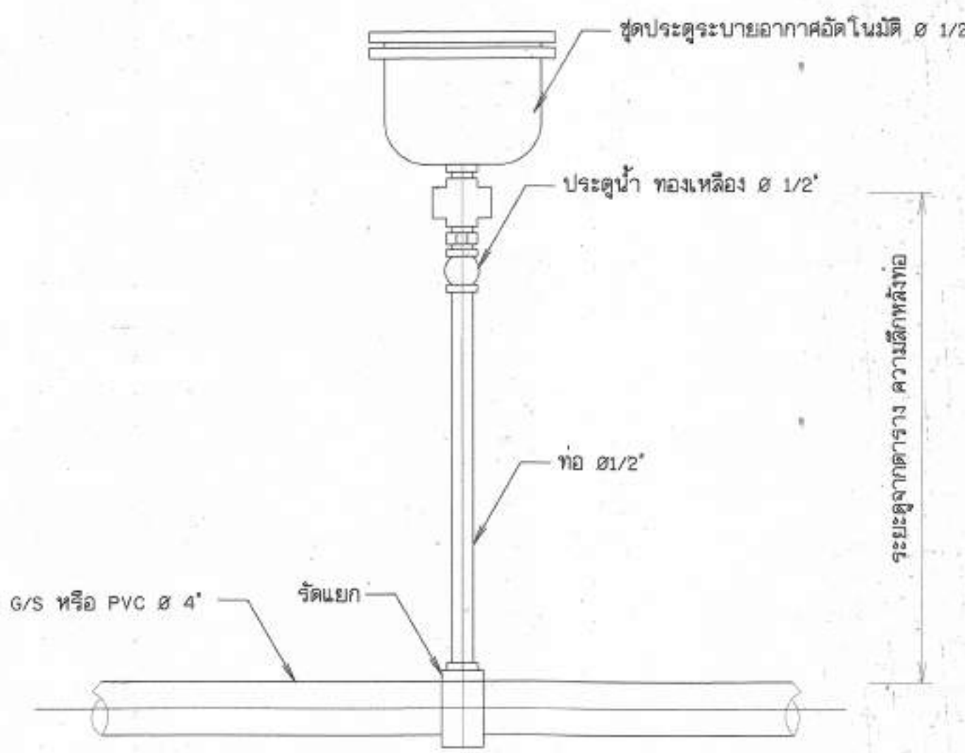
12. การติดตั้งประตูลมปรับอากาศอัตโนมัติ ไม่แสดงมาตราส่วน
