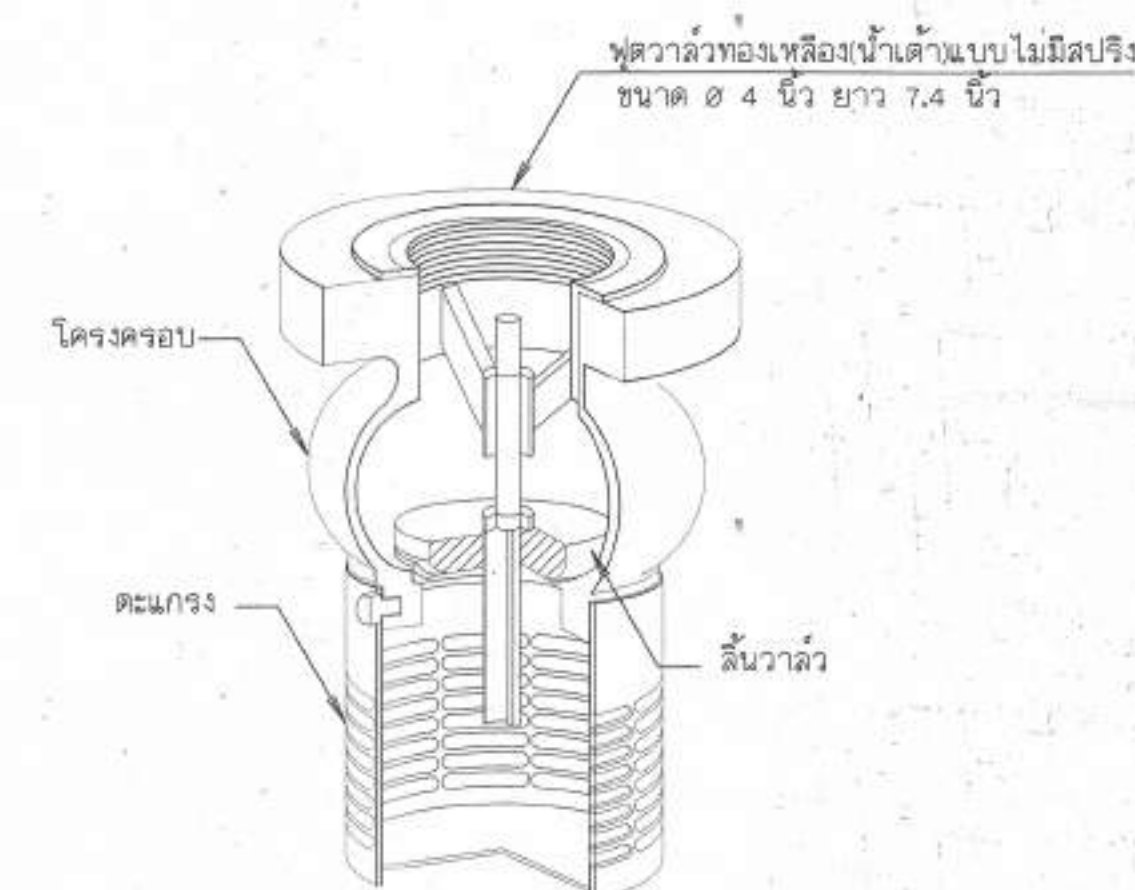
15. การต่อท่อเครื่องสูบน้ำ ไม่แสดงมาตราส่วน
