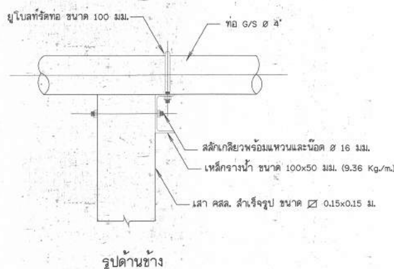
13. เสาคอม่อรับท่อชุด และแบบขยายอุปกรณ์รัดท่อ ไม่แสดงมาตราส่วน
