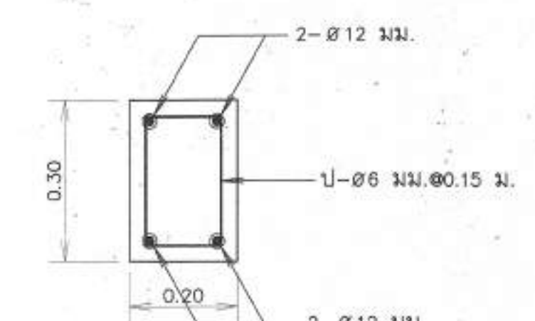
ขยายคานคอดิน GB มาตราส่วน 1:10
