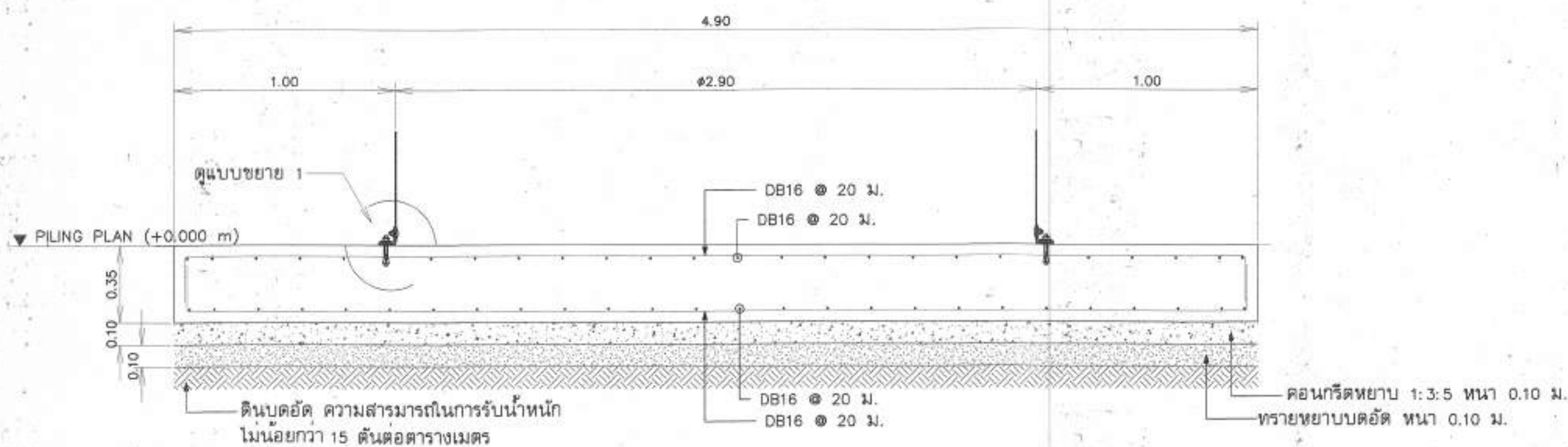
รูปตัด ก - ก
