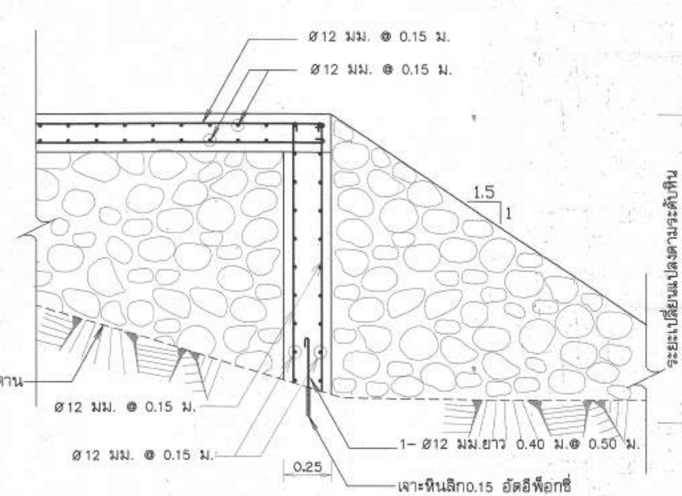
รูปตัดแสดงการเสริมเหล็ก คาน GB1 มาตราส่วน 1:20
