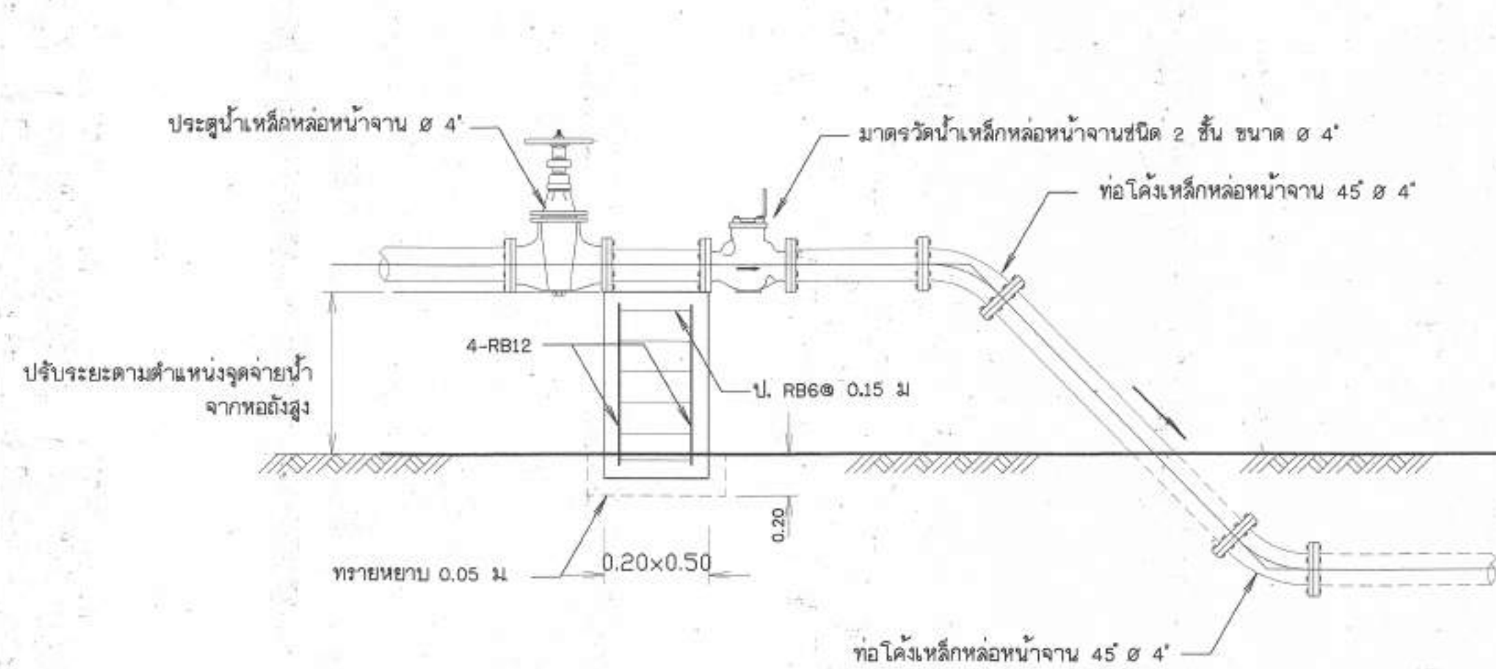
14. การติดตั้งมาตรวัดน้ำบนพื้นดิน Ø 4" ไม่แสดงมาตราส่วน
