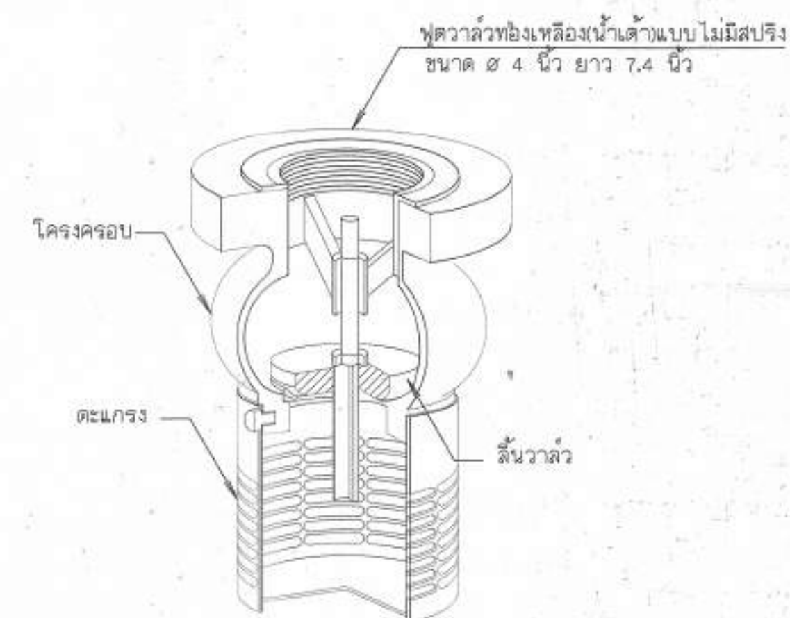
15. ฟุตวาล์วทองเหลือง (น้ำดื่ม) แบบไม่มีสปริง ไม่แสดงขนาดวาล์ว
