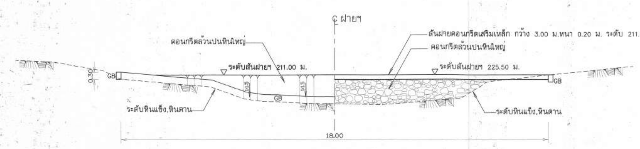
รูปตัด ก-ก มาตราส่วน 1:75
