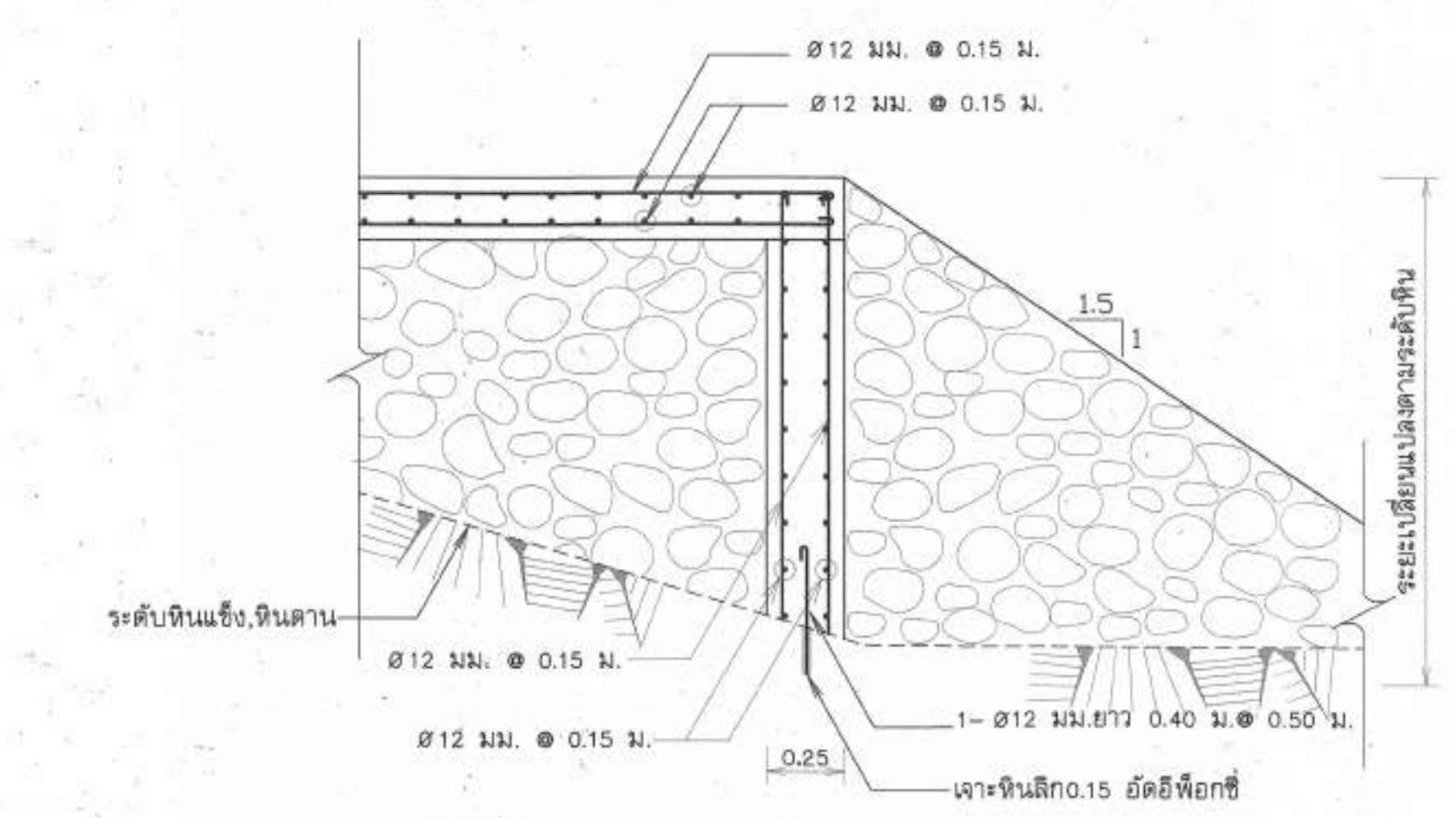
รูปตัด แสดงการเสริมเหล็ก คาน GB1 มาตราส่วน 1:20
