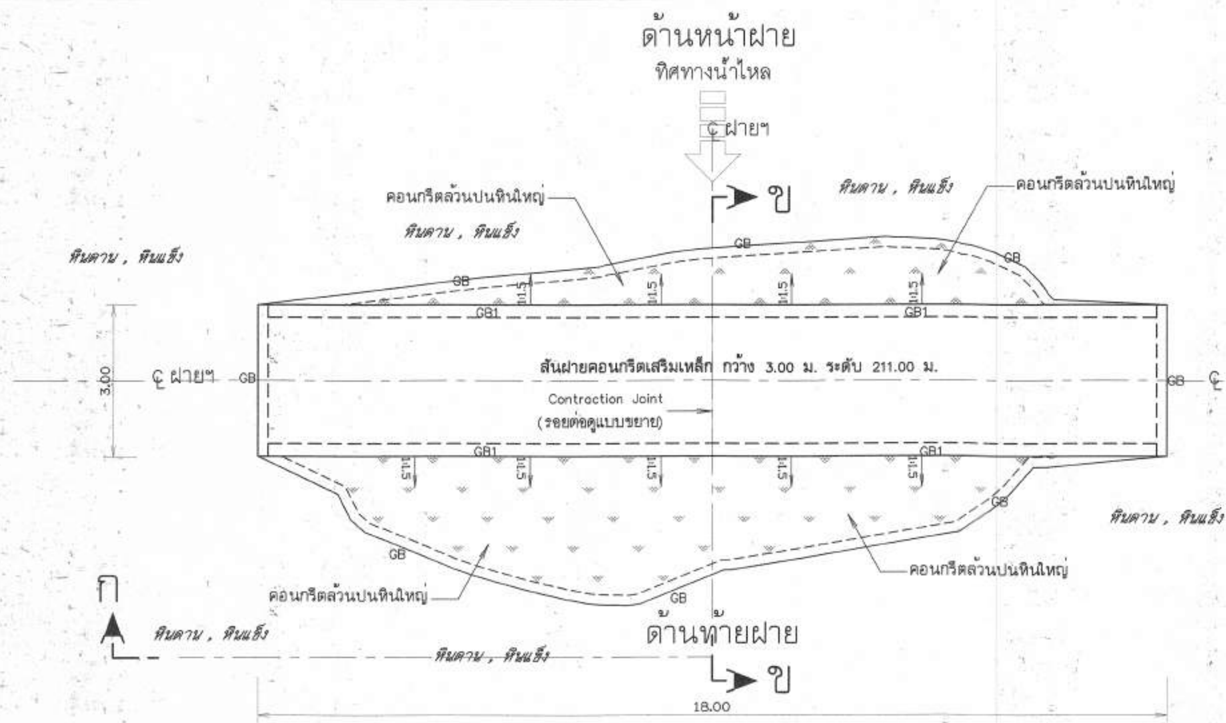
แบบแปลนทั่วไป มาตราส่วน 1:75
