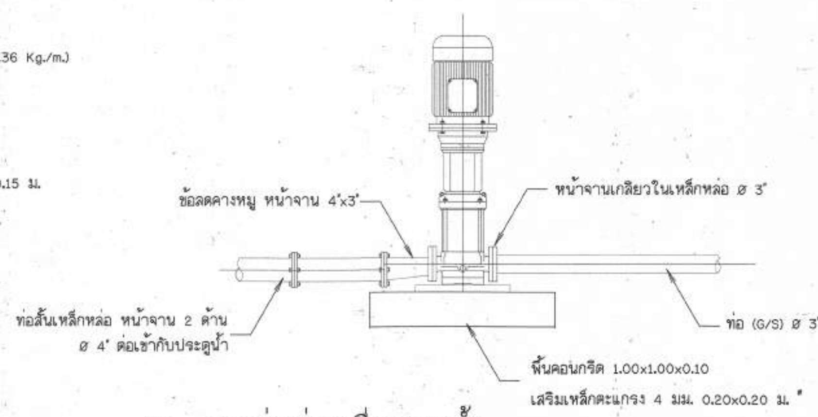
15. การต่อท่อเครื่องสูบน้ำ ไม่แสดงขนาดวาล์ว
