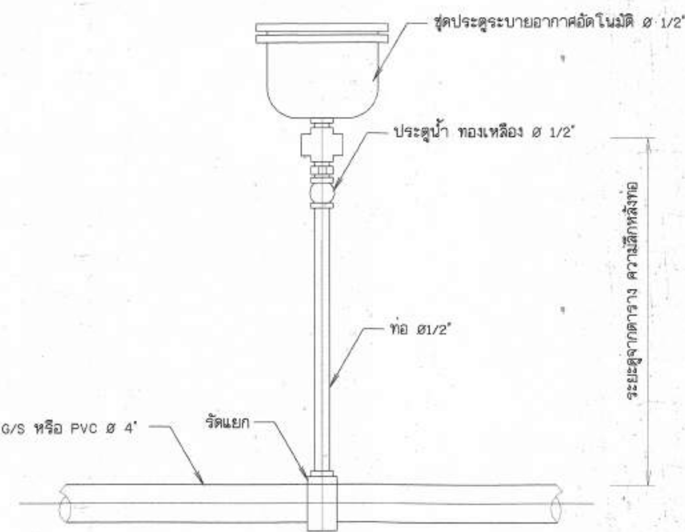
12. การติดตั้งประตูปะบายอากาศอัดโนมัติ ไม่แสดงขนาดวาล์ว
