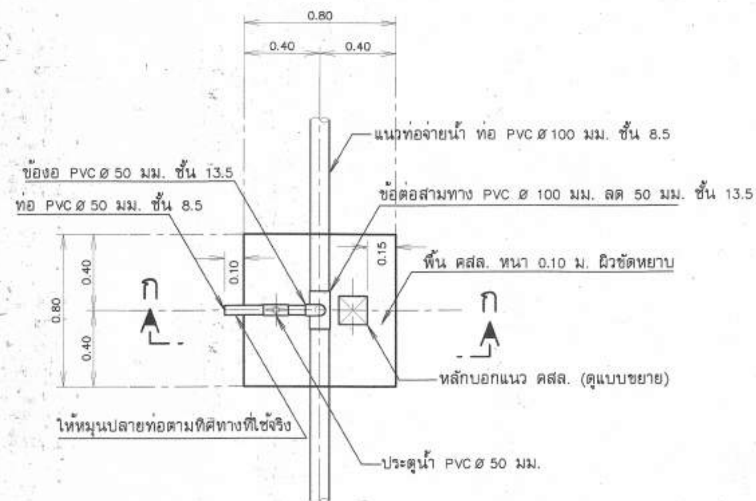
แบบแปลนอาคารจุดปล่อยน้ำ มาตราส่วน 1:20
