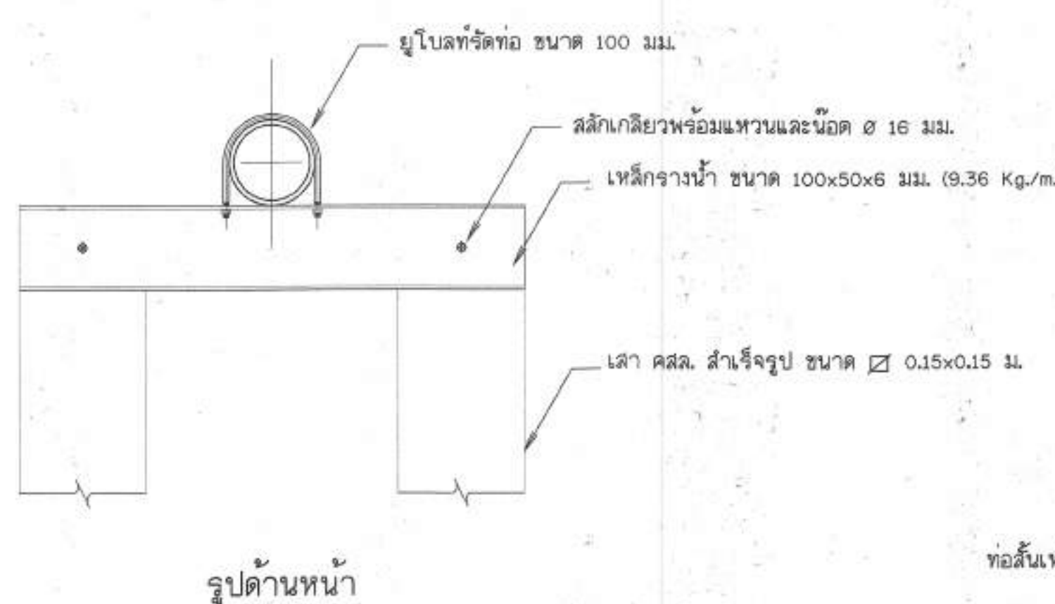
13. เสาคอมม่อนรับท่อดูด และแบบขยายอุปกรณ์วัดท่อ ไม่แสดงขนาดวาล์ว
