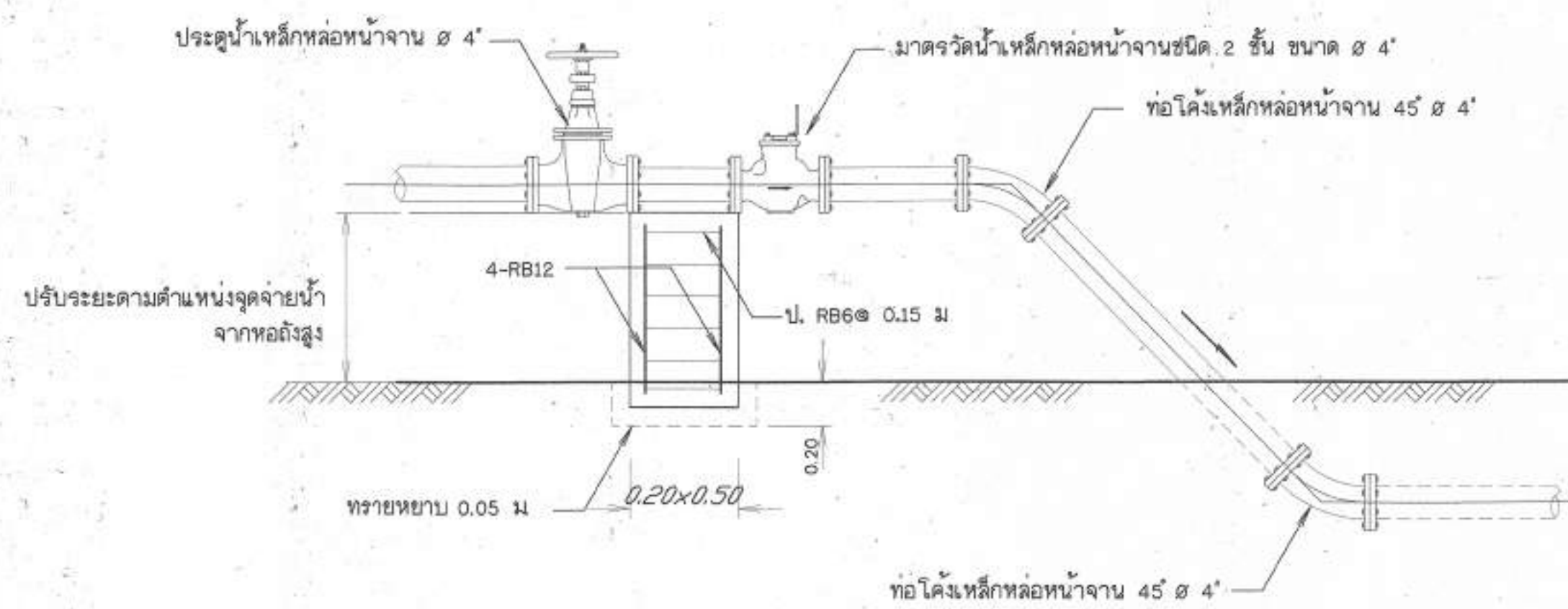
14. การติดตั้งมาตรวัดน้ำบนพื้นดิน Ø 4" ไม่แสดงขนาดวาล์ว
