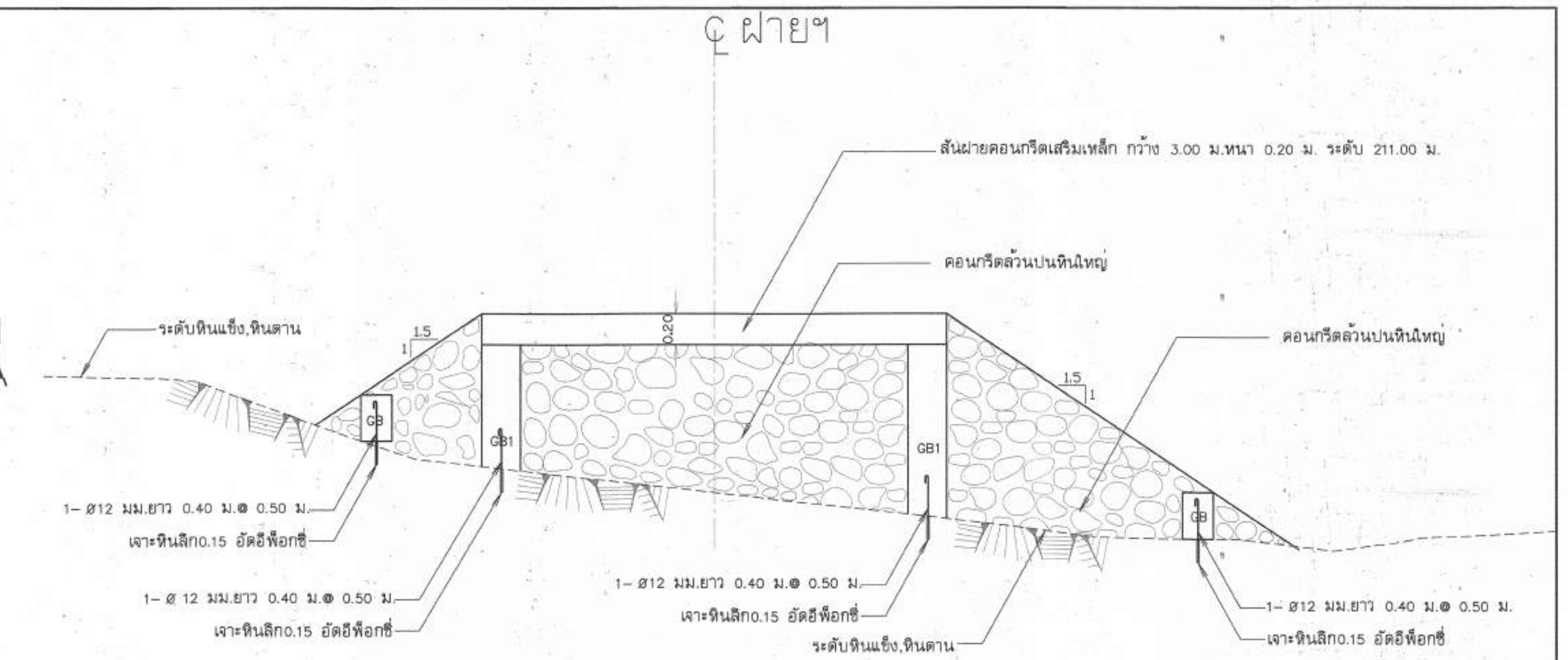
รูปตัด ข-ข มาตราส่วน 1:25
