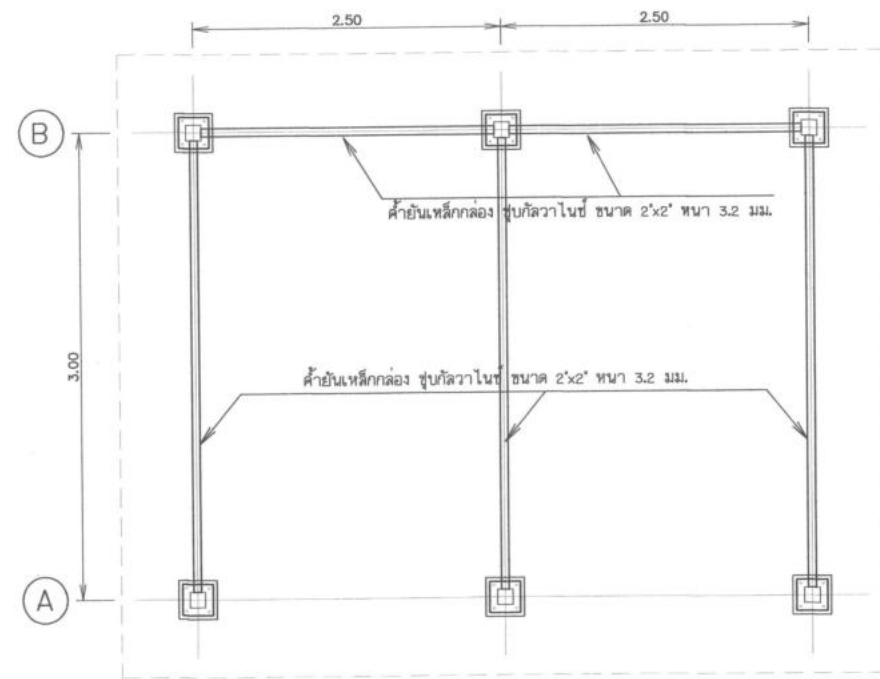
รูปแสดงค้ำยันโครงสร้างรับแผง ชั้น 2 ไม่แสดงขนาดจั่วส่วน
