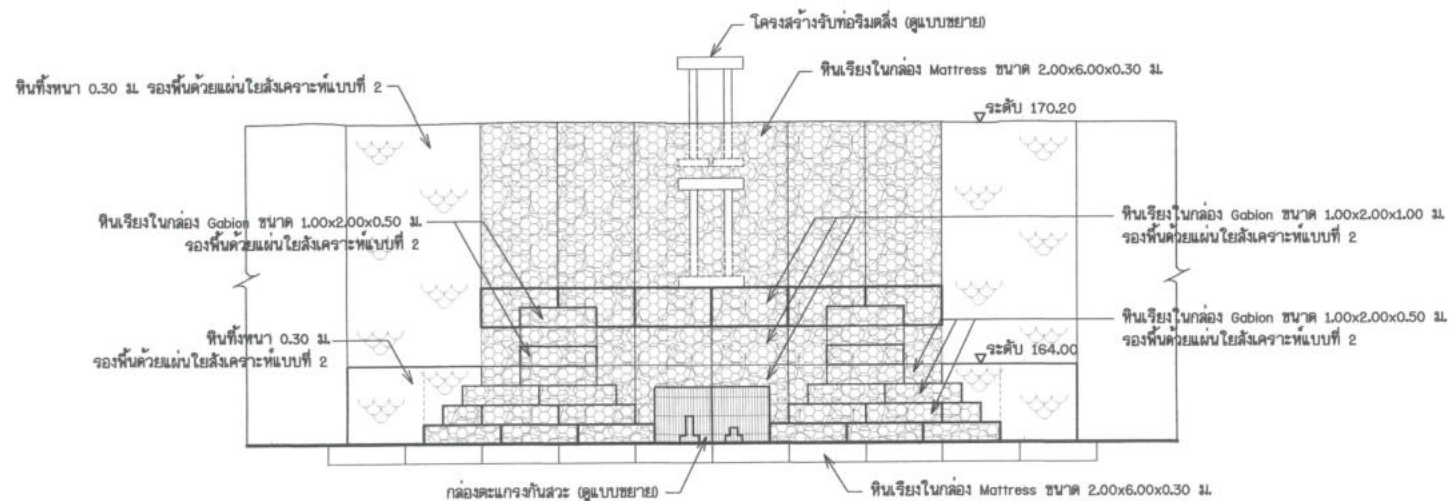
รูปด้าน 1 ไม่แสดงขนาดราส่วน
