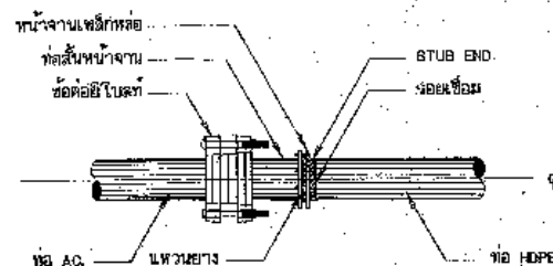
การบรรจุบดท่อ AC กับท่อ HDPE
