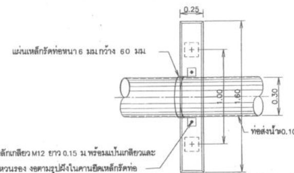
รายละเอียดแผ่นเหล็กยึดท่อ ไม่แสดงขนาดราส่วน
