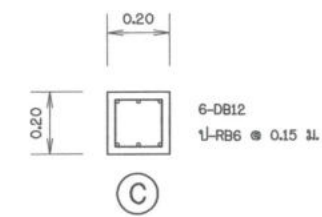
ขยายโครงสร้างรับท่อริมตลิ่ง ไม่แสดงขนาดราส่วน
