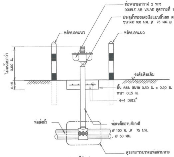
รูปแสดงการติดตั้งท่อระบายอากาศ มาตราส่วน 1:20
