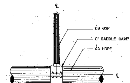
การบรรจุบดท่อสามทาง HDPE กับท่อ GSP
