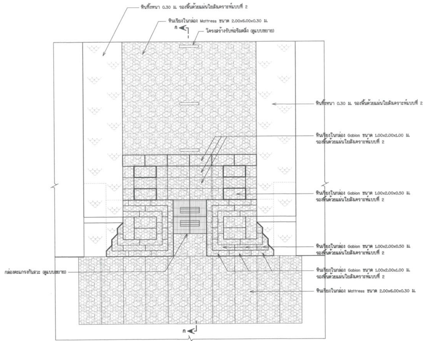
แปลนแสดงบ่อสูบน้ำ ไม่แสดงขนาดราส่วน
