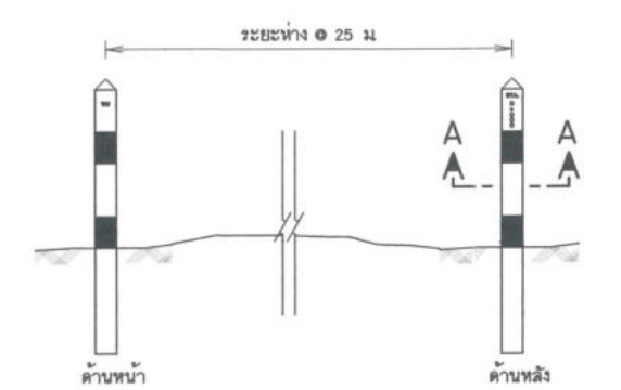
แสดงการวางหลักบอกแนวท่อ มาตราส่วน 1:20
