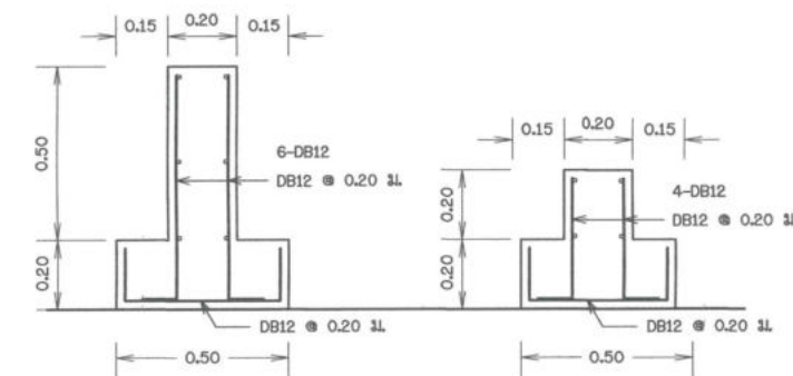
ขยายแท่นรับเครื่องสูบน้ำ ไม่แสดงขนาดราส่วน
