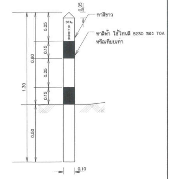
แสดงลัดส่วนหลักบอกแนวท่อ มาตราส่วน 1:10
