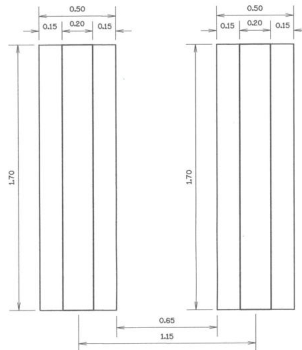
แปลนแท่นรับเครื่องสูบน้ำ ไม่แสดงขนาดราส่วน
