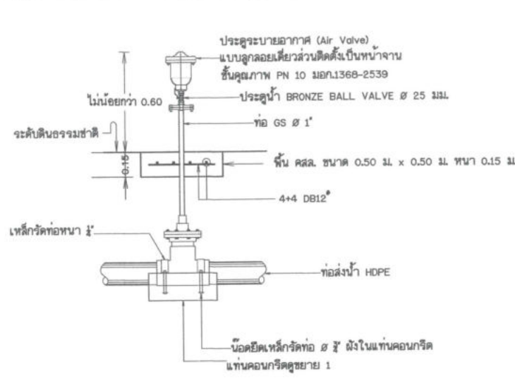
รูปตัดอาคารท่อระบายอากาศ Ø 25 มม. (ใช้สำหรับท่อส่งน้ำที่มีขนาดไม่เกิน 6 นิ้ว) มาตราส่วน 1:20
