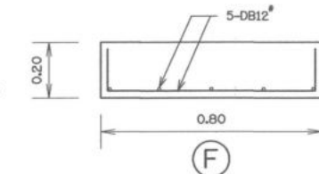
ขยายโครงสร้างรับท่อริมตลิ่ง ไม่แสดงขนาดราส่วน
