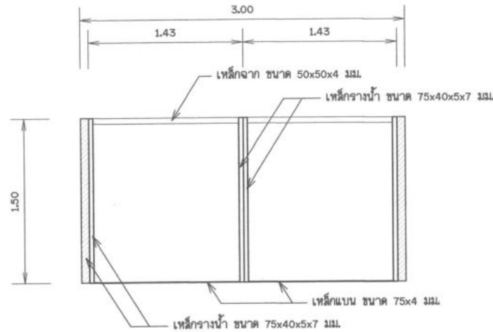
รูปด้าน 1 ไม่แสดงขนาดราส่วน
