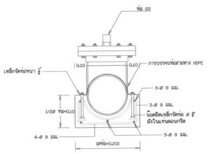
รูปตัดขยาย "1" มาตราส่วน 1:10
