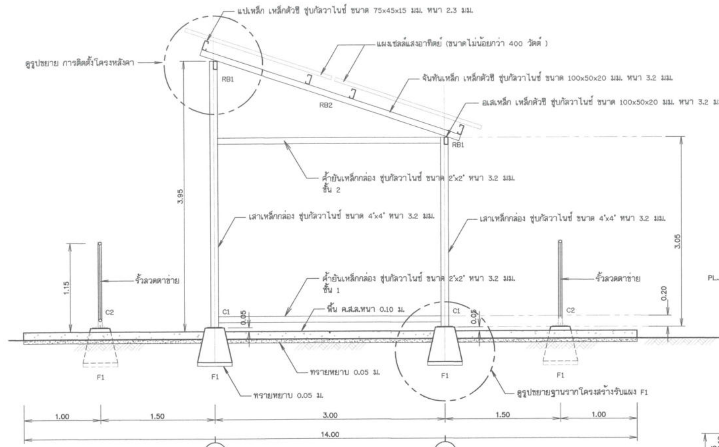
รูปด้านข้าง ไม่แสดงขนาดจั่วส่วน
