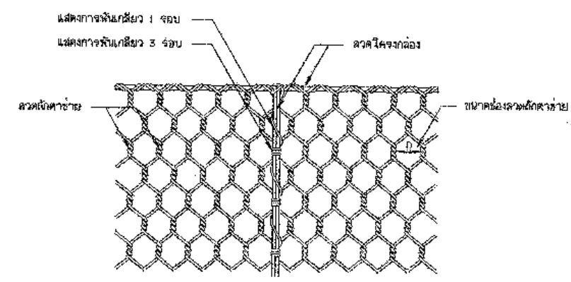
รูปแสดงการพันลวดระหว่างกล่องลวดตาข่ายและเสาปิด
