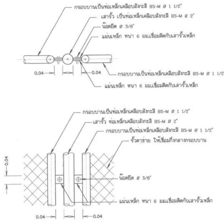
แบบขยายบานพับยึดเหล็ก
