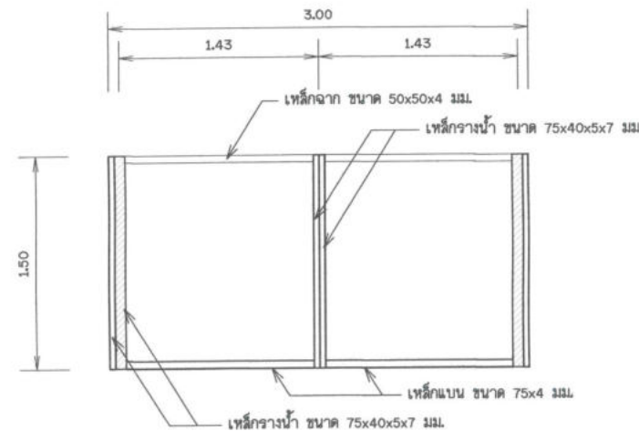
รูปด้าน 2 ไม่แสดงขนาดราส่วน
