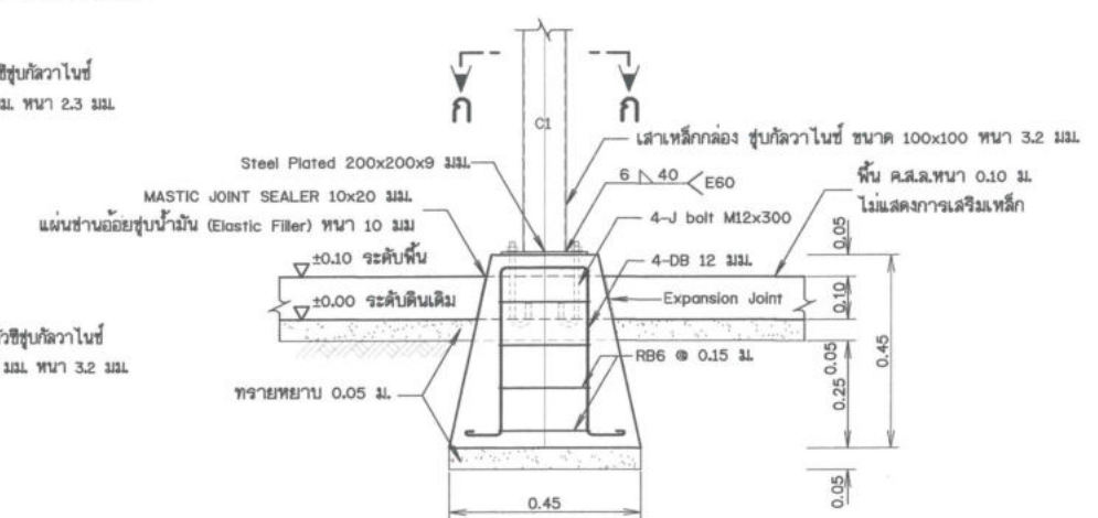
รูปขยายฐานรากโครงสร้างรับแผง F1 (ต่อม่อ คสล. หล่อสำเร็จรูปพร้อมติดตั้ง) ไม่แสดงขนาดจั่วส่วน
