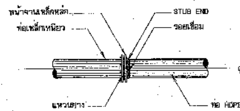
การบรรจุบดท่อเหล็กเหนียวกับท่อ HDPE
