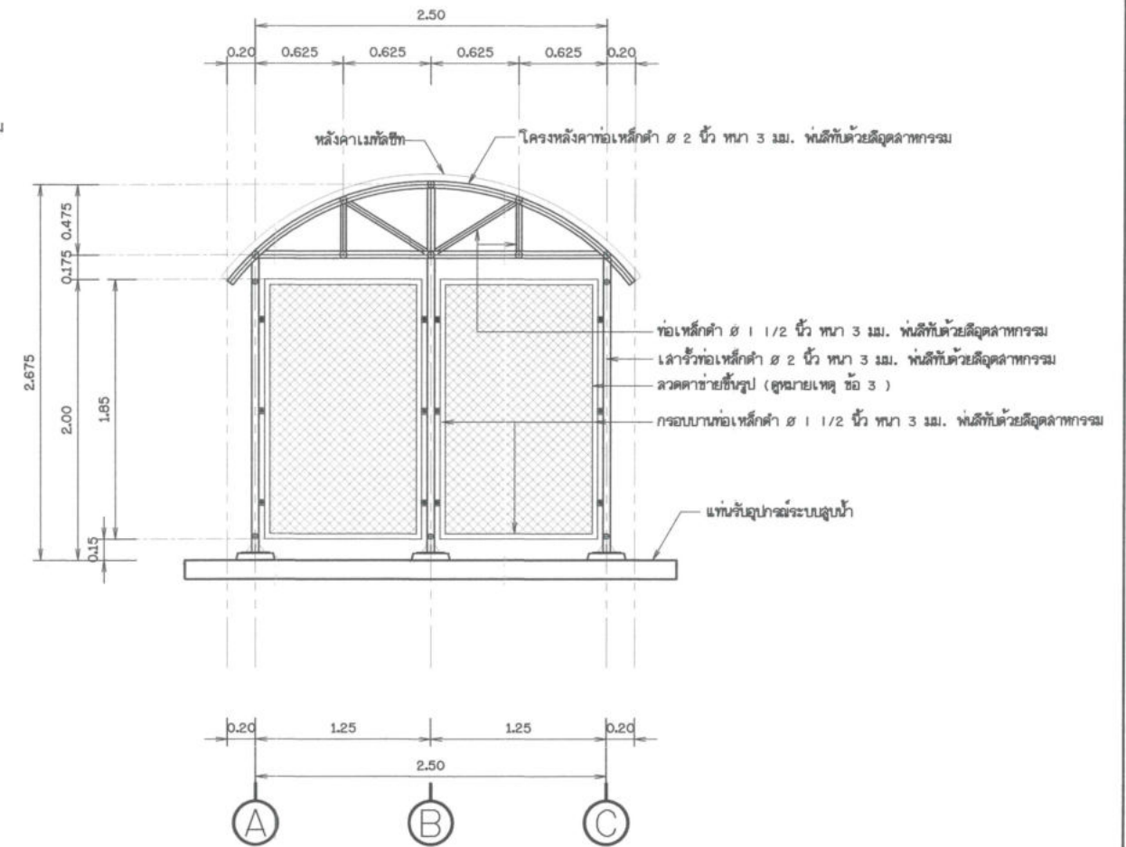
รูปตัด ข - ข ไม้แฉ่งขนาดราวสาม
