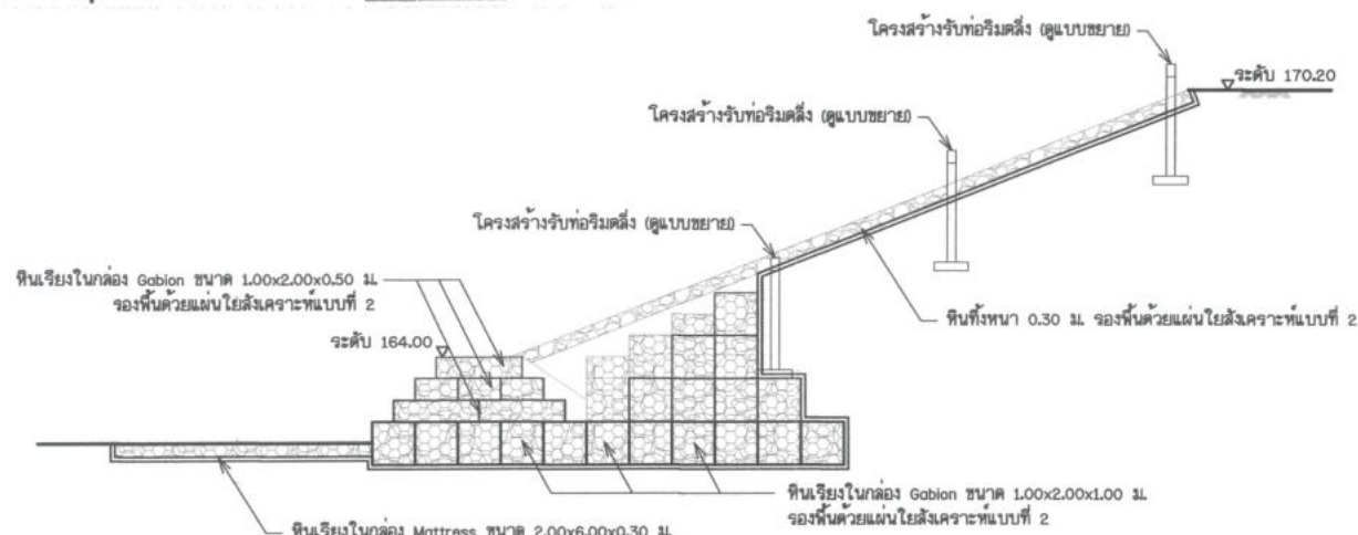
รูปตัด ก - ก ไม่แสดงขนาดราส่วน
