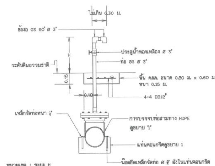
หมายเหตุ : ระยะ H ไม่เกิน 0.60 ม. สำหรับประตูปะบายตะกอน รูปตัดอาคารประตูปะบายตะกอน Ø 75 มม. มาตราส่วน 1:20
