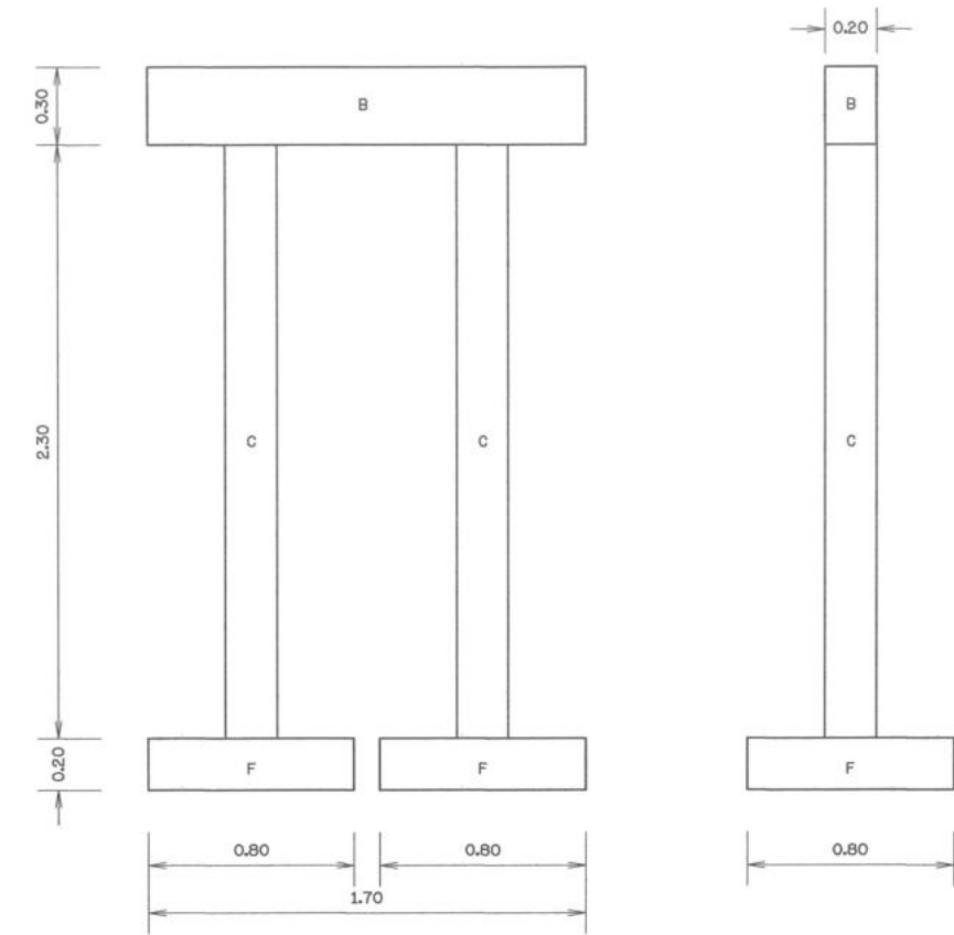
แบบโครงสร้างรับท่อริมตลิ่ง ไม่แสดงขนาดราส่วน
