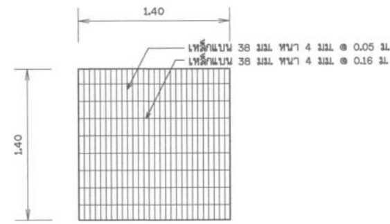
ฝาตะแกรงกันสวะ (ด้านบน) ไม่แสดงขนาดราส่วน
