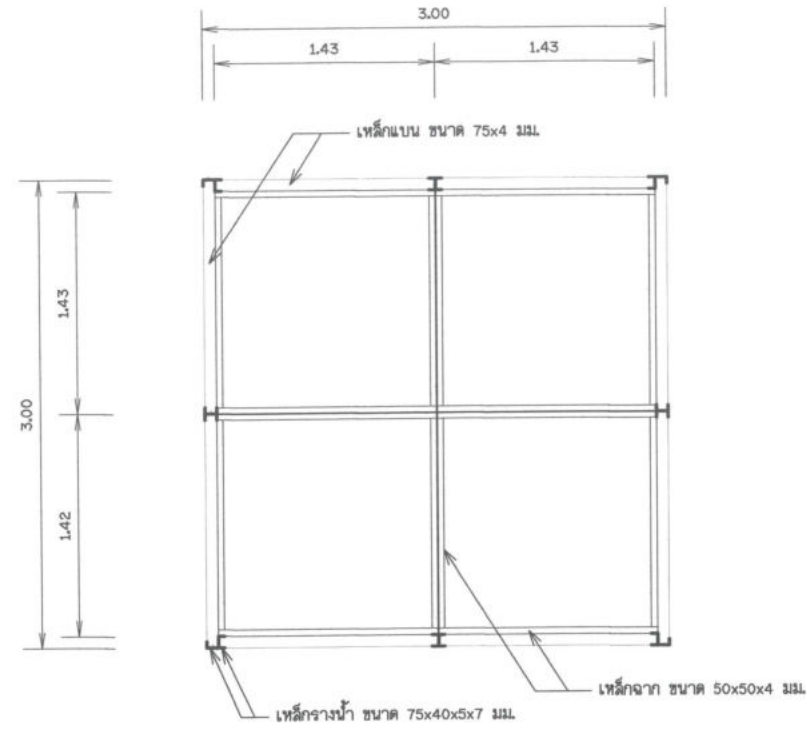
แปลนกล่องตะแกรงกันสวะ ไม่แสดงขนาดราส่วน
