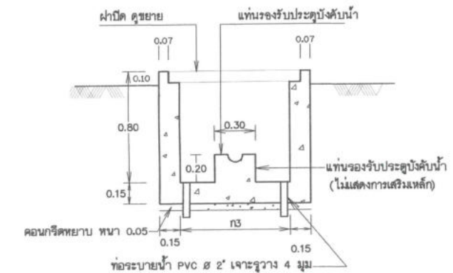
รูปตัด 1 - 1 มาตราส่วน 1:20
