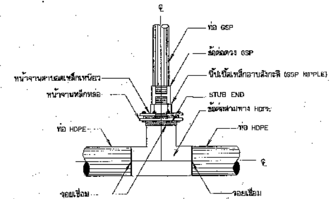
การบรรจุบดท่อสามทาง HDPE กับท่อ GSP แบบข้อต่อ
