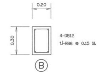
แบบโครงสร้างรับท่อริมตลิ่ง ไม่แสดงขนาดราส่วน
