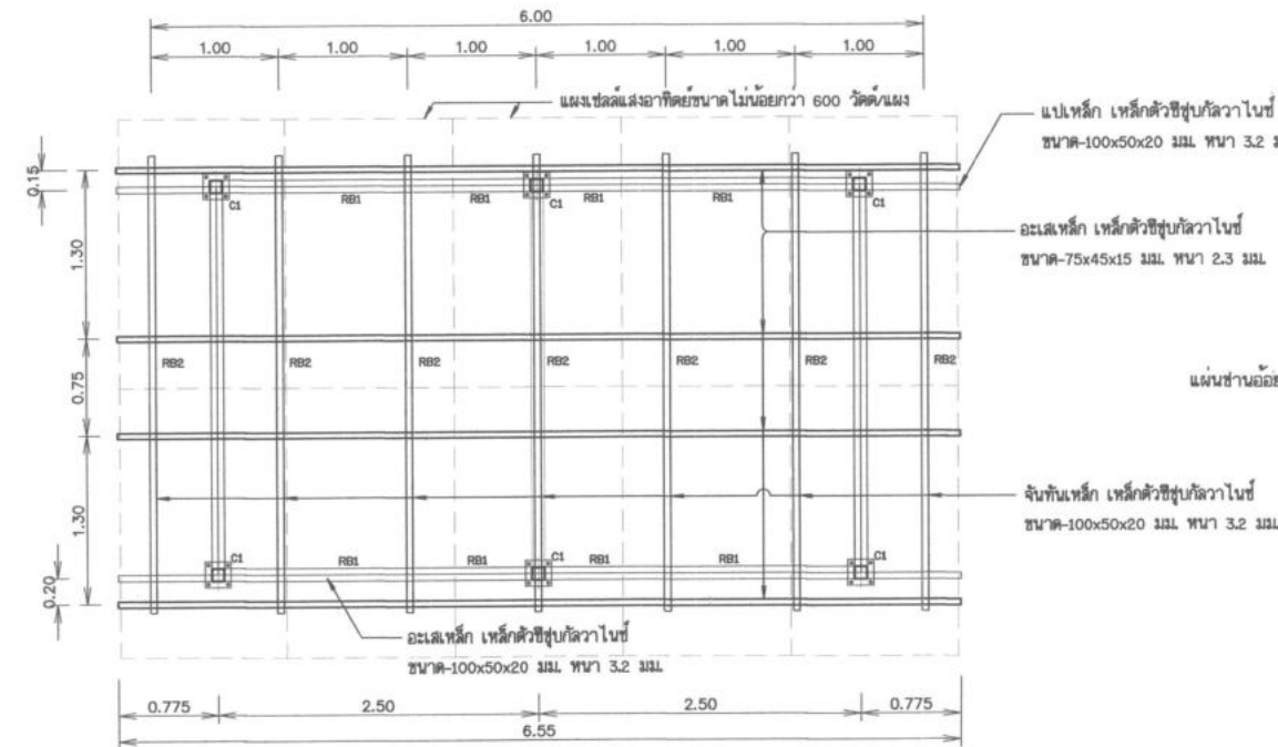
แปลนฐานรากและโครงหลังคาชั้น 1 จำนวน 10 แผง ไม่แสดงขนาดจั่วส่วน
