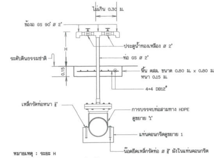
หมายเหตุ : ระยะ H ไม่เกิน 0.60 ม. สำหรับจุดปล่อยน้ำ รูปตัดอาคารจุดปล่อยน้ำ 2 ด้าน มาตราส่วน 1:20
