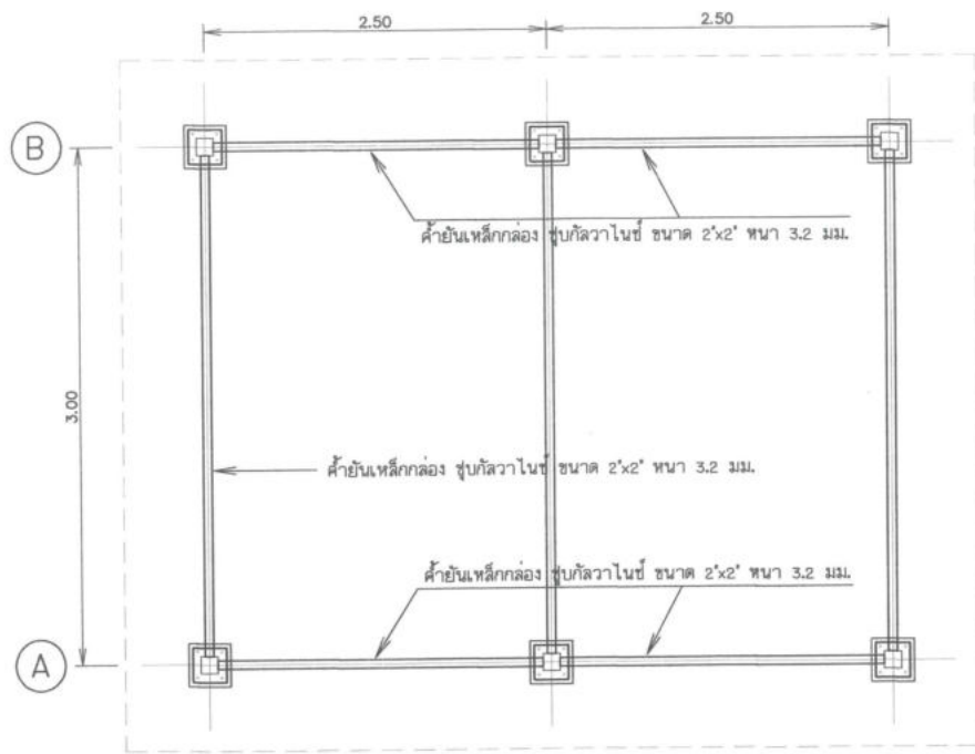
รูปแสดงค้ำยันโครงสร้างรับแผง ชั้น 1 ไม่แสดงขนาดจั่วส่วน
