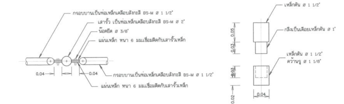
แบบขยายบานพับหัวเหล็ก
