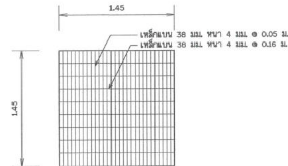
ฝาตะแกรงกันสวะ (ด้านข้าง) ไม่แสดงขนาดราส่วน
