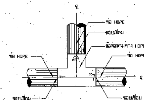
การบรรจุบดท่อสามทาง HDPE กับท่อ HDPE
