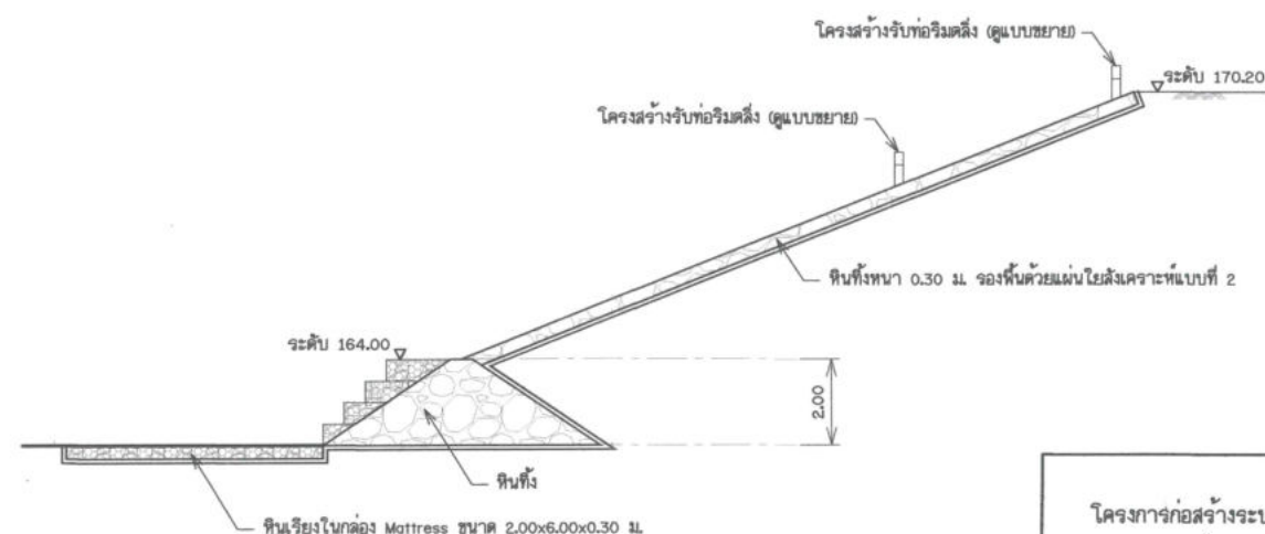
รูปด้าน 2 ไม่แสดงขนาดราส่วน
