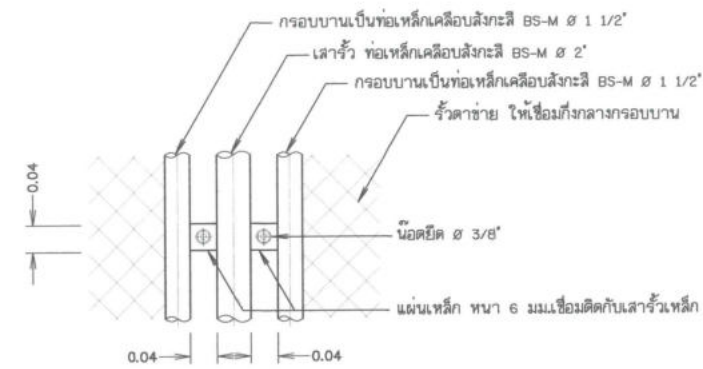
แบบขยายบานพับหัวเหล็ก
