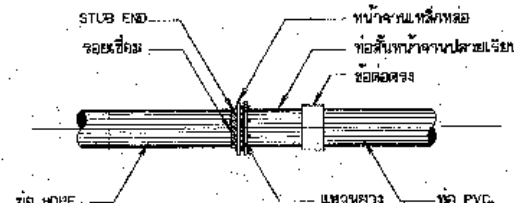
การบรรจุบดท่อ HDPE กับท่อ PVC.
