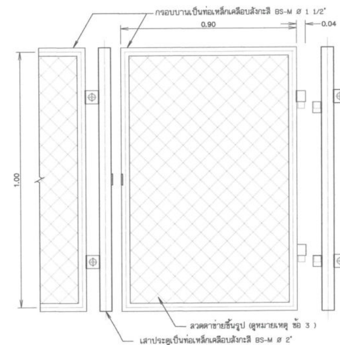
แบบขยายรายละเอียดประตู
