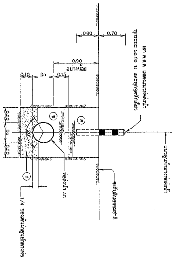
รูปตัดขวางการฝังท่อพีวีซีชนิดใยหิน (ท่อAC)
