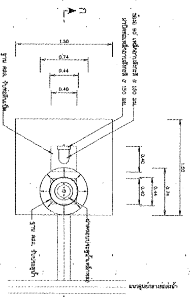
แปลนอาคารประตูประปาเขตคลอง 1:20
