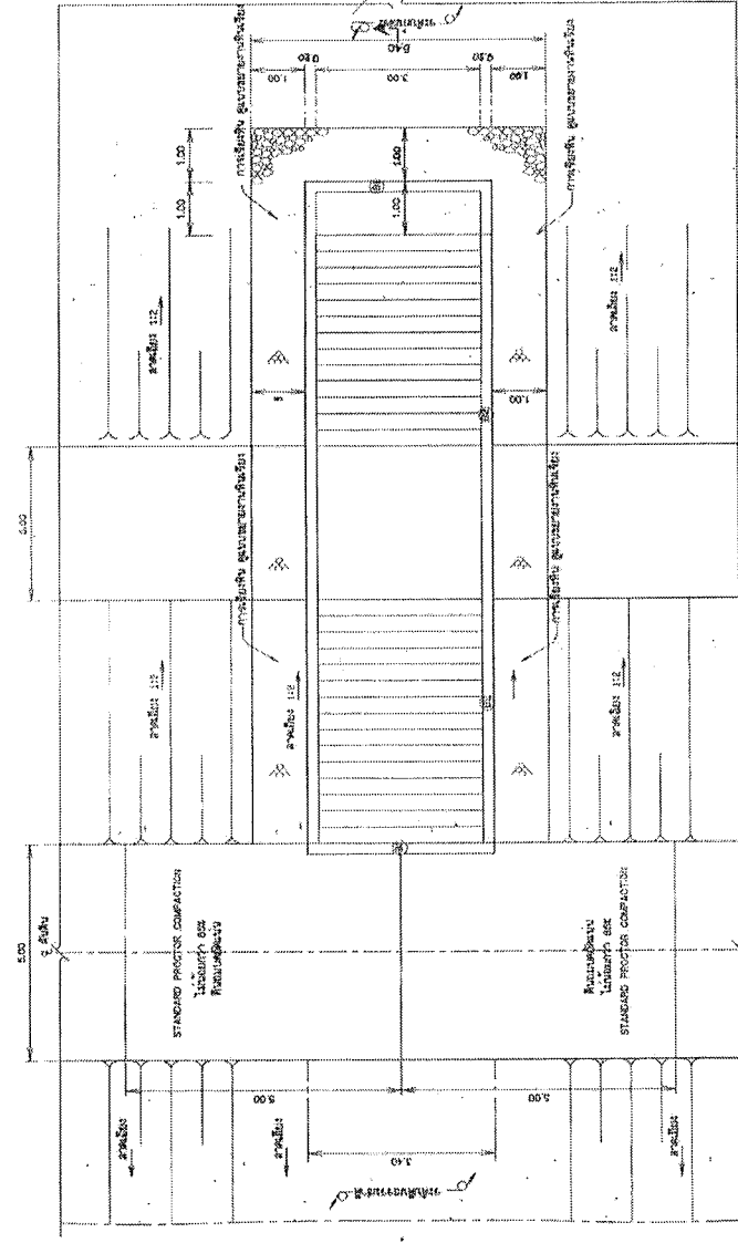
แปลนอาคารบันได คลอด
