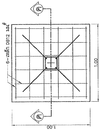
แบบขยายฐานราก F 1 : 20
