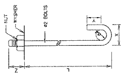
มาตรฐานการยึด HOOKED BOLT
