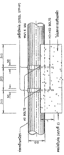
รูปตัด ข-ข
