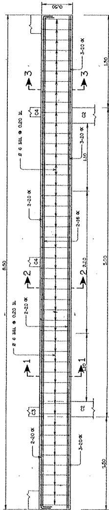
คาน RB1
