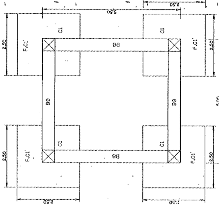
แปลนฐานรากคานายึด มาตราส่วน 1:50
