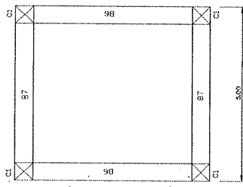
แปลนคานายึด มาตราส่วน 1:50
