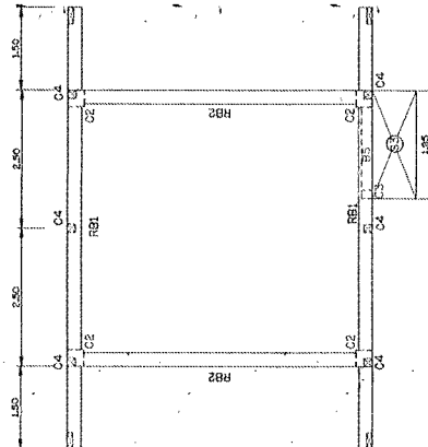
แปลนคานหลังคา
