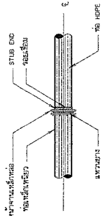
การประจบท่อเชื่อมเหล็กกับท่อ HDPE
