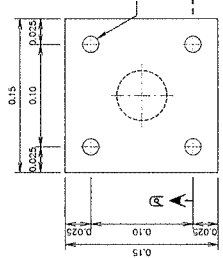
รูปขยายแผนผังหลักหน้าแปลน
