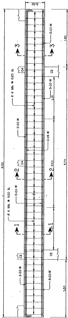
คาน RB1 มาตราส่วน 1:20
