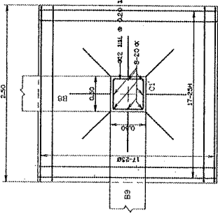
แปลนฐานราก F.C1 ขนาดส่วน 1:25
