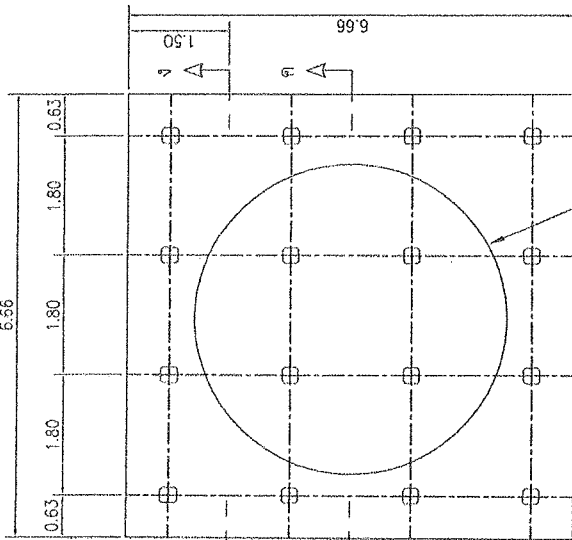
แปลฐานรากแบบฐานแผ่ NOT TO SCALE
