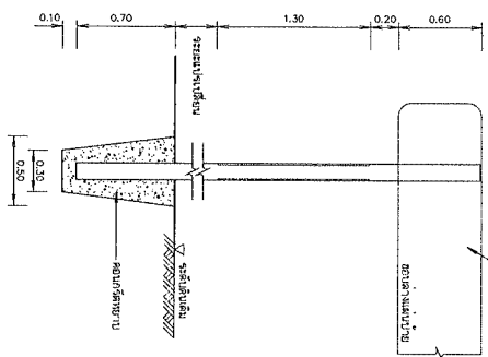
รายละเอียดการติดตั้งเสาป้าย มาตราส่วน 1:20
