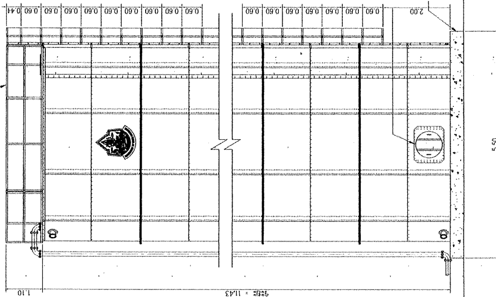
รูปตัด ๑-๒ NOT TO SCALE
