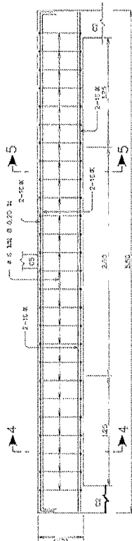
คาน RB2 ขนาด 1:20
