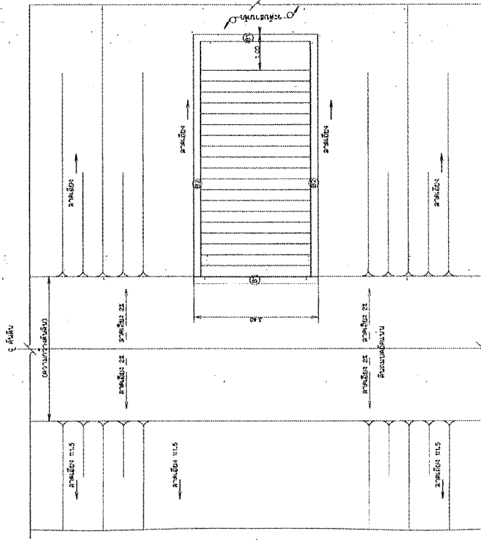
แปลนอาคารบันได คลัง
