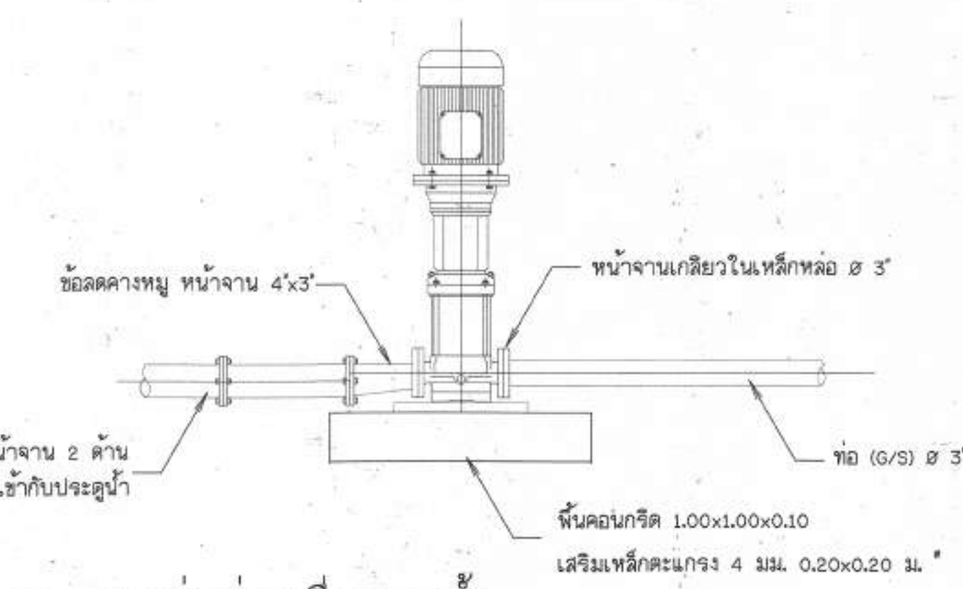
15. การต่อท่อเครื่องสูบน้ำ ไม่แสดงขนาดวาล์ว
