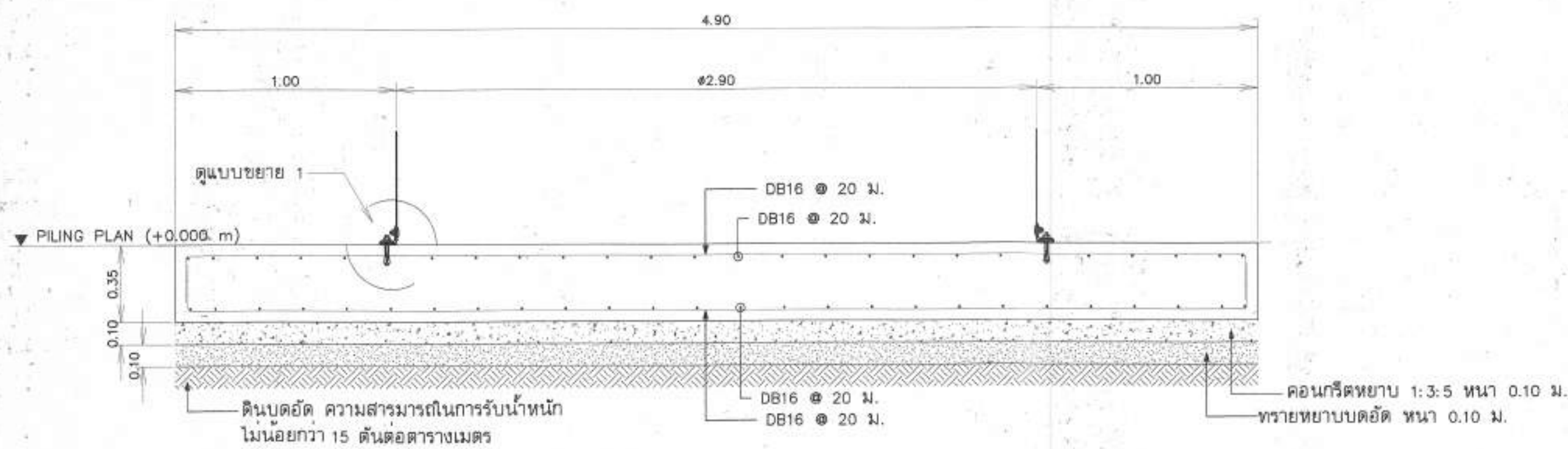
รูปตัด ก - ก มาตราส่วน 1:20
