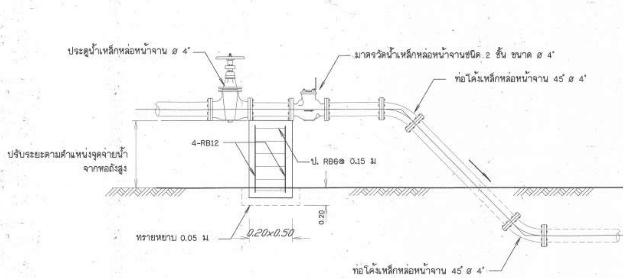
14. การติดตั้งมาตรวัดน้ำบนพื้นดิน ๑ 4" ไม่แสดงขนาดวาล์ว
