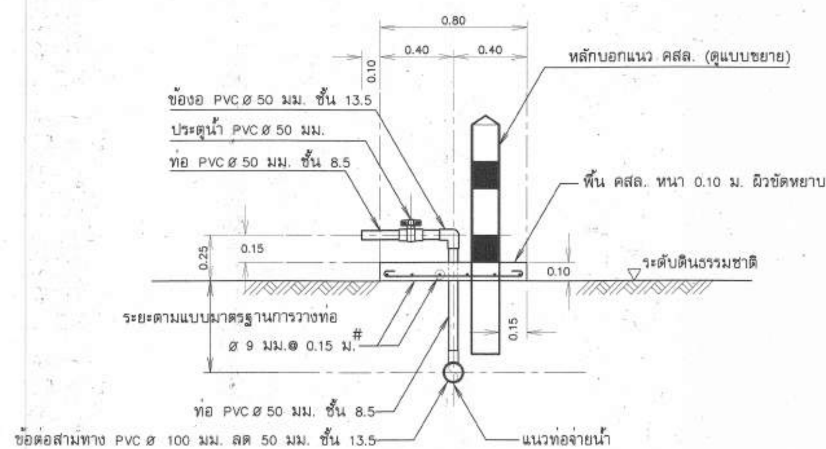
รูปตัด ก - ก แสดงการติดตั้งอาคารจุดปล่อยน้ำ มาตราส่วน 1:20
