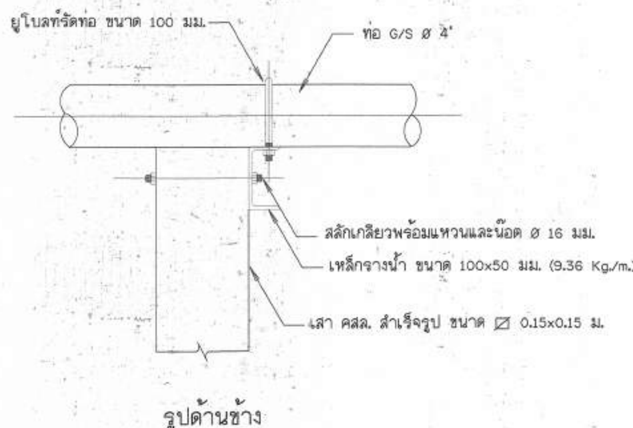
13. เสาดอม่อรับท่อชุด และแบบขยายอุปกรณ์วัดท่อ ไม่แสดงขนาดวาล์ว
