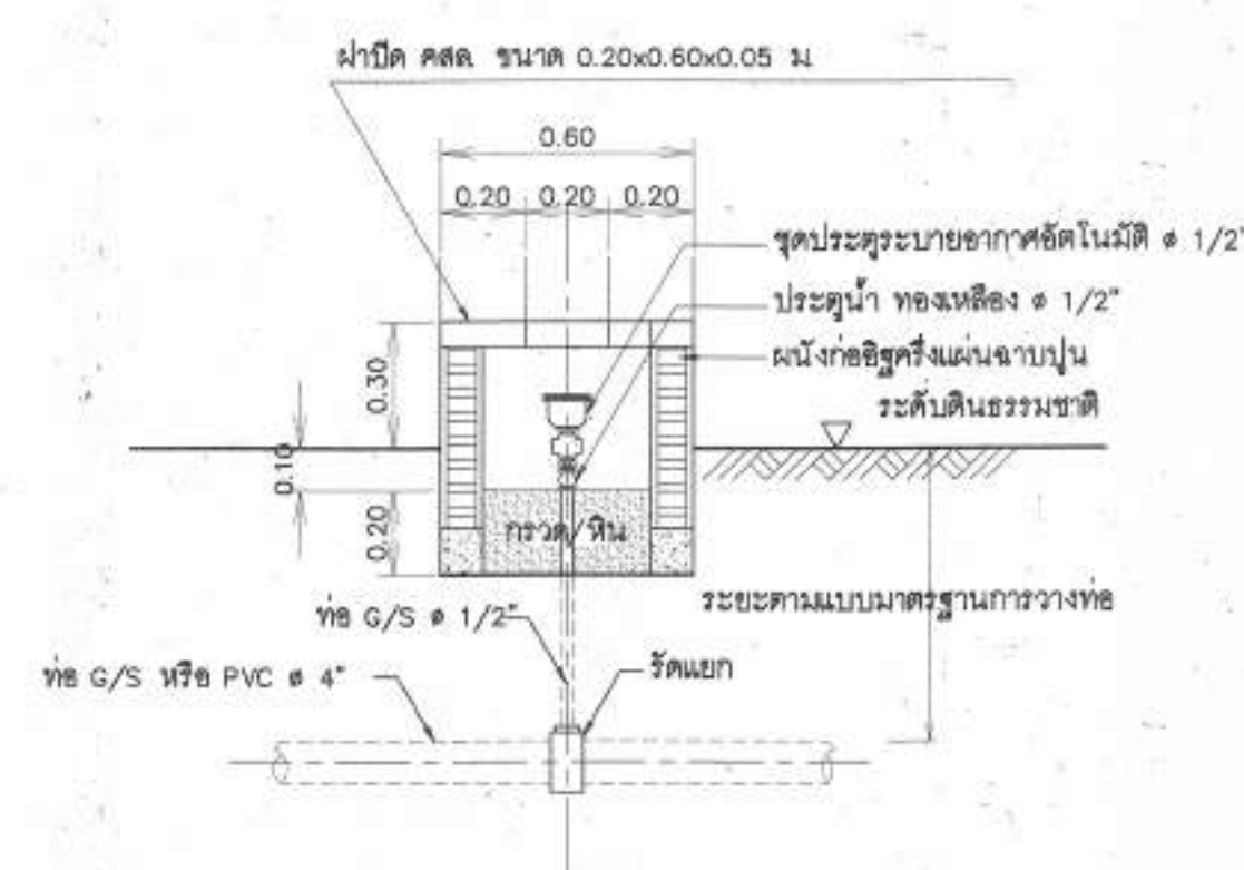
การติดตั้งประตูประบายอากาศอัตโนมัติ มาตราส่วน 1:20
