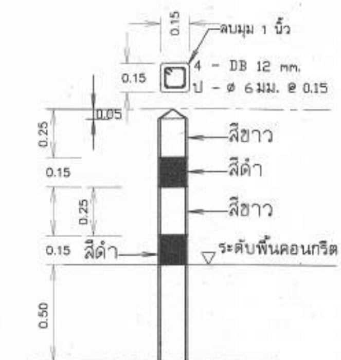
แบบขยายหลักบอกแนว มาตราส่วน 1:20
