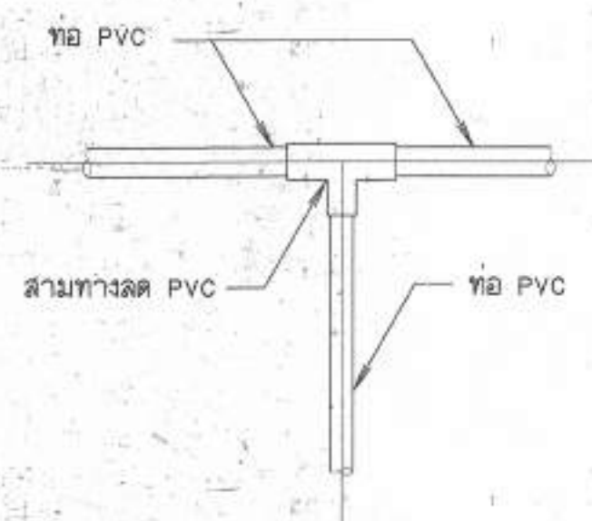
9. แบบการต่อสามทางลด PVC ไม่แสดงขนาดวาล์ว
