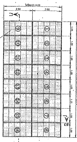
แปลนแผ่นเหล็กและอาภัพขนาด 400 วัตต์ NOT TO SCALE
