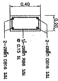
แบบขยายความ GB 1 : 20
