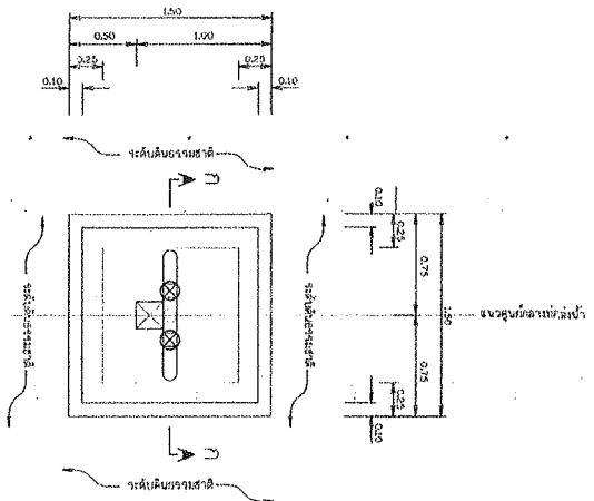
แบบอาคารจุดปล่อยน้ำ
