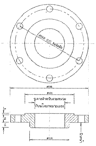
แบบแปลนหลักหล่อ 4
