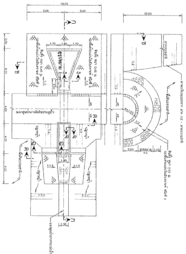
แปลนอาคารบังคับน้ำแบบท่อใต้สำหรับฝายน้ำล้น (ข)
