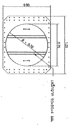
แบบขยาย 2 NOT TO SCALE
