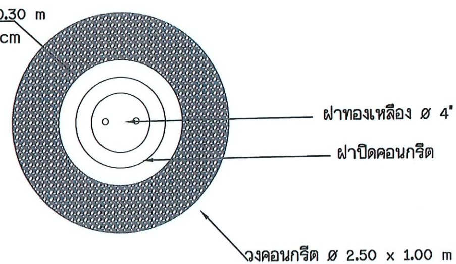
แบบบ่อวงคอนกรีตด้านบน
