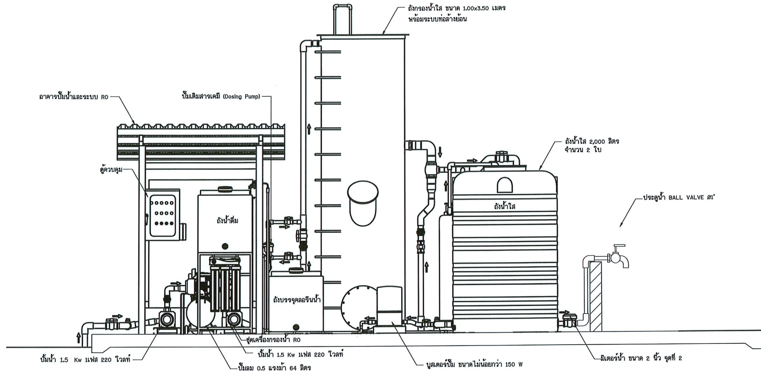
แบบแสดงแผนผังการติดตั้งระบบผลิตน้ำดื่มสะอาด
