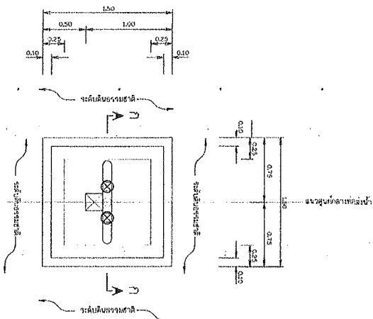
แบบอาคารจุดปล่อยน้ำ 1:20
