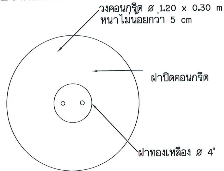
แบบบ่อวงคอนกรีตด้านบน
