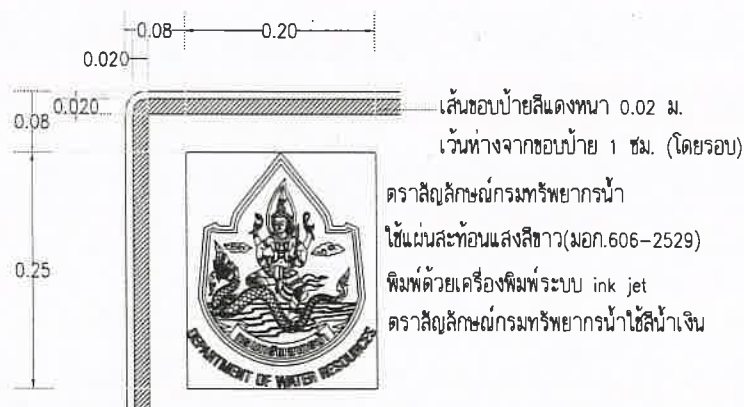
ขยายสัญลักษณ์กรมทรัพยากรน้ำ SCALE 1:10
