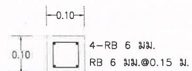
แบบขยายเหล็กเสริมหลักบ่อแกว่ง มาตราส่วน 1:15
