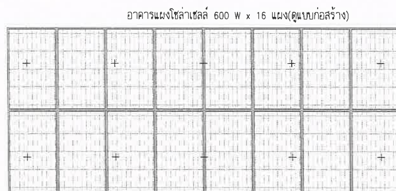
แสดงรูปแบบการวางแผงโซลาร์เซลล์ทั่วไป Solar Pump 18.5 Kw 2 ชุด SCALE 1:125
