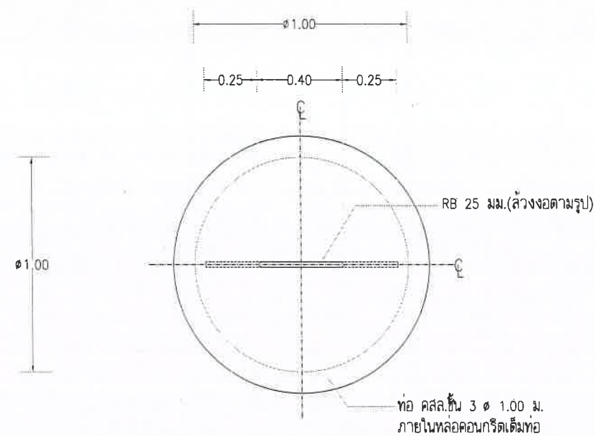
แปลนแท่นสมอยึดอาคารโรงสูบน้ำ SCALE 1:25
