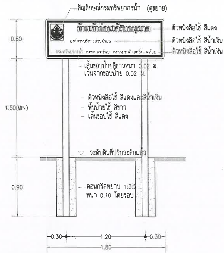
แสดงรูปด้านหน้าป้ายเตือน SCALE 1:35
