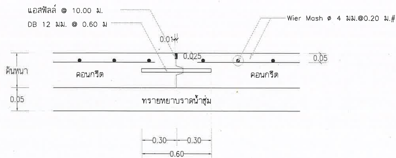
[LONGITUDINAL JOINT] เมื่อความกว้างคั่นมากกว่าหรือเท่ากับ 5.00 ม.
