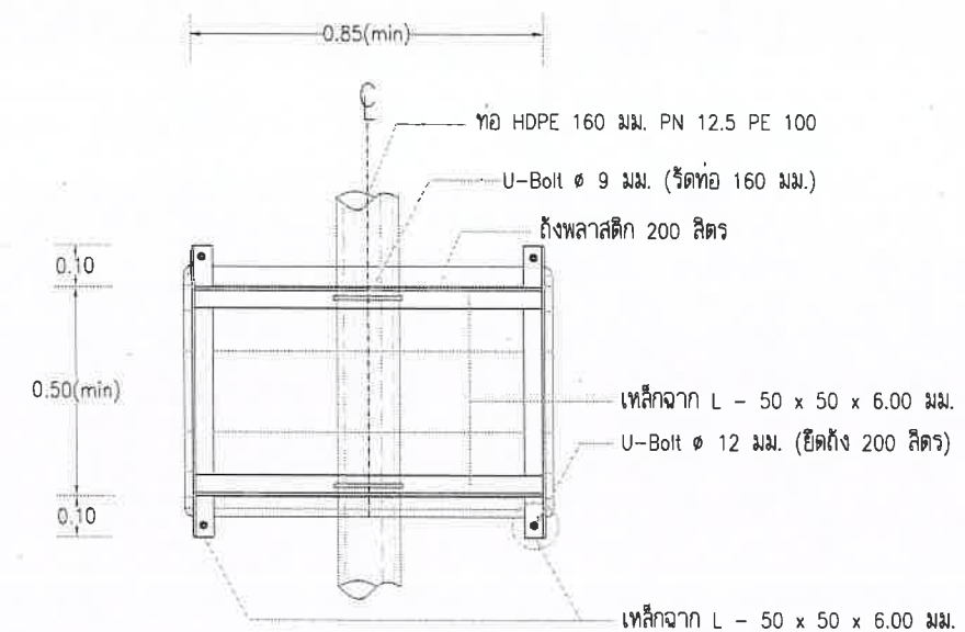
แปลนท่นลอย SCALE 1:20
