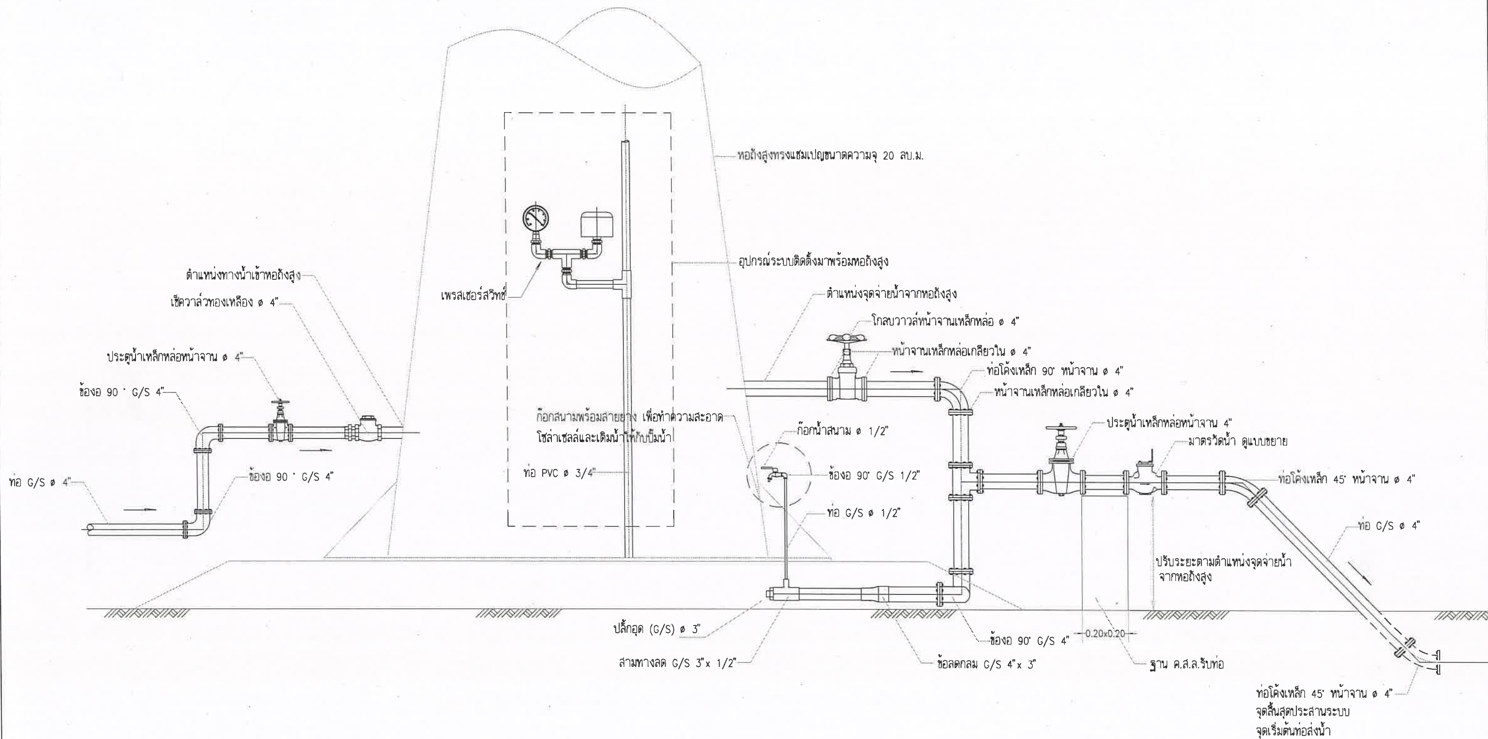
รูปแสดงรายละเอียดท่อและอุปกรณ์ระบบส่งน้ำ ไม่แสดงมาตราส่วน
