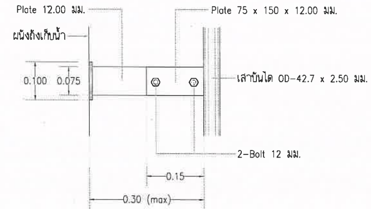
ขยายจุดยึดบันได SCALE 1:10
