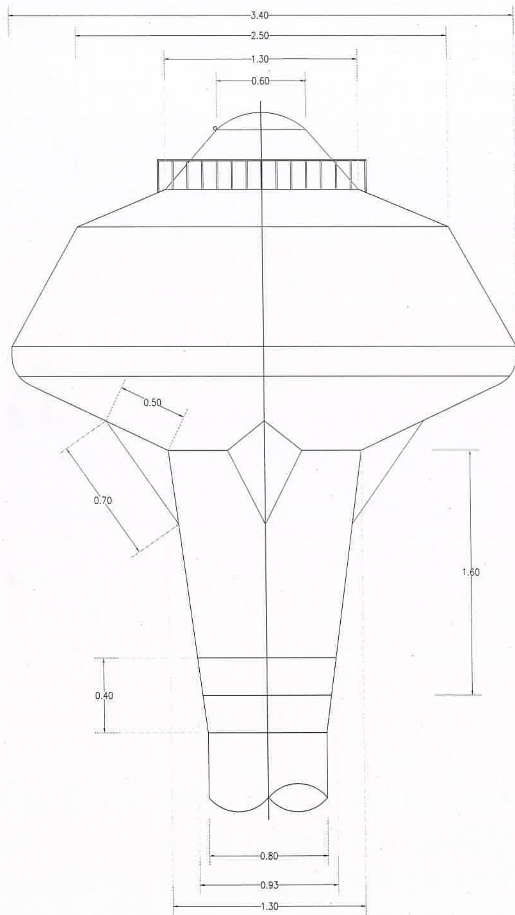
แบบขยายแมนโฮลบนท่อถึงสูง ไม่แสดงมาตราส่วน
