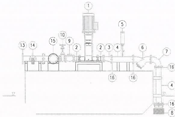
รูปตัดแสดงการประสานอุปกรณ์ภายในโรงสูบน้ำ SCALE 1:50
