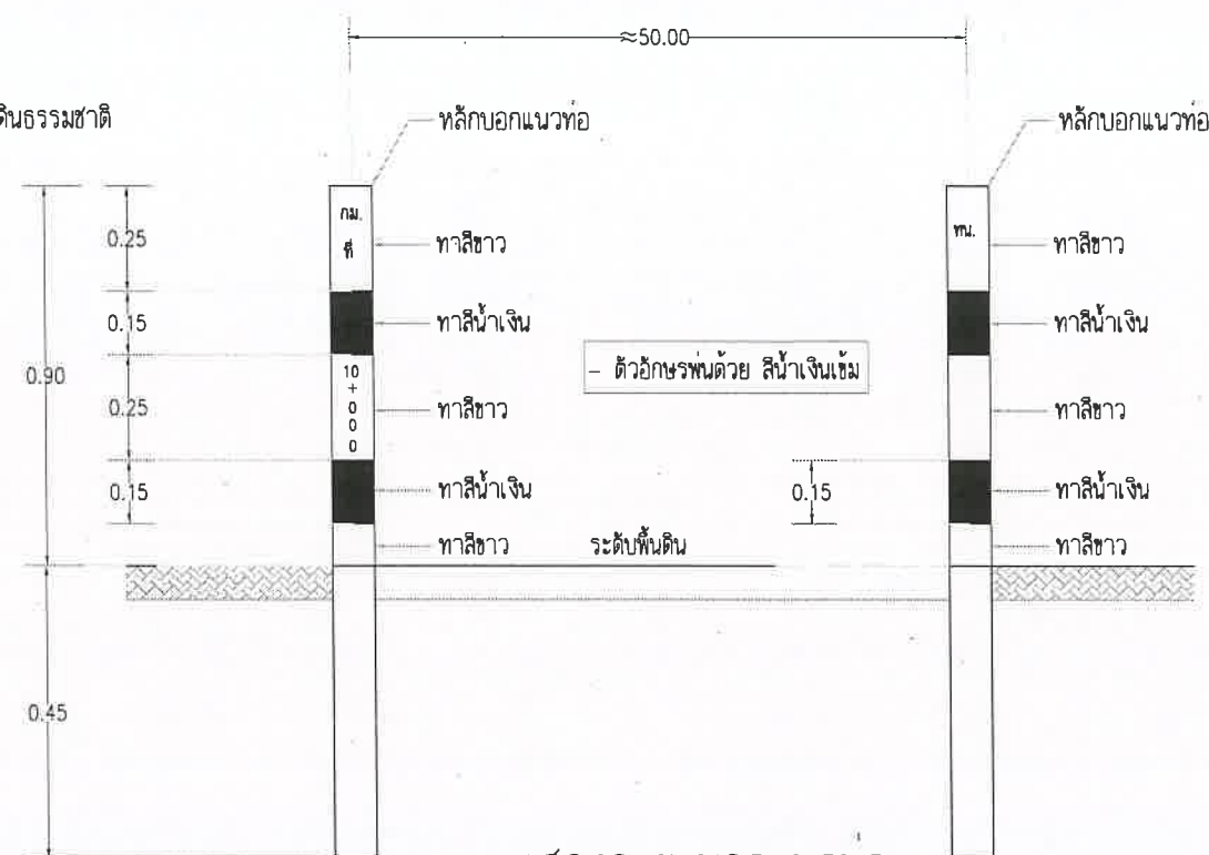
แสดงระยะบ่อแกว่งท่อ
