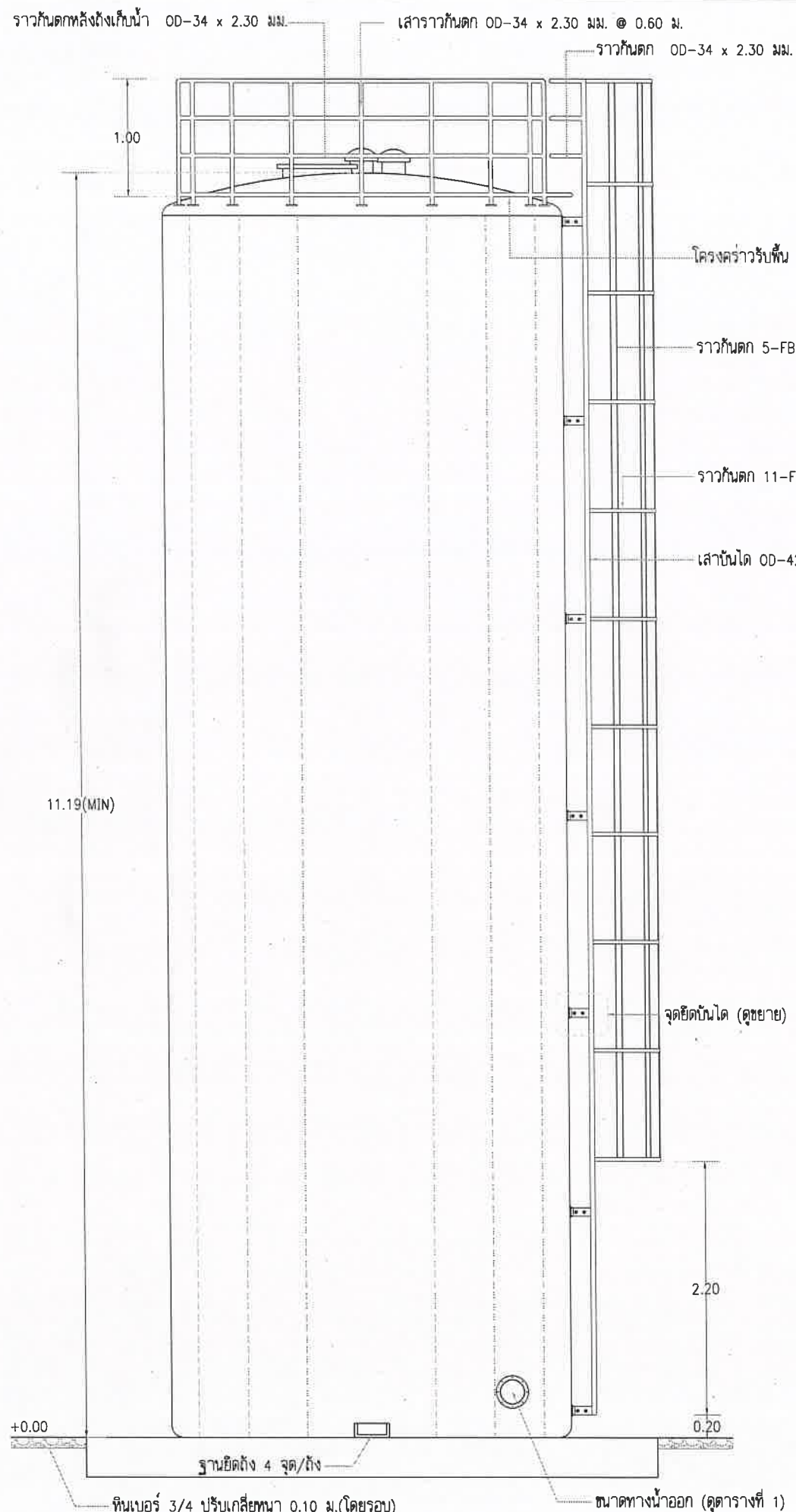
รูปด้านถังเก็บน้ำ SCALE 1:50
