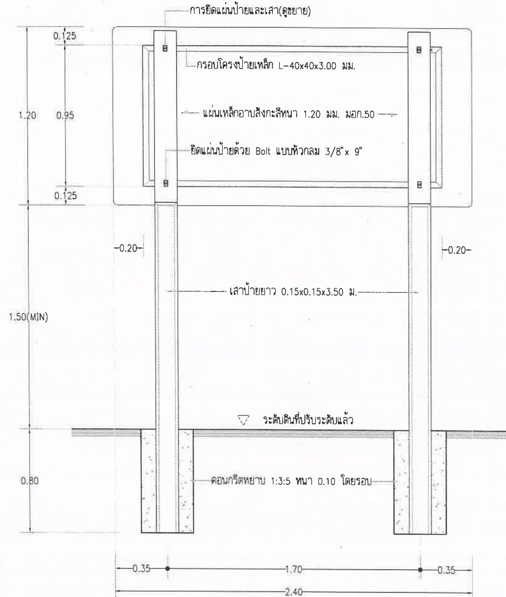
แสดงรูปด้านหลังป้ายโครงการ
