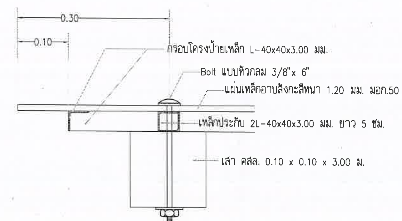
ขยายการขีดแผนป้ายและเสา SCALE 1:7.5
