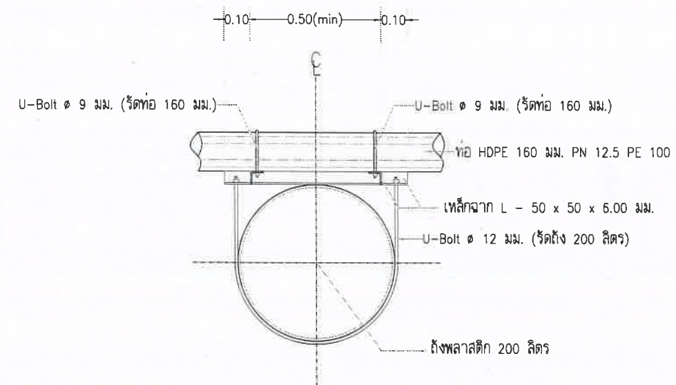
รูปตัดตามขวางท่นลอย SCALE 1:20
