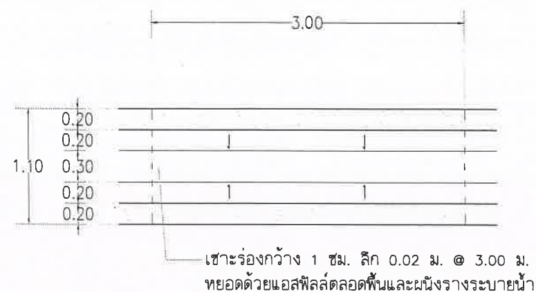
แปลนรางระบายน้ำ มาตราส่วน 1:50
