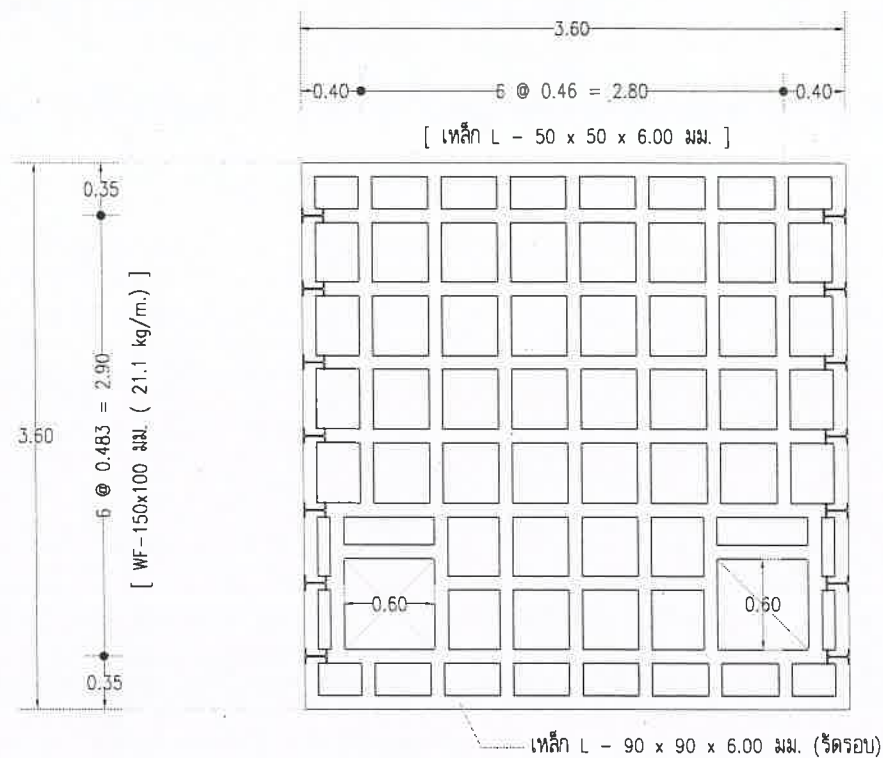
แปลนโครงสร้างพื้นบน อาคารโรงสูบน้ำขนาด 3.60 x 3.60 ม. SCALE 1:50
