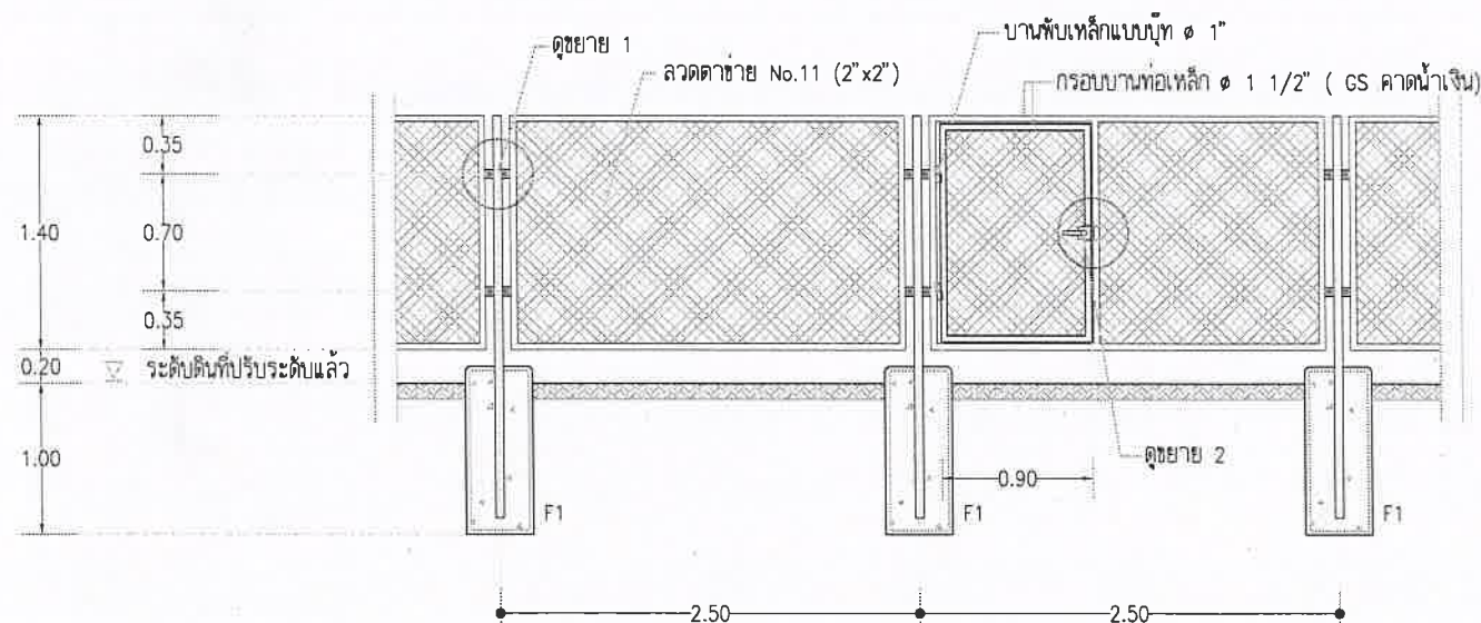
รูปด้านรั้วโปร่ง-ประตู SCALE 1:50
