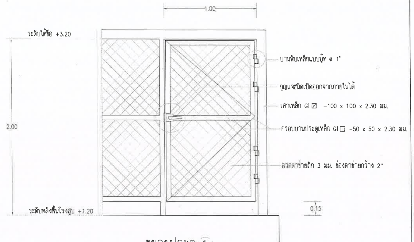
ขยายประตู 1 SCALE 1:25
