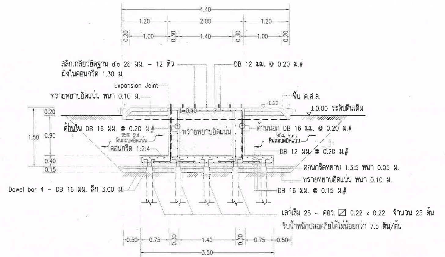
รูปตัดฐานรากหอดึงสูง (แบบเสาเข็ม) Not To Scale
