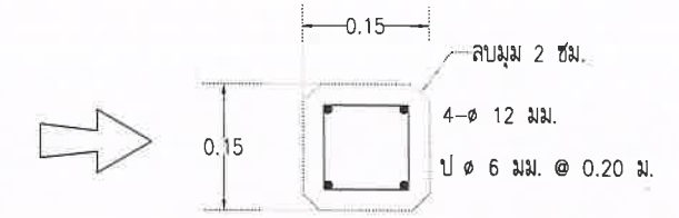
ขยายเสาป้ายฐานเสา - ใต้แผ่นป้าย
