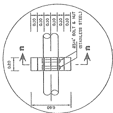
รูปตัด ก-ก
