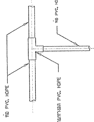
แบบการต่อสายทางลด PVC, HDPE ไม่แสดงมาตรฐาน
