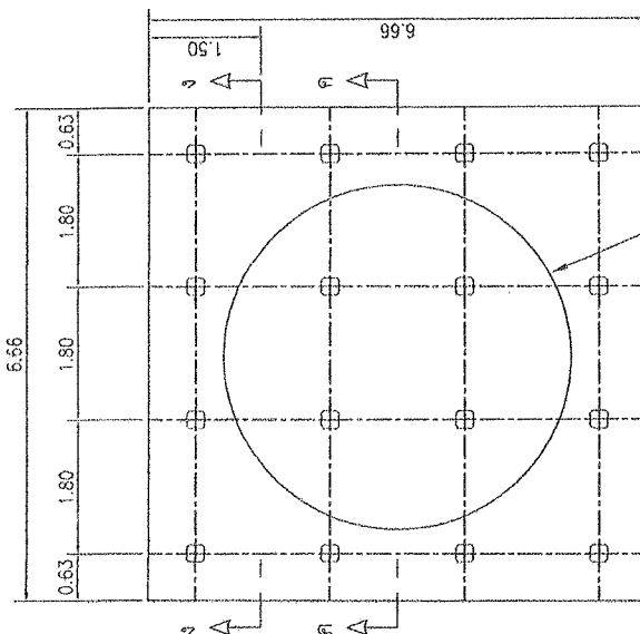
แปลนฐานรากแบบฐานแผ่ NOT TO SCALE
