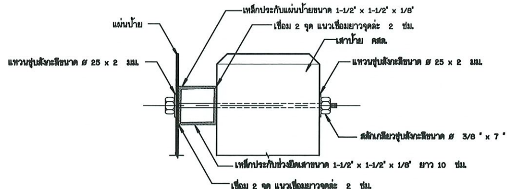
รูปตัดขยายการยึดแผ่นป้ายและเสา ไม่แสดงมาตราส่วน
