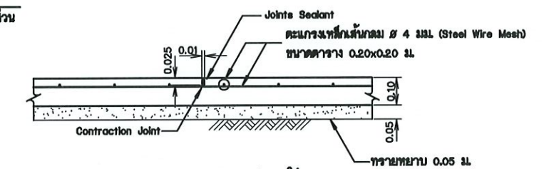
แบบขยายรอยต่อพื้น (Contraction Joint) ไม่แสดงขนาดตัว
