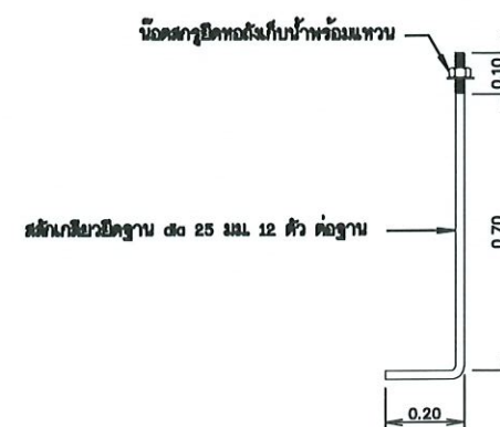
แบบขยายสลักเกลียวยึดฐาน
