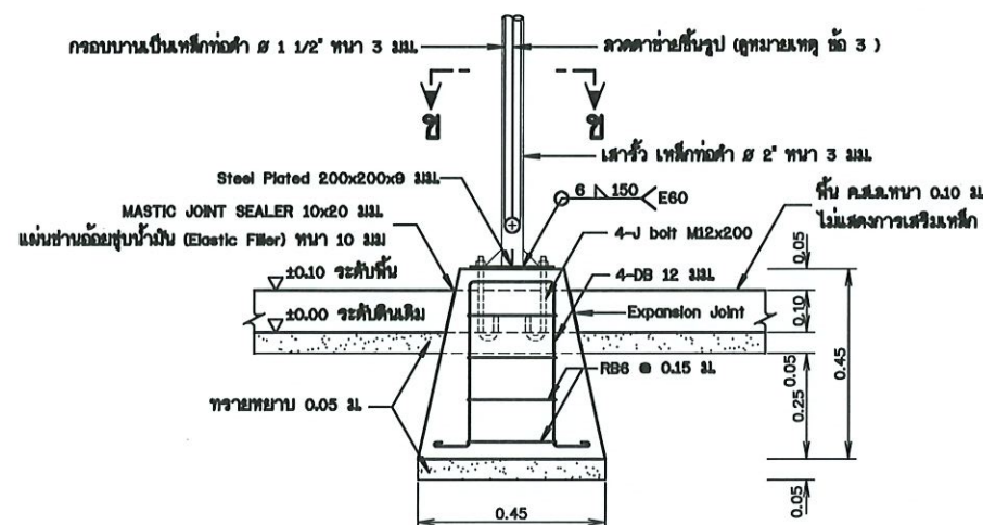
รูปขยายฐานรากโครงสร้างรับแผง F1 โดย อดิศักดิ์ อดิศักดิ์ ไม่แสดงมาตราส่วน
