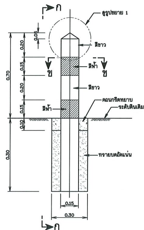
เสา ค.ส.ล. แสดแนวท่อส่งน้ำ
