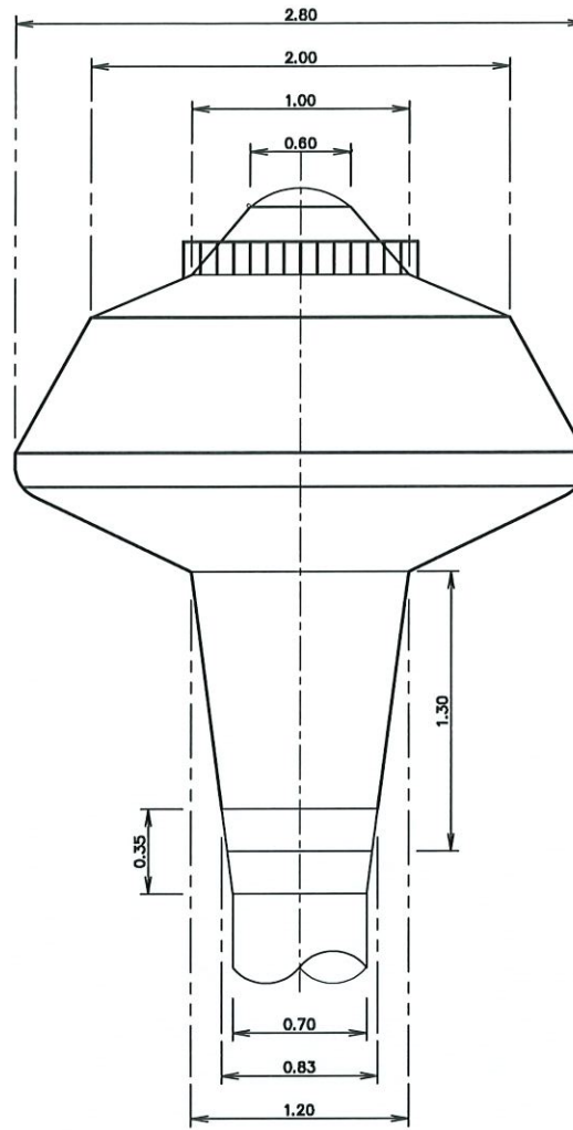
แบบขยายแมนโฮลบนท่อถึงสูง
