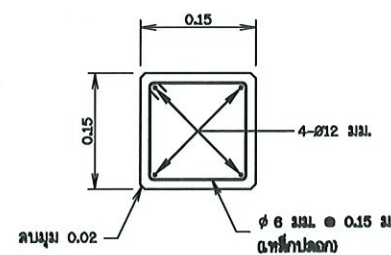
รูปตัด ข-ข
