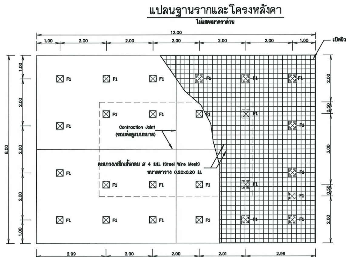
รูปขยายพื้นคอนกรีต ไม่แสดงมาตราส่วน
