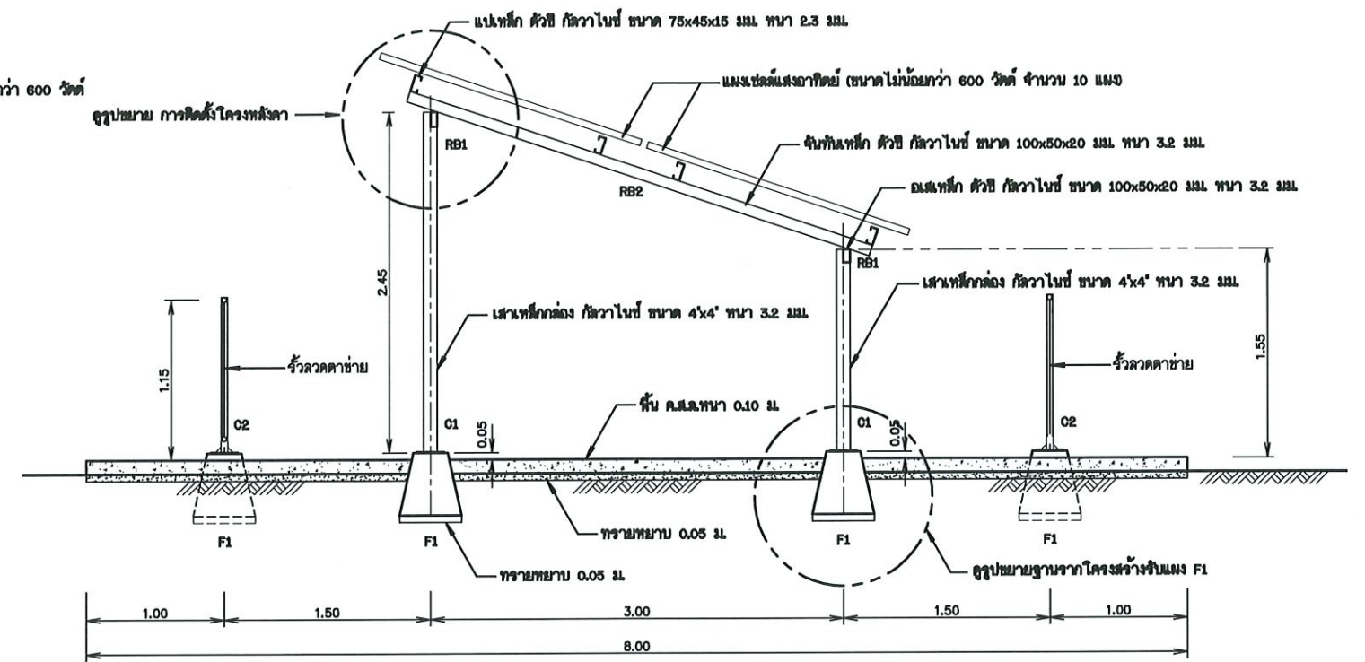
รูปด้านข้าง
