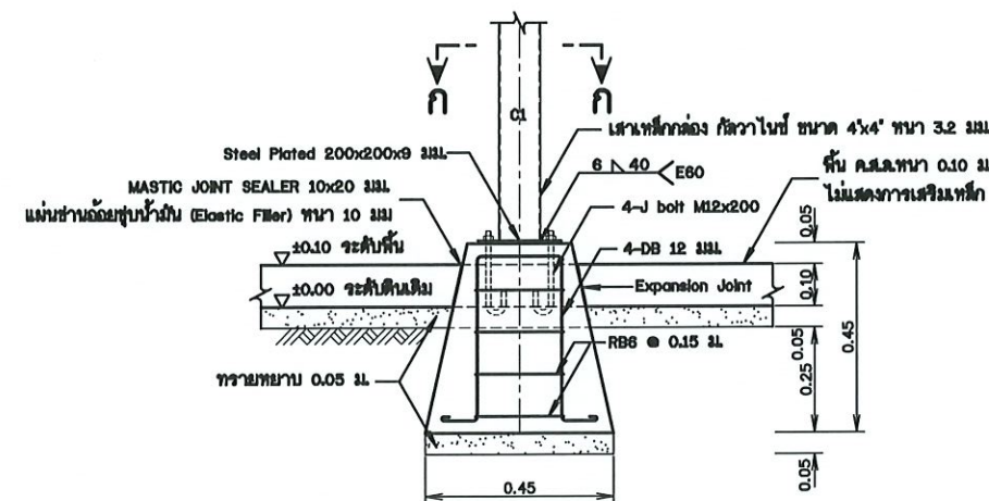
รูปขยายฐานรากโครงสร้างรับแผง F1 (ตอนจบ คสล. ท่อส่งน้ำรูปทรงแปดเหลี่ยม) ไม่แสดงขนาดส่วน
