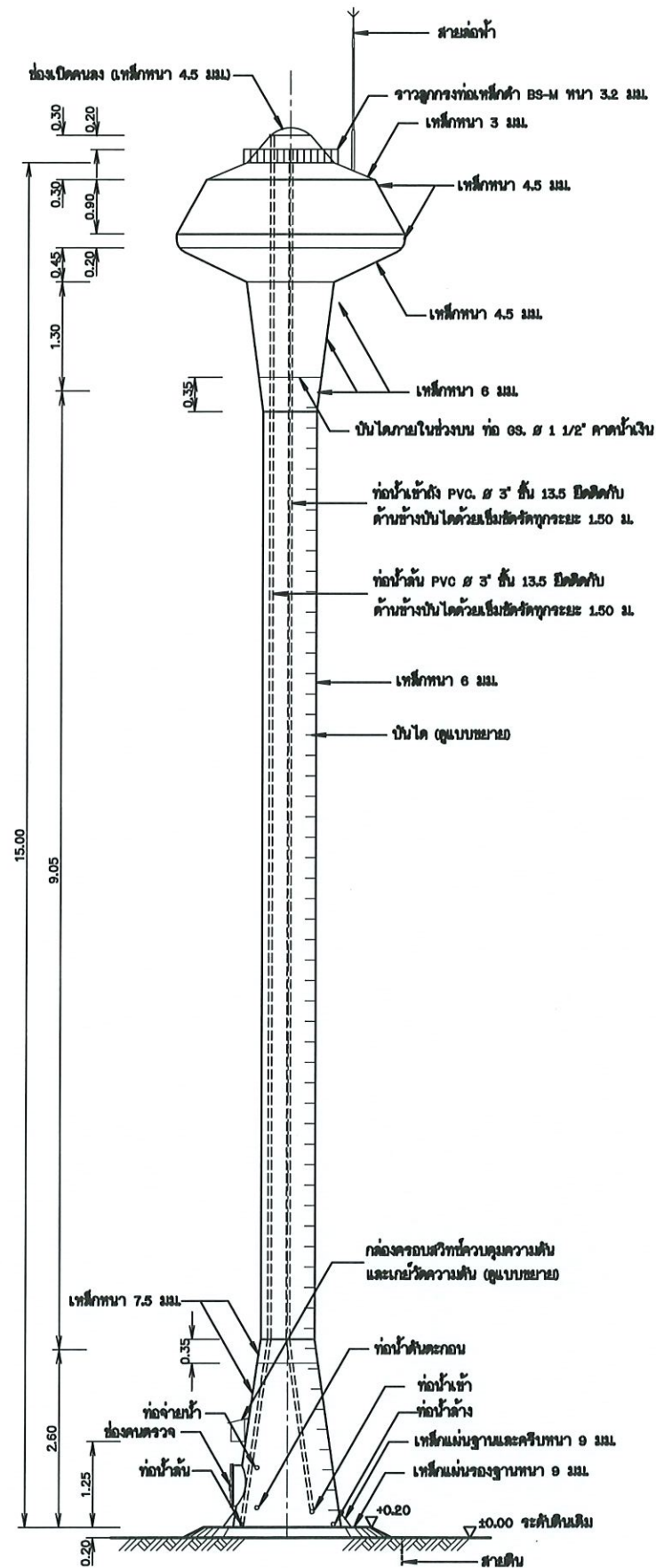
รูปด้านข้างท่อถึงสูง แบบถังเหล็กรูปทรงแปมแปญ
