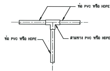
9. แบบการต่อสามทางลด PVC หรือ HDPE 10. แบบการต่อสามทาง PVC หรือ HDPE ไม่แสดงขนาดบางส่วน
