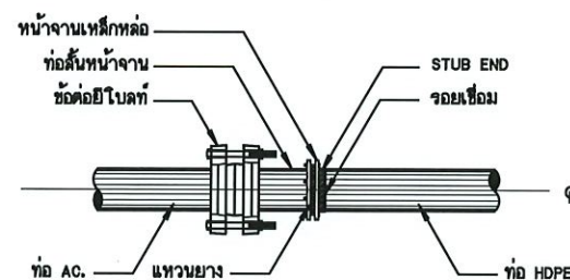
การบรรจุบล็อกลูก AC. กับท่อ HDPE
