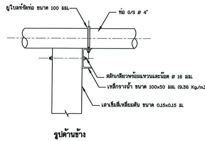
13. เสาตอม่อรองรับท่อชุด และแบบขยายอุปกรณ์รัดท่อ ไม่แสดงขนาดบางส่วน
