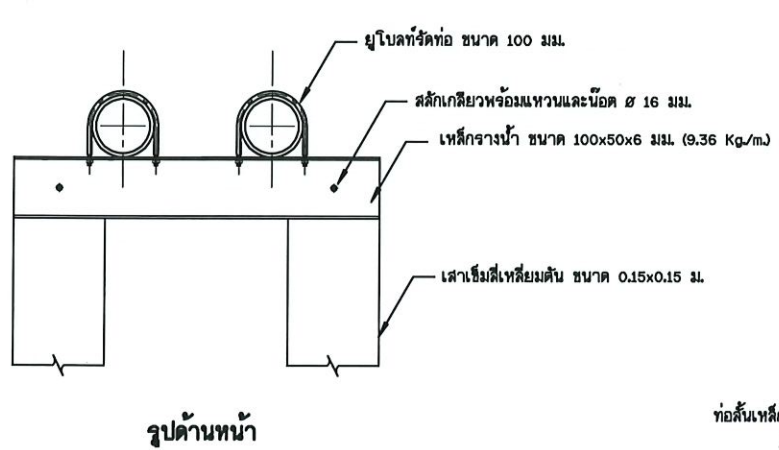
13. เสาตอม่อรองรับท่อชุด และแบบขยายอุปกรณ์รัดท่อ ไม่แสดงขนาดบางส่วน
