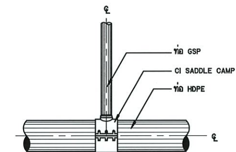
การบรรจุบล็อกลูกสามทาง HDPE กับท่อ GSP
