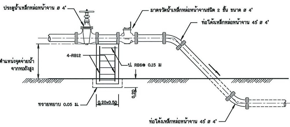
14. การติดตั้งมาตรวัดน้ำบนพื้นดิน 4" ไม่แสดงขนาดบางส่วน
