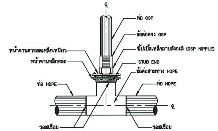
การบรรจุบล็อกลูกสามทาง HDPE กับท่อ GSP แบบข้อต่อ
