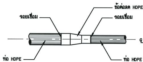
การบรรจุบล็อกลูก HDPE กับข้อต่อ HDPE
