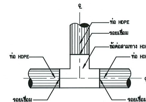
การบรรจุบล็อกลูกสามทาง HDPE กับท่อ HDPE
