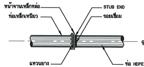
การบรรจุบล็อกลูกเหล็กเหนียวกับท่อ HDPE
