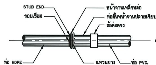
การบรรจุบล็อกลูก HDPE กับท่อ PVC.
