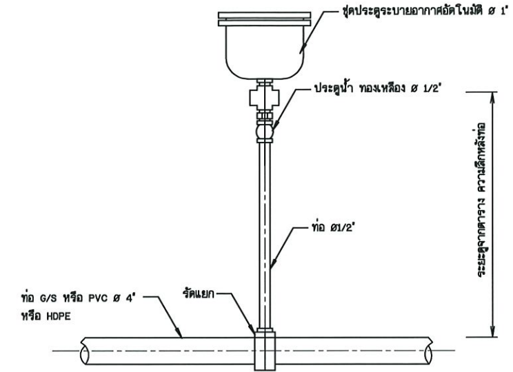
12. การติดตั้งประตูละบายอากาศอัตโนมัติ ไม่แสดงขนาดบางส่วน
