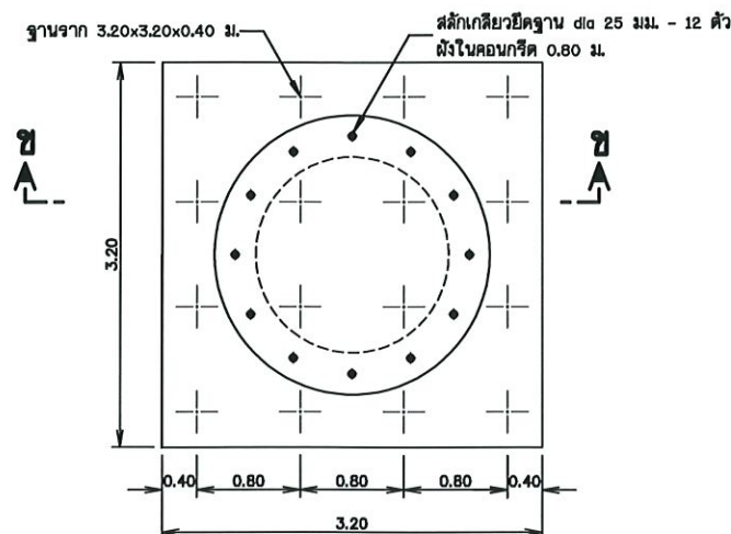
แปลน ฐานรากหอดึงสูง (แบบเสาเข็ม)
