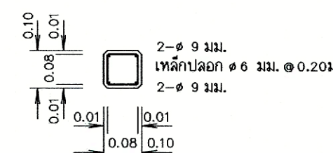
รูปตัด ข - ข
