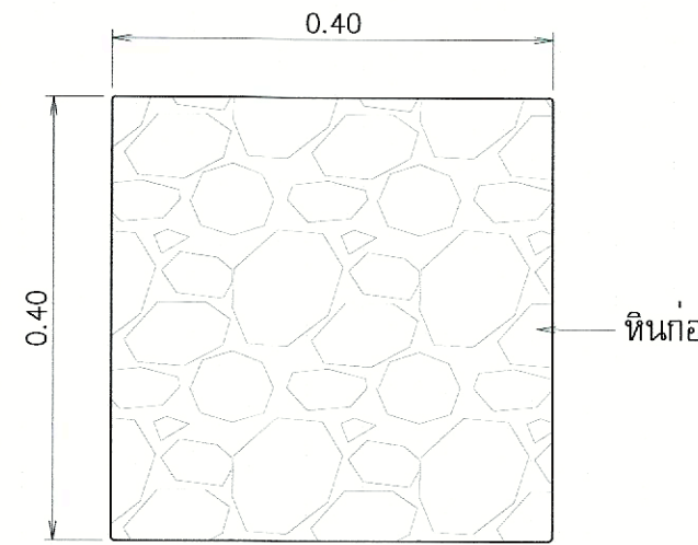
รูปขยายฝายหินก่อ ก1-ก1
