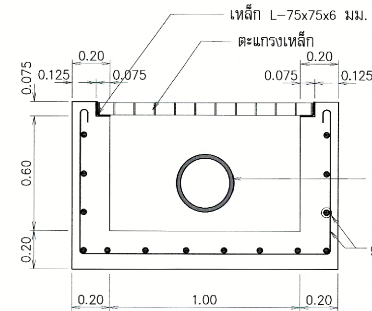
รูปตัดขวางรวมน้ำ ก2-ก2
