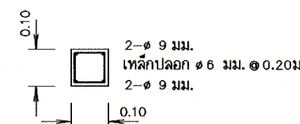
รูปตัด ก - ก
