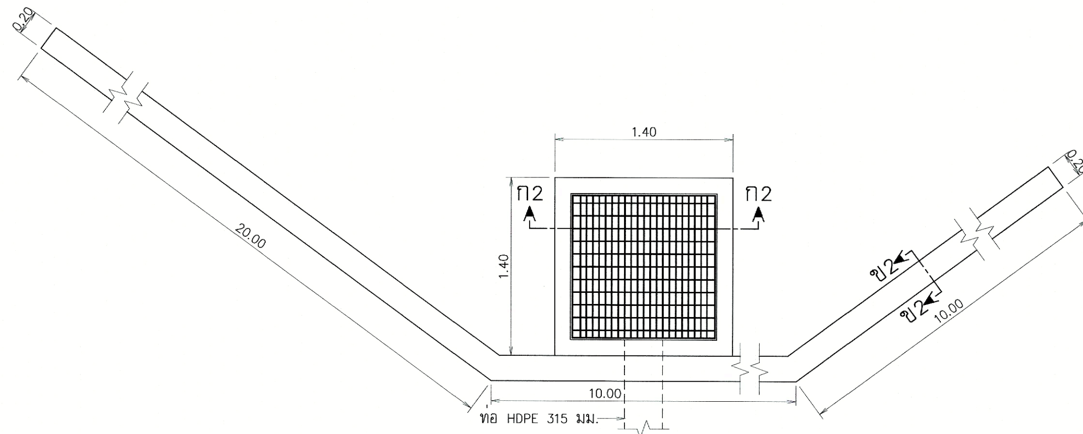
รูปขยายรางรวมน้ำ
