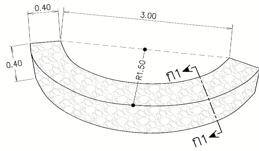
ฝายหินก่อ
