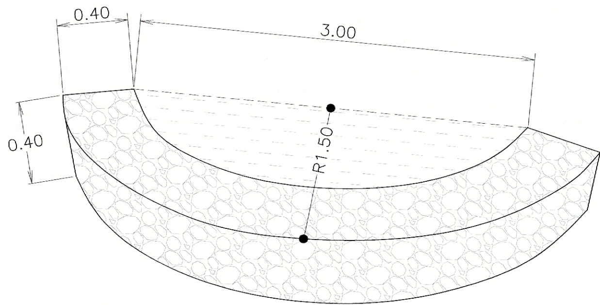
มิติฝายหินก่อ
