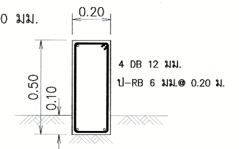
รูปขยายคาน ข2-ข2
