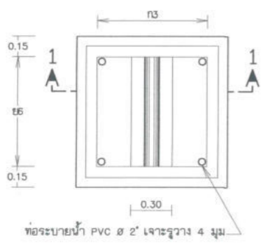
แปลนบ่อประตูบังคับน้ำ มาตราส่วน 1:20
