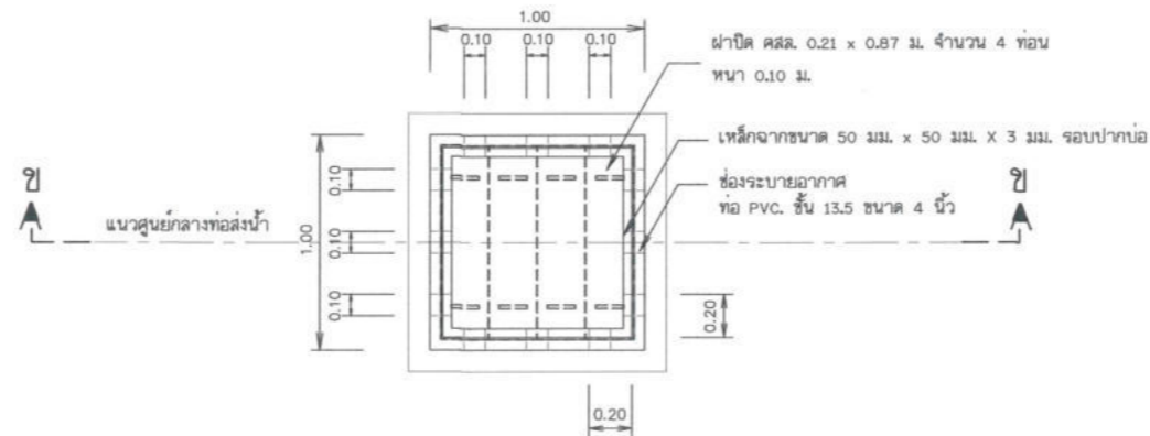
แปลนอาคารท่อระบายอากาศ
