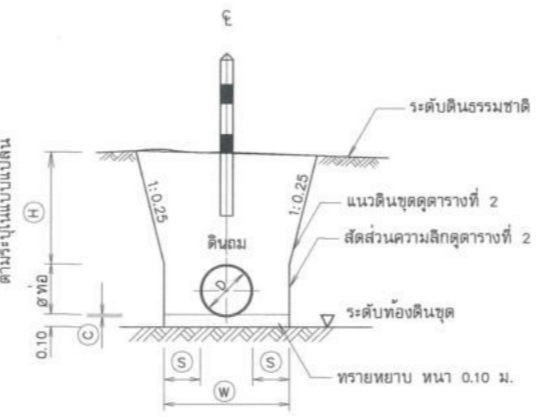
รูปตัดทั่วไปแสดงการวางท่อ มาตราส่วน 1:50
