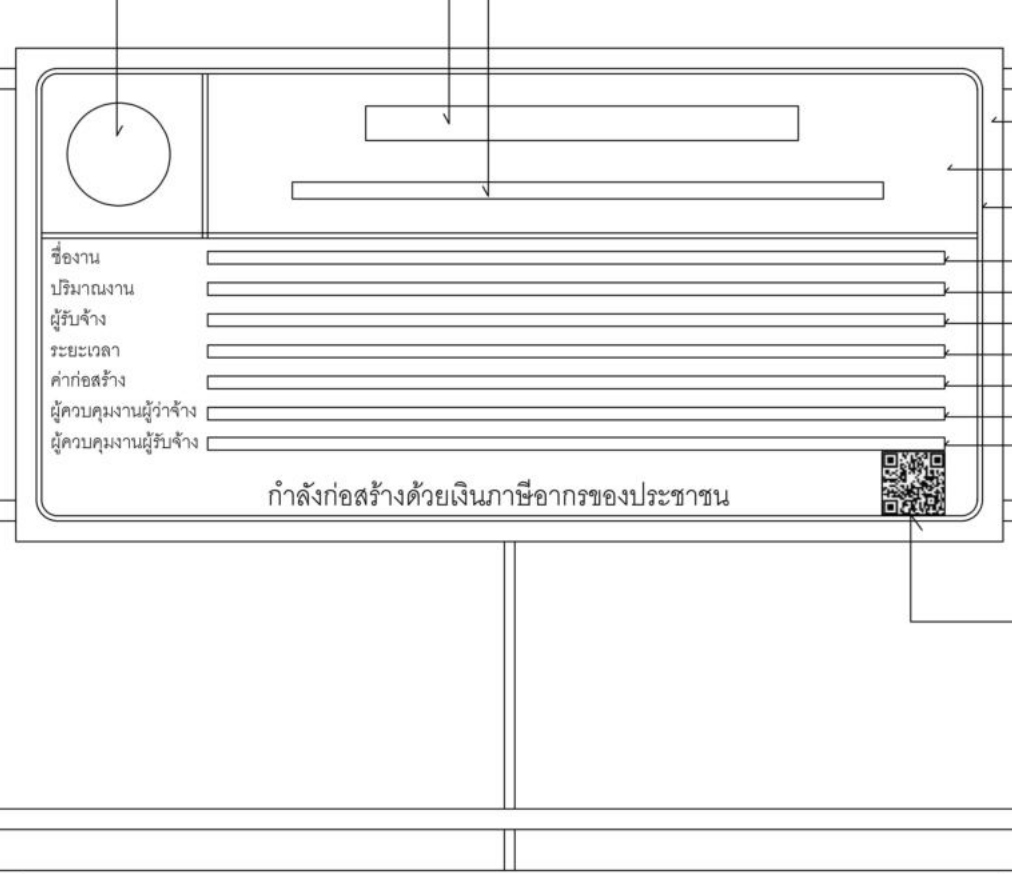
รูปด้านหน้า 1 : 50
