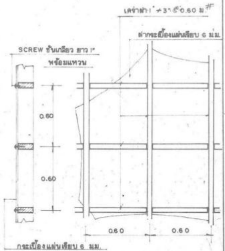
รูปขยายโครง, ฝา 1820
