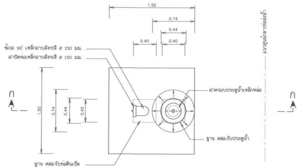
แบบแปลนอาคารประตูลอยตะกอน
