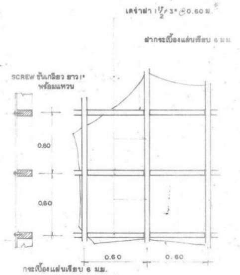
รูปขยายโครงฝ้า, ฝ้า 1820
