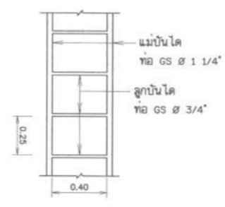
ขยายบ้นโด มาตราส่วน 1:20
