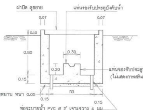
รูปตัด 1 - 1 มาตราส่วน 1:20
