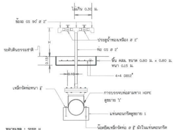
หมายเหตุ : ระยะ H H ไม่เกินกว่า 0.60 ม. สำหรับจุดปล่อยน้ำ
