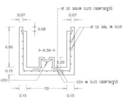
เหล็กเสริมบ่อประตูบังคับน้ำ มาตราส่วน 1:20
