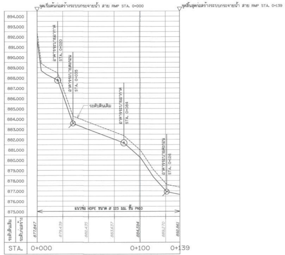
รูปตัดตามแนวยาว สาย RMP STA. 0+000 - 0+139
