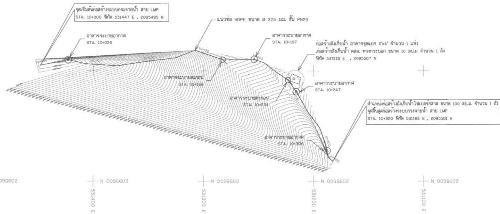
แปลนทั่วไป สาย LMP STA. 10+000 - 10+320 มาตรฐาน 1:1,000
