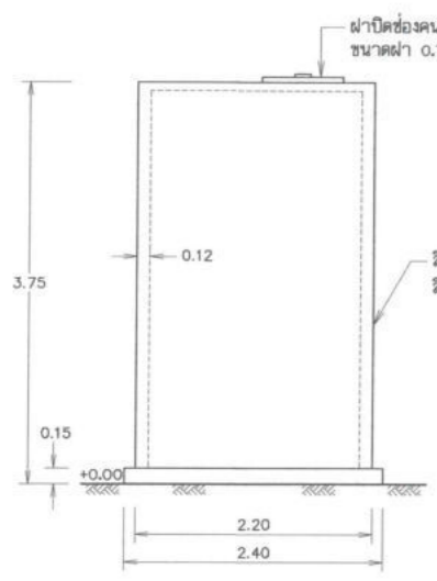
ด้านข้าง มาตราส่วน 1:40
