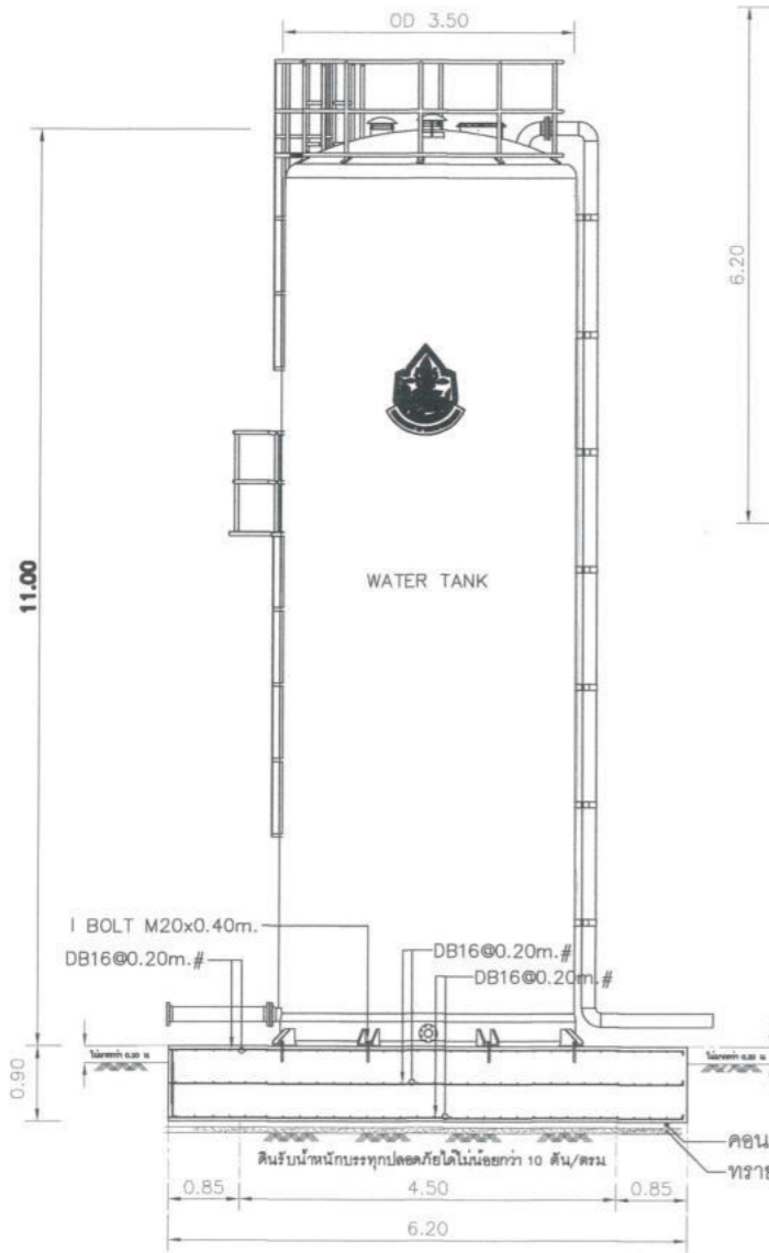
แบบขยายฐานรากแบบฐานแผ่ มาตราส่วน 1 : 100
