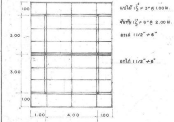
แปลนโครงหลังคา 18100
