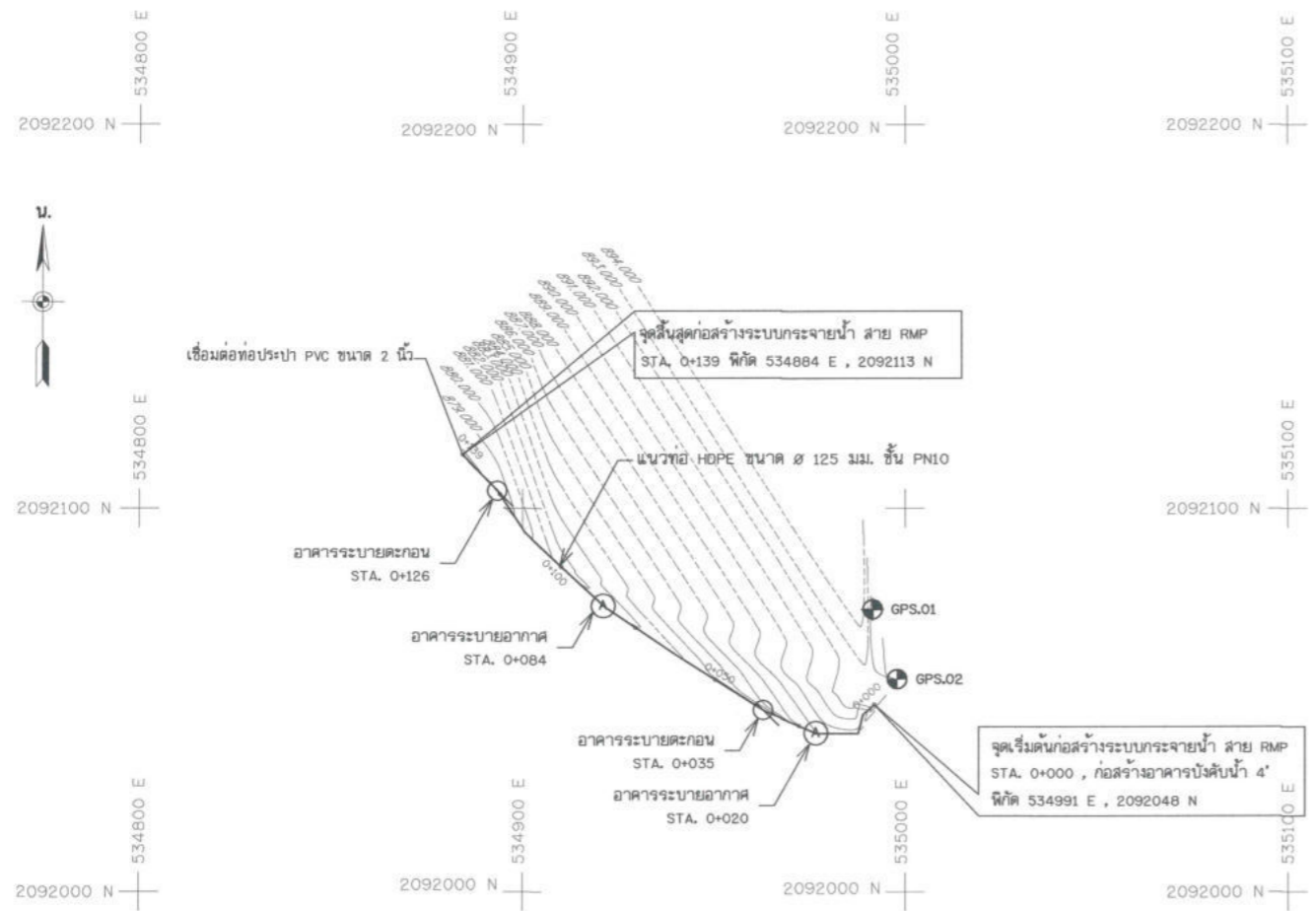
แปลนทั่วไป สาย RMP STA. 0+000 - 0+139 มาตราส่วน 1:1,000
