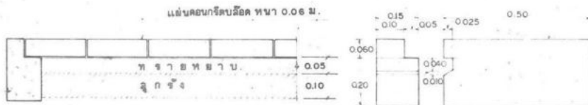
ขยายคันท่อน้ำ ๒10
