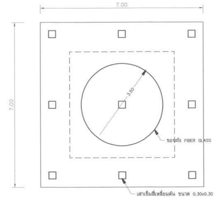
แปลนฐานแบบมีเข็ม มาตราส่วน 1 : 100
