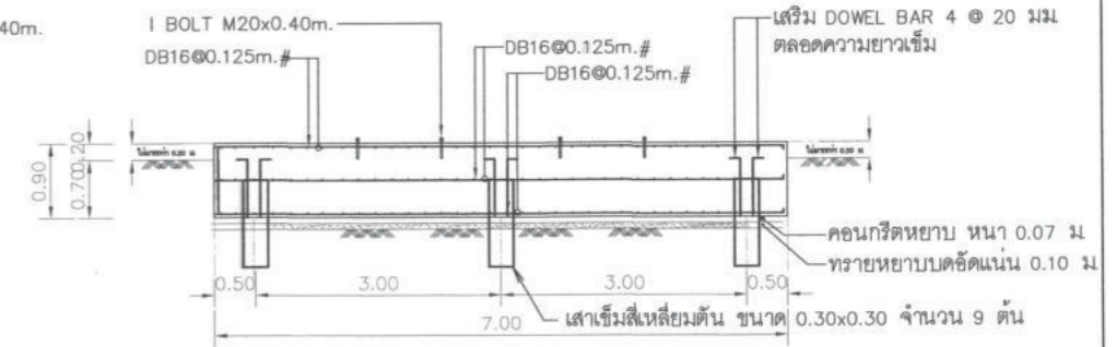
แบบขยายฐานรากแบบมีเข็ม มาตราส่วน 1 : 100
