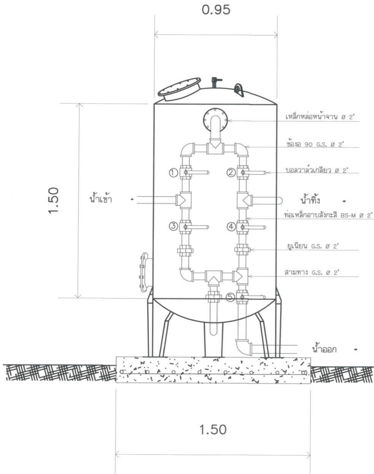
แบบแสดงอุปกรณ์ประกอบถังกรองน้ำภายนอก
