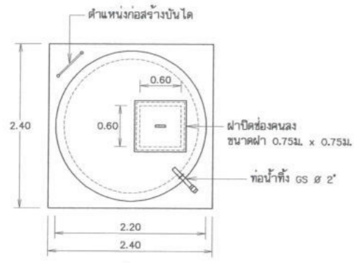
แปลน มาตราส่วน 1:40
