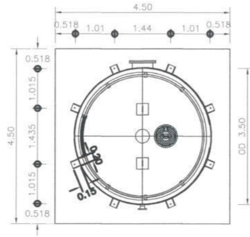
ตำแหน่งขายัดถัง มาตราส่วน 1 : 100
