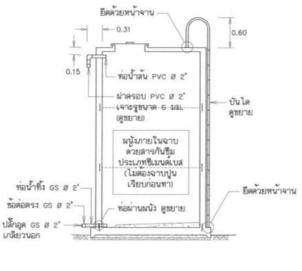
รูปตัด (2) มาตราส่วน 1:40
