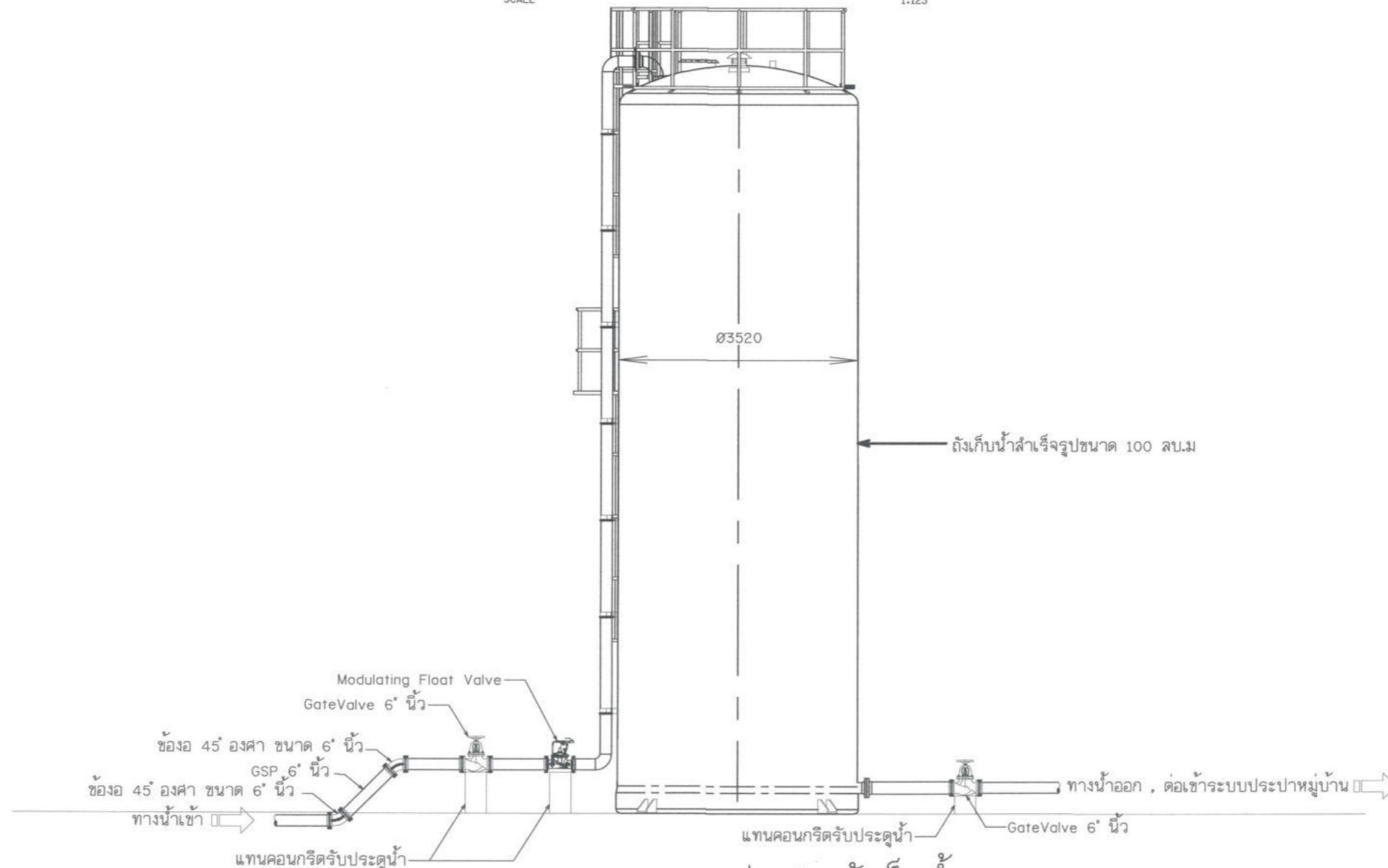
แบบขยายงานประสาณถังเก็บน้ำ SCALE 1:125
