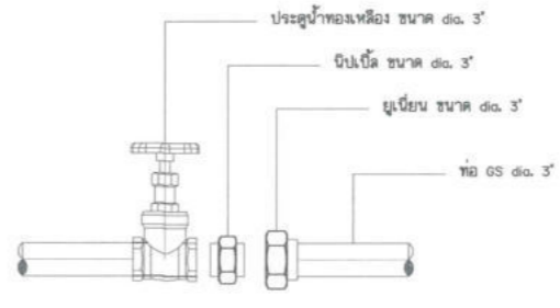
แบบขยายการประสานท่อระหว่างถัง มาตราส่วน 1:20
