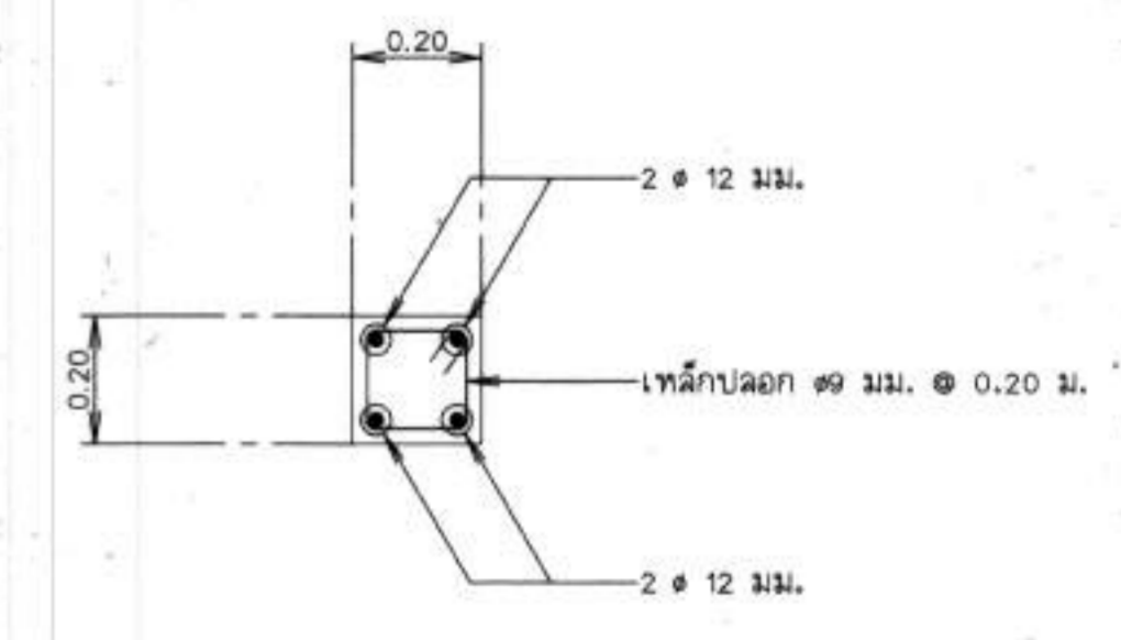
รูปตัด ค - ค มาตราส่วน 1:12.5
