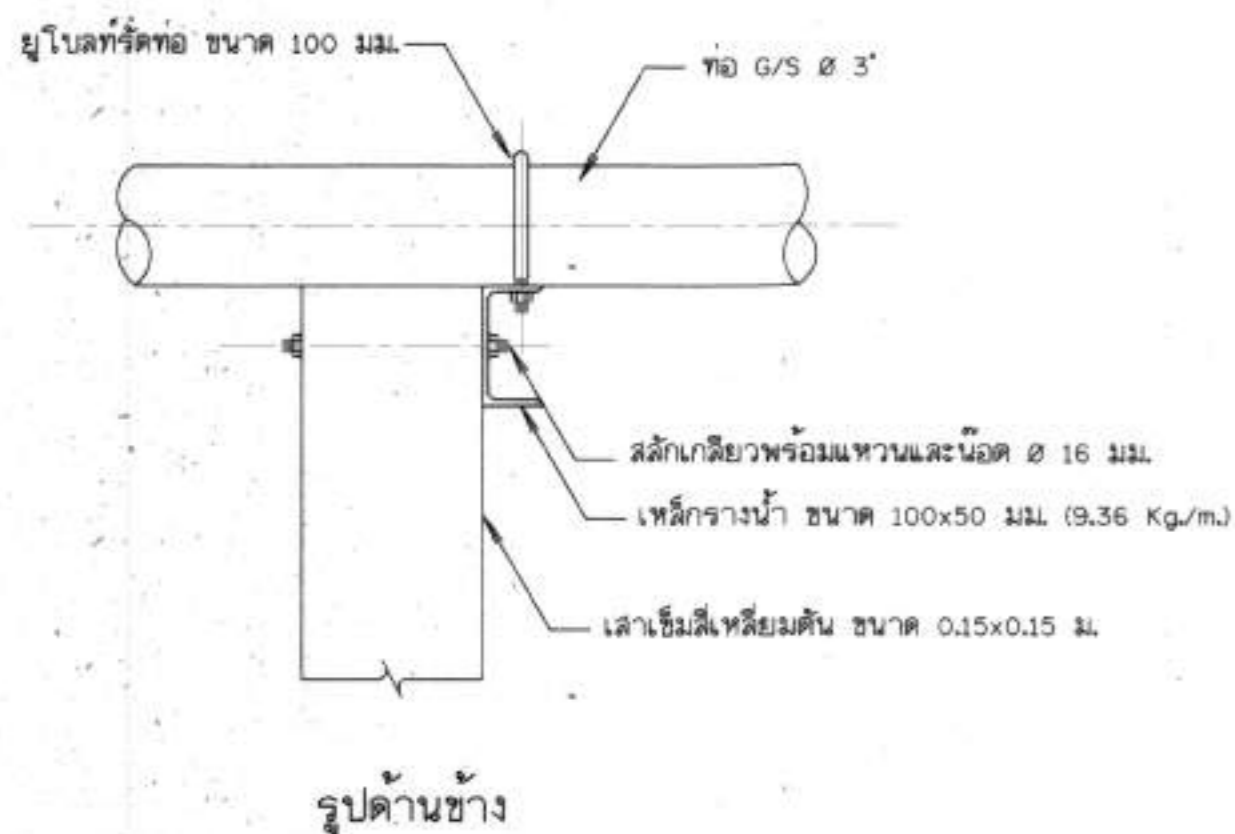
13. เสาคอมม่อรับท่อจุด และแบบขยายอุปกรณ์รัดท่อ ไม่แสดงขนาดบางส่วน
