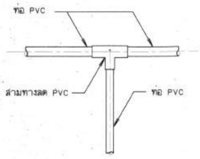
9. แบบการต่อสามทางลด PVC ไม่แสดงขนาดบางส่วน
