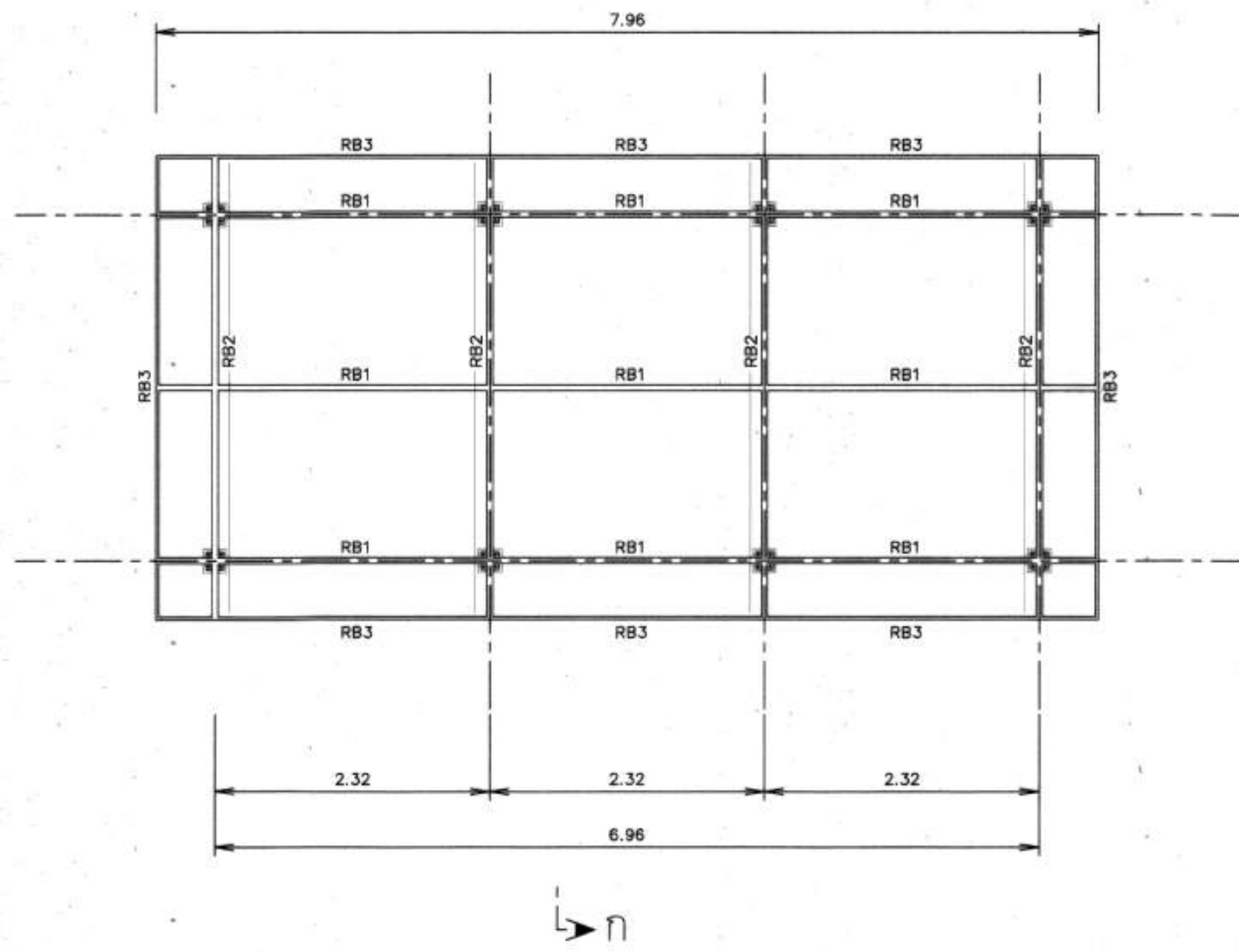
แปลนโครงเหล็กรับแผงเซลล์แสงอาทิตย์
