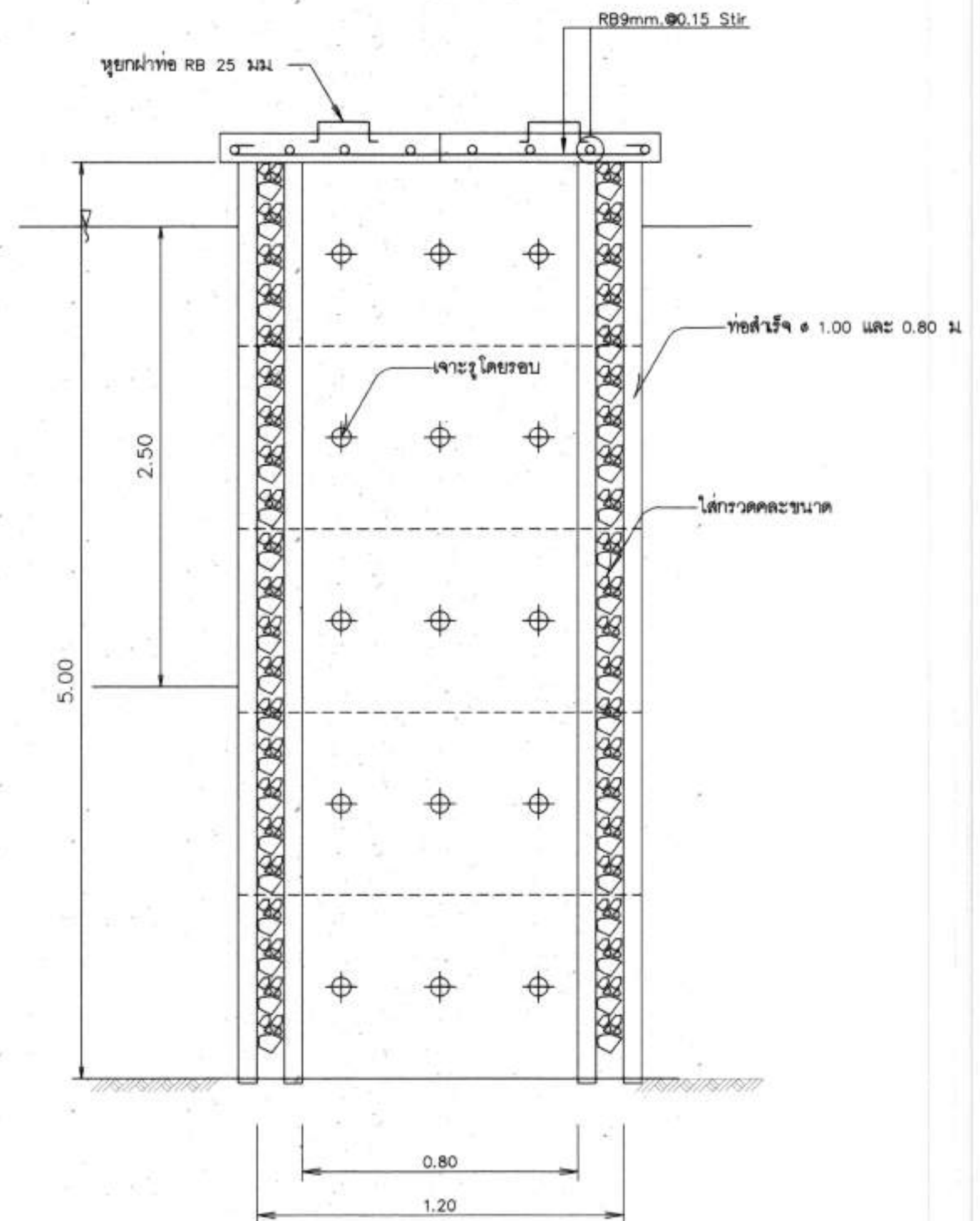
รูปตัดอาคารทรงน้ำดิบ มาตราส่วน 1:25
