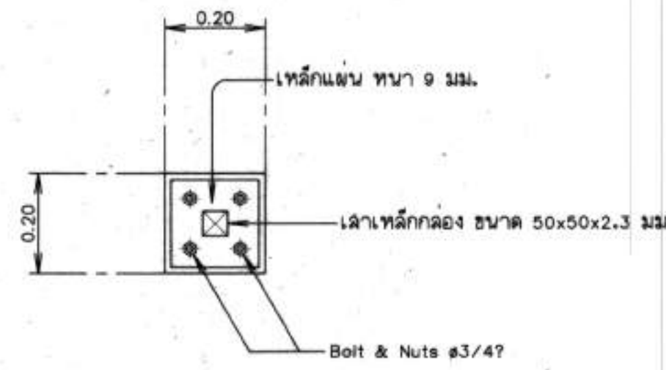
ขยายรอยต่อเสา คสล-เสาเหล็ก
