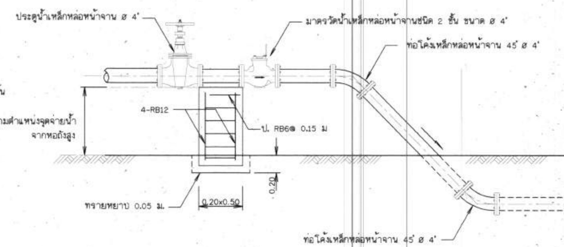
14. การติดตั้งมาตรวัดน้ำบนพื้นดิน 4\"/>
