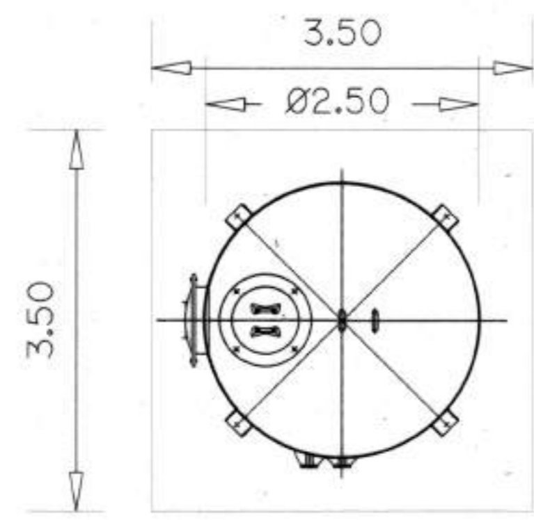
PLAN SCALE : 1:100
