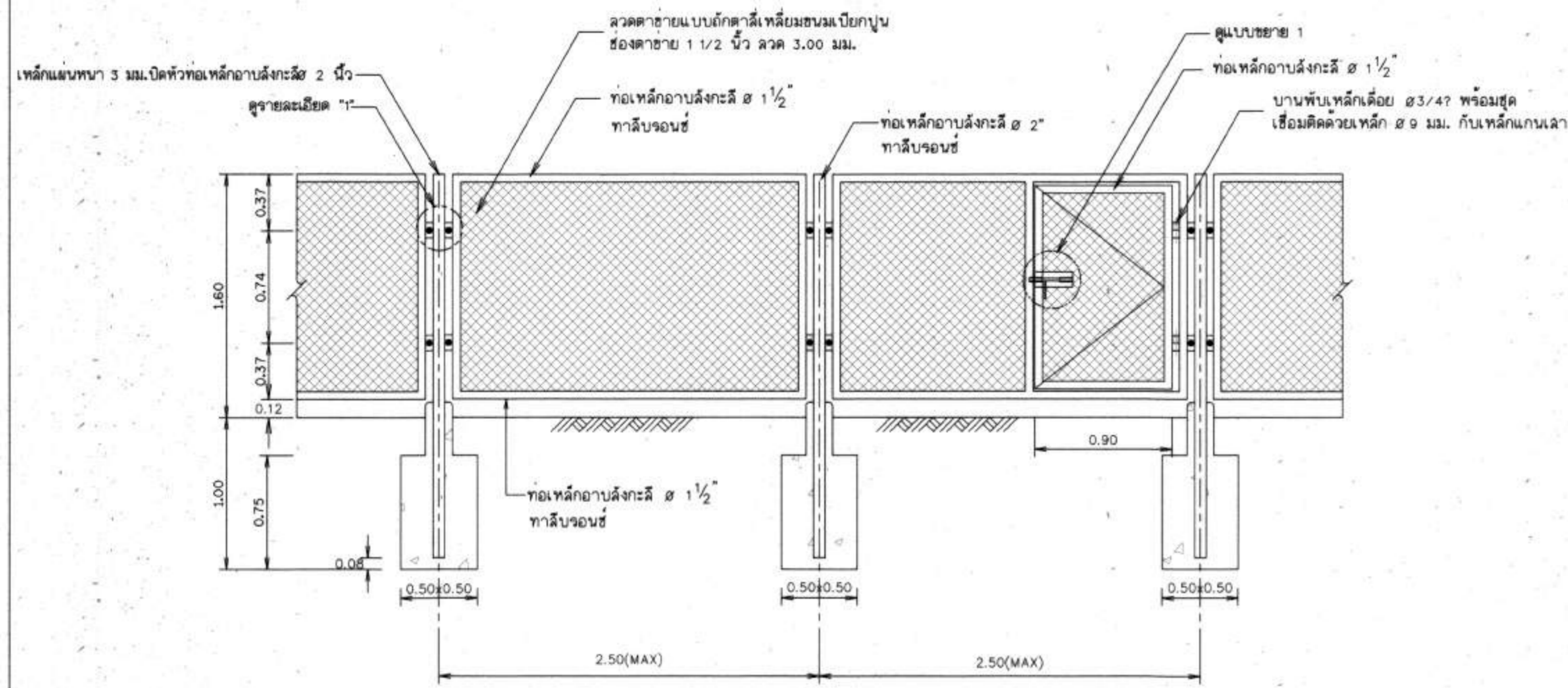
รูปแสดงแบบขยายรั้ว มาตราส่วน 1:25
