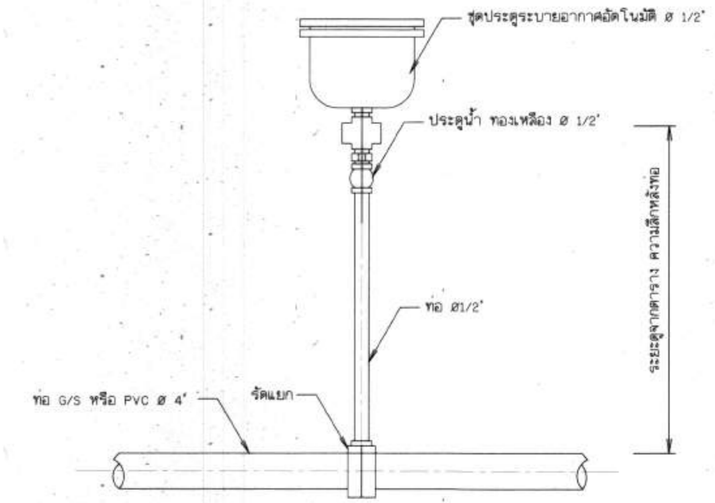
12. การติดตั้งประตูประบายอากาศอัตโนมัติ ไม่แสดงขนาดบางส่วน
