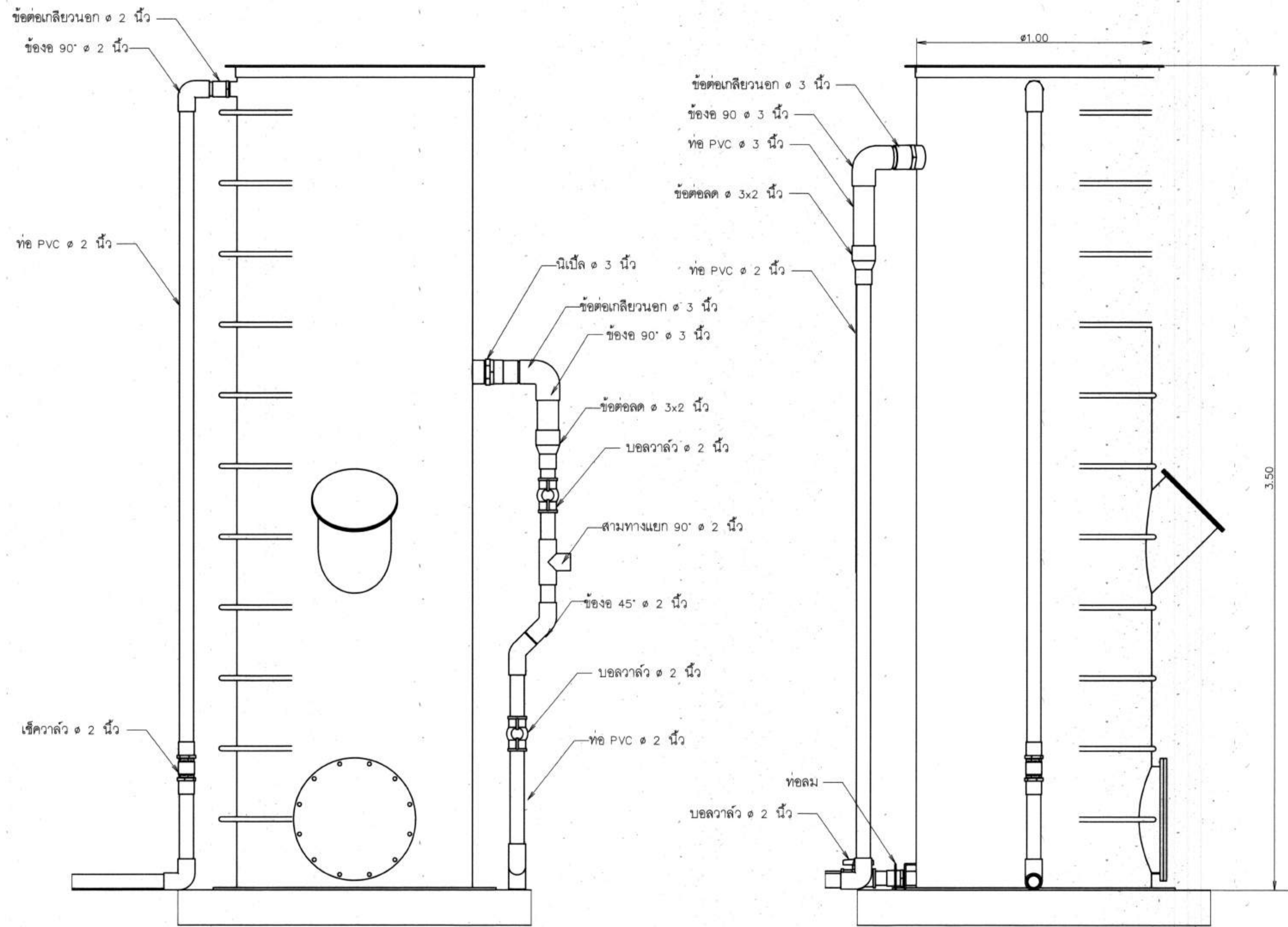
แบบขยายชุดวาล์วถึงกรองน้ำใส มาตราส่วน 1:10
