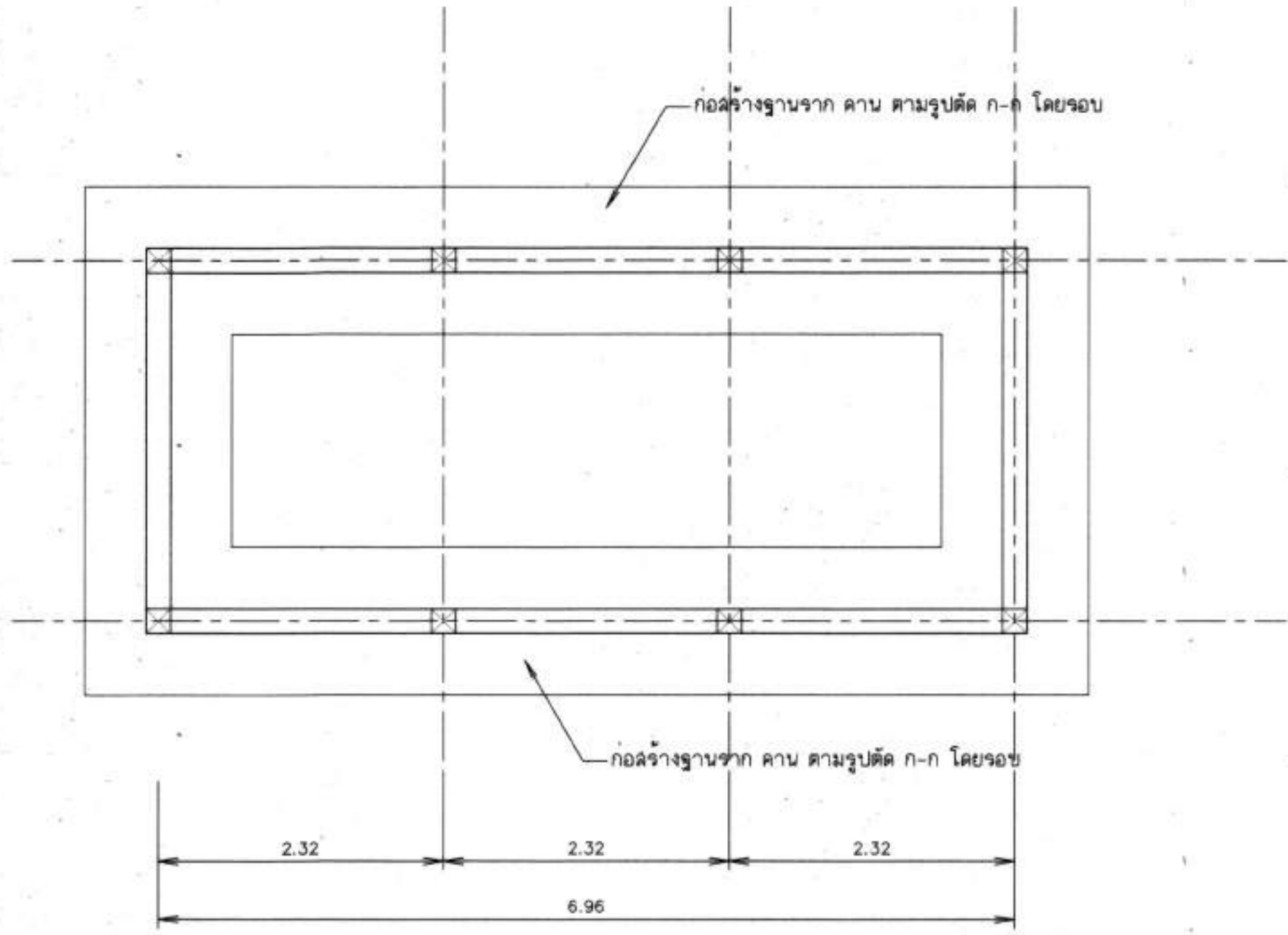
แปลนฐานรากอาคารโรงสูบน้ำ มาตราส่วน 1:40
