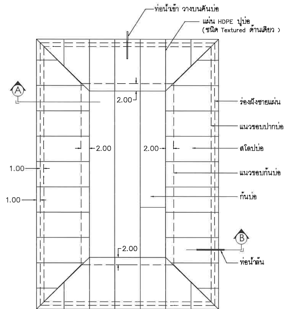
แปลนแนวปูแผ่น HDPE.
