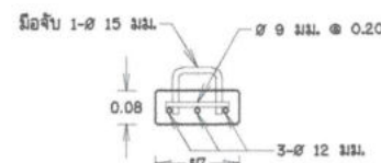
รูปตัดแนว 2 - 2
