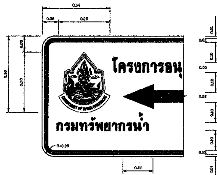
รูปขยายตราสัญลักษณ์ มาตรฐาน 1115
