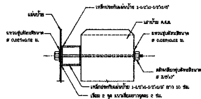
รูปตัดขยายการยึดแผ่นป้ายและเสา มาตรฐาน 1120
