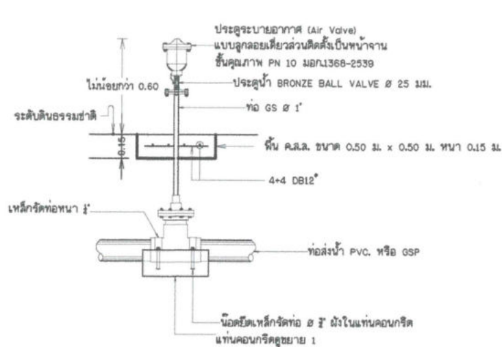
รูปตัดอาคารประตูปะบายอากาศ (Air Valve)
