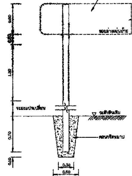
รายละเอียดการติดตั้งเสาป้าย มาตรฐาน 1120
