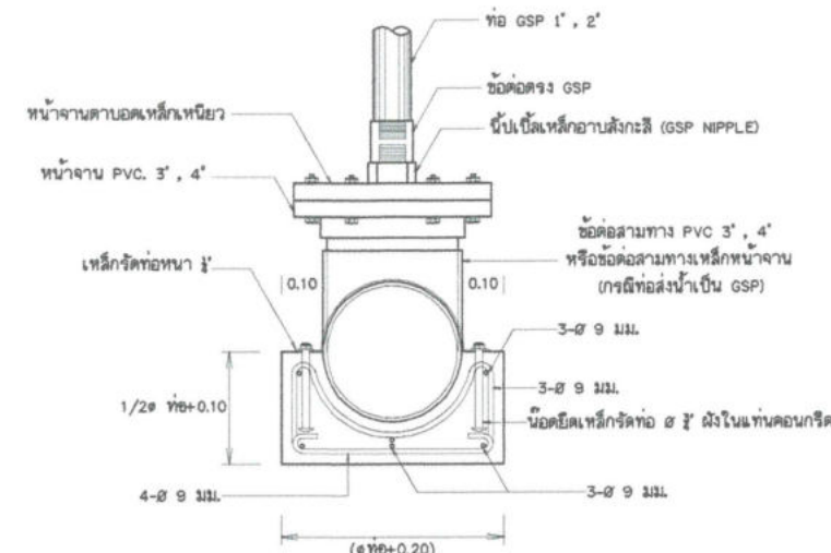
รูปตัดขยาย 1"
