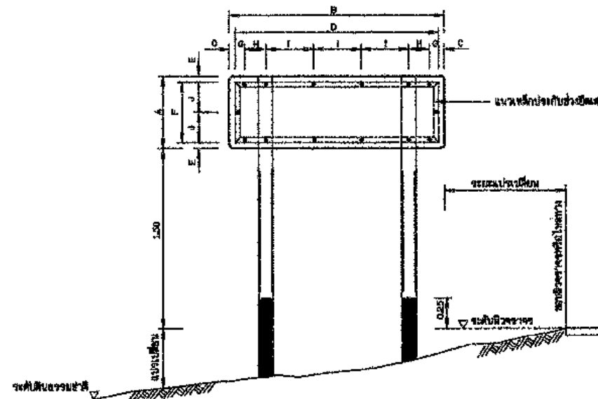
รูปแสดงการประกอบแผ่นป้าย มาตรฐาน 1120
