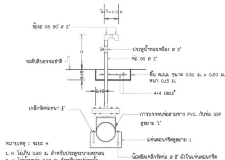
รูปตัดอาคารประตูปะบายตะกอนและอาคารจุดปล่อยน้ำ
