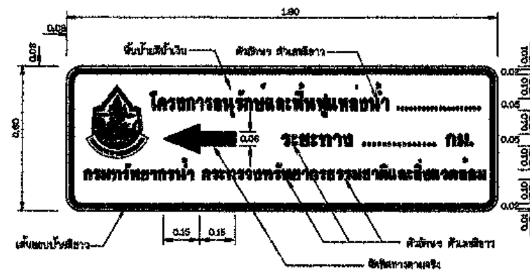
ป้ายแนะนำโครงการ มาตรฐาน 1110
