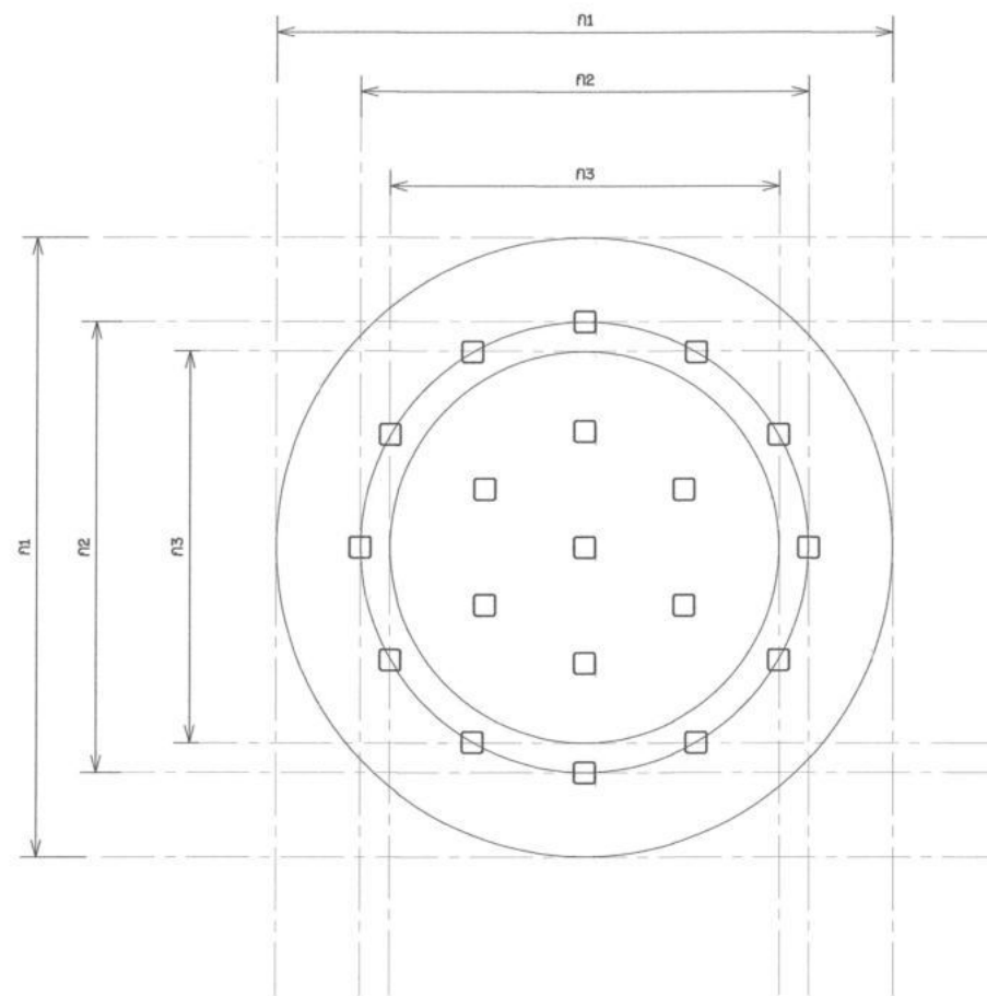
แปลนเสาเข็ม รับถังเหล็กเคลือบแก้วขนาด 300 ลบ.ม. มาตราส่วน 1:100
