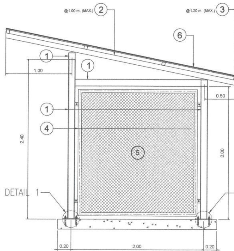
ELEVATION B
