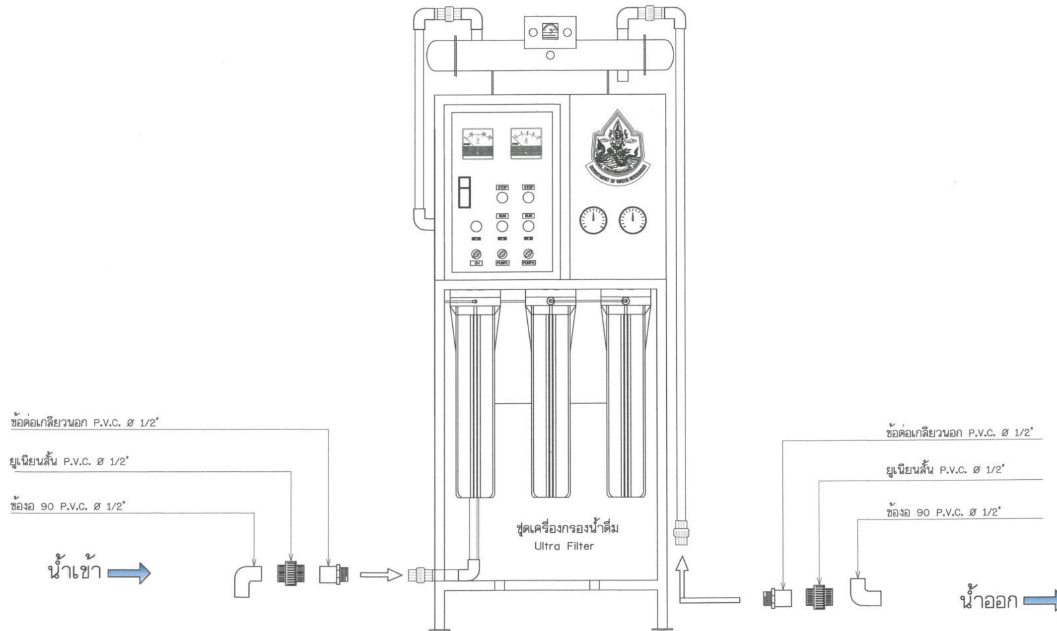
แบบขยายการติดตั้งอุปกรณ์ท่อเครื่องกรองน้ำดื่ม
