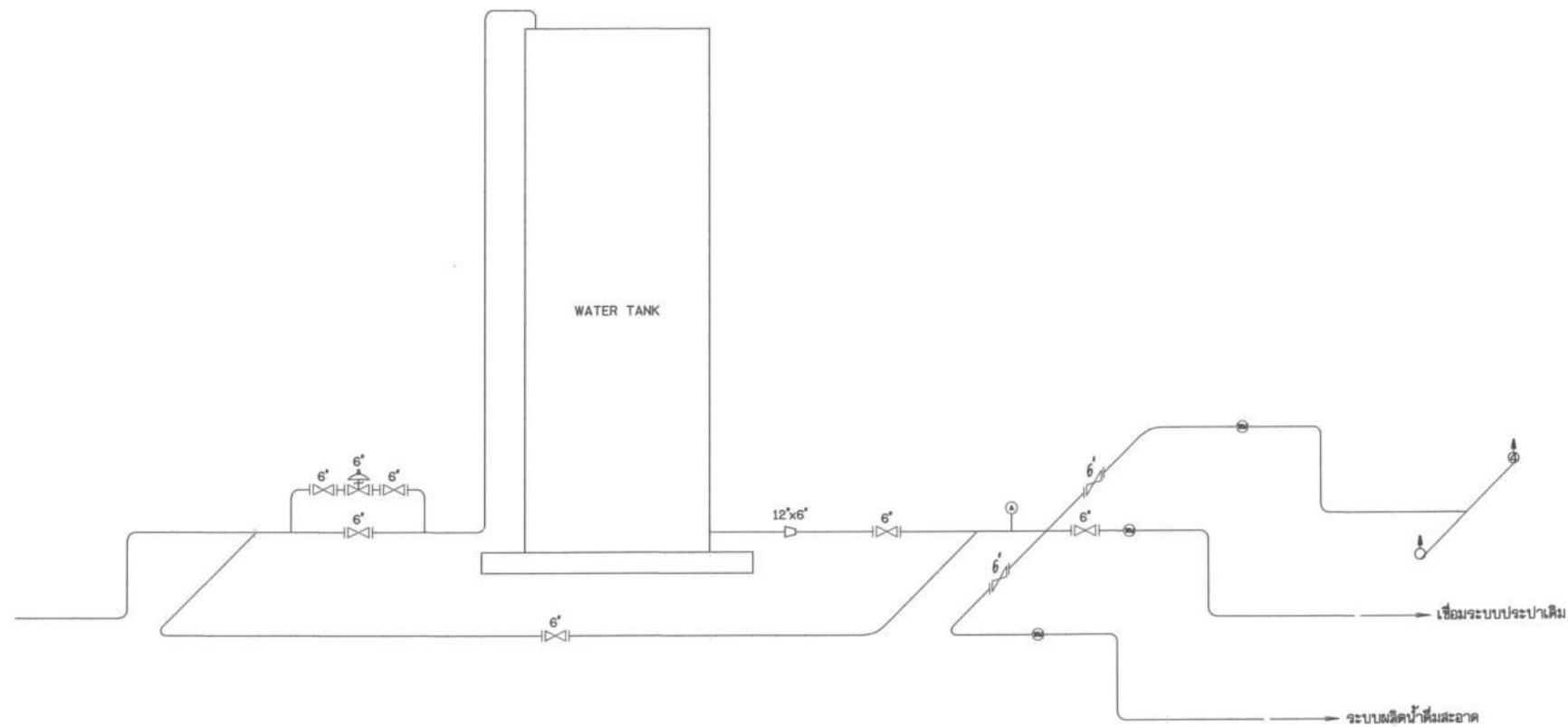
งานประสาณท่อกับถัง FBE ขนาดความจุไม่น้อยกว่า 1,100 ลบ.ม. จุดที่ 1 ไม่แสดงขนาดราส่วน
