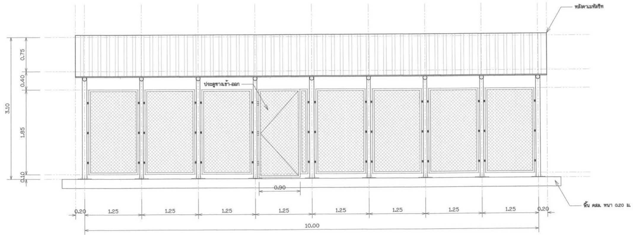
รูปด้าน ①
