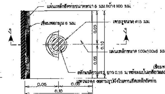
แปลน
