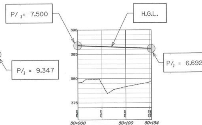
รูปตัดตามแนวยาวแสดง H.G.L. สาย 1R-LMP2 STA. 50+000 - 50+154
