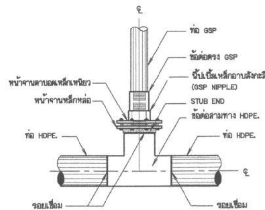
การบรรจบท่อสามทาง HDPE.
