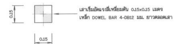
แบบขยายเสาเข็ม
