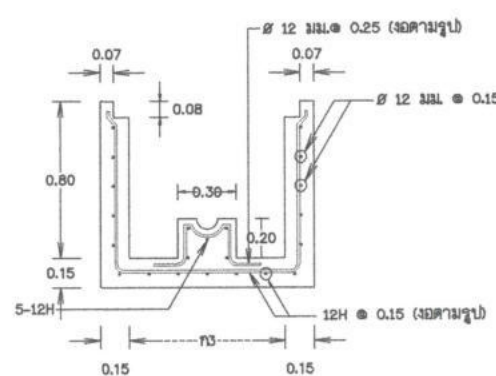
เหล็กเสริมบ่อประตูปรับระดับน้ำ มาตราส่วน 1:20
