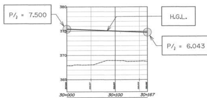
รูปตัดตามแนวยาวแสดง H.G.L. สาย 2R-LMP1 STA. 30+000 - 30+167
