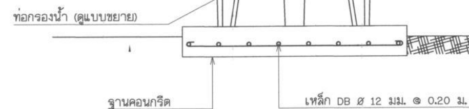
แบบแสดงฐานรากและส่วนประกอบสารกรองถังกรองน้ำ
