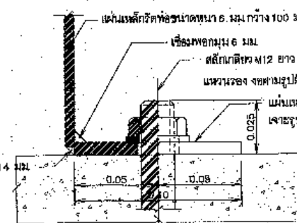
รูปตัด ง-ง
