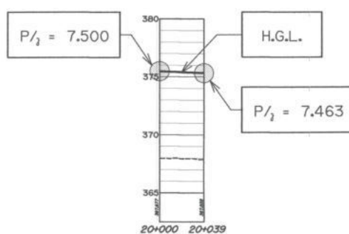
รูปตัดตามแนวยาวแสดง H.G.L. สาย 1R-LMP1 STA. 20+000 - 20+039
