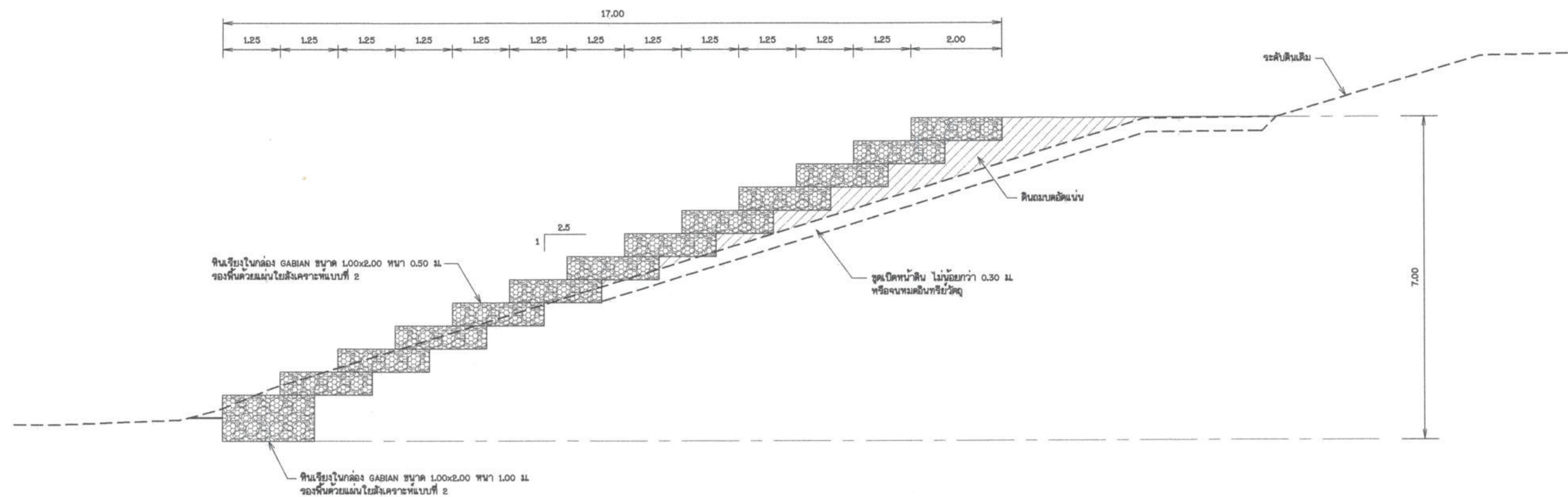
รูปตัดขยายงานป้องกันการกัดเซาะ ไม่แสดงขนาดราส่วน
