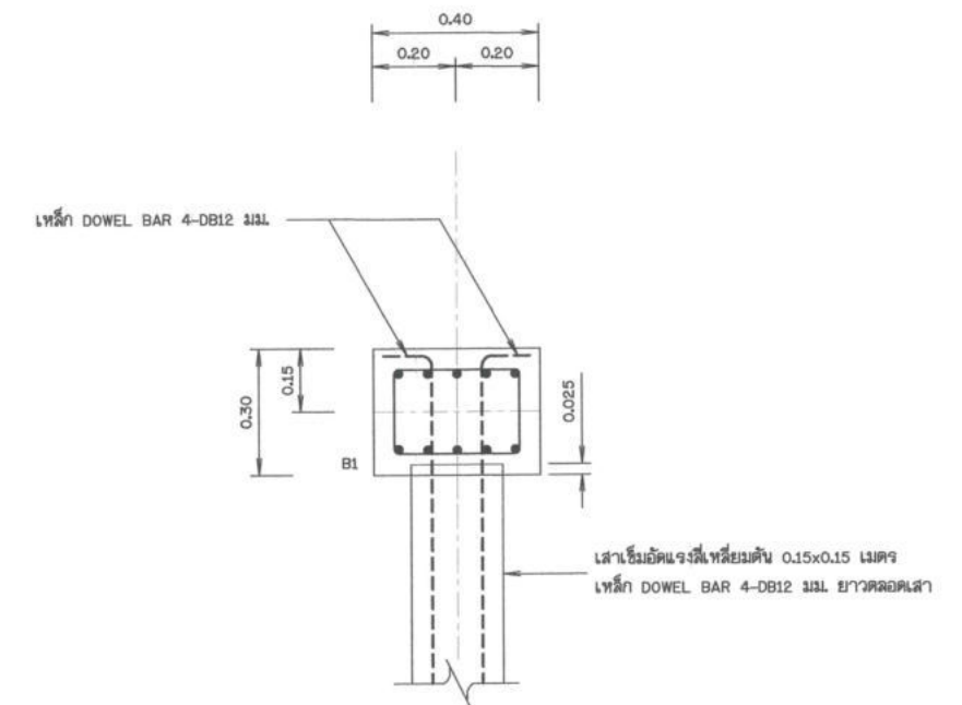
รูปตัด ก1 - ก1
