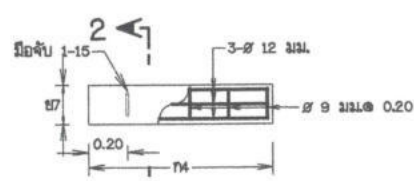
ขยายฝาปิด มาตราส่วน 1:20
