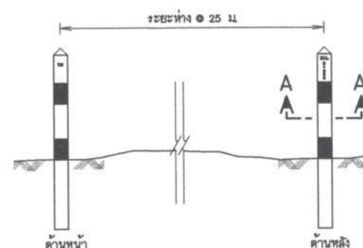
แสดงการวางหลักบ่อแนวท่อ มาตราส่วน 1:20
