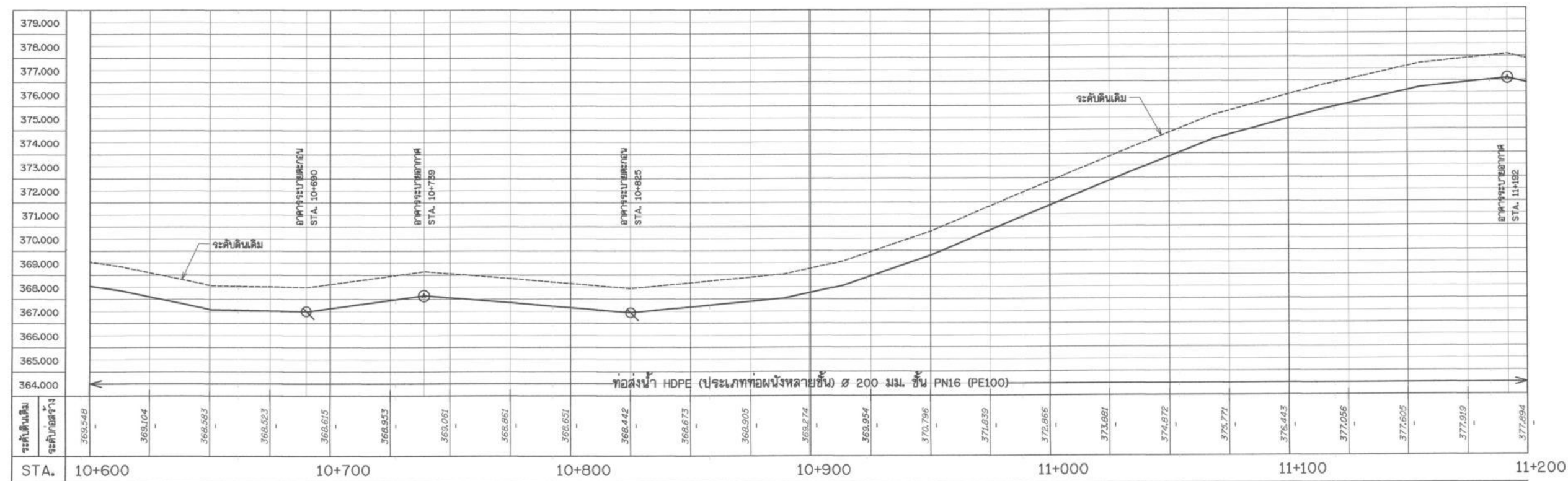
รูปตัดตามแนวยาว สาย LMP2 STA. 10+600 - 11+200 มาตรฐาน : 1:1,000 แนวตั้ง : 1:100
