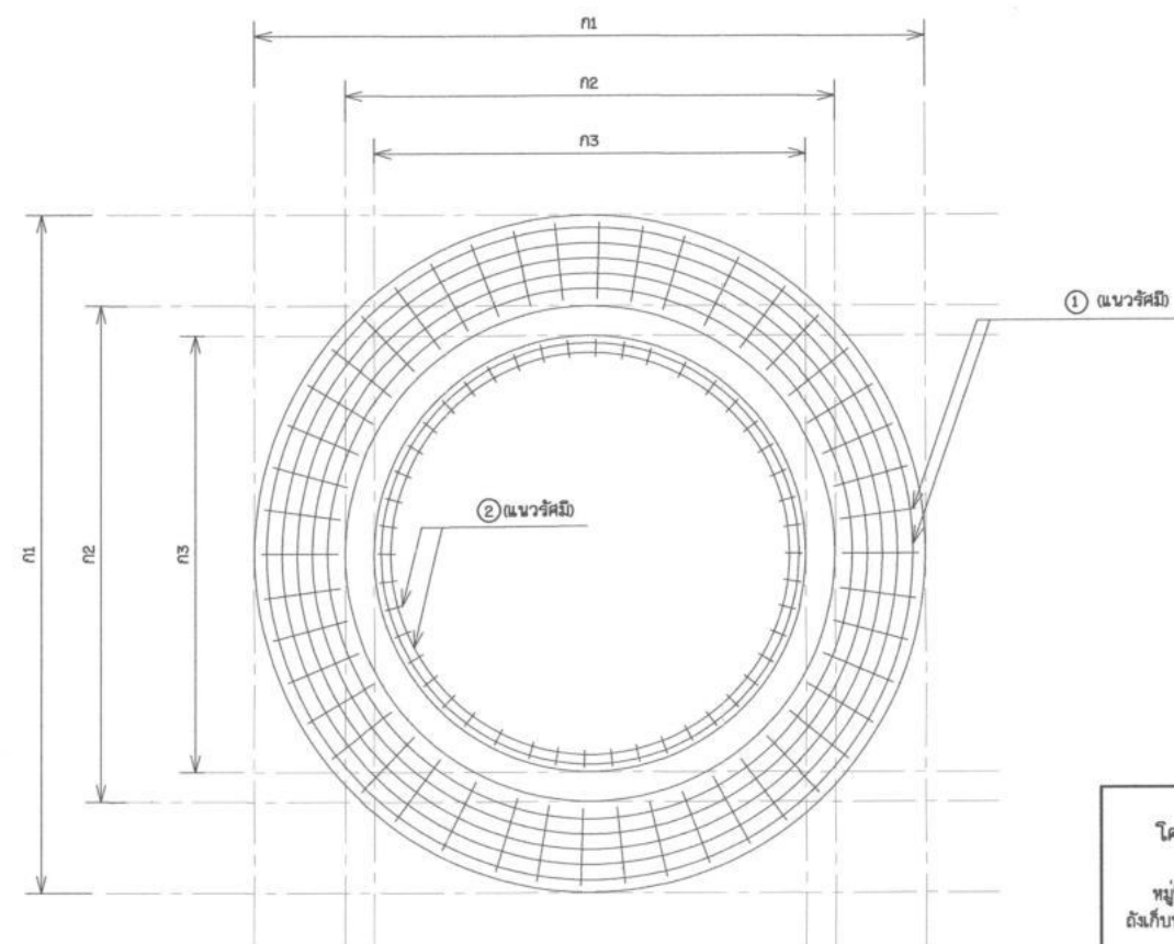
แปลนเหล็กเสริมขอบ รับถังเหล็กเค็ลือบแก้ว มาตราส่วน 1:100
