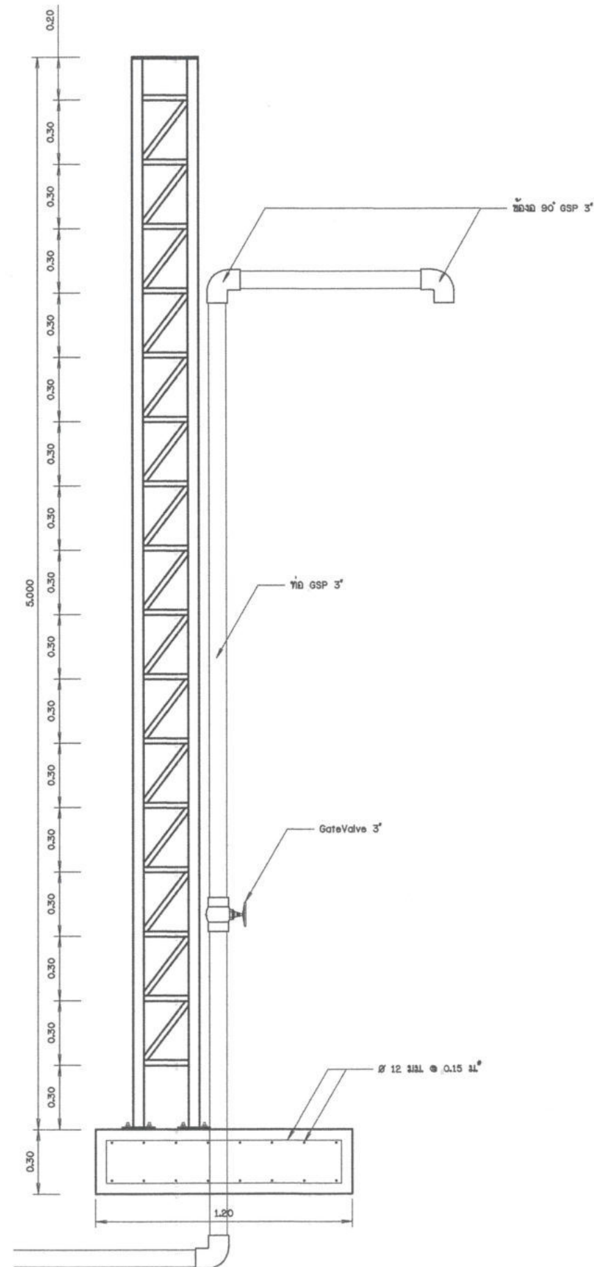
แบบขยายด้านข้าง 1:20
