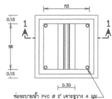
แปลนบ่อประตูปรับระดับน้ำ มาตราส่วน 1:20
