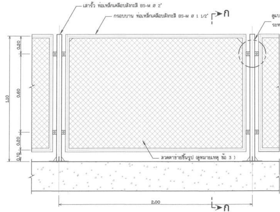
แบบขยายรื้อลวดตาข่าย
