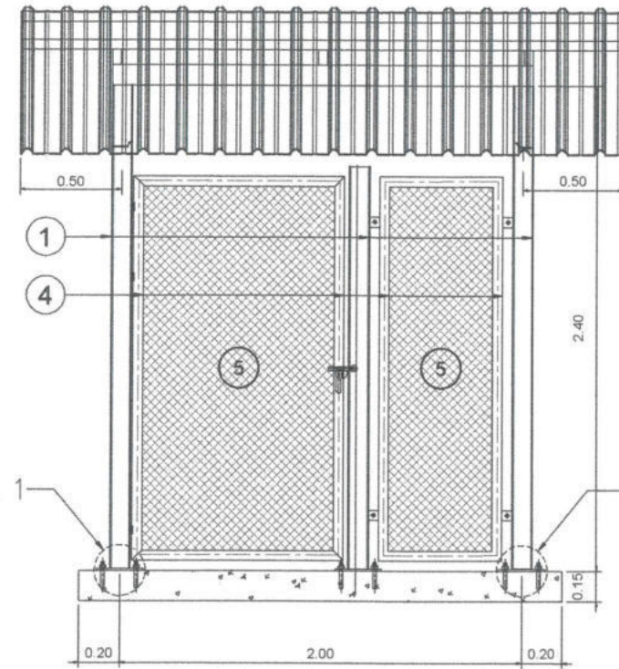
ELEVATION A
