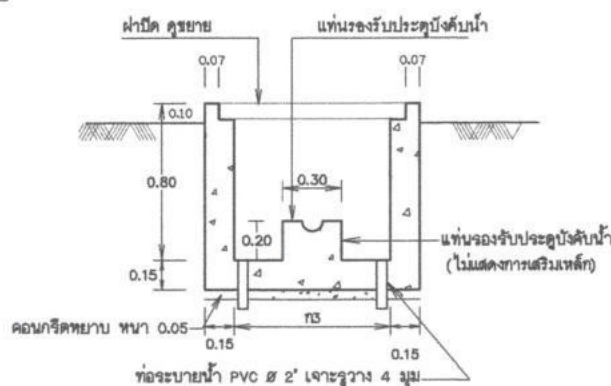
รูปตัด 1 - 1 มาตราส่วน 1:20
