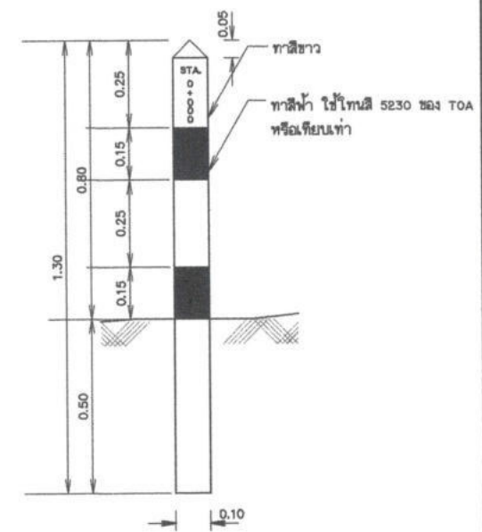
แสดงสัดส่วนหลักบ่อแนวท่อ มาตราส่วน 1:10
