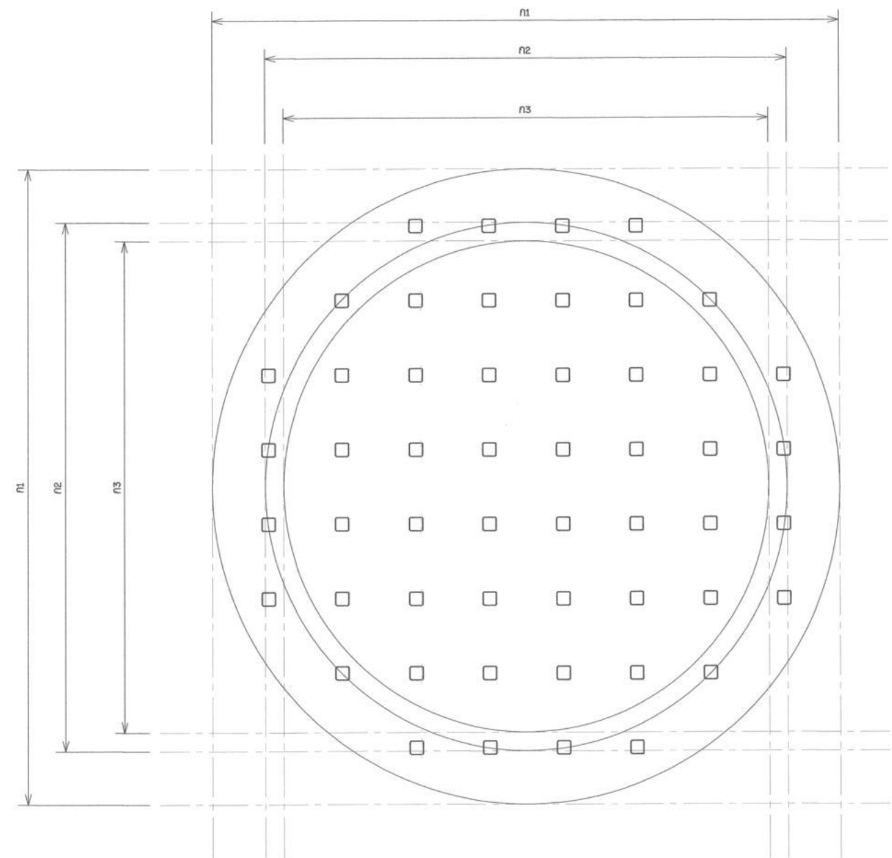
แปลนเสาเข็ม รับถังเหล็กเคลือบแก้วขนาด 1,100 ลบ.ม. มาตราส่วน 1:100
