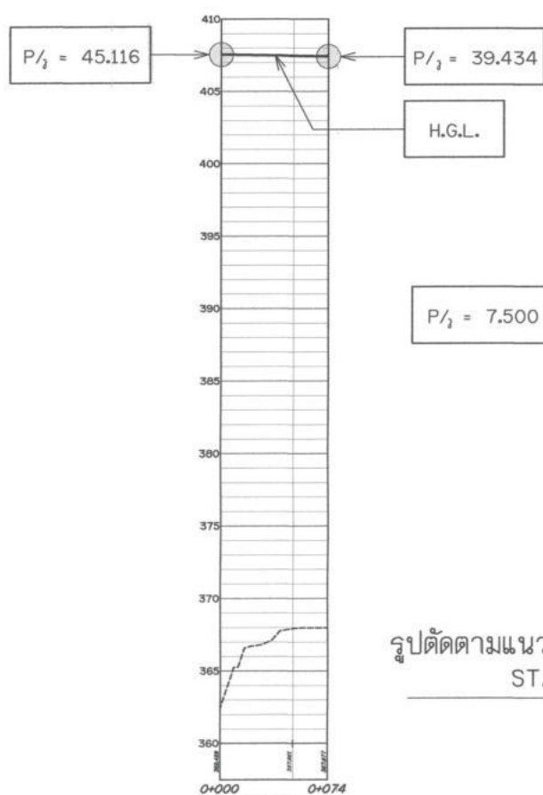
รูปตัดตามแนวยาวแสดง H.G.L. สาย LMP1 STA. 0+000 - 0+074
