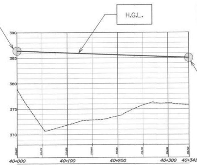
รูปตัดตามแนวยาวแสดง H.G.L. สาย 1L-LMP2 STA. 40+000 - 40+341
