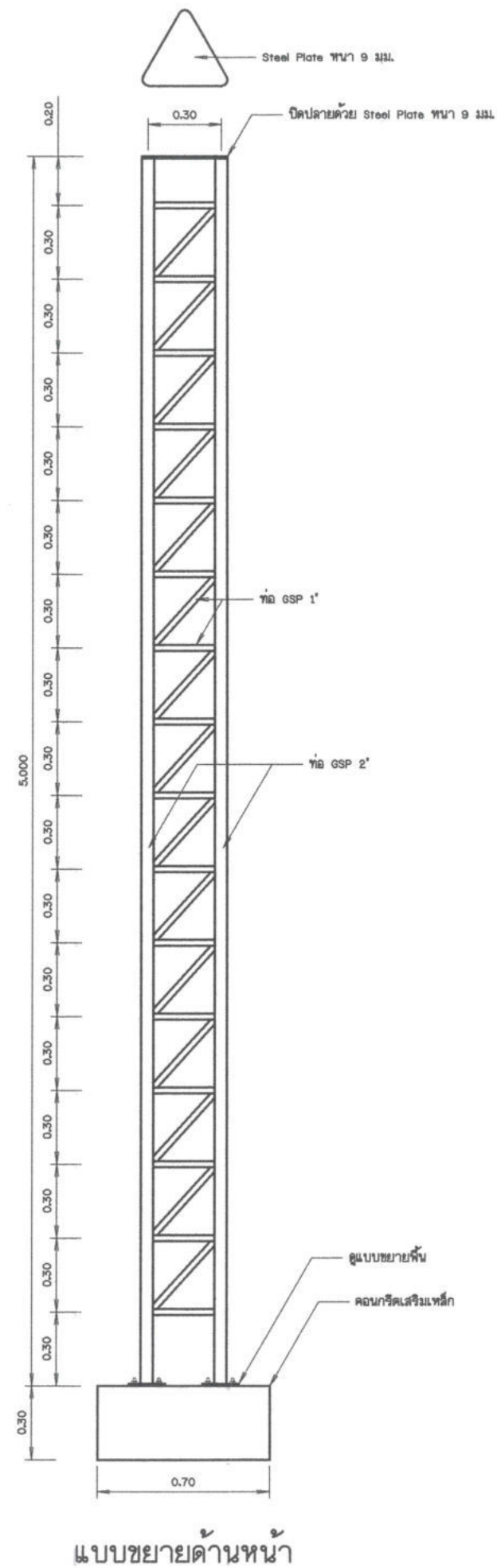
แบบขยายด้านหน้า 1:20
