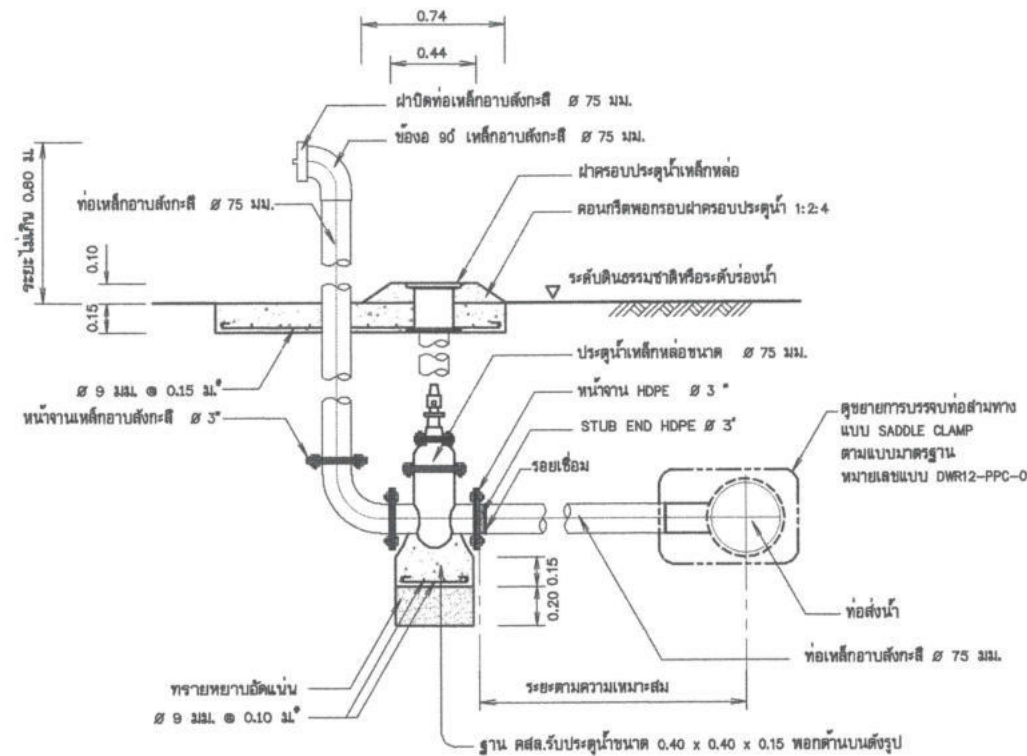
ประตูปรับระดับน้ำขนาด Ø 75 มม. มาตราส่วน 1:20
