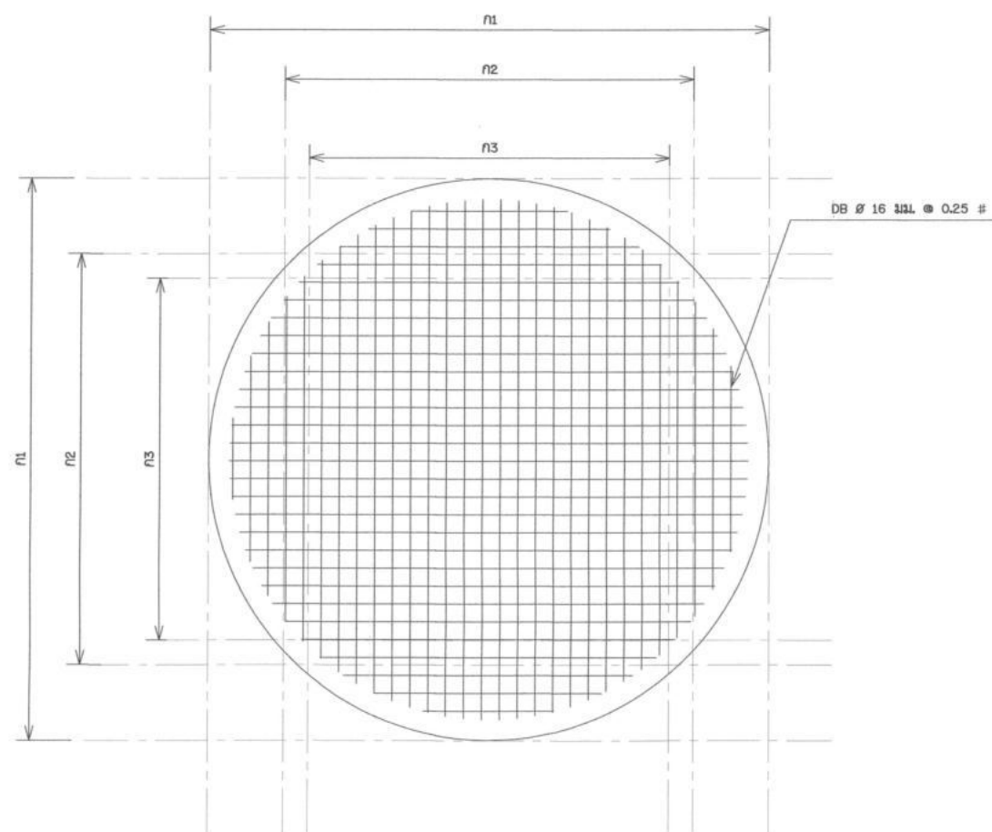
แปลนเหล็กเสริมชั้นบน รับถังเหล็กเค็ลือบแก้ว มาตราส่วน 1:100
