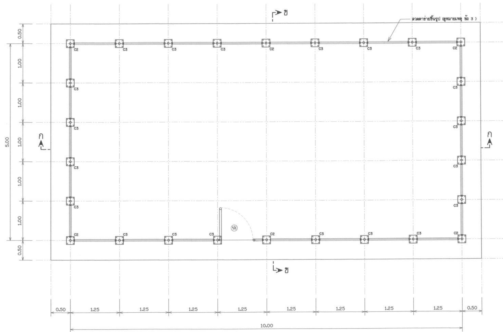
แปลนเสาและรั้ว มาตราส่วน 1:50
