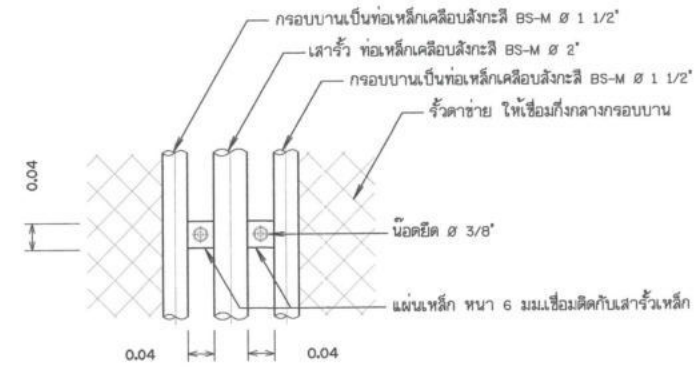
แบบขยายรายละเอียดแสดงการยึดระหว่างรื้อกับเสา
