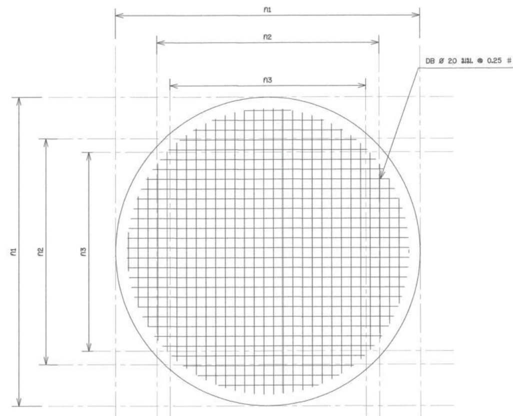
แปลนเหล็กเสริมชั้นล่าง รับถังเหล็กเค็ลือบแก้ว มาตราส่วน 1:100
