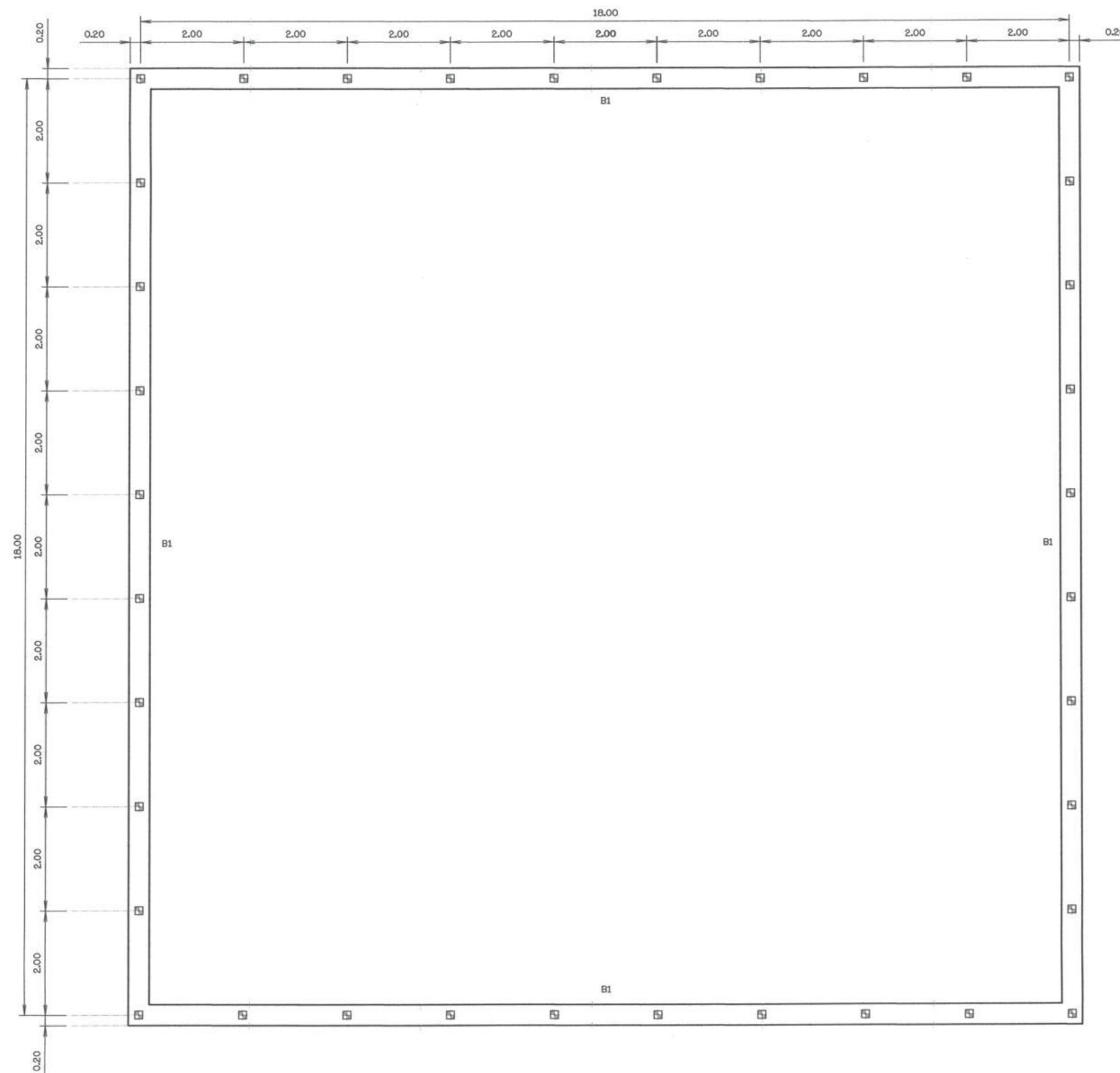
แปลนตำแหน่งเสาเข็ม
