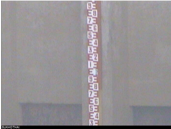
ค่าระดับวิกฤติน้ำแล้ง <45.84 ม.รทก., วิกฤติน้ำท่วม >49.26 ม.รทก. สถานการณ์น้ำ : ปกติ ค่าระดับน้ำปัจจุบัน =46.74 ม.รทก.
