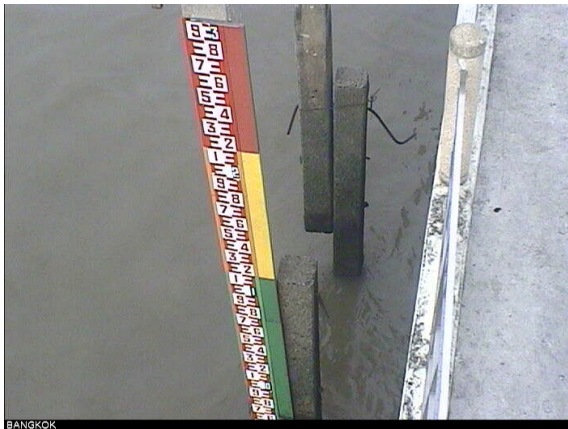
BANGKOK ค่าระดับวิกฤตน้ำแล้ง <0 ม.รทก., วิกฤตน้ำท่วม >2.20 ม.รทก. สถานการณ์น้ำ : ปกติ ค่าระดับน้ำปัจจุบัน =0.5 ม.รทก.
