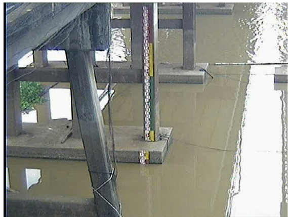
ระดับวิกฤตน้ำแล้ง <15.16 ม.รทก., วิกฤตน้ำท่วม >19.90 ม.รทก. สถานการณ์น้ำ : ปกติ ระดับน้ำปัจจุบัน =16.4 ม.รทก.
