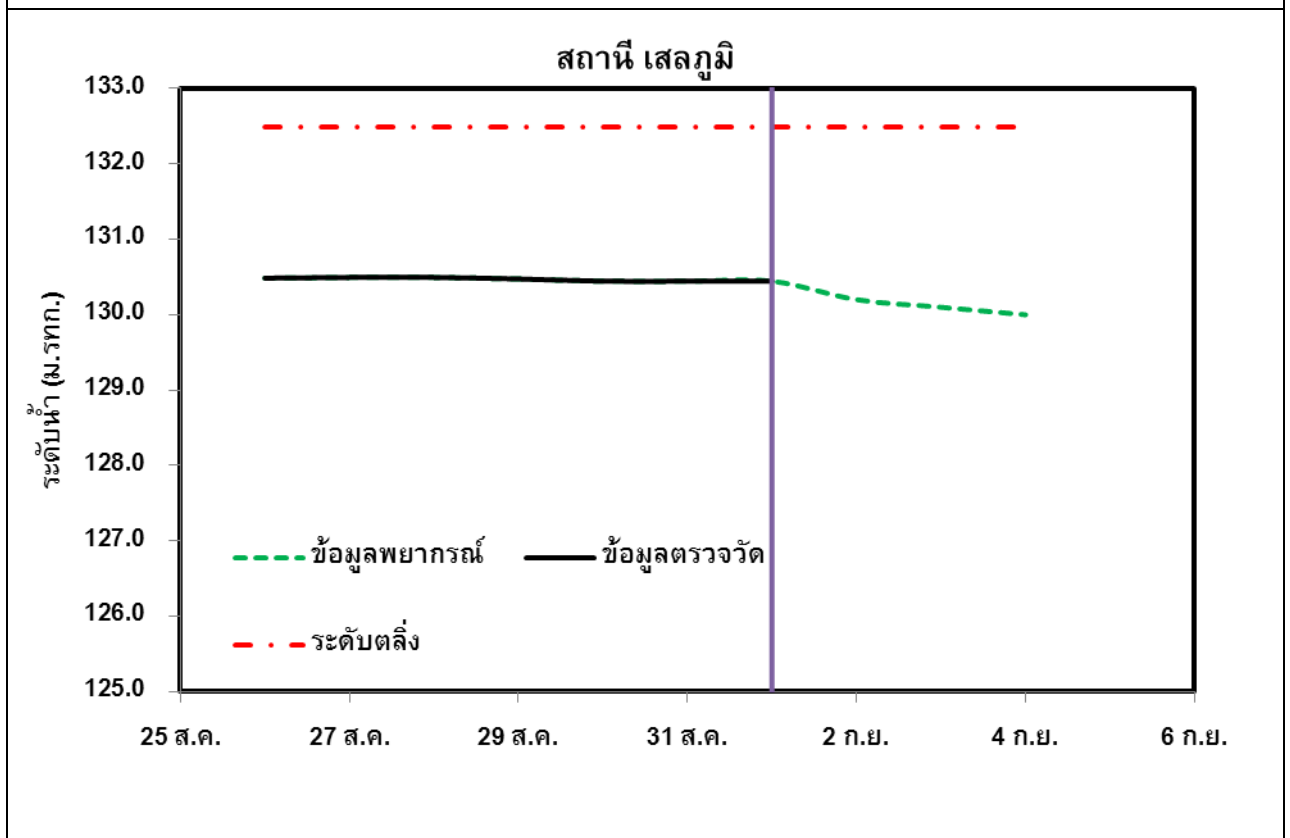
รูปที่ ๔ กราฟการพยากรณ์ระดับน้ำจุดสำคัญในพื้นที่ลุ่มน้ำชี
