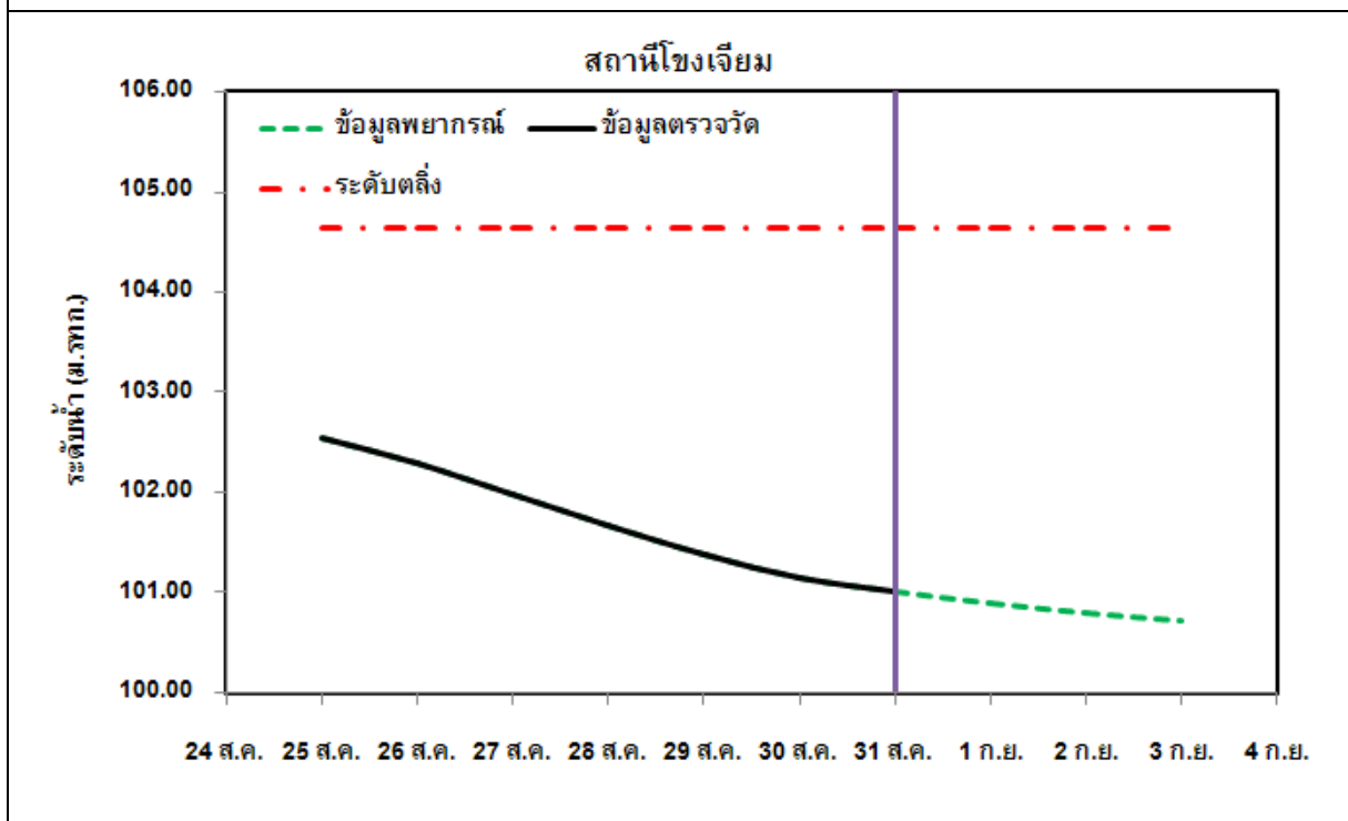
รูปที่ ๒ กราฟการพยากรณ์ระดับน้ำจุดสำคัญในแม่น้ำโขง (ต่อ)
