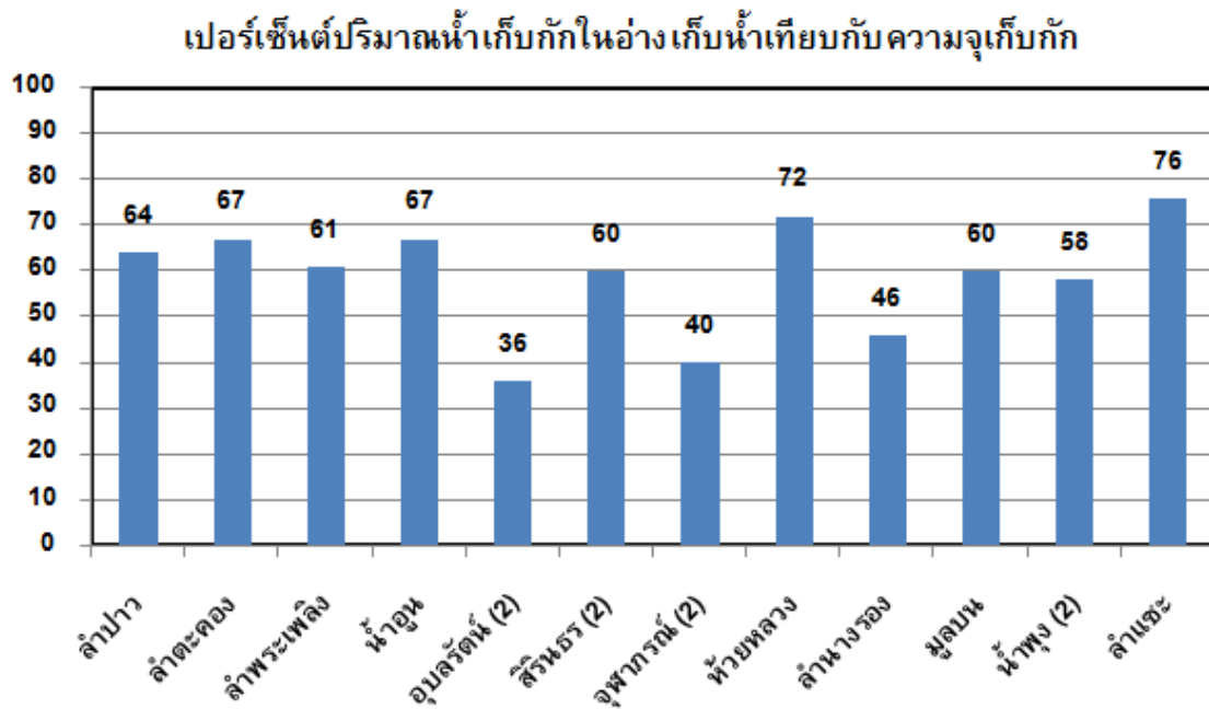
รูปที่ ๑๒ กราฟแสดงเปอร์เซ็นต์ปริมาณน้ำในอ่างเทียบกับความจุเก็บกักของอ่างขนาดใหญ่
