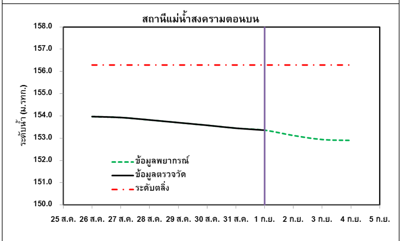
รูปที่ ๓ กราฟการพยากรณ์ระดับน้ำจุดสำคัญในพื้นที่ลุ่มน้ำโขง
