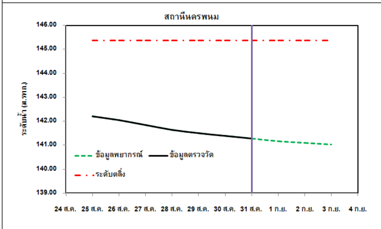
รูปที่ ๒ กราฟการพยากรณ์ระดับน้ำจุดสำคัญในแม่น้ำโขง
