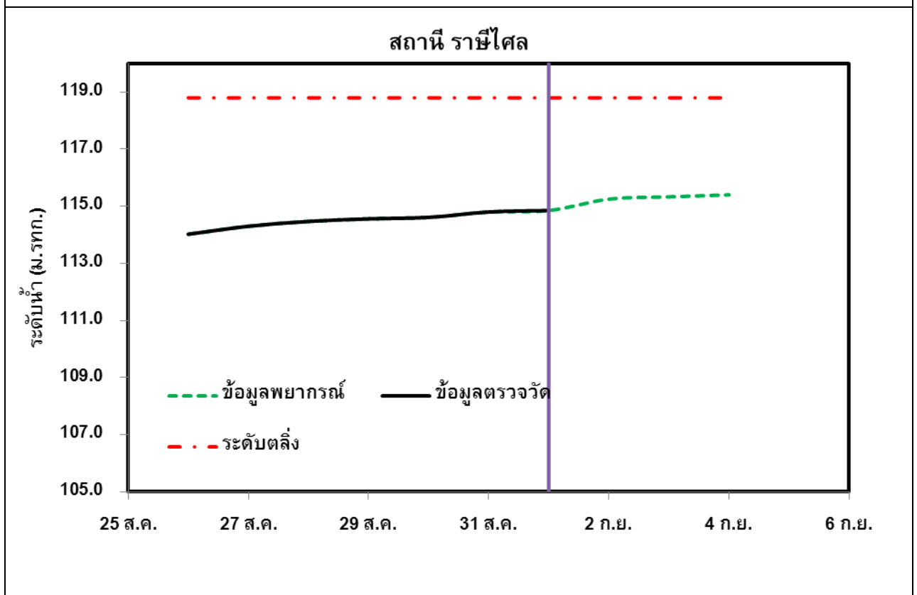
รูปที่ ๕ กราฟการพยากรณ์ระดับน้ำจุดสำคัญในพื้นที่ลุ่มน้ำมูล
