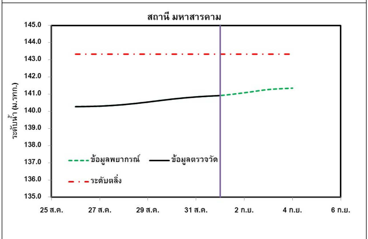
รูปที่ ๔ กราฟการพยากรณ์ระดับน้ำจุดสำคัญในพื้นที่ลุ่มน้ำชี (ต่อ)
