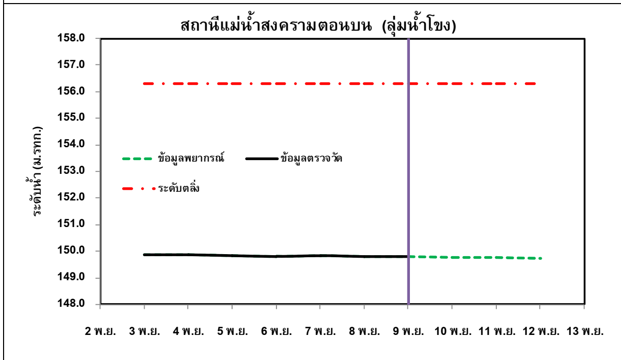
รูปที่ 2 กราฟการพยากรณ์ระดับน้ำจุดสำคัญในพื้นที่ลุ่มน้ำโขง (ต่อ)
