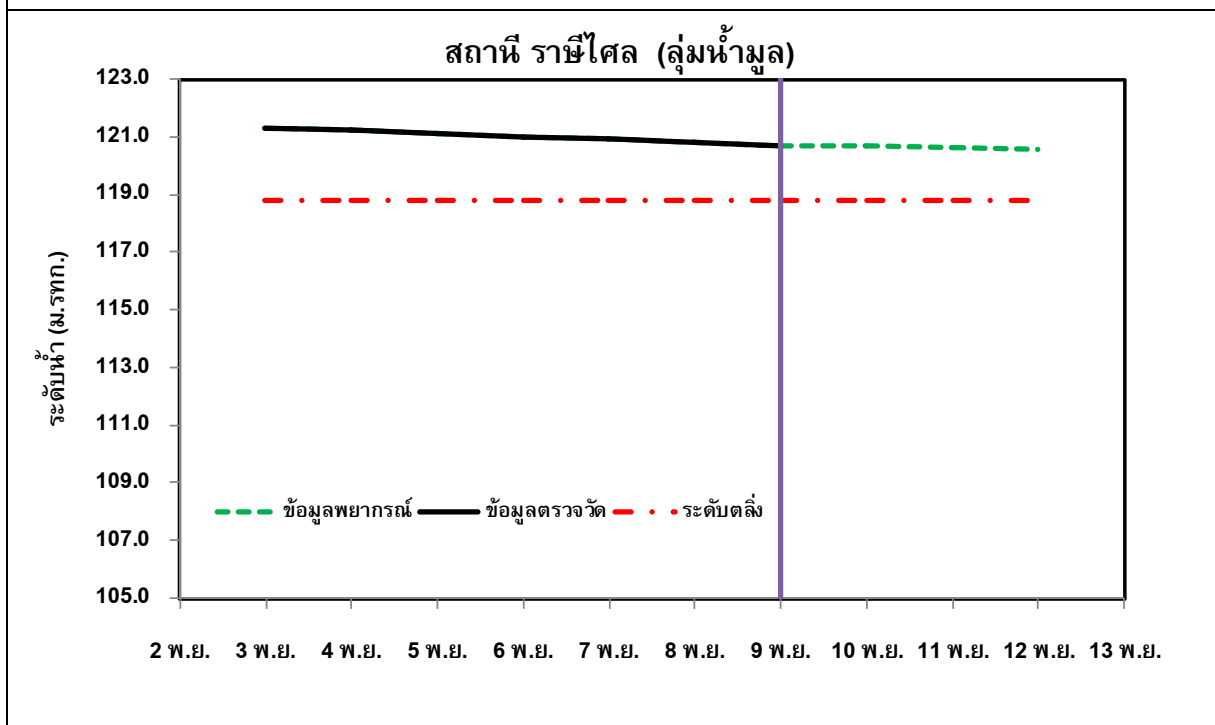
รูปที่ 4 กราฟการพยากรณ์ระดับน้ำจุดสำคัญในพื้นที่ลุ่มน้ำมูล
