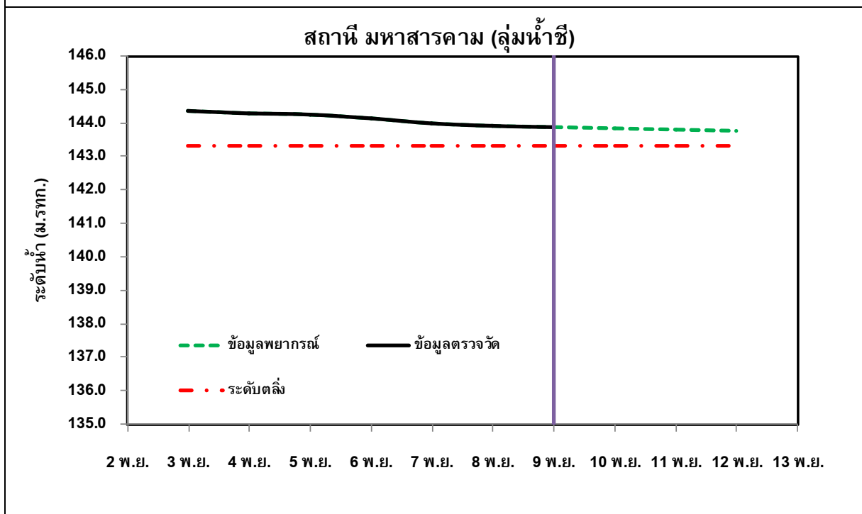
รูปที่ 3 กราฟการพยากรณ์ระดับน้ำจุดสำคัญในพื้นที่ลุ่มน้ำชี (ต่อ)
