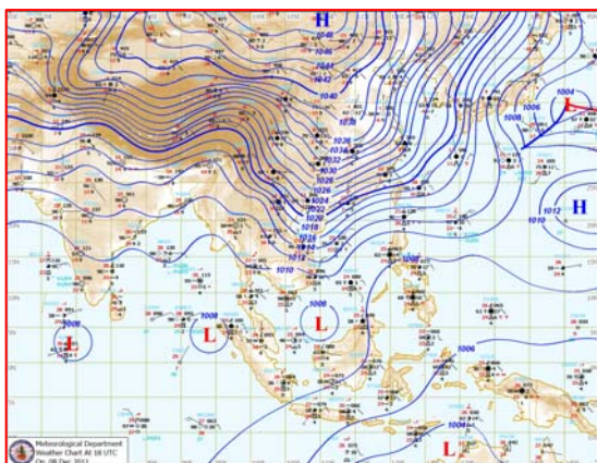
แผนที่อากาศ วันที่ ๙ ธ.ค. ๒๕๕๔ เวลา ๐๑.๐๐ น.
