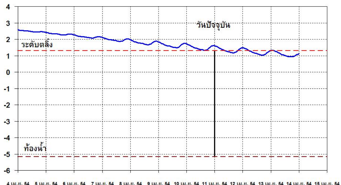
รูปที่ 5-1 แสดงการคาดการณ์ระดับน้ำ ณ จุดฝักระวัง แม่น้ำตาปี ที่สถานี X.5B อ.พุนพิน จ.สุราษฎร์ธานี
