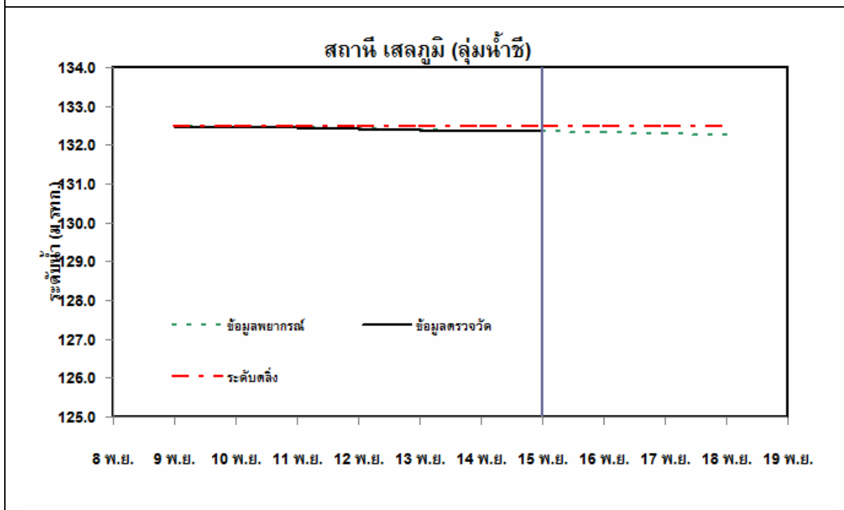
รูปที่ 3 กราฟการพยากรณ์ระดับน้ำจุดสำคัญในพื้นที่ลุ่มน้ำชี
