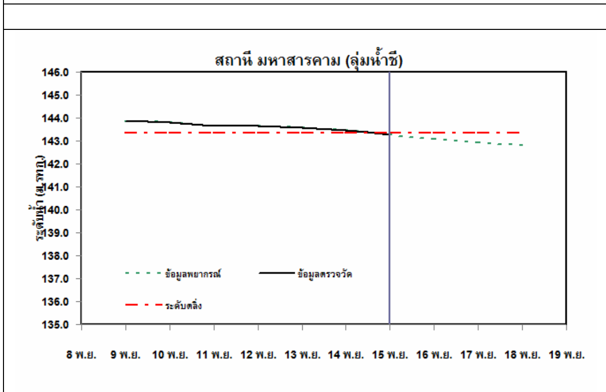
รูปที่ 3 กราฟการพยากรณ์ระดับน้ำจุดสำคัญในพื้นที่ลุ่มน้ำชี (ต่อ)
