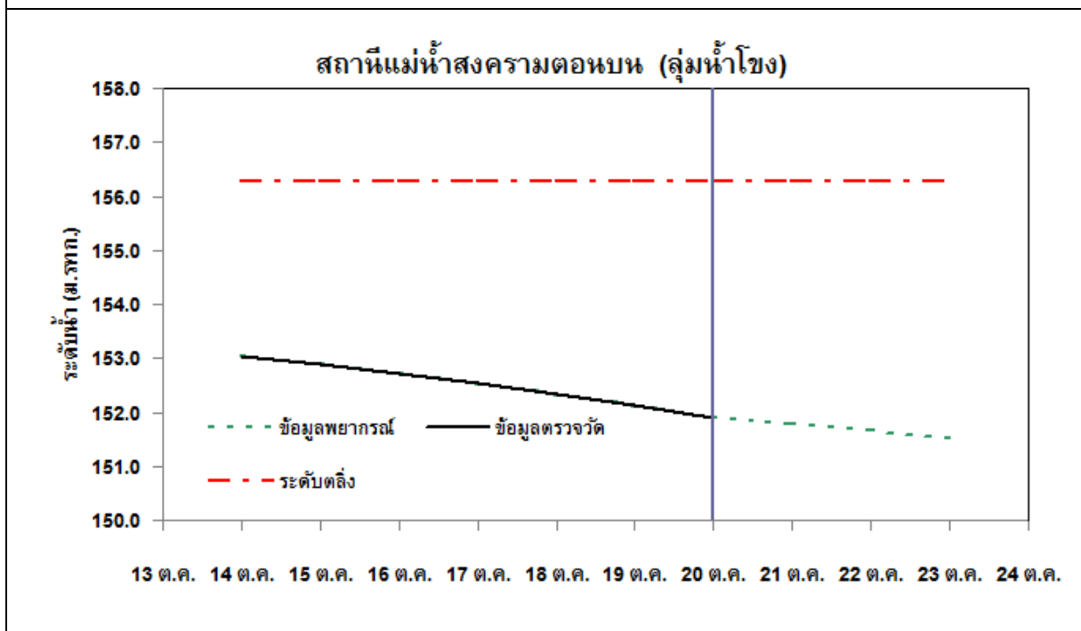
รูปที่ 3 กราฟการพยากรณ์ระดับน้ำจุดสำคัญในพื้นที่ลุ่มน้ำโขง
