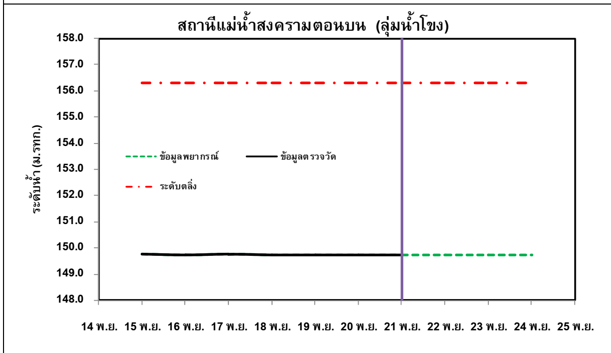
รูปที่ 2 กราฟการพยากรณ์ระดับน้ำจุดสำคัญในพื้นที่ลุ่มน้ำโขง
