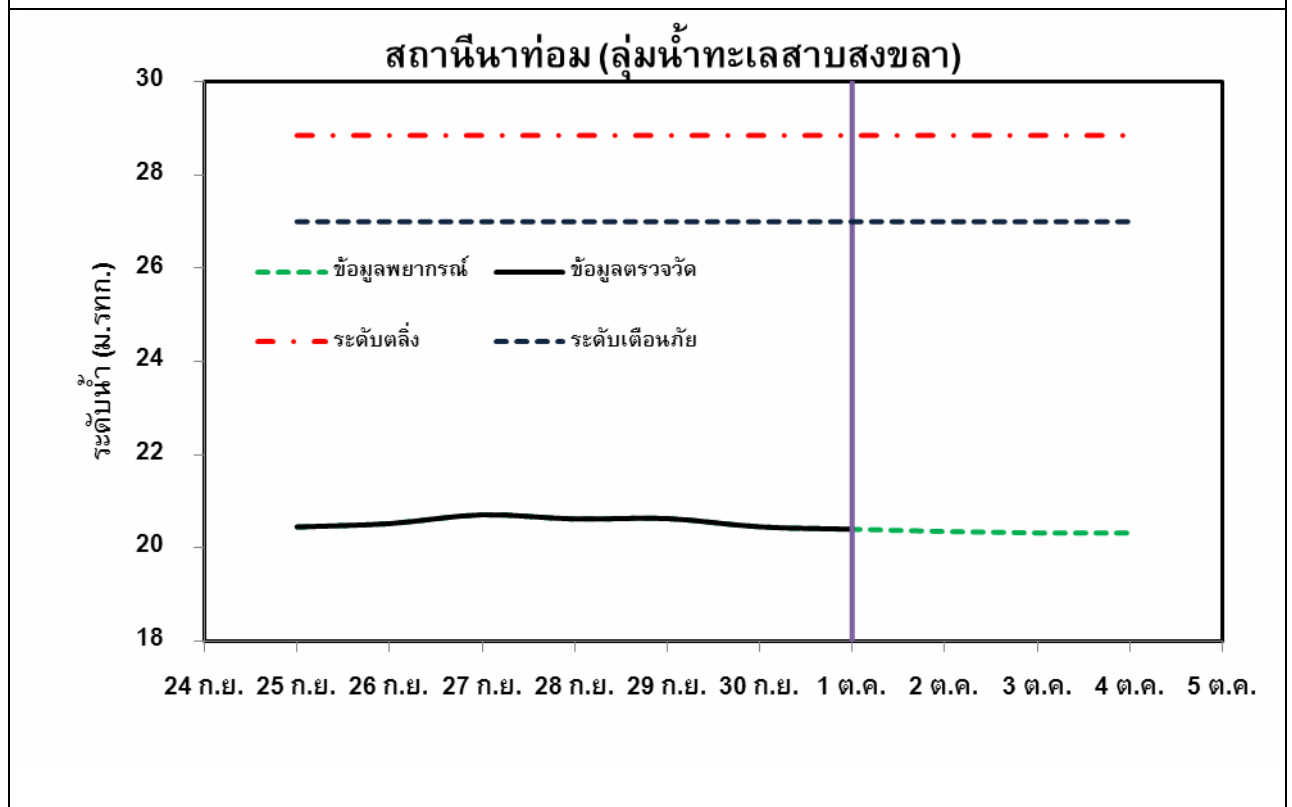
รูปที่ 2 กราฟการพยากรณ์ระดับน้ำจุดสำคัญในพื้นที่ลุ่มน้ำทะเลสาบสงขลา (ต่อ)
