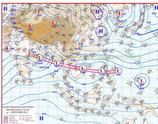
แผนที่อากาศ วันที่ ๕ ก.ย. ๒๕๕๕ เวลา ๐๑.๐๐ น.
