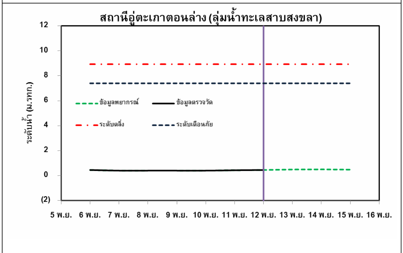
รูปที่ 2 กราฟการพยากรณ์ระดับน้ำจุดสำคัญในพื้นที่ลุ่มน้ำทะเลสาบสงขลา
