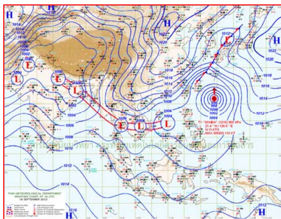
แผนที่อากาศ วันที่ ๑๕ ก.ย. ๒๕๕๕ เวลา ๐๑.๐๐ น.
