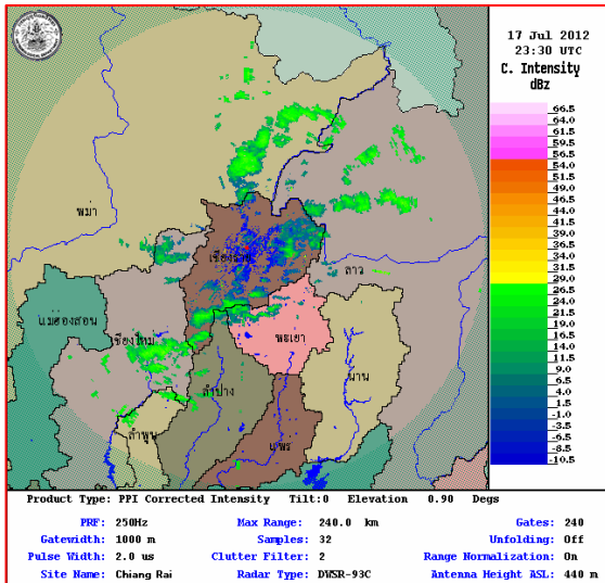
สถานีเชียงใหม่
