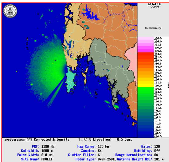
สถานีภูเก็ต
