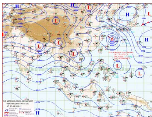
แผนที่อากาศ วันที่ ๑๘ ก.ค. ๒๕๕๕ เวลา ๐๑.๐๐ น.
