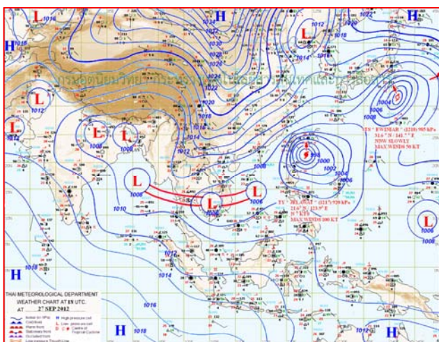
แผนที่อากาศ วันที่ ๒๘ ก.ย. ๒๕๕๕ เวลา ๐๑.๐๐ น.
